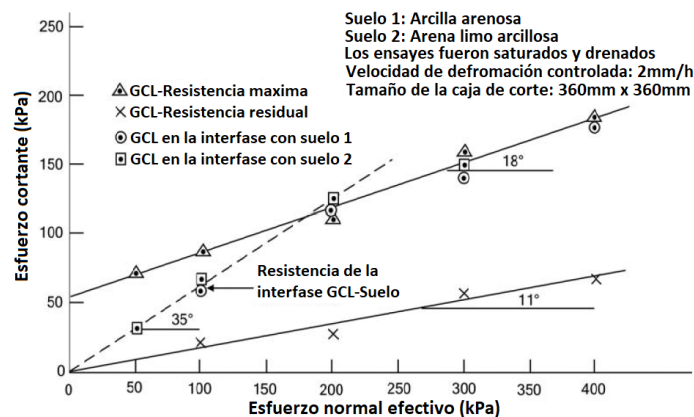
Figura 5.16: Envolventes de resistencia al corte para el núcleo de bentonita GCL e interfases entre GCL y dos suelos (Blight, 2010).
