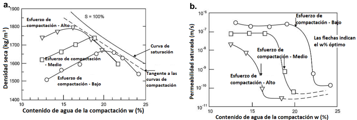
Figura 5.8: Relación entre a) contenido de agua de la compactación y densidad seca, b) permeabilidad y contenido de agua de la compactación (Blight, 2010).
