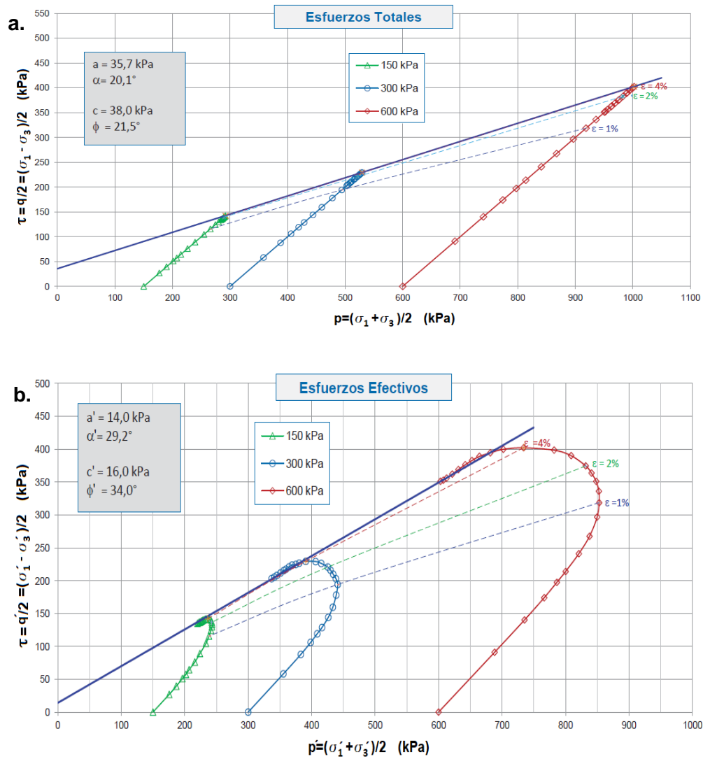
Figura 9.11: Trayectorias en esfuerzos, a) totales y b) efectivos, ensayos de compresión triaxial consolidado no drenado CU (Nyrstar, 2017).
