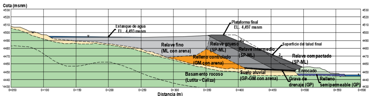
Figura 9.9: Sección geotécnica del depósito de relaves "Oasis".
