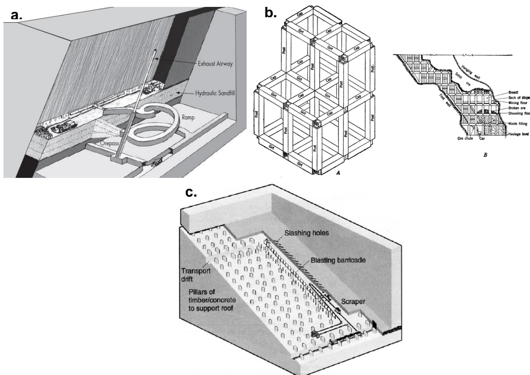
Figura 2.4: Minería a) corte y relleno, b) cuadros conjugados, c) frentes largos y frentes cortos (modificado de SME, 2011).
