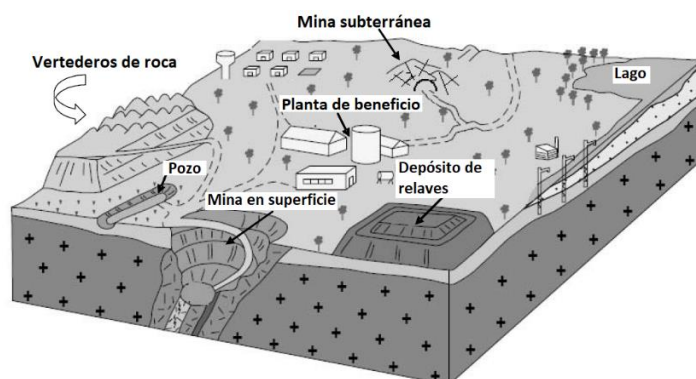
Figura 2.8: Esquema de los componentes en una operación minera (modificado de Yilmaz, 2011).
