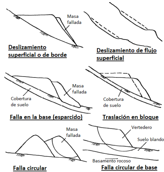
Figura 5.22: Posibles modos de falla en depósitos de roca de desecho (modificado de Robertson, 1999).
