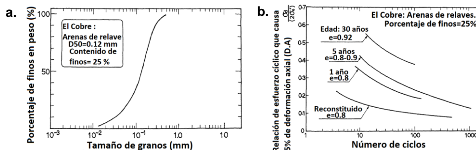
Figura 5.17: a) Curva de gradación de los relaves, b) Curvas de la relación de resistencia cíclica (5% de deformación de doble amplitud) versus el número de ciclos en relaves (finos=25 %) para edades de envejecimiento de 1, 5 y 30 años (Troncoso, Ishihara y Verdugo, 1988).
