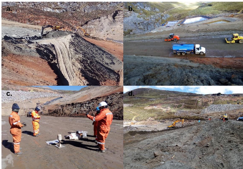
Figura 9.17: a) Trabajos de corte en el talud aguas abajo, b) conformación y compactación de una capa de relleno en un terraplén del dique, c) verificación del grado de compactación, y d) nivelado y perfilado en el talud aguas abajo del depósito (Nyrstar, 2017).
