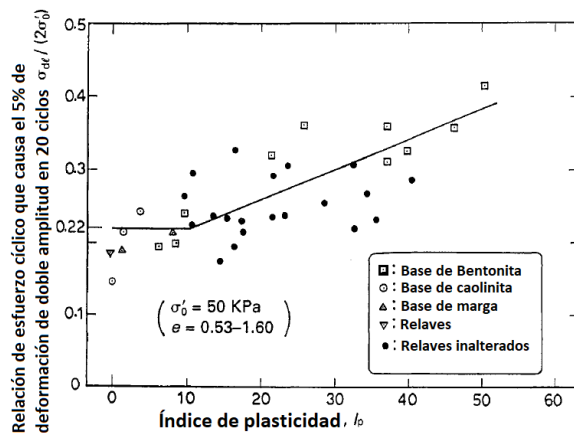
Figura 5.14: Efectos del índice de plasticidad en la resistencia cíclica de arenas con presencia de finos (Ishihara, 1996).
