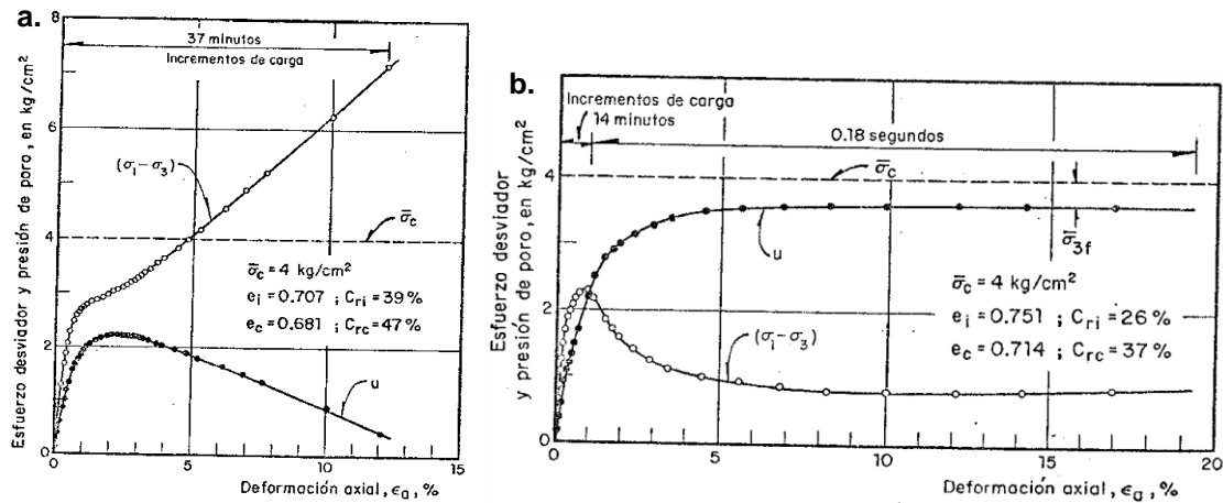
Figura 5.10: Comportamiento de arenas en condiciones no drenadas de un espécimen, a) dilatante y b) contractivo (modificado de Castro, 1969).
