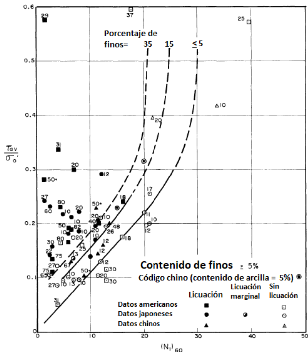
Figura 5.13: Relaciones de resistencia cíclica que causa la licuación y los valores de N_1 para arenas limosas con sismos de magnitud M = 7.5 (Seed et al., 1985).
