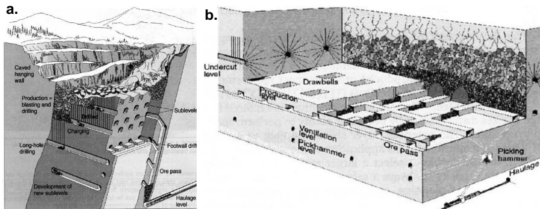
Figura 2.5: Minería, a) sublevel caving y b) block caving (modificado de SME, 2011).
