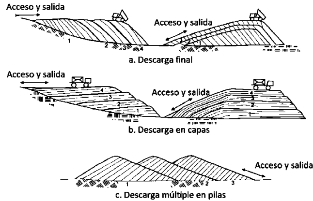
Figura 3.1: Tipos de formas de almacenamiento en vertederos (modificado de Blight, 2010).
