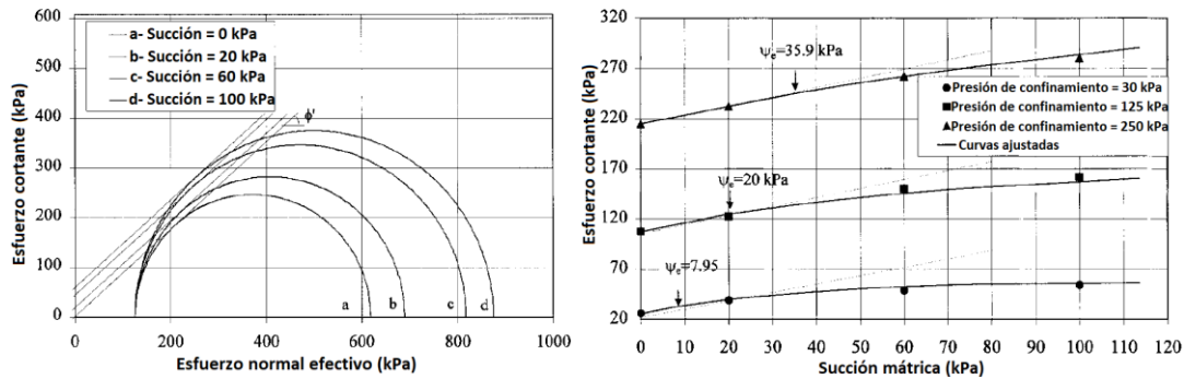
Figura 5.6: Ensayo triaxial consolidado no drenado en un residuo minero granular (Rassam y Williams, 1999).
