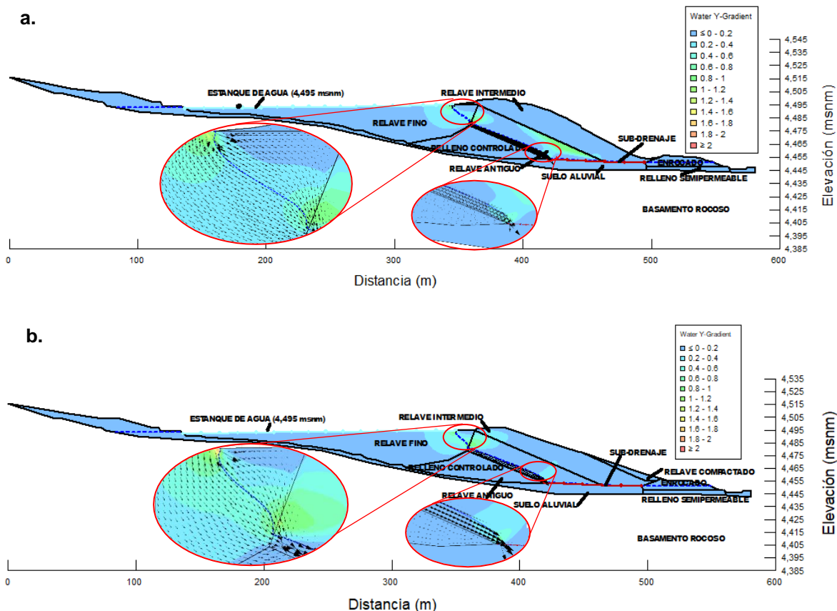
Figura 9.12: Gradientes máximo y de salida en, a) etapa de operación N_v = 4495 msnm y b) etapa de cierre temporal N_v = 4,497 msnm.
