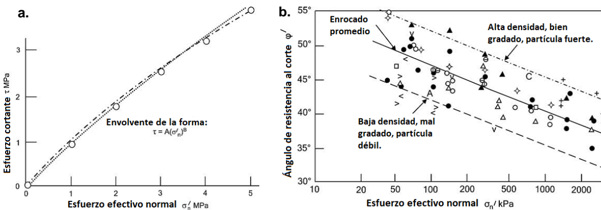
Figura 5.15: a. Ejemplo de envolventes curva para un enrocado a altos esfuerzos, b. Conjunto de valores de \phi' respecto al esfuerzo confinante para determinar la resistencia al corte de rocas estéril de mina (Marsal, 1979; Barton, 2008).
