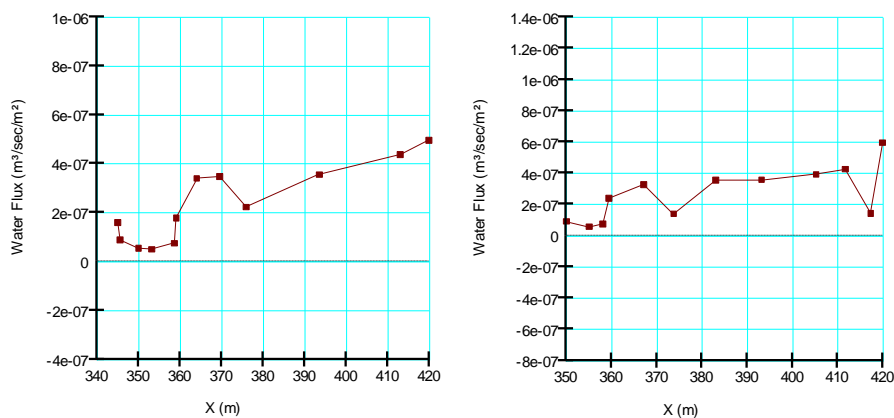
Figura 9.13: Perfiles de velocidad de flujo de agua respecto al eje horizontal, a) etapa de operación N_v = 4,497 msnm, b) etapa de cierre temporal N_v = 4,499 msnm.
