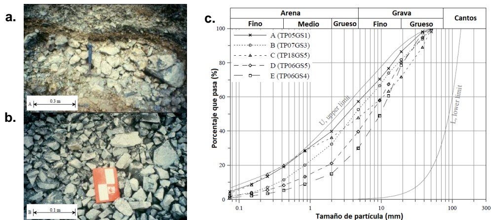
Figura 5.3: Estructura interna de la roca de desecho en un vertedero, a) material en estrato, b) material nuevo superficial, y c) curvas de distribución granulométrica de rocas de desecho (Herasymuik, 2006).
