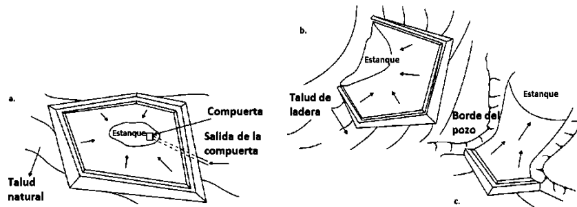
Figura 3.3: Formas de embalse para almacenamiento de residuos, a) Dique tipo anillo, b) Dique tipo valle cruzado y c) Pozo existente en cierre (modificado de Blight, 2010).
