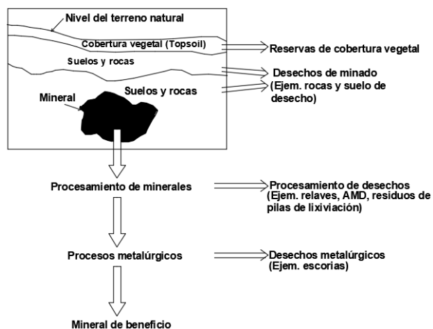
Figura 2.9: Flujo esquemático de productos y residuos en una explotación minera (modificado Lottermoser, 2010).
