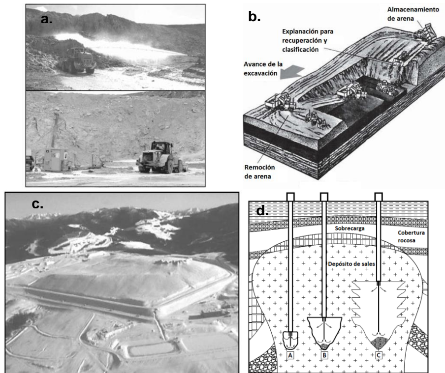
Figura 2.2: a) hidráulica, b) de placeres, c) pilas de lixiviación y d) con disoluciones (modificado de SME, 2011).
