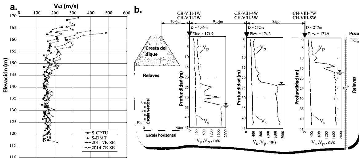
Figura 5.1: a) Perfiles de velocidad de onda de corte de relaves obtenidos a partir de la prueba de cross-hole, S-DMT y S-CPTU. b) Ubicación de la profundidad de saturación a partir de mediciones de V_p y V_s de un depósito de relaves de cobre en Polonia (Jamiolkowski y Masella 2014).
