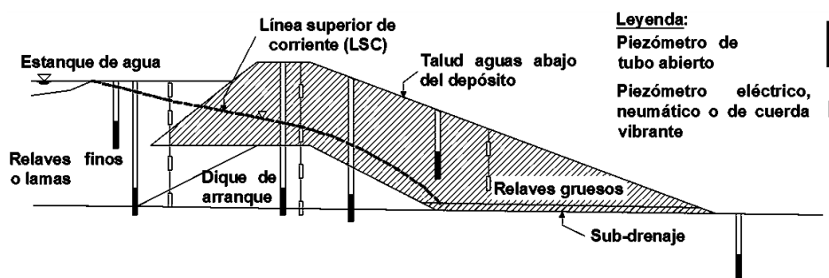
Figura 7.3: Sección de un esquema de monitoreo piezométrico en un depósito construido con el método del eje central.
