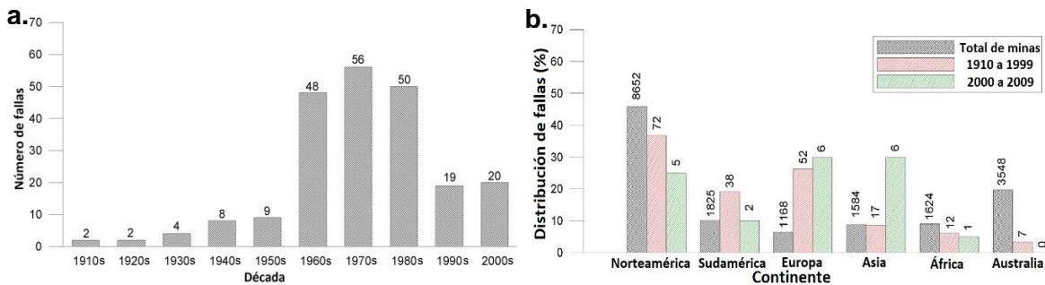
Figura 6.3: a) Fallas registradas en el tiempo, b) distribución de fallas por región (Azam y Li, 2010).
