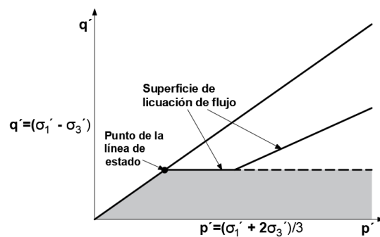
Figura 5.11: Zonas de susceptibilidad a flujo por licuación y movilidad cíclica (modificado de Kramer, 1996).
