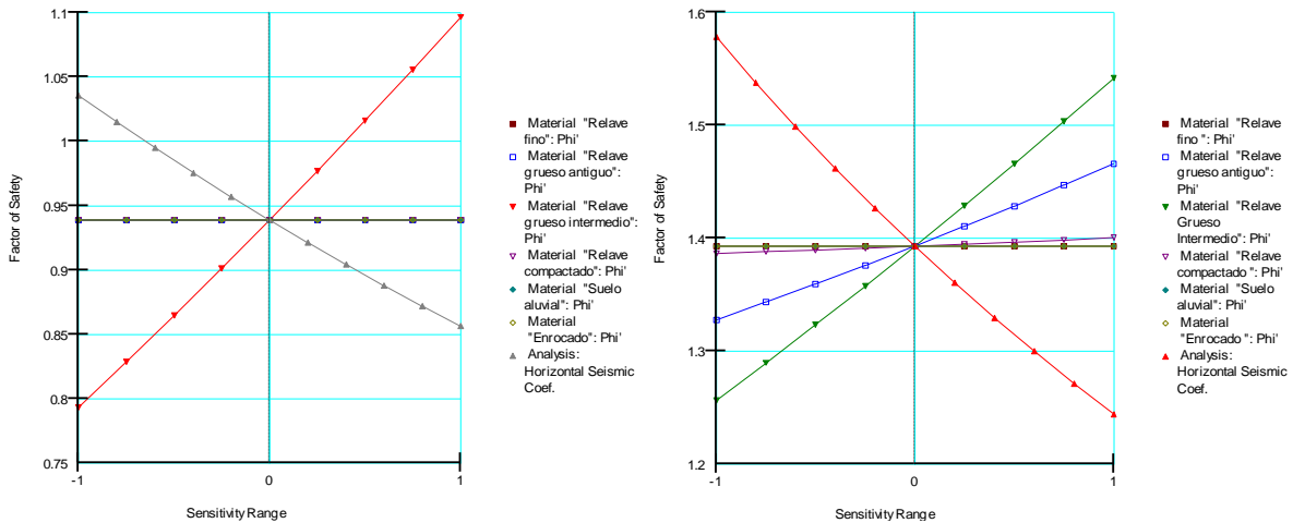
Figura 9.16: Factores de seguridad obtenido del análisis de sensibilidad para la condición con sismo, a) etapa de operación N_v=4,499 y b) etapa de cierre temporal N_v= 4,497 .
