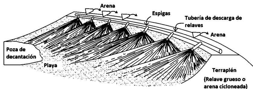
Figura 3.8: Descarga con espigas de arenas de relave en un depósito (Valenzuela, 2016).
