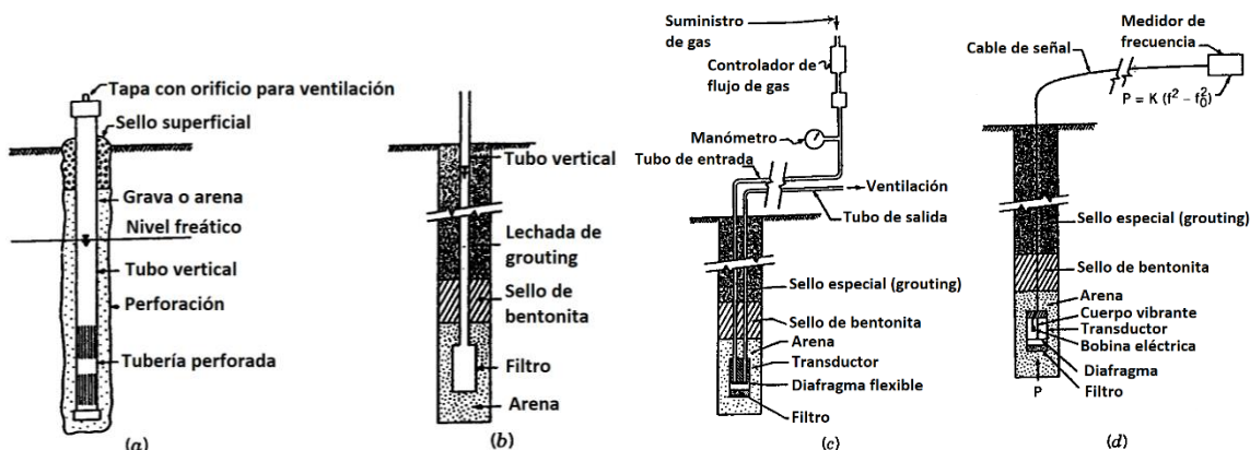
Figura 7.2: Piezómetros, a) Pozos de observación, b) Tubo abierto, c) Neumático y d) Cuerda vibrante (Abramson et al., 2002).
