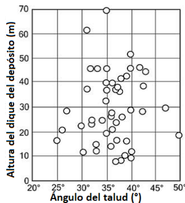
Figura 5.7: Relación entre el ángulo medio del talud externo y la altura para 46 depósitos estables de relaves de oro en una zona semiárida de África (modificado de Blight, 2010).
