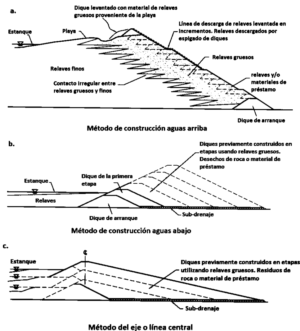
Figura 3.6: Métodos de construcción de depósitos de residuos mineros tipo relaves (Martin et al. 2002).
