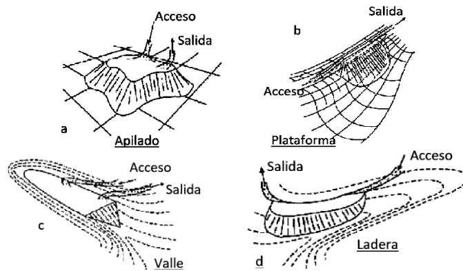
Figura 3.2: Tipos de vertederos de residuos definidos por la topografía, a) apilado, b) plataforma, c) valle y d) ladera (modificado de Blight, 2010).
