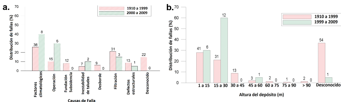
Figura 6.1: a) Distribución de fallas por causa, b) Distribución de fallas por altura de depósito (Azam y Li, 2010).
