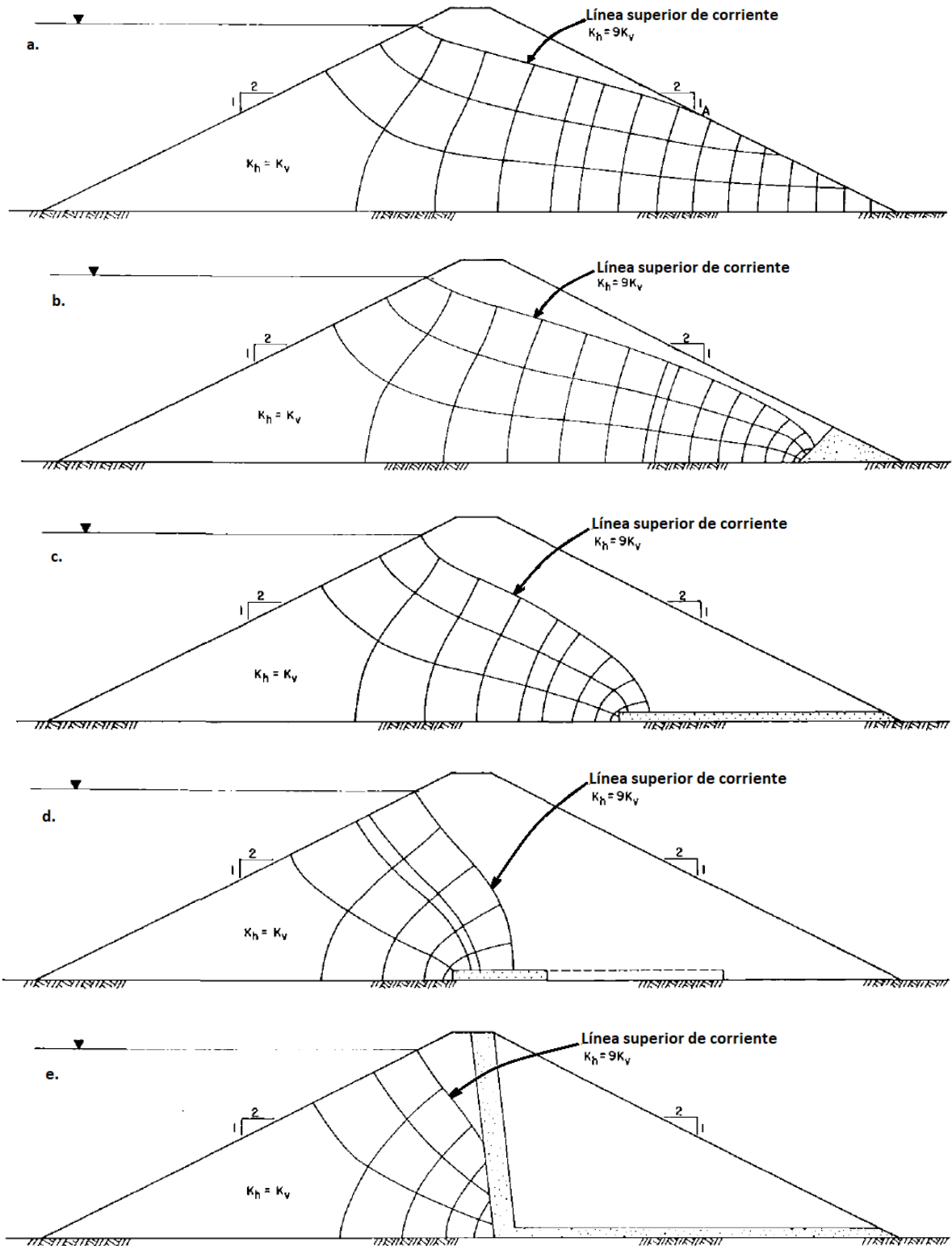
Figura 5.19: Red de flujo en una presa homogénea a) sin drenaje, b) con drenaje al pie de talud, c) con drenaje tipo capa drenante (dren blanket), d) con drenaje en bandas y e) con dren inclinado (modificado de Klohn, 1979).
