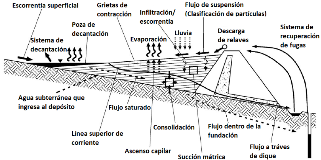
Figura 5.18: Esquema de un depósito de relaves convencional en el cual se indica los factores y fenómenos involucrados en su operación (modificado de Zandarín et al., 2008).
