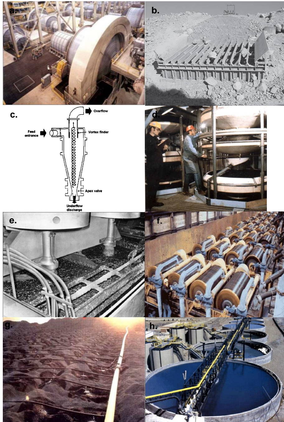
Figura 2.7: a) molinos en etapa de operación, b) cribado estático, c) hidrociclón, d) cono Reichert, e) celda de flotación mecánica, f) separadores de tambor de baja intensidad, g) pila de lixiviación, y h) espesador continuo (SME, European comission, 2004).
