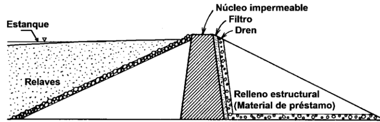
Figura 3.7: Métodos de construcción tipo presa de almacenamiento de agua (modificado de USEPA, 1994).
