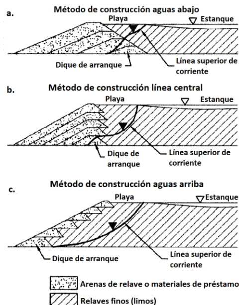
Figura 5.23: Variación de la línea superior de corriente respecto a los métodos de construcción en depósitos de relaves (modificado de Castro, 2003).
