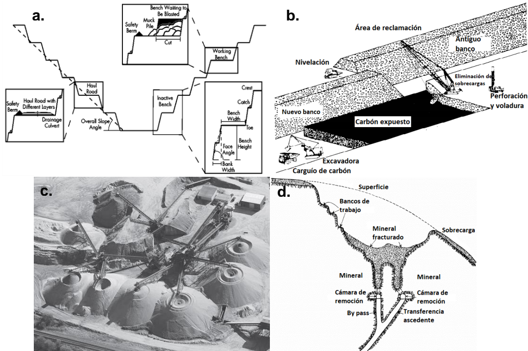
Figura 2.1: a) cielo abierto, b) cielo abierto por frentes, c) cantera y d) glory hole (modificado de SME, 2011).
