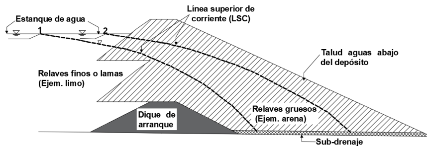
Figura 5.20: Efecto de la ubicación de los estanques de agua en la formación de la línea superior de corriente (LSC) en un depósito de relaves construido por el método de línea central (modificado de Kossov et al., 2014).
