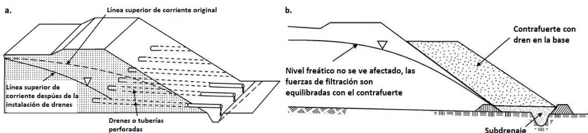
Figura 5.21: Métodos para mejorar el drenaje en taludes, a) drenes perforados y b) adición de contrafuertes con drenajes en la base (modificado de Abramson et al., 2002).
