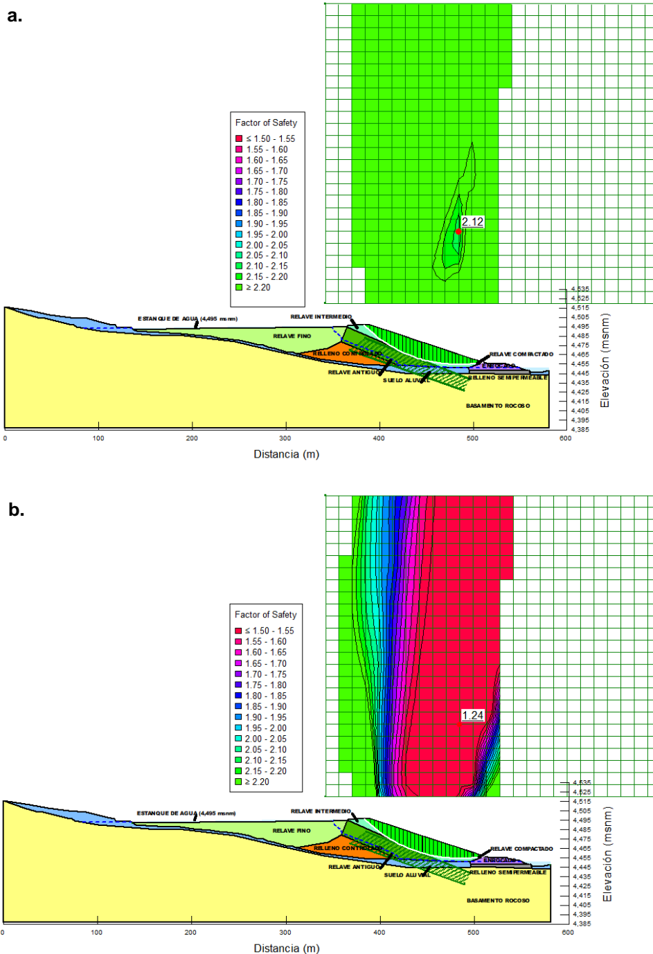
Figura 9.15: Factores de seguridad en la etapa de cierre temporal N_v = 4497 , a) condición estática y b) condición con sismo.
