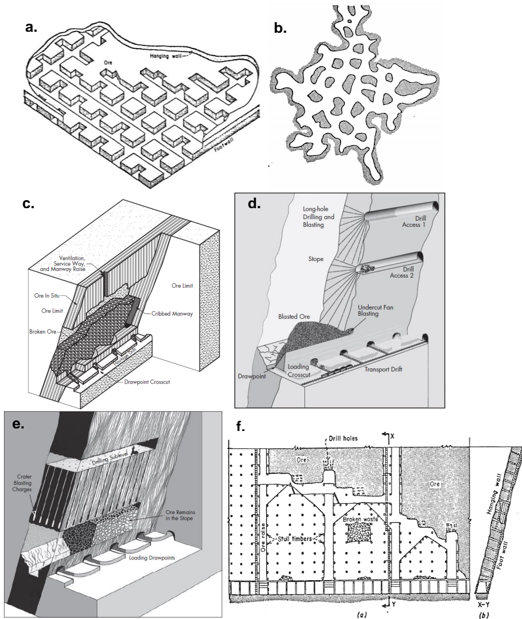
Figura 2.3: a) Cámaras y pilares, b) pilares, c) cámaras almacén, d) subniveles, e) gradas de retroceso vertical, y f) stull stopping. (Jackson y Gardner, 1936, SME, 2011).
