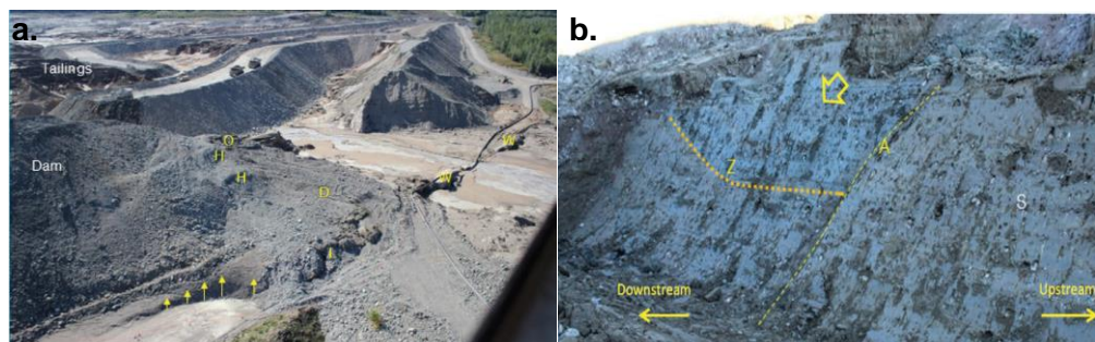
Figura 6.5: Mount Polley en Canadá en el año 2014, a) Falla en la cimentación, b) Superficie de corte en el núcleo del dique remanente (Morgenstern, Vick y Van Zyl, 2015).
