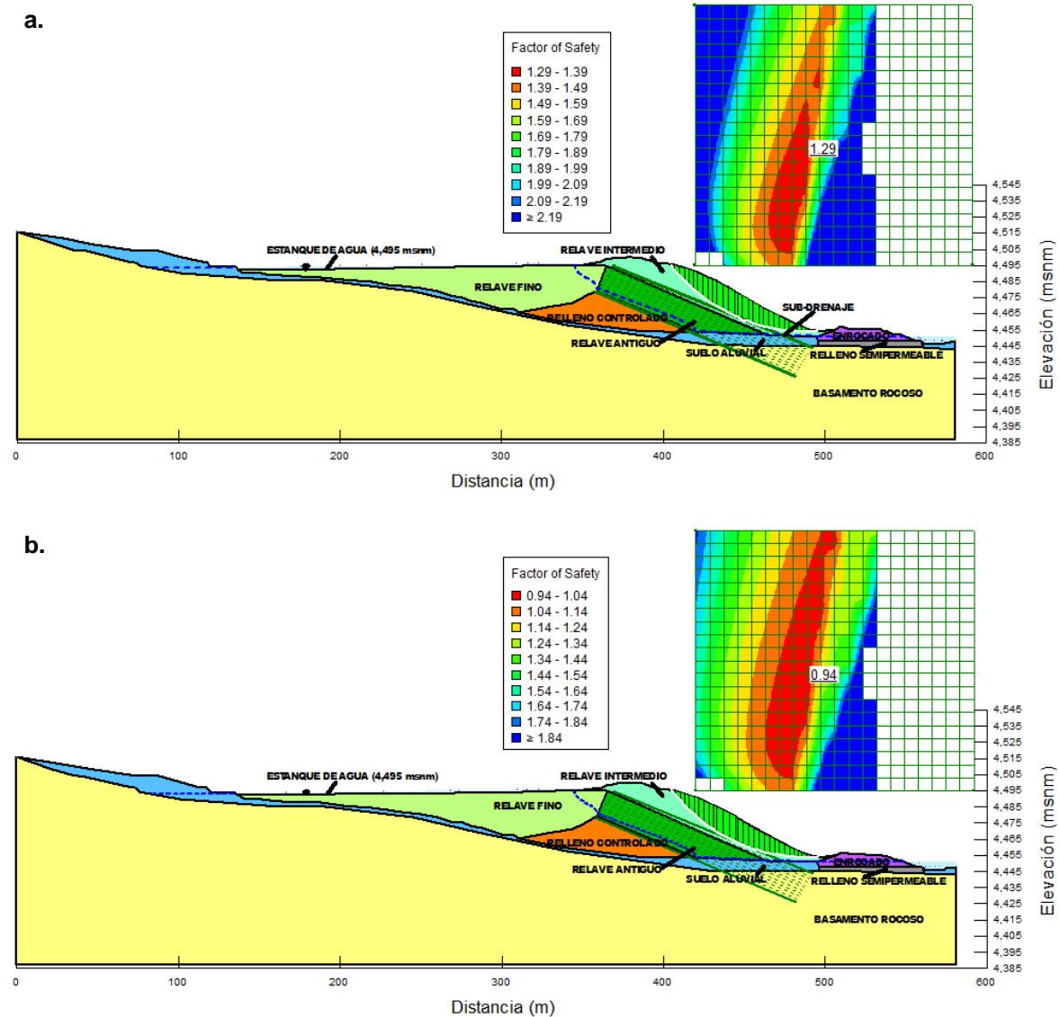
Figura 9.14: Factores de seguridad en la etapa de operación Nv= 4,499, a) condición estática y b) condición pseudo-estática.
