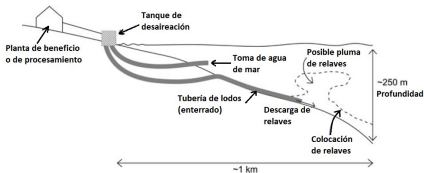
Figura 3.5: Esquema de la sección transversal de la disposición de relaves en aguas profundas (modificado de Lottermoser, 2010).
