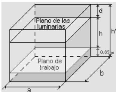
Figura 36. Geometría del local (cuadrada o rectangular).
