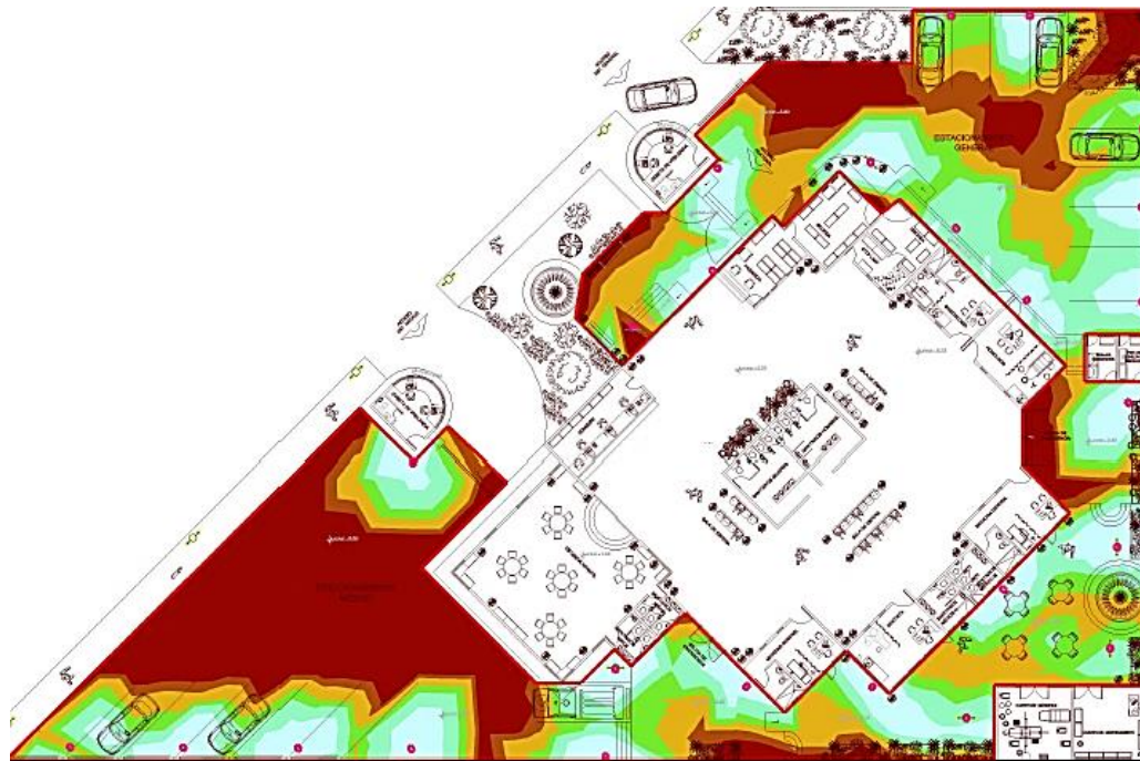
Figura 55. Resumen cálculo de iluminación con RELUX de: Estacionamientos (área exterior)
