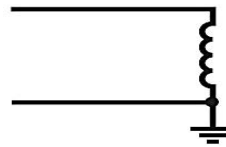
(k) Una fase: Dos conductores Punto final conectado a tierra
