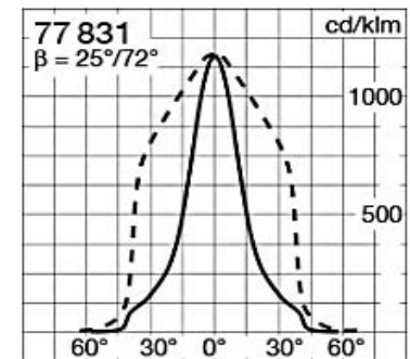
Figura 40. Coordenadas cartesianas. [21]
