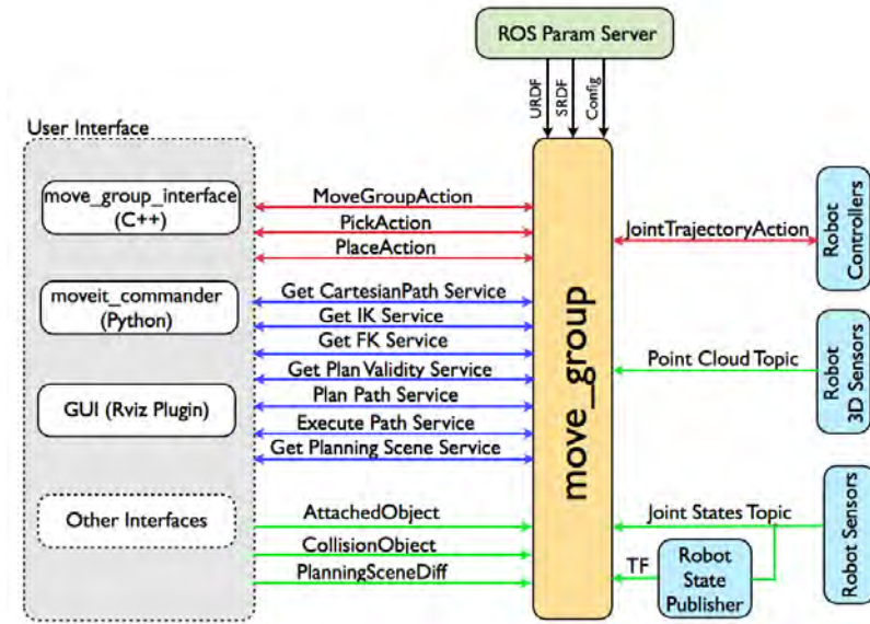
Figura 4.23: Imagen de la estructura de la paquetería moveIt! . [32]
