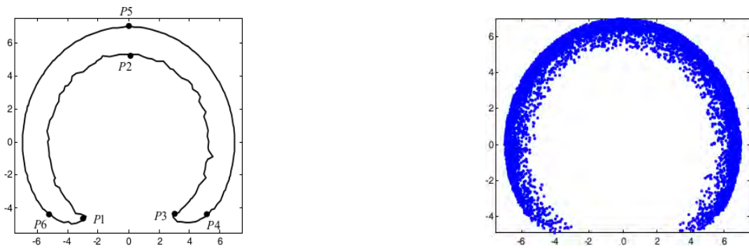
(a) Nube de puntos del espacio de trabajo en 2D. (b) Curva de la frontera del espacio de trabajo del brazo robótico.
