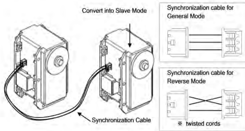
Figura 4.7: Configuración maestro-esclavo en servomotores dynamixel.
