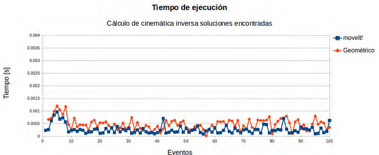
Figura 6.18: Gráfica de tiempo de ejecución para el cálculo de la cinemática inversa por método geométrico(rojo) y por método numérico (azul). Caso de solución encontrada.
