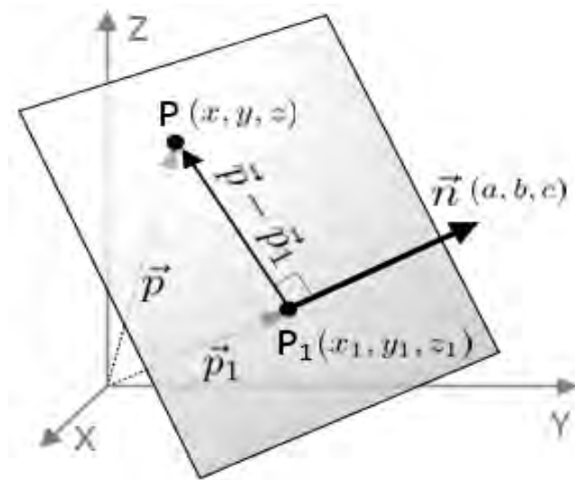
Figura 2.9: Ecuación de un plano definido por un punto y su normal.
