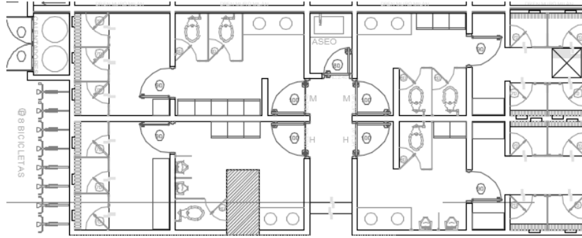
Ilustración 3.1, Planta sótano -1
