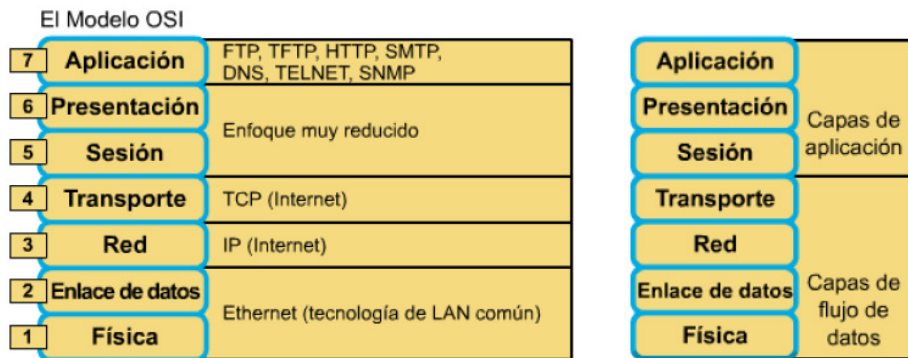
Imagen A-3.2: Modelo de Interconexión de Sistemas Abiertos OSI (Rigotti, 2008).
