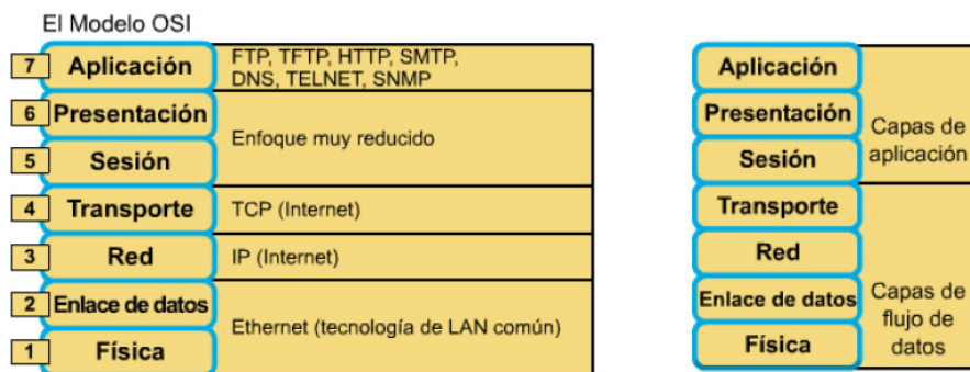
Imagen 1.1: Modelo de Interconexión de Sistemas Abiertos, “Modelo OSI” (Rigotti, 2008).
