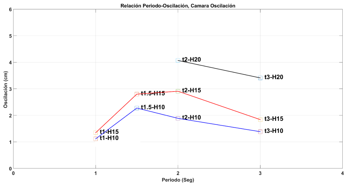
Figura 5.3.2. Panel a) Relación de máximos de oscilación, período y altura de ola (cámara de resonancia). Panel b) Relación de máximos de oscilación, período y altura de ola (cámara de oscilación).
