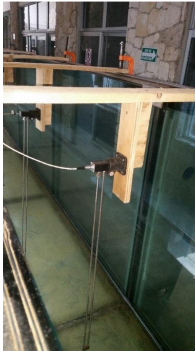
Figura 4.3.7. Colocación de sensores de resistividad eléctrica para la obtención de datos de superficie libre.
