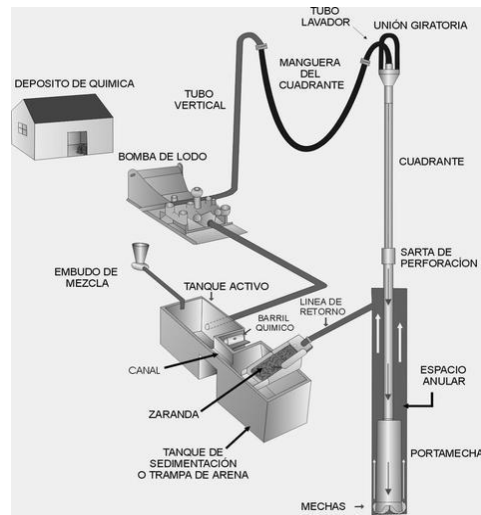
Figura3. Las partes del proceso de circulación.
