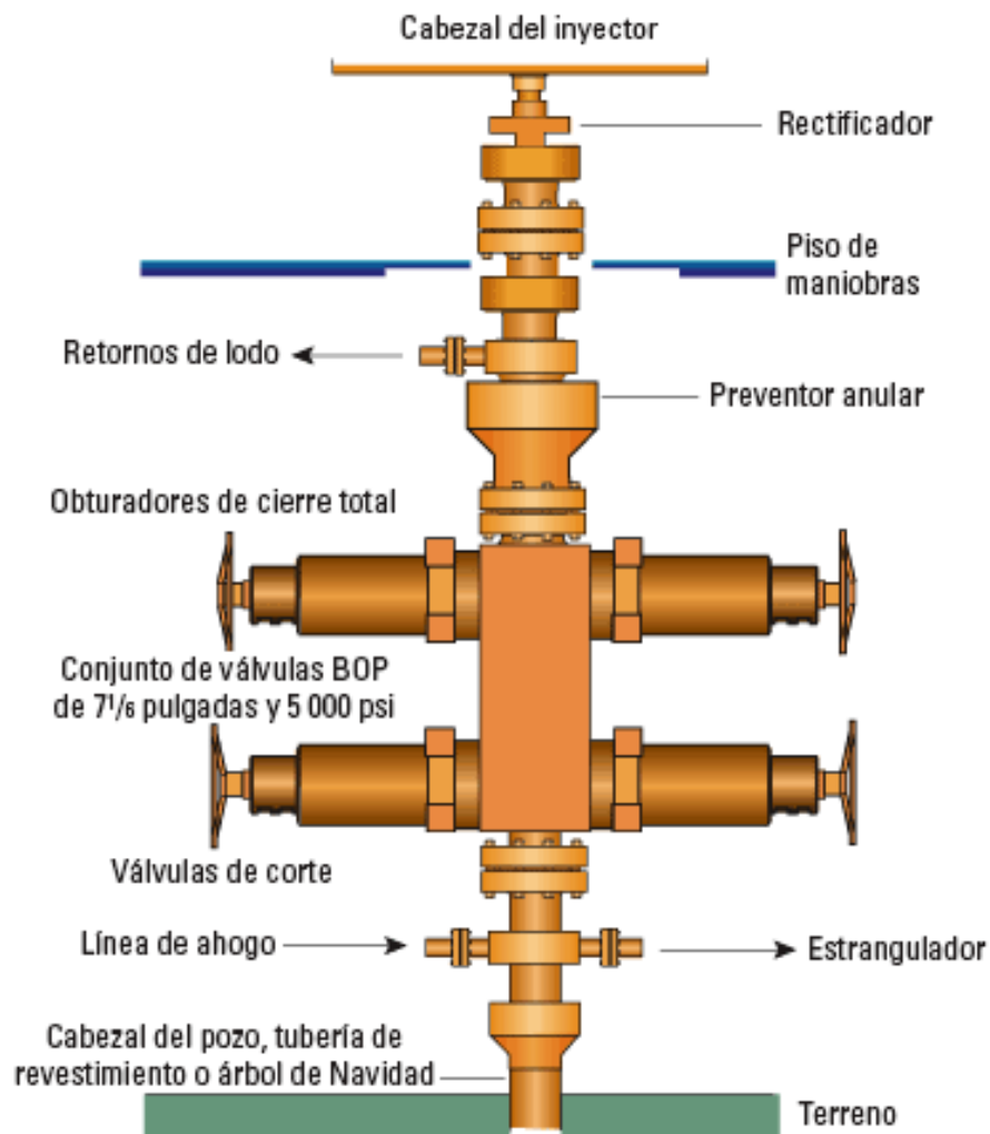
Figura 8. Preventor de reventones. Esta configuración de BOP es típica para un pozo perforado con un diámetro de más de 4 pulgadas.
