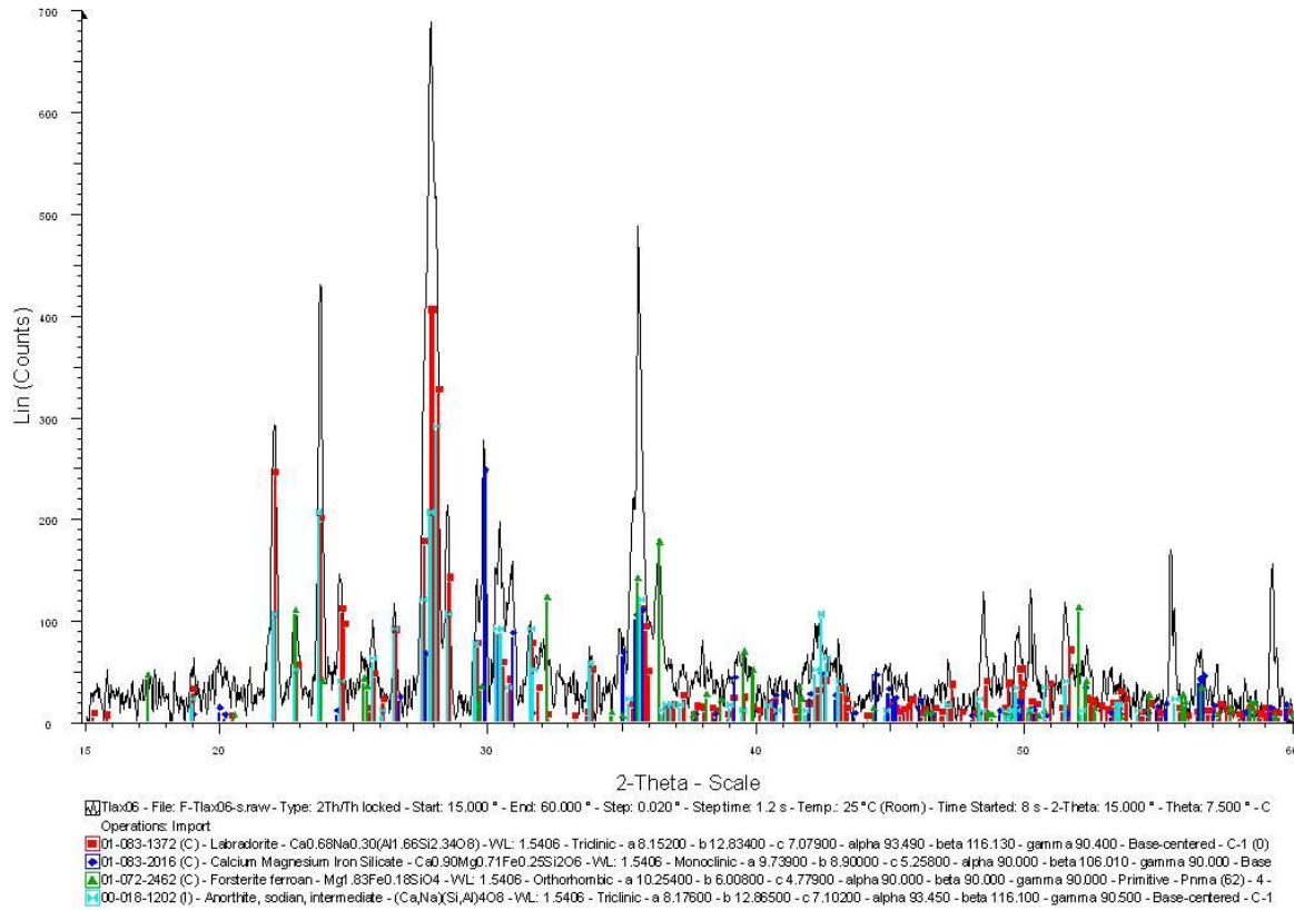
Gráfica A 4.- Difracción de rayos-X de polvos para Tlax-06.
