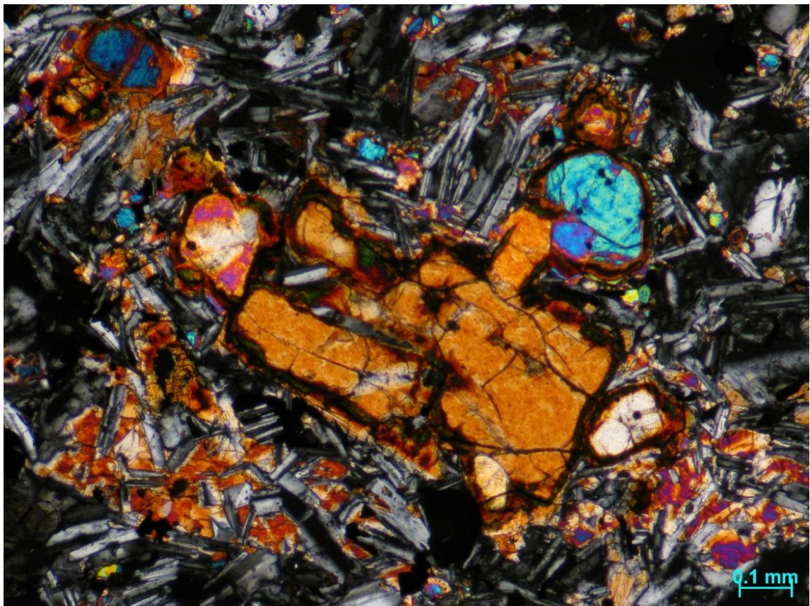
Figura 30.- Fotografía con microscopio óptico, zoom 10X y nicols cruzados de la lámina Tlax-05.
