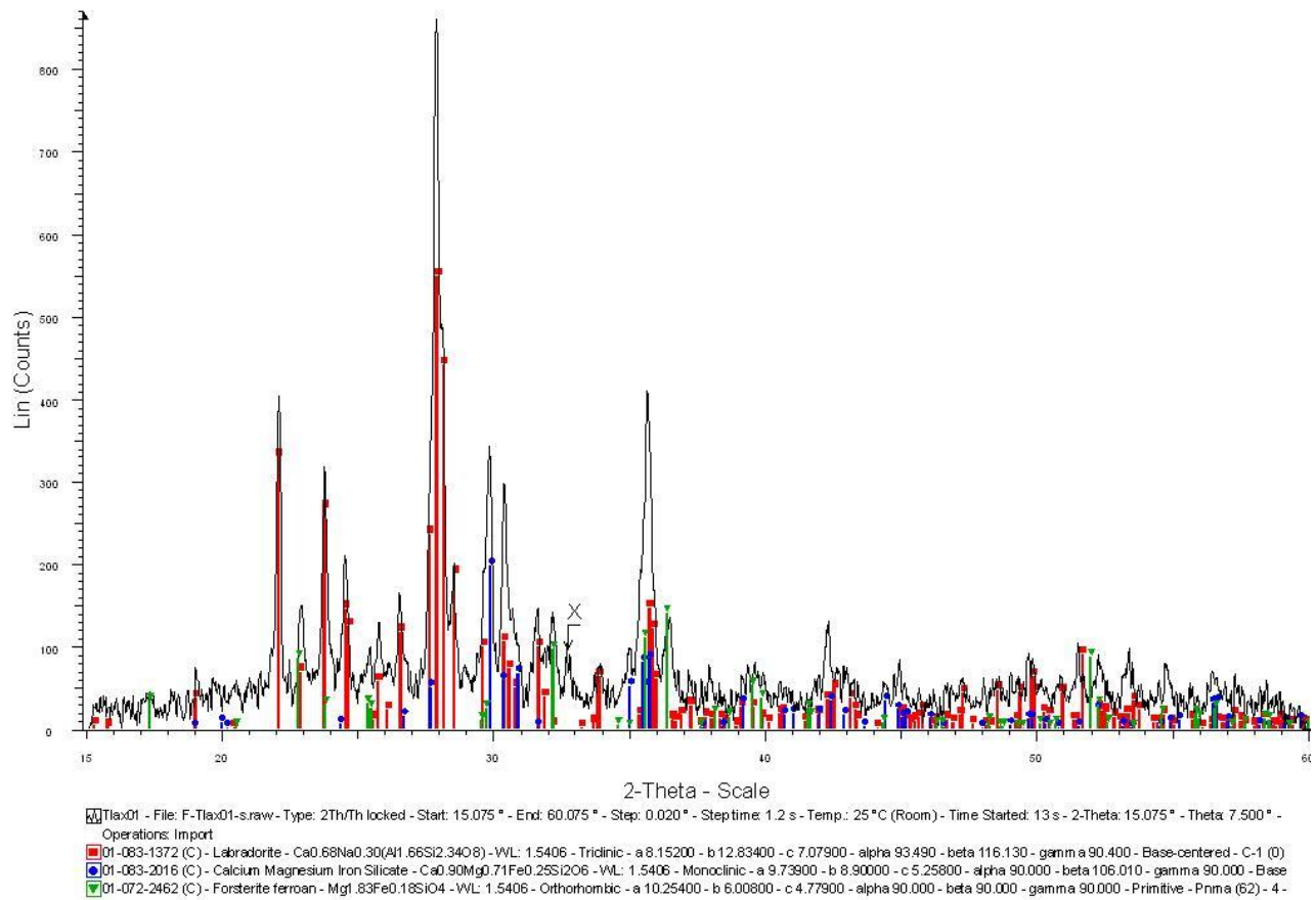
Gráfica A 1.- Difracción de rayos-X de polvos para Tlax-01.
