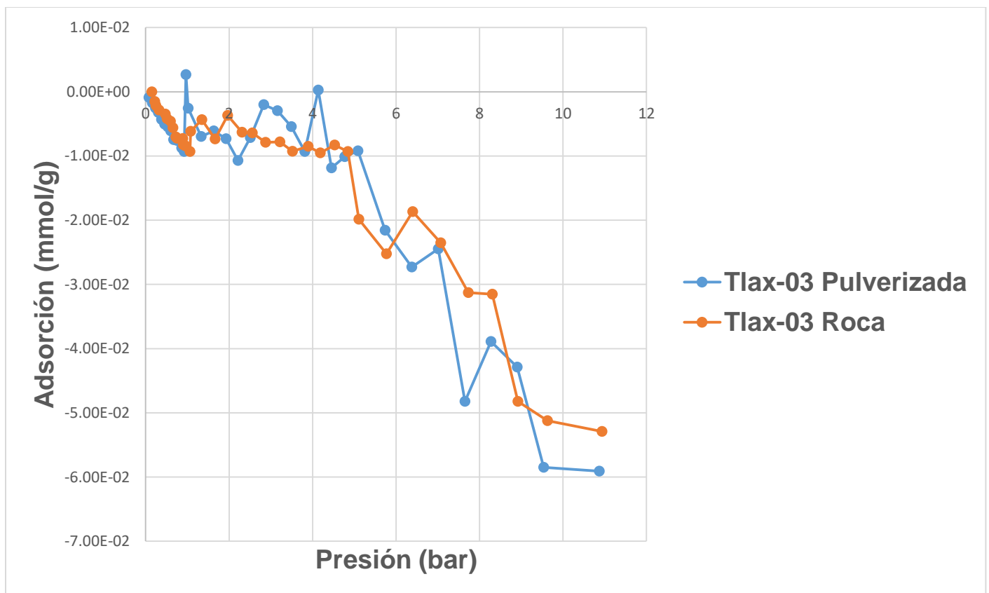
Gráfica 4.- Comparación de la capacidad de adsorción que tiene Tlax03, tanto la muestra de roca como el polvo de ésta.
