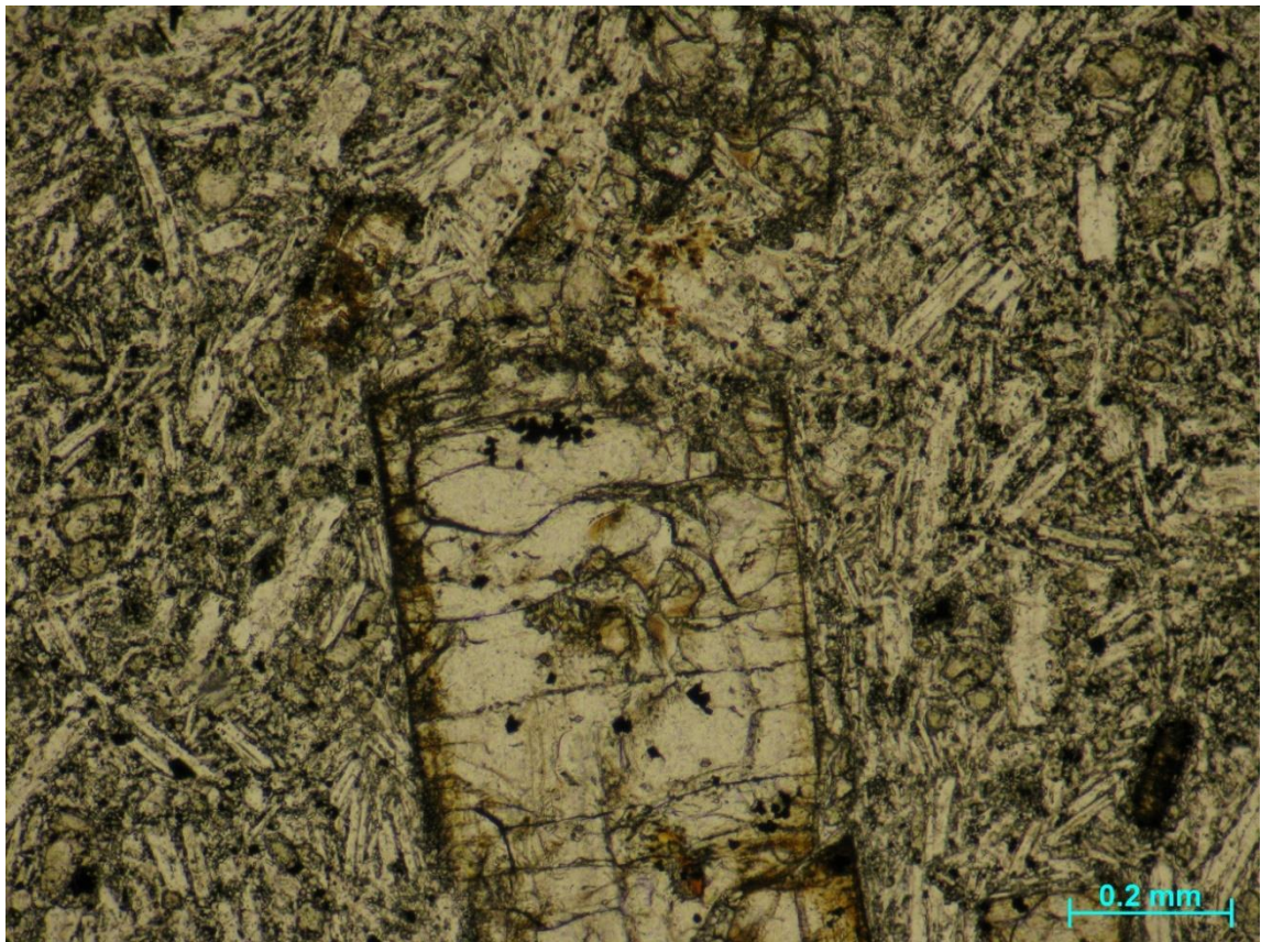
Figura A 12.- Fotografía con microscopio óptico, zoom 10X y nicoles paralelos de la lámina Tlax7'.
