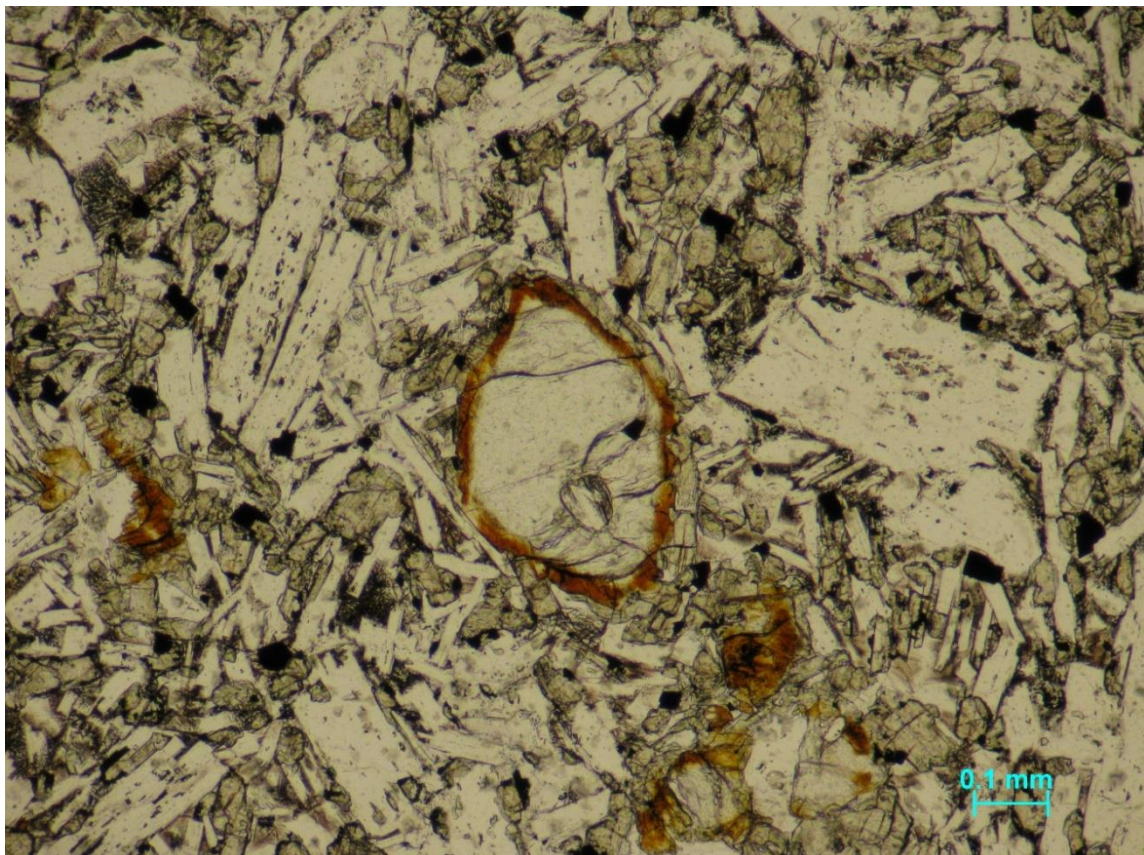
Figura 27.- Fotografía con microscopio óptico, zoom 10X y nicoles paralelos de la lámina Tlax-03.
