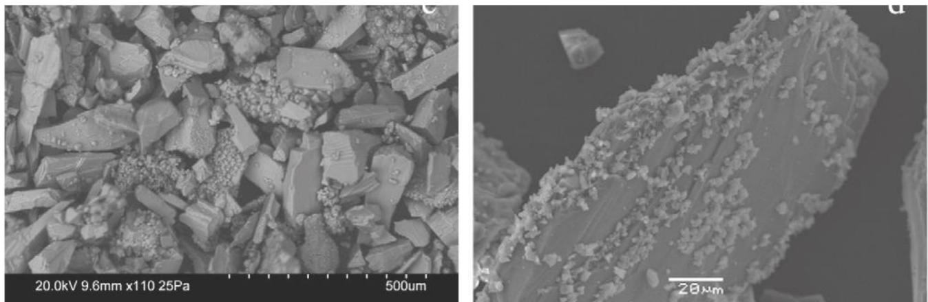
Figura 16.- Imágenes de microscopía electrónica de dióxidos aplastados con la precipitación secundaria de calcita. 33
