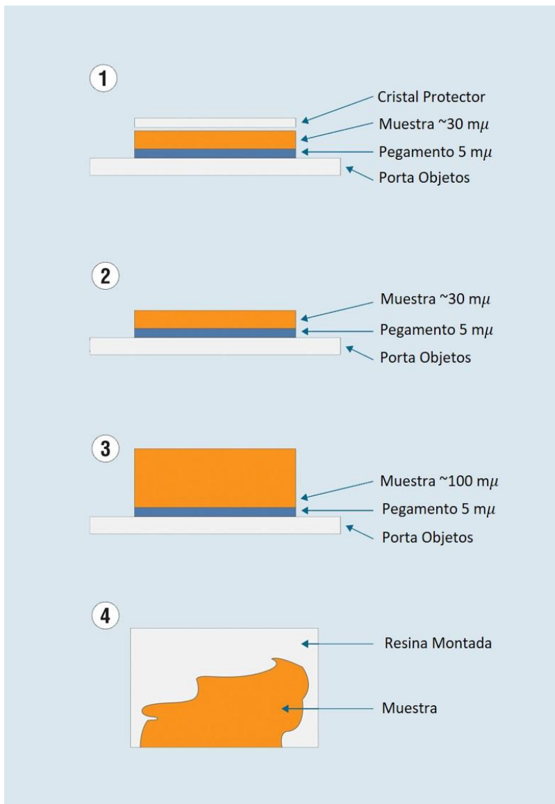
Figura 23.- Imagen de los diferentes tipos de lámina delgada que se pueden crear. 38
