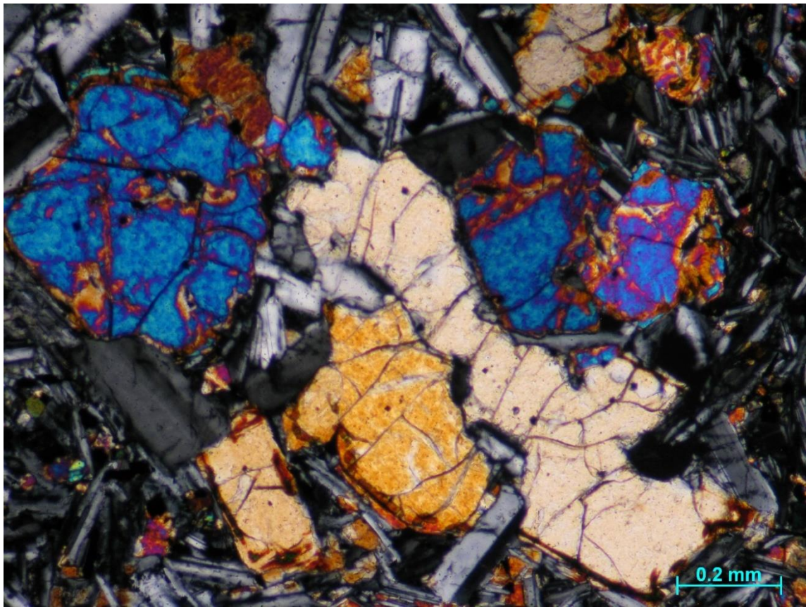
Figura A 8.- Fotografía con microscopio óptico, zoom 10X y nicoles cruzados de la lámina Tlax6.
