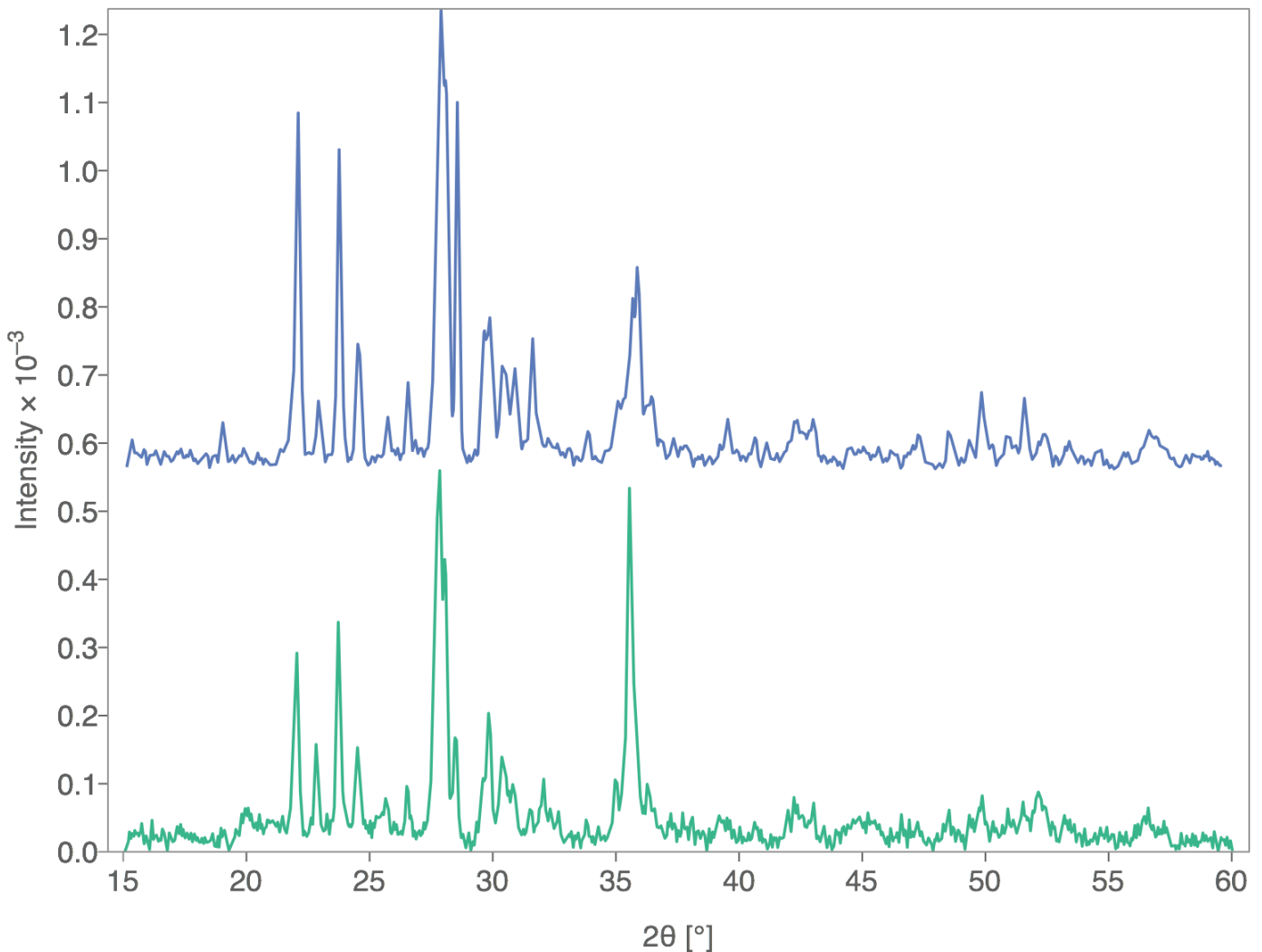
Gráfica 3.- Comparación de difracción de rayos-X de polvo entre Tlax-03 (verde) y Tlax-05 (azul).
