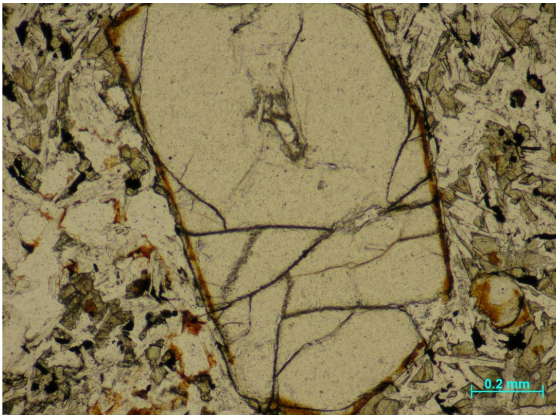
Figura A 9.- Fotografía con microscopio óptico, zoom 10X y nicoles paralelos de la lámina Tlax6.
