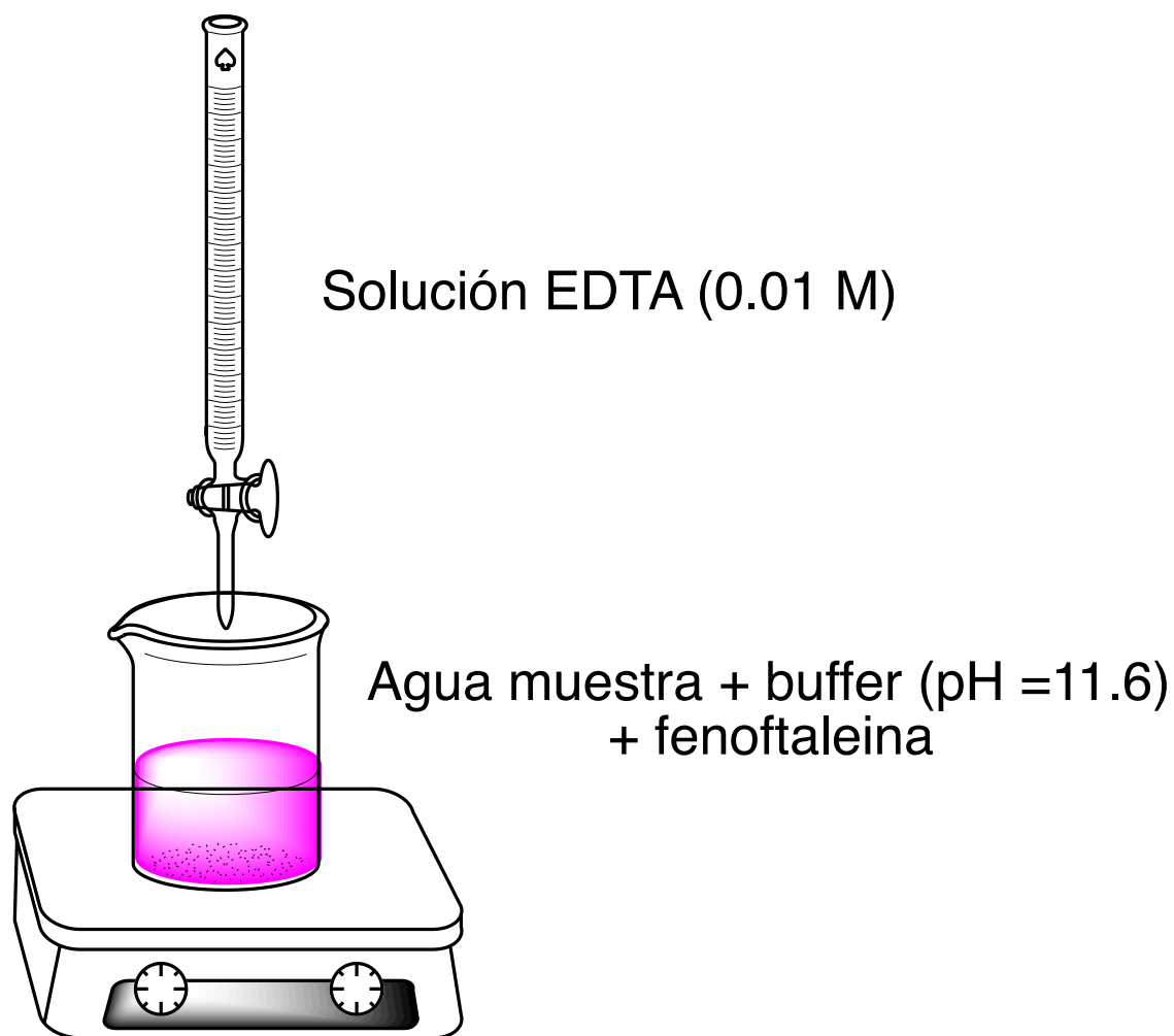
Figura 35.- Dispositivo empleado para la determinación de iones de \text{Ca}^{2+} , \text{Mg}^{2+} y \text{Fe}^{2+} .
