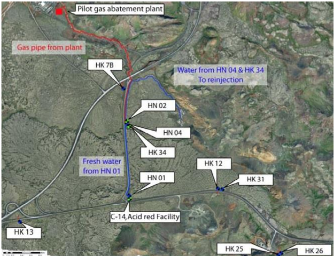
Figura 13.- Mapa de la distribución del pozo inyector, los de monitoreo, la planta Hellisheidi y la fuente de agua. 35
