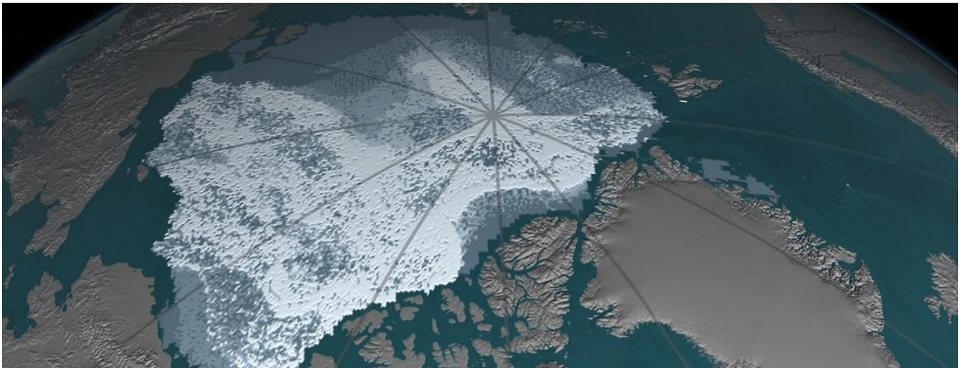
Figura 2.- Imagen del océano Ártico en septiembre de 1984. 8
