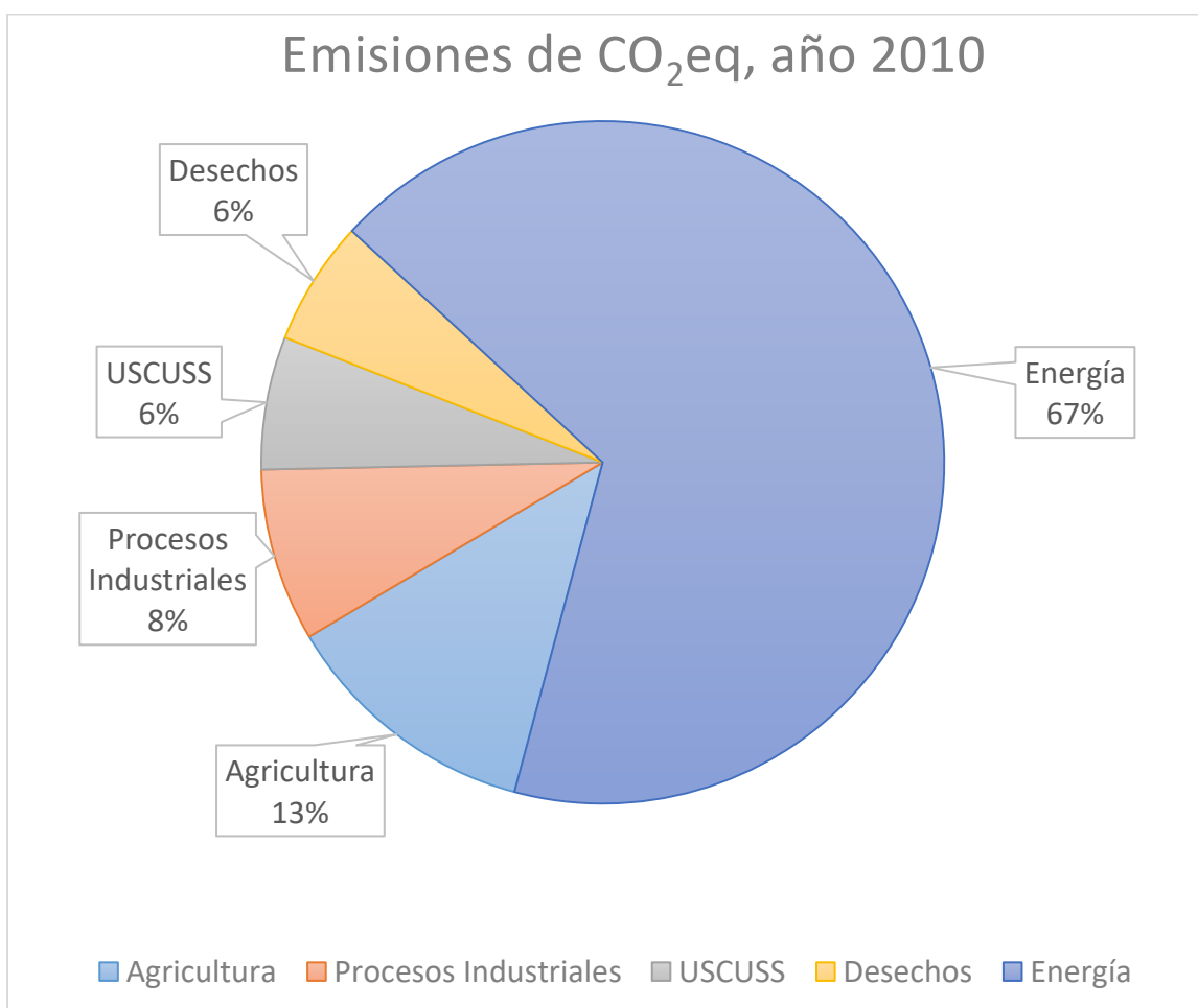
Gráfica 1.- Contribución de emisiones de GEI por categoría, 2010. 28
