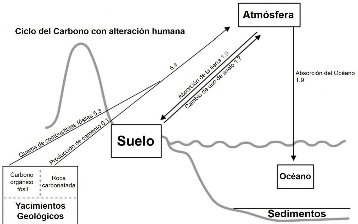
Figura 8.- Esquema de las perturbaciones causadas en el ciclo del carbono debido a actividades humanas. Los valores representan los petagramos de CO 2 producidos o tomados por diferentes partes del sistema al año (Pg/año). 30
