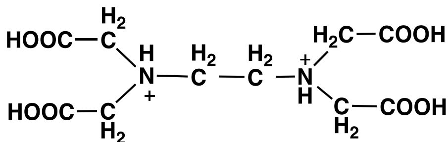
Figura 34.- Estructura del EDTA. 41
