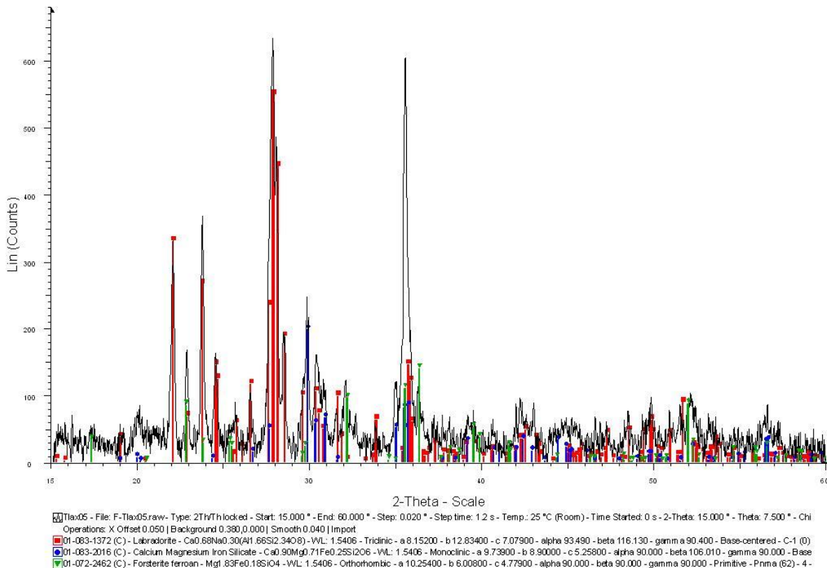
Gráfica A 3.- Difracción de rayos-X de polvos para Tlax-05.
