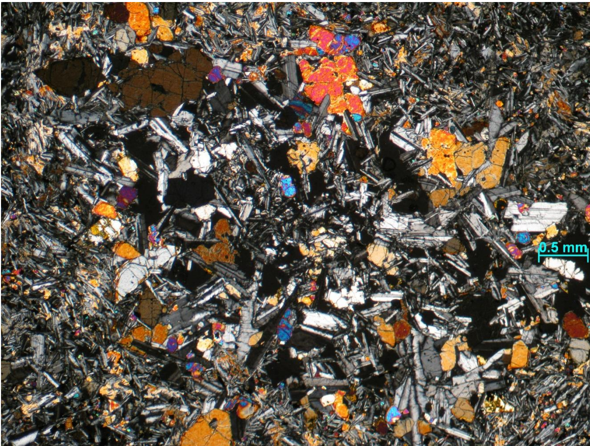
Figura A 7.- Fotografía con microscopio óptico, zoom 2.5X y nicoles cruzados de la lámina Tlax6'.
