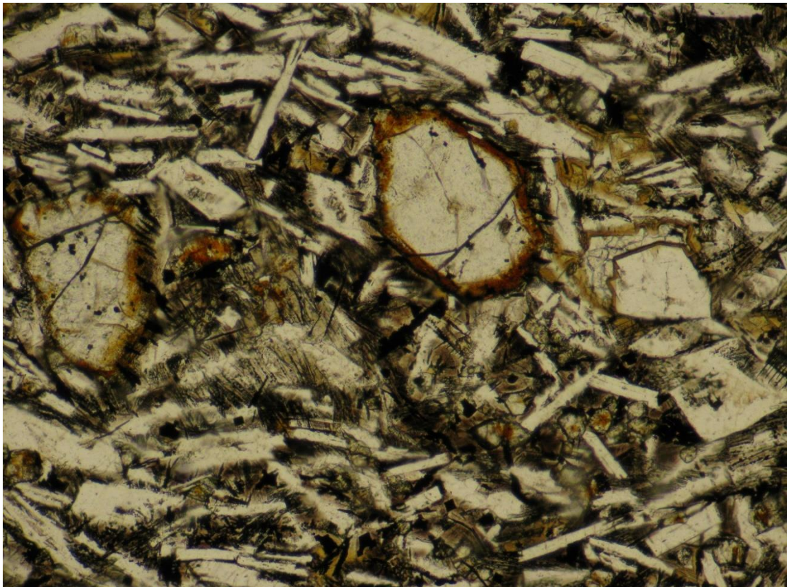
Figura A 3.- Fotografía con microscopio óptico, zoom 10X y nicoles paralelos de la lámina Tlax1'.
