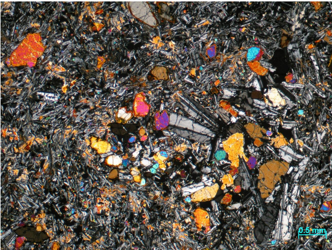
Figura 28.- Fotografía con microscopio óptico, zoom 2.5X y nicoles cruzados de la lámina Tlax5'.
