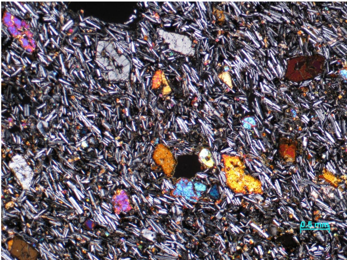
Figura A 2.- Fotografía con microscopio óptico, zoom 2.5X y nicoles cruzados de la lámina Tlax1'.
