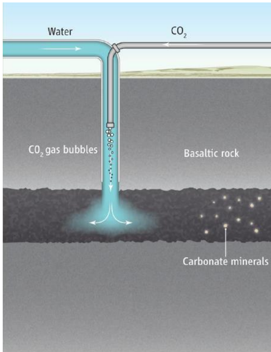
Figura 11.- Diagrama de la inyección de CO 2 y agua a la formación basáltica. 33
