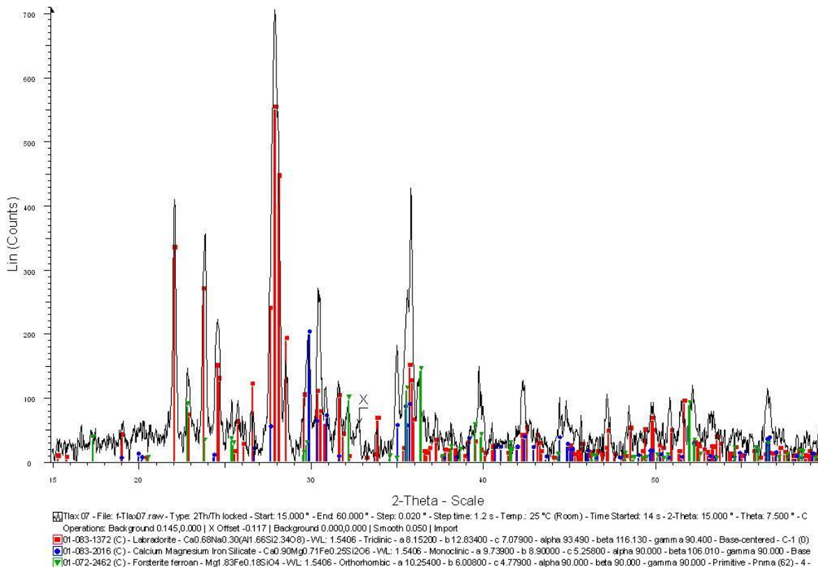
Gráfica A 5.- Difracción de rayos-X de polvos para Tlax-07.
