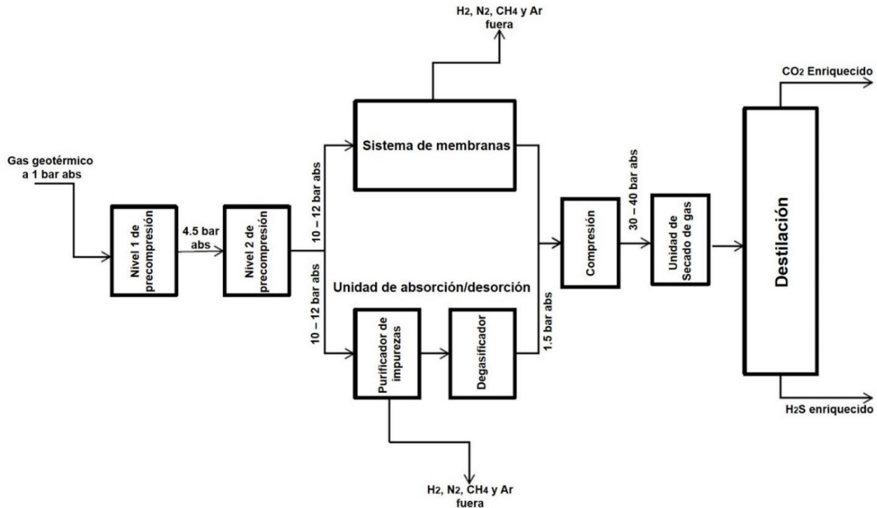
Figura 12.- Diagrama simplificado de la estación de separación de gas operada por la planta de energía en Hellisheidi, Islandia. 34
