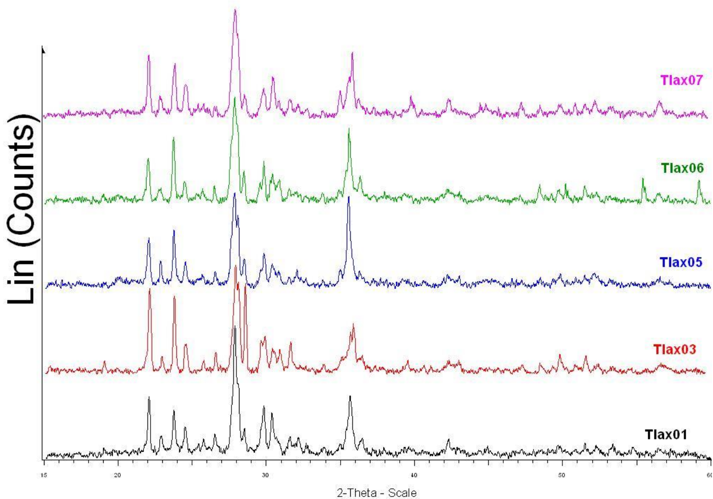
Gráfica A 6.- Comparación de los resultados de difracción de Rayos X de polvo para Tlax-01, Tlax-03, Tlax-05, Tlax-06 y Tlax-07.
