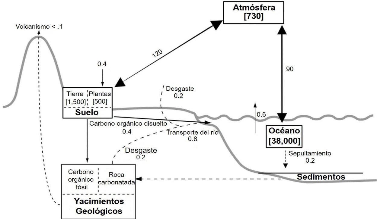
Figura 7.- Esquema de los principales componentes del ciclo natural del carbono. Los valores representan los petagramos 1 de CO 2 producidos o tomados por diferentes partes del sistema al año (Pg/año). 30
