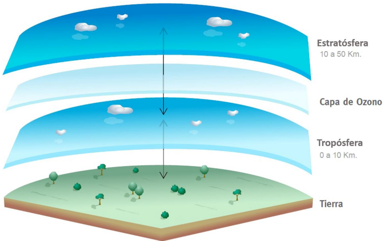
Figura 1.- Posición de la capa de Ozono dentro de la atmósfera de la Tierra. 4
