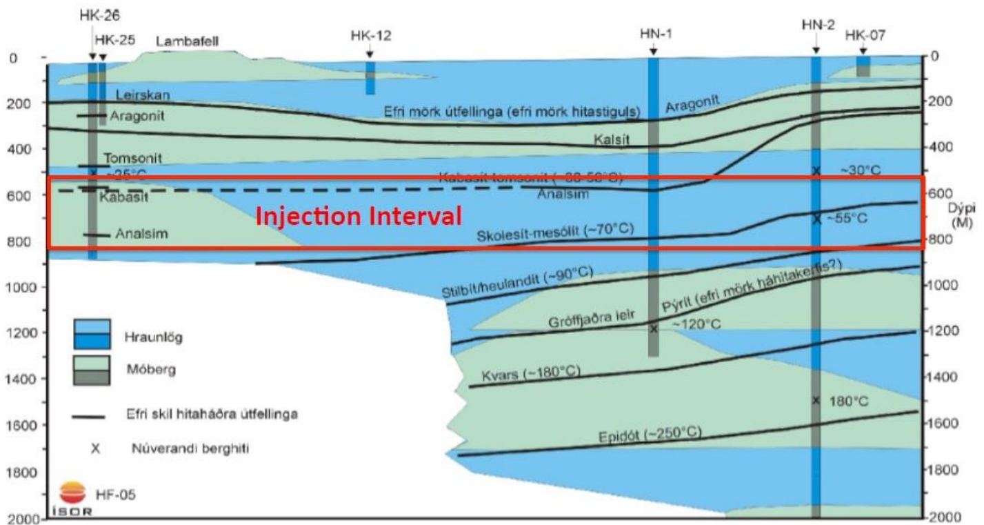
Figura 15.- Diagrama del subsuelo en el sitio de inyección del proyecto CarbFix. 32 Hraunlög – Flujo de lava; Móberg – Toba 1 ; Efri skil hitaháðra útfellinga – Precipitación de calor en el flanco superior; X Núverandi berghiti – Roca sedimentaria existente; Lambafell – Campo de lava; Kvars – Cuarzo;
