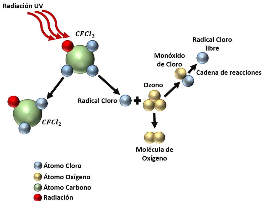
Figura 6.- Al momento en que la radiación UV quita la molécula de cloro ya sea de los CFCs o de los HCFCs, el átomo de cloro (Cl) se combina con una molécula de ozono (O 3 ) lo cual provoca que el ozono se convierta en oxígeno, liberándose después para volver a combinarse con otras moléculas de ozono y así sucesivamente, teniendo en promedio un átomo de cloro la capacidad de destruir hasta 100,000 moléculas de ozono. El proceso se detiene cuando el átomo de cloro se mezcla con algún compuesto químico que lo neutraliza. 25
