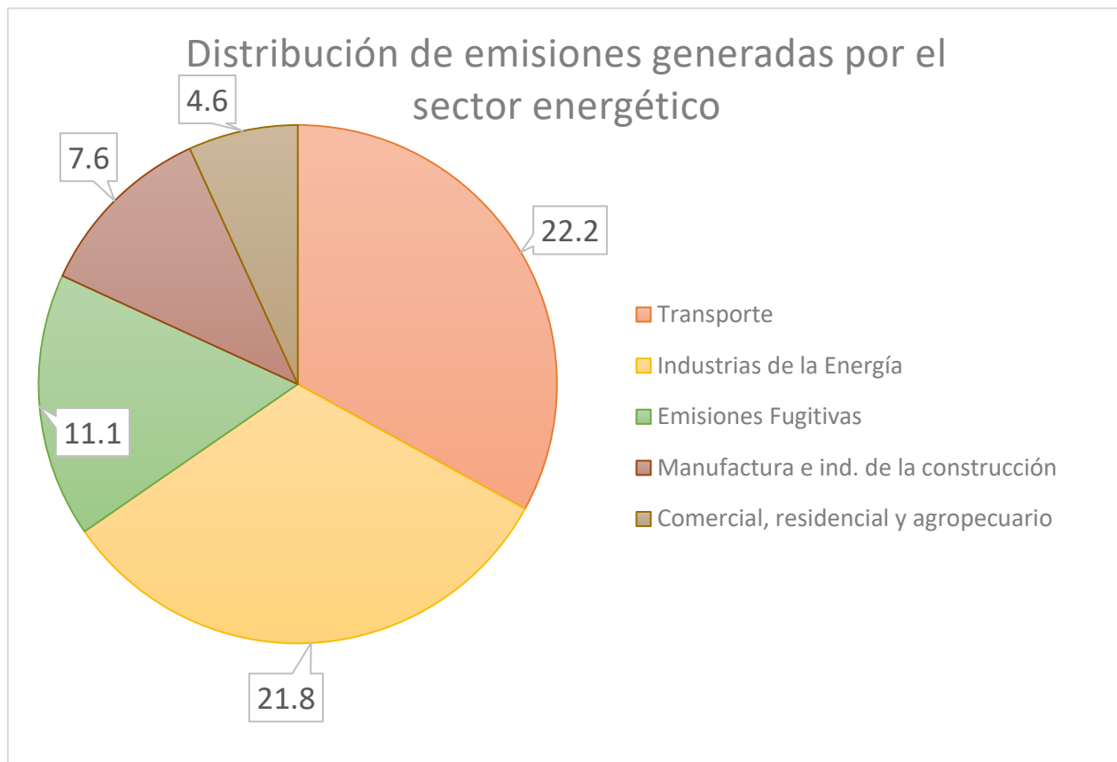
Gráfica 2.- Contribución de emisiones de GEI generados en el sector energético, 2010. 28
