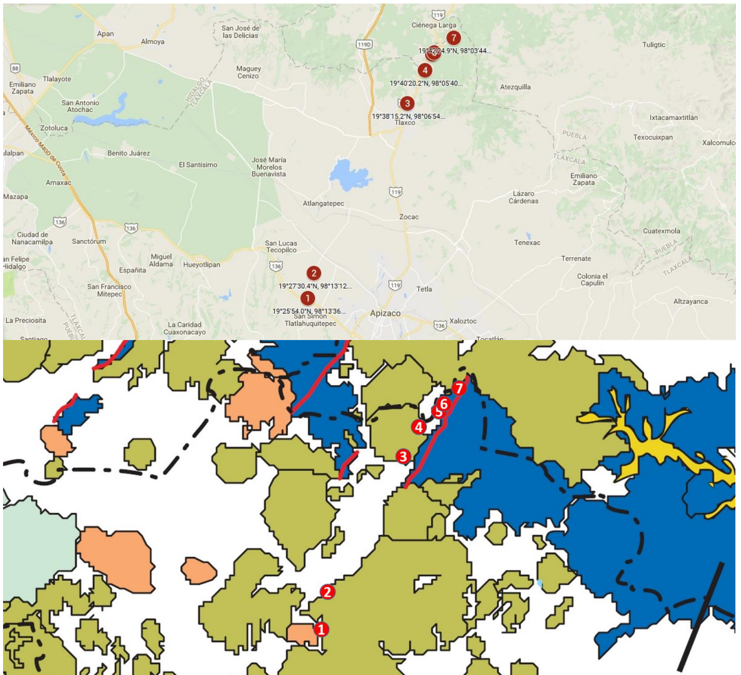
Figura 22.- Localización de los puntos de recolección de basaltos en el mapa de la faja volcánica Transmexicana.
