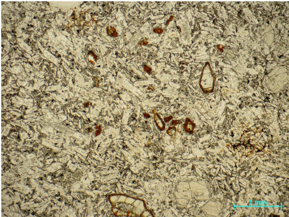
Figura A 6.- Fotografía con microscopio óptico, zoom 2.5X y nicoles paralelos de la lámina Tlax4.
