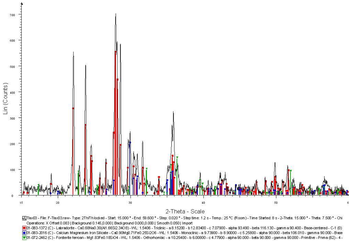
Gráfica A 2.- Difracción de rayos-X de polvos para Tlax-03.
