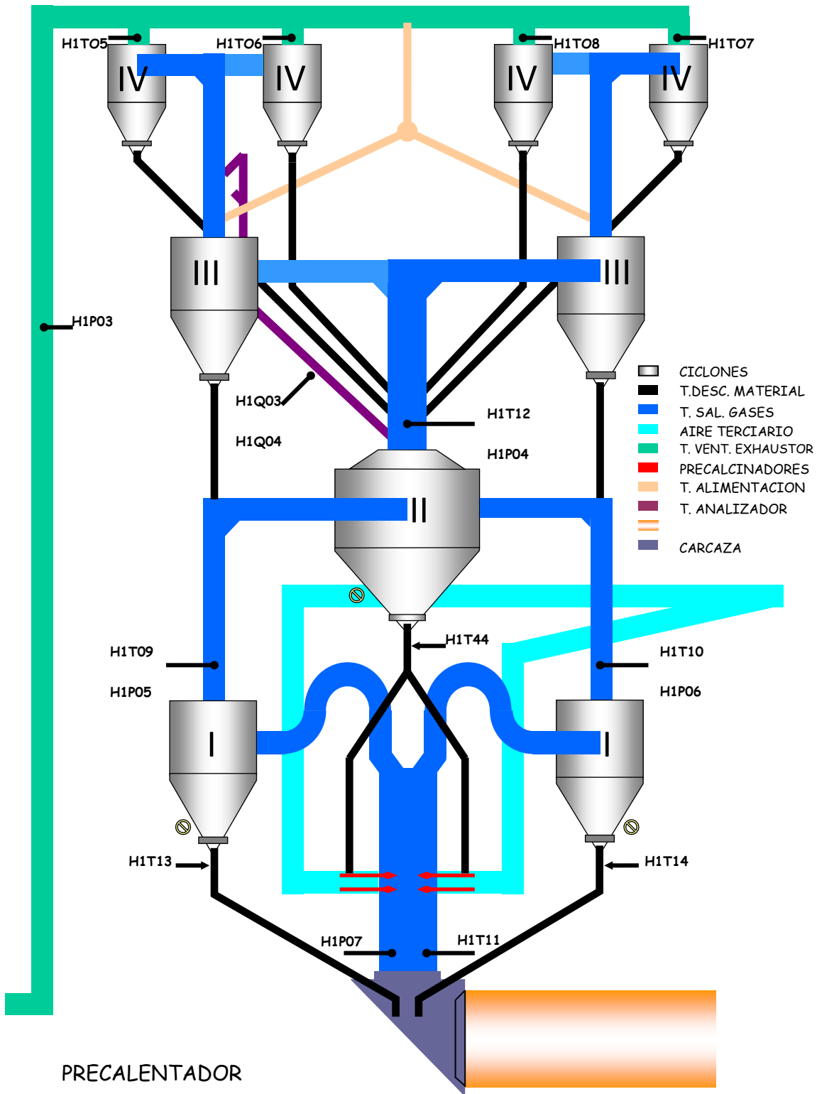
IMAGEN 4.10.2.2. DESCRIPCIÓN ETAPAS DEL HORNO ROTARIO NO. 4.
