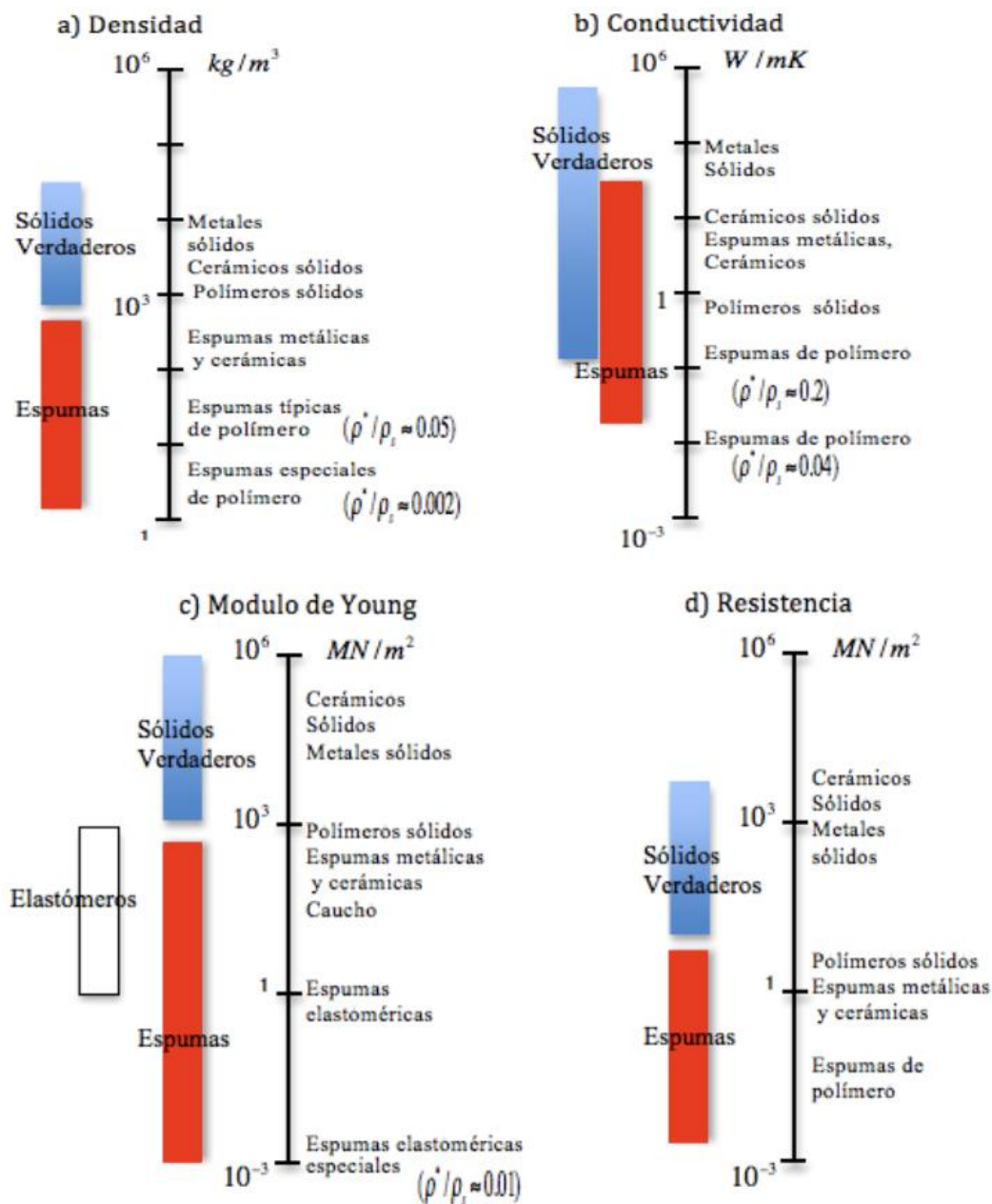
Figura 2.7: Rango de propiedades: a) densidad, b) conductividad térmica, c) módulo de Young, d) resistencia
