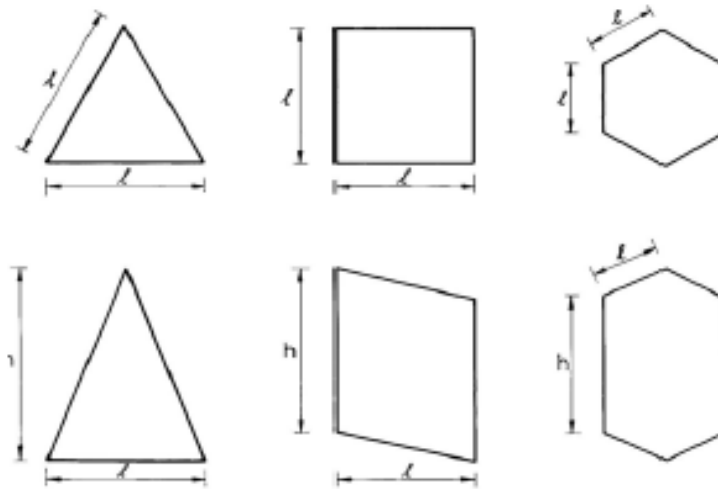
Figura 2.3: Formas poligonales de celda unitaria en materiales celulares tridimensionales
