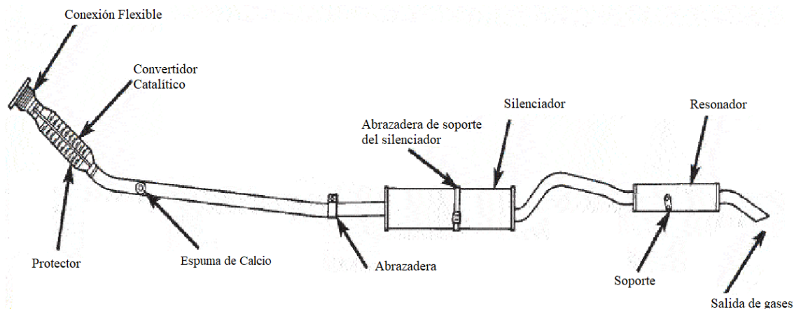
Figura 4.4: Esquema del sistema de escape de gases contaminantes
