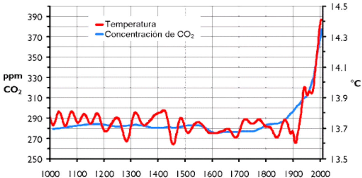
Figura 1.4: Evolución de concentraciones de bióxido de carbono y temperatura
