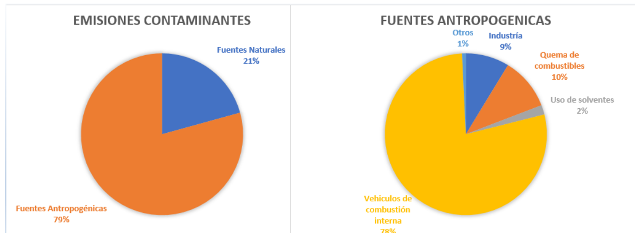
Figura 1.1: Fuentes contaminantes
