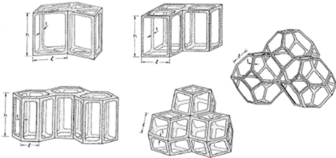
Figura 2.6: Agrupamiento de celadas formado mallas tridimensionales
