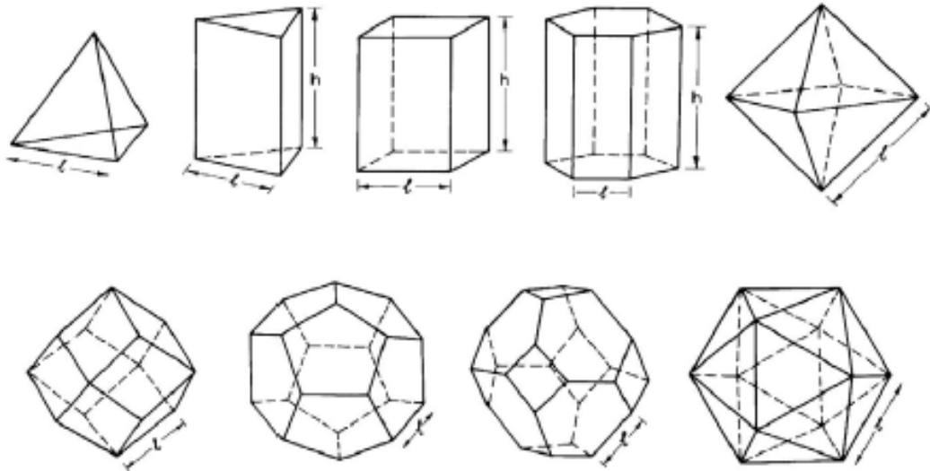
Figura 2.5: Formas poliédricas de celda unitaria en sólidos celulares tridimensionales
