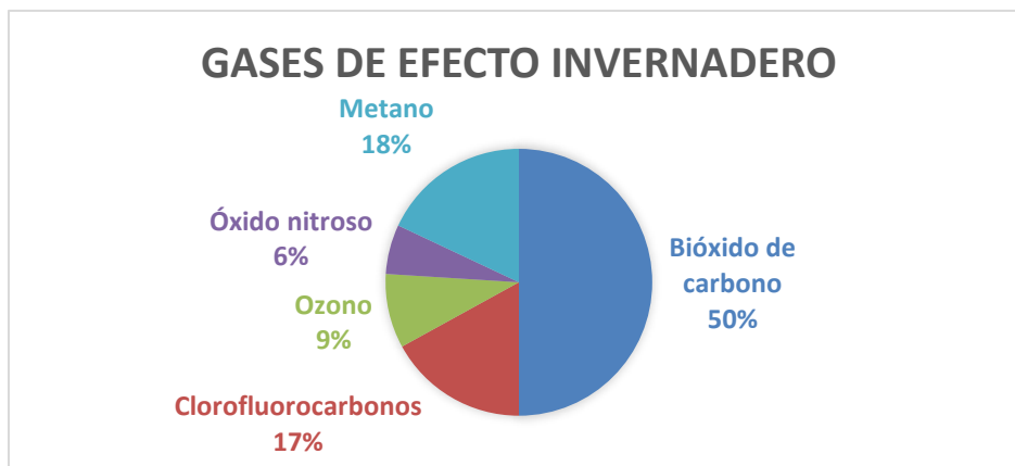
Figura 1.3: Gases de efecto invernadero
