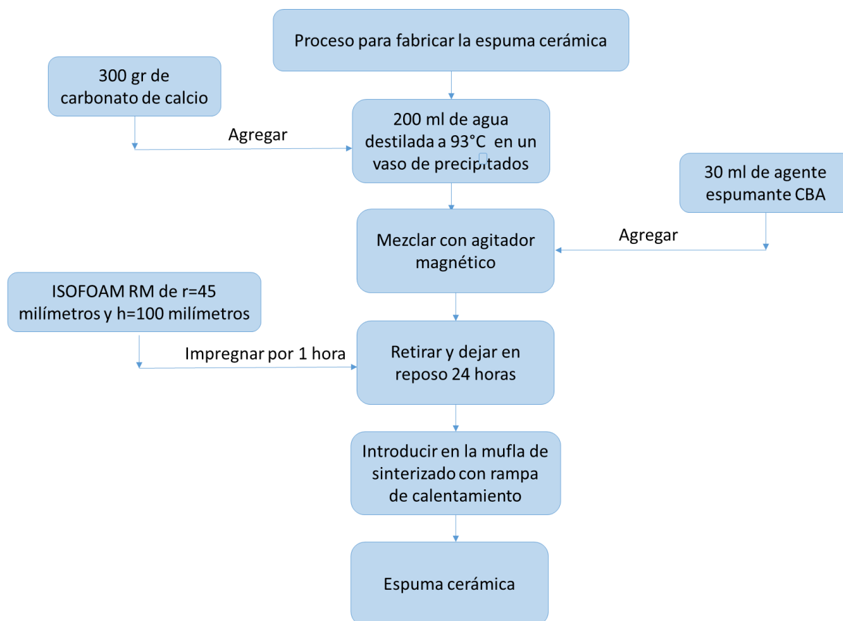
Figura 4.6: Diagrama de flujo para producir el filtro cerámico
