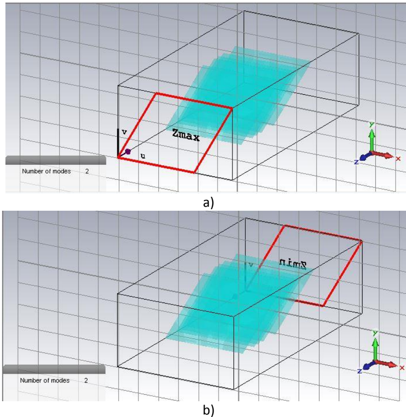
Figura 4.28.- Estructura de 5 capas con los puertos de a) entrada y b) salida
