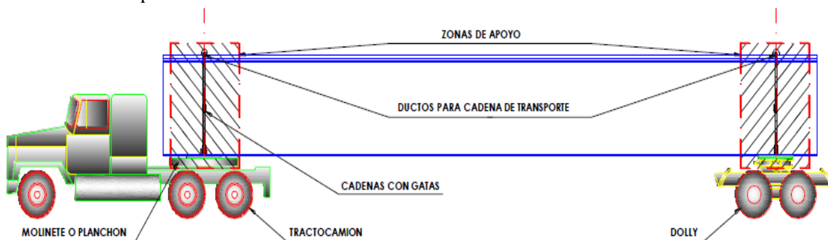
Figura 53. Elementos y arreglos de arneses para transportar travesaños cajón.
