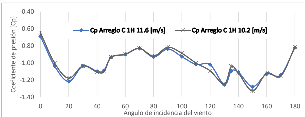
Figura 6.37. Cp de la cubierta del Arreglo C 1H variando el ángulo de incidencia del viento.
