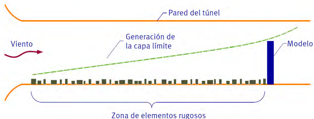
Figura 4.5. Generación de capa límite en un túnel de viento.
