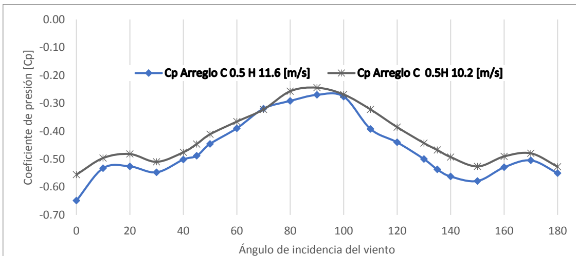
Figura A.29. Cp. del Muro 4 ARREGLO C 0.5H variando el ángulo de incidencia del viento.
