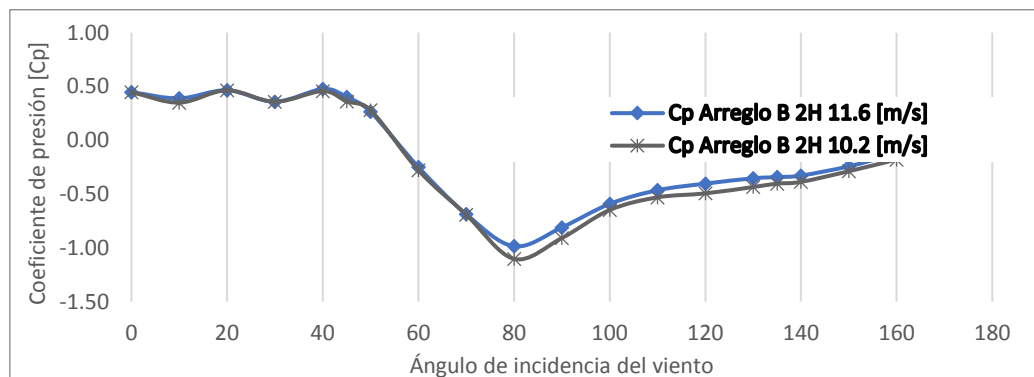
Figura 6.27. Cp del Muro 1 del Arrreglo B 2H variando el ángulo de incidencia del viento.
