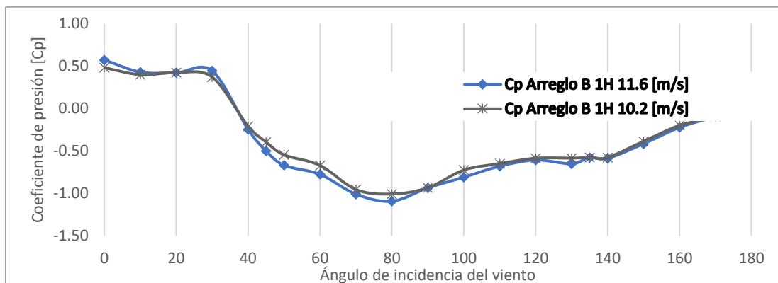
Figura 6.21 Cp. del Muro 1 del Arreglo B 1H variando el ángulo de incidencia del viento.
