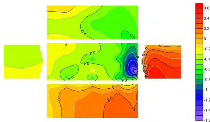
Figura A.7. Contorno de presión del Modelo Aislado con un ángulo de incidencia de 150°gr vel=11.6 m/s
