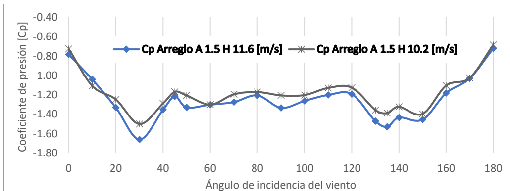
Figura 6.16. Cp cubierta Arreglo A 1.5H variando el ángulo de incidencia del viento.
