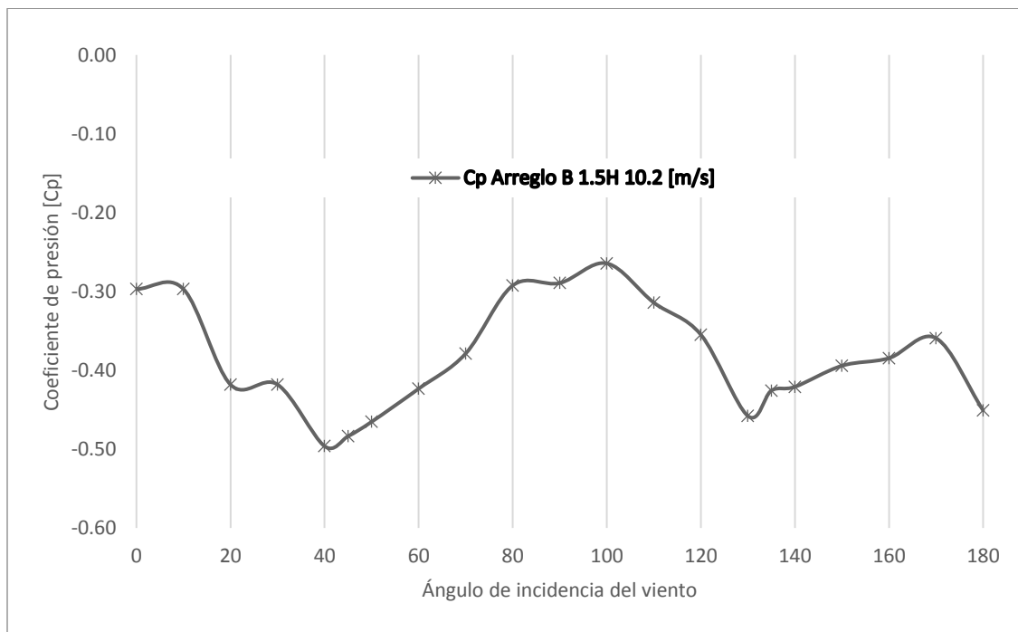
Figura A.23. Cp. del Muro 4 ARREGLO B 1.5H variando el ángulo de incidencia del viento.
