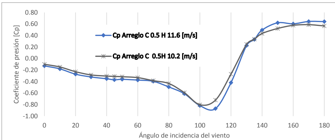
Figura A.28. Cp. del Muro 3 ARREGLO C 0.5H variando el ángulo de incidencia del viento.
