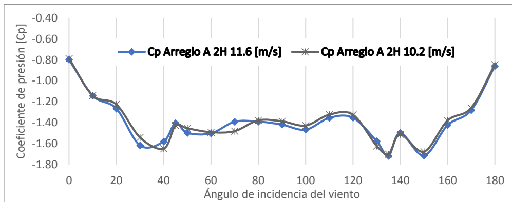
Figura 6.19. Cp de la cubierta del Arreglo A 2H variando el ángulo de incidencia del viento.
