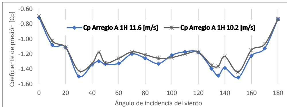
Figura 6.13. Cp de la cubierta del Arreglo A 1H variando el ángulo de incidencia del viento.
