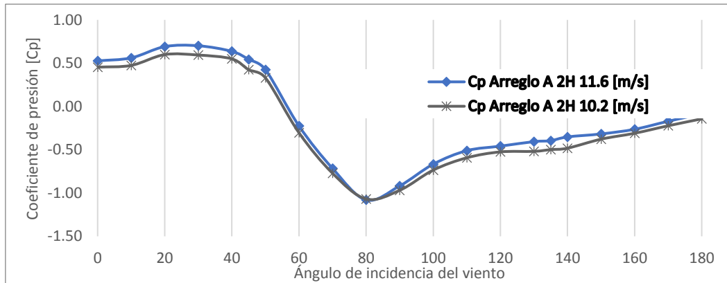
Figura 6.18. Cp del Muro 1 del Arreglo A 2H variando el ángulo de incidencia del viento.
