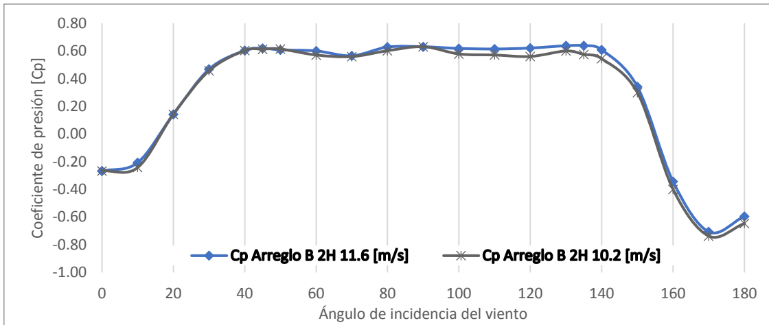
Figura A.24. Cp. del Muro 2 ARREGLO B 2H variando el ángulo de incidencia del viento.
