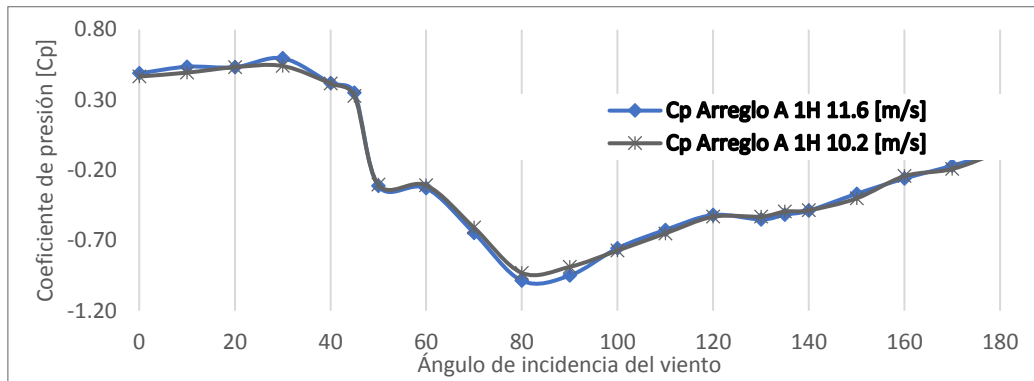
Figura 6.12. Cp. del Muro 1 del Arreglo A 1H variando el ángulo de incidencia del viento.
