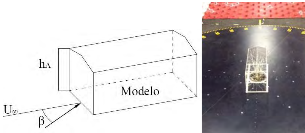
Figura 6.1. Colocación del modelo y dirección del viento.
