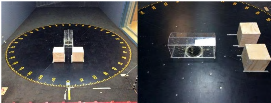
Figura 6.23. Arreglo B con una separación de 30 cm (1.5 H)
