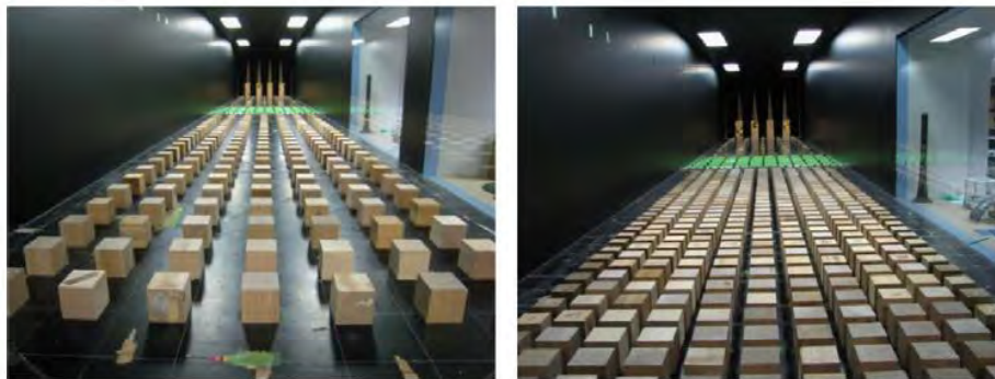
Figura 3.6. Pruebas en túnel de viento con diferente densidad urbana. (Kim, et al., 2015)
