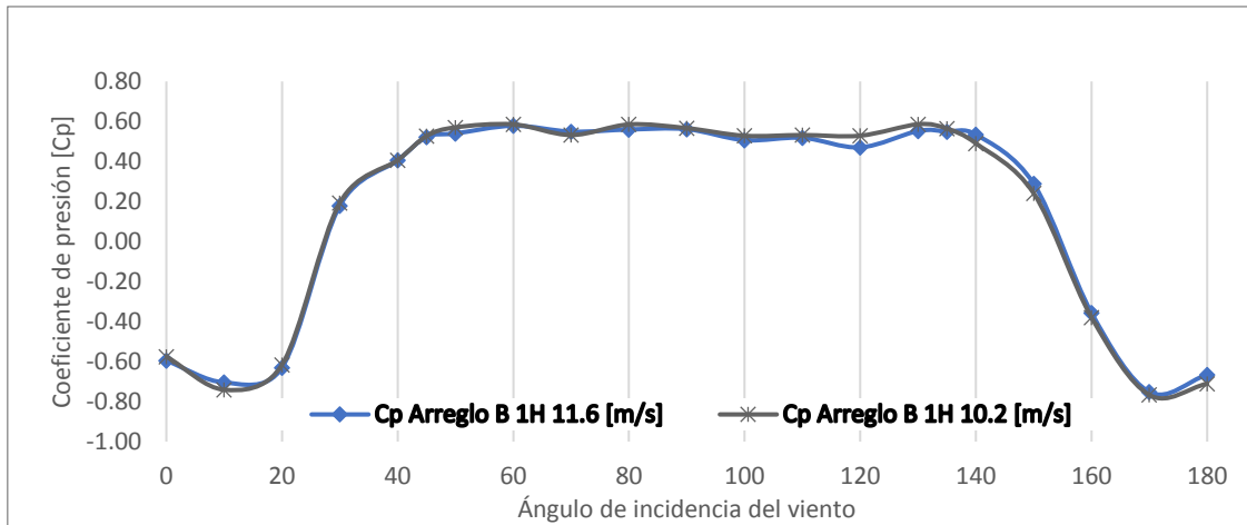
Figura A.1. Cp del Muro 2 del Modelo Aislado variando el ángulo de incidencia del viento.
