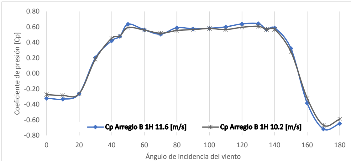
Figura A.18. Cp. del Muro 2 ARREGLO B 1H variando el ángulo de incidencia del viento.
