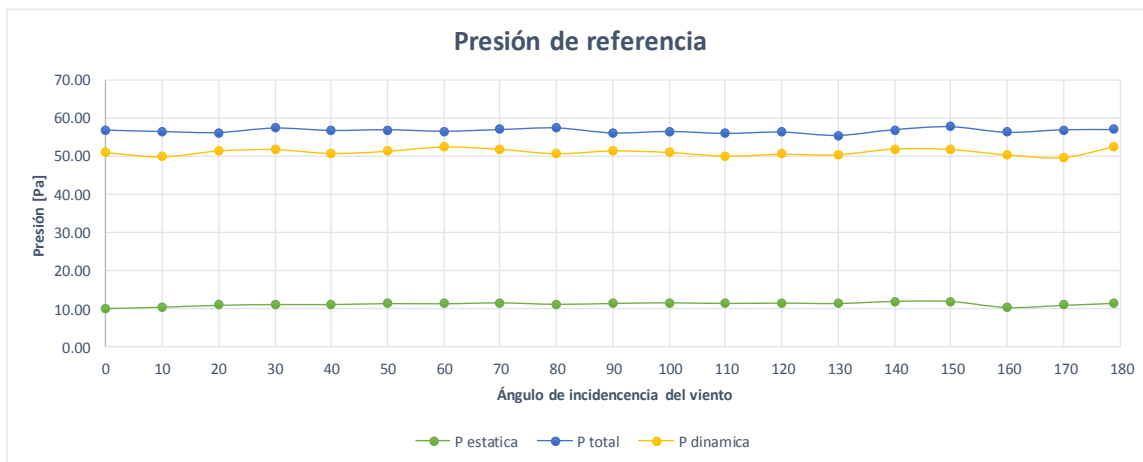
Figura 6.3. Presión de referencia para el Modelo aislado con una velocidad de 10.2 m/s
