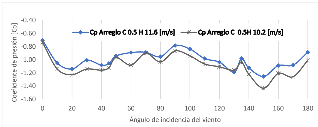
Figura 6.31. Cp cubierta Arreglo C 0.5H variando el ángulo de incidencia del viento.
