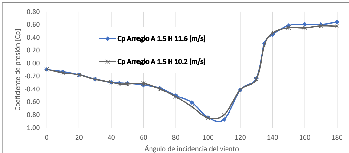
Figura A.13. Cp. del Muro 3 ARREGLO A 1.5H variando el ángulo de incidencia del viento.
