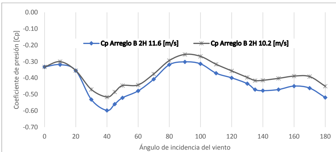
Figura A.26. Cp. del Muro 4 ARREGLO B 2H variando el ángulo de incidencia del viento.
