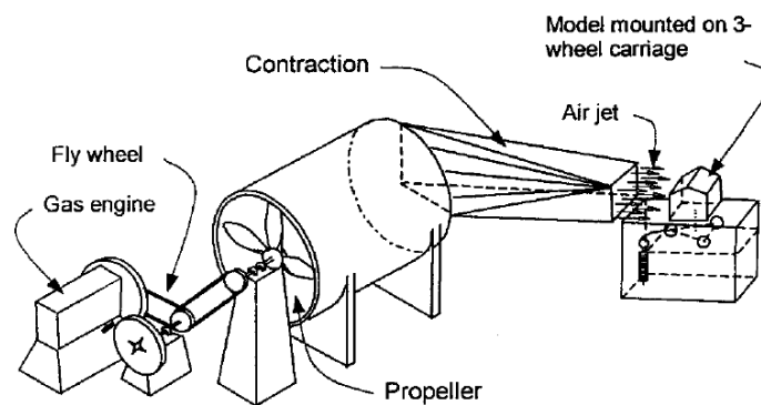
Figura 4.1. Esquema de la máquina de soplado de Kernot (Aynsley, et al., 1977)
