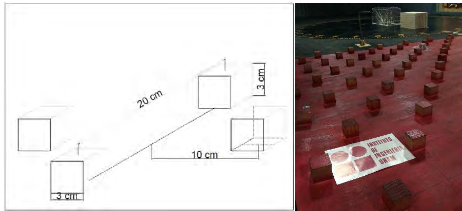
Figura 5.15. Cubos para generar rugosidad.
