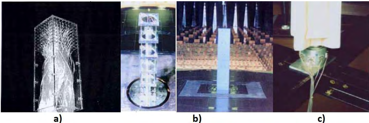
Figura 4.13. a) Modelo rígido b) Modelo aerolastico c) Modelo de balance de base (Tamura, 2007).
