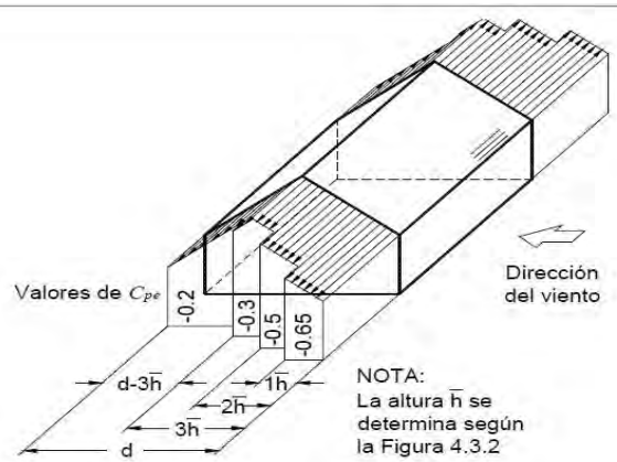
Figura 3.2. Coeficientes de presión para Nave Industrial, (MOCDV, 2008)
