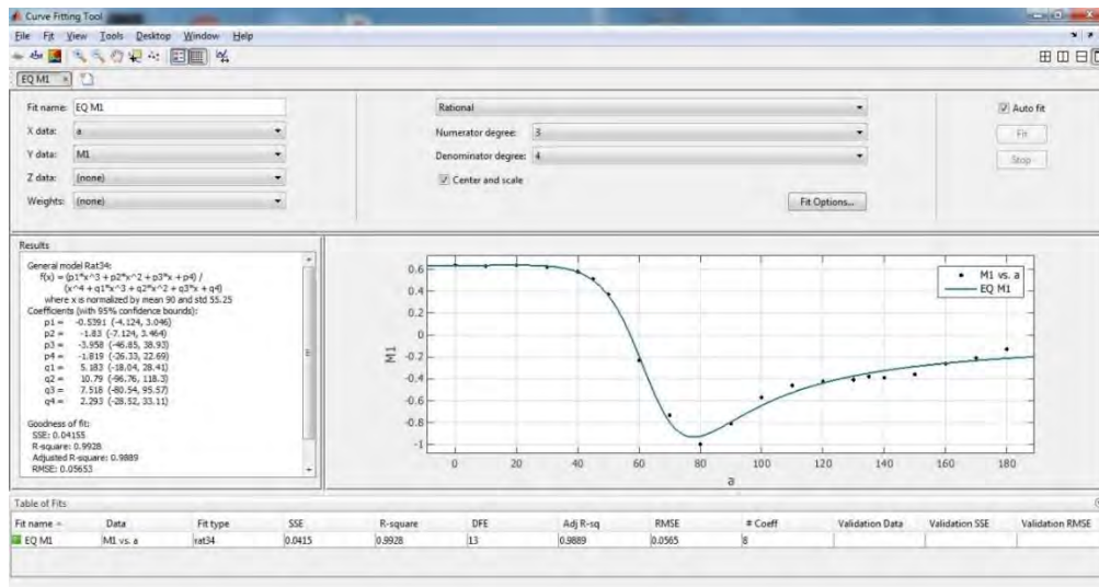
Figura 6.40. Interfaz del programa de ajuste de curvas de Matlab resultados para Muro 1
