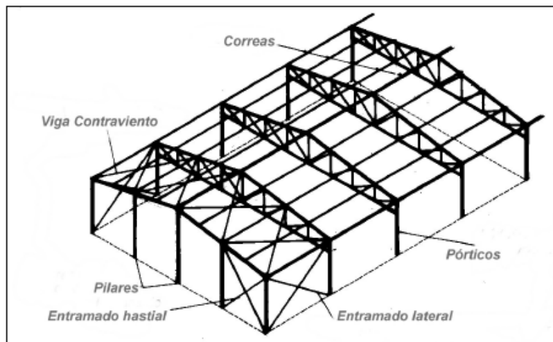
Figura 2.8. Componentes de una Nave Industrial. (Argüelles et al, 2008)
