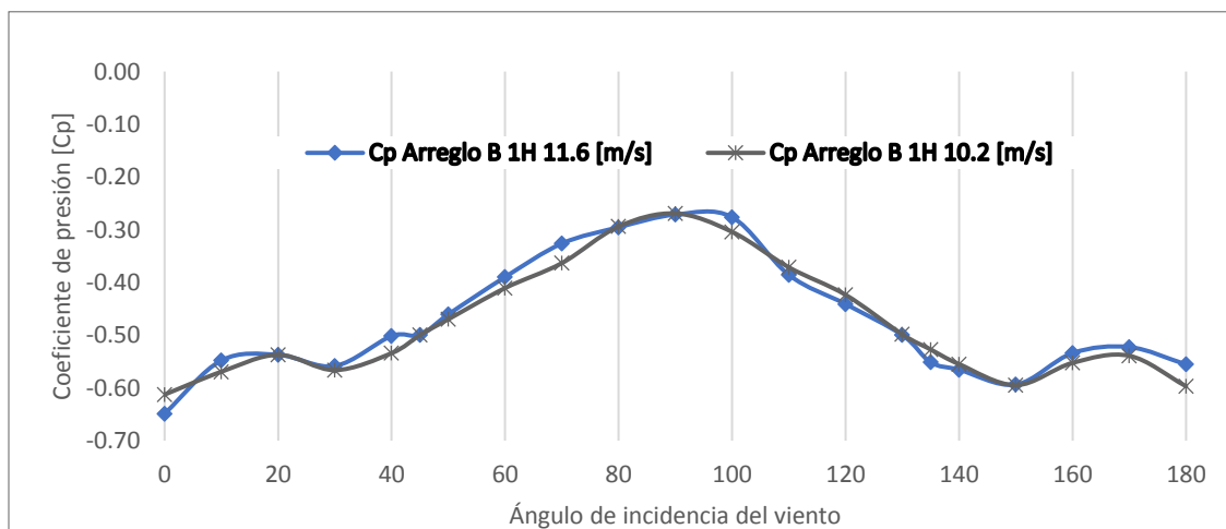
Figura A.3. Cp del Muro 4 del Modelo Aislado variando el ángulo de incidencia del viento.
