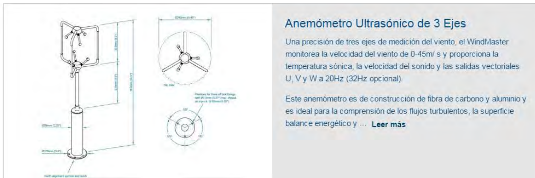
Figura 5.7. Ficha técnica de un Anemómetro ultrasónico
