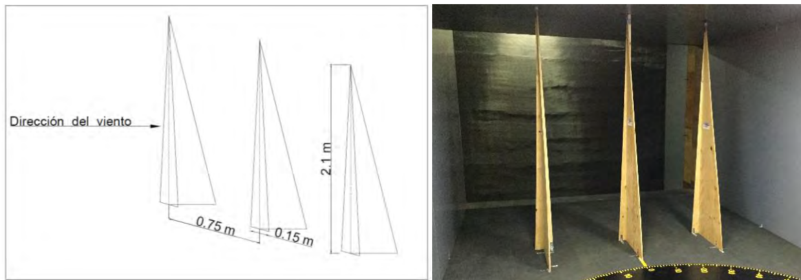
Figura 5.14. Agujas triangulares para generación de vórtices, diseño de Irwin (1980).
