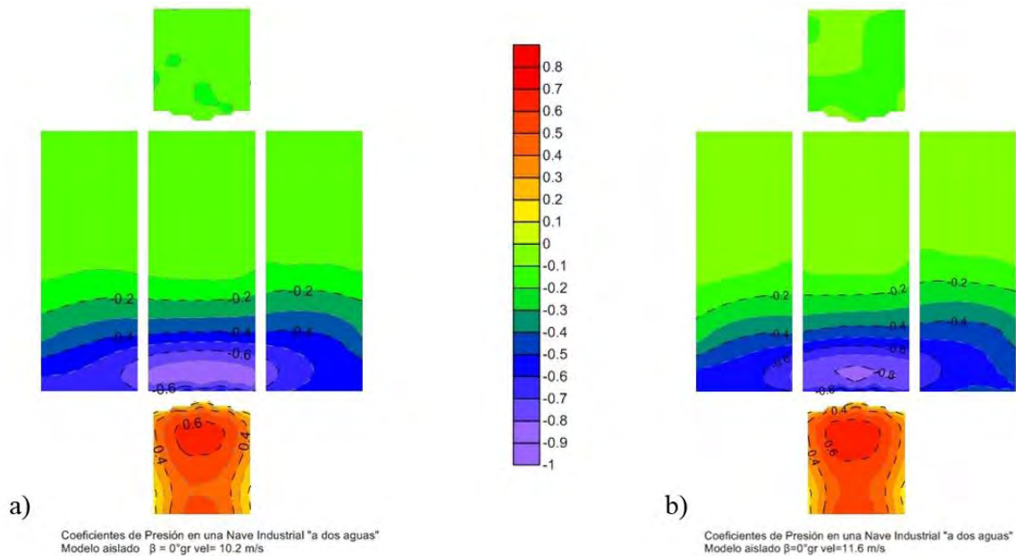
Figura 6.7. En la figura a) El contorno de los Cp a una vel= 10.2 m/s y b) vel=11.6 m/s con una distribución muy similar.
