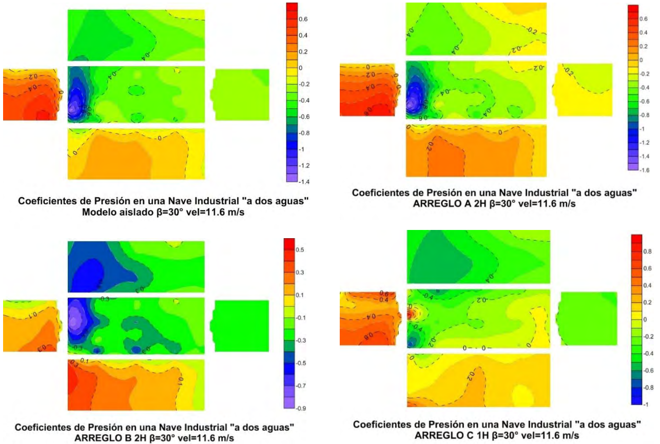
Figura 6.38. Comparación de los contornos de presión para \beta = 30^\circ
