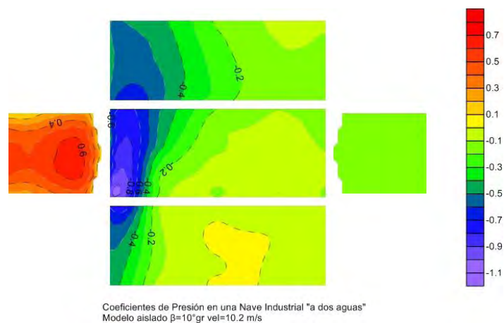
Figura A.5. Contorno de presión del Modelo Aislado con un ángulo de incidencia de 10^\circ gr vel=10.2 m/s
