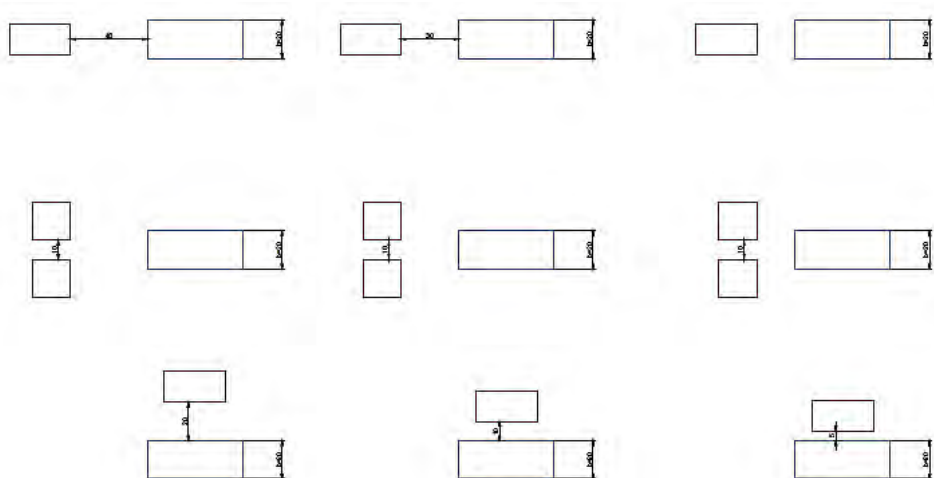
Figura 5.9. Separaciones de los arreglos A,B y C para pruebas experimentales.
