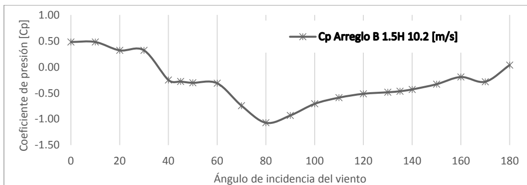
Figura 6.24. Cp Muro 1 Arreglo B 1.5H variando el ángulo de incidencia del viento.
