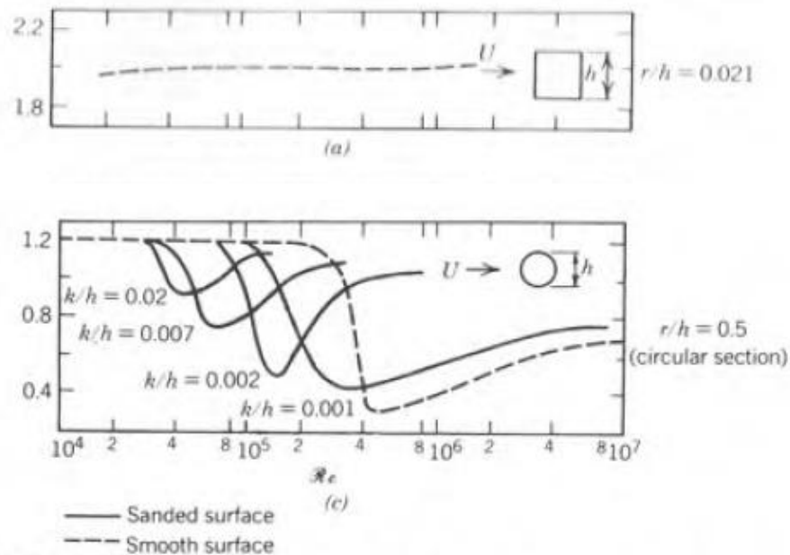
Figura 5.10. Influencia del n^\circ Re en superficies cilíndricas (Simiu & Scanlan, 1996).
