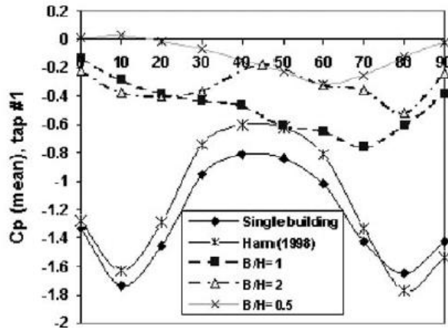
Figura 3.5. Resultados: diferentes arreglos de densidad urbana (Chang & Meroney, 2003)
