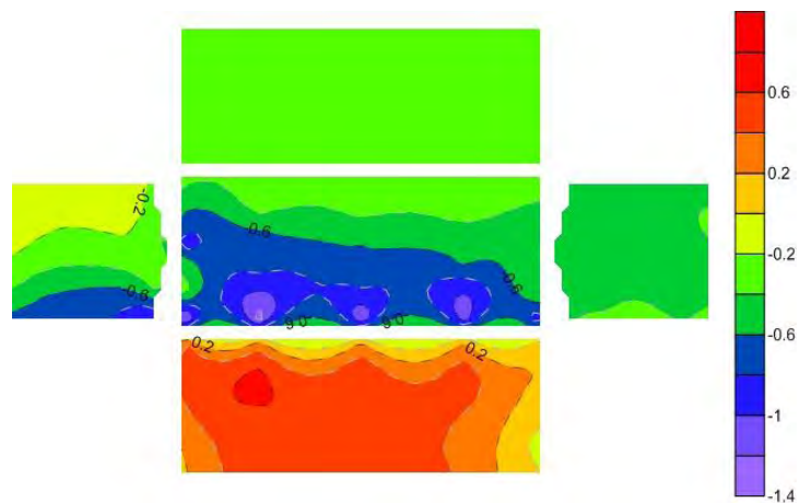
Figura A.5. Contorno de presión del Modelo Aislado con un ángulo de incidencia de 80°gr vel=11.6 m/s
