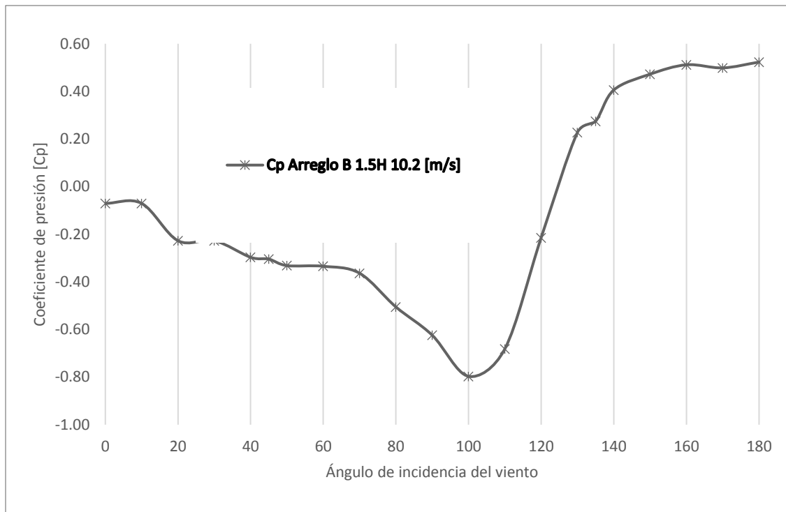
Figura A.22. Cp. del Muro 3 ARREGLO B 1.5H variando el ángulo de incidencia del viento.
