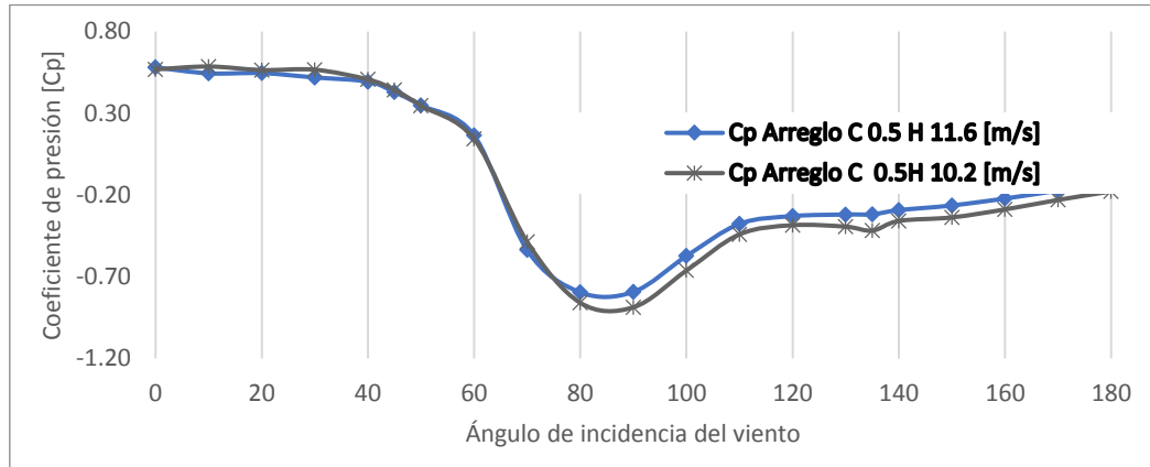
Figura 6.30. Cp del Muro 1 del Arreglo C 0.5H variando el ángulo de incidencia del viento.
