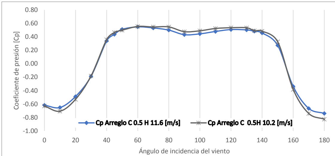
Figura A.27. Cp. del Muro 2 ARREGLO C 0.5H variando el ángulo de incidencia del viento.
