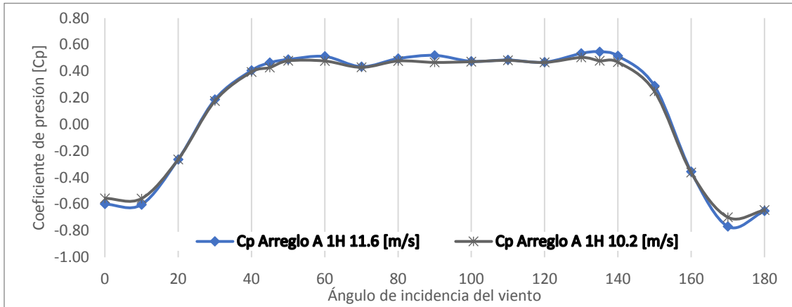
Figura A.9. Cp del Muro 2 ARREGLO A 1H variando el ángulo de incidencia del viento.
