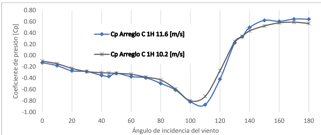
Figura A.34. Cp. del Muro 3 ARREGLO C 1H variando el ángulo de incidencia del viento.
