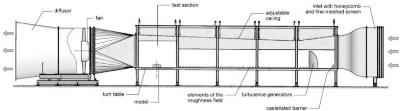
Figura 4.3. Diseño de un túnel de circuito abierto (Holmes, 2003)
