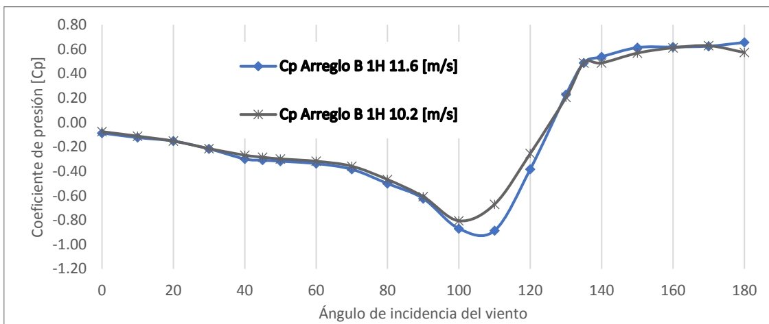
Figura A.19. Cp. del Muro 3 ARREGLO B 1H variando el ángulo de incidencia del viento.
