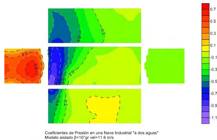
Figura A.6. Contorno de presión del Modelo Aislado con un ángulo de incidencia de 10^\circ gr vel=11.6 m/s
