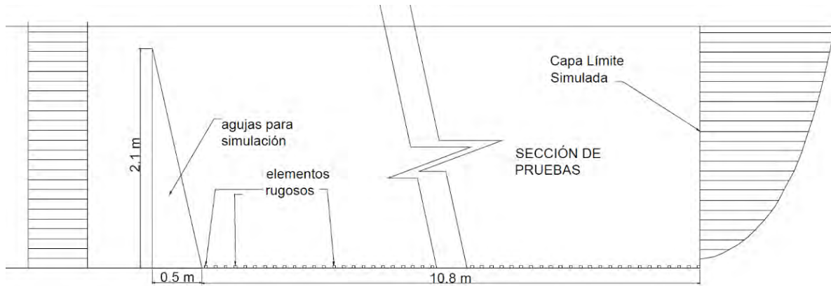
Figura 5.13 Elementos colocados para la simulación de la capa límite de un terreno tipo II.
