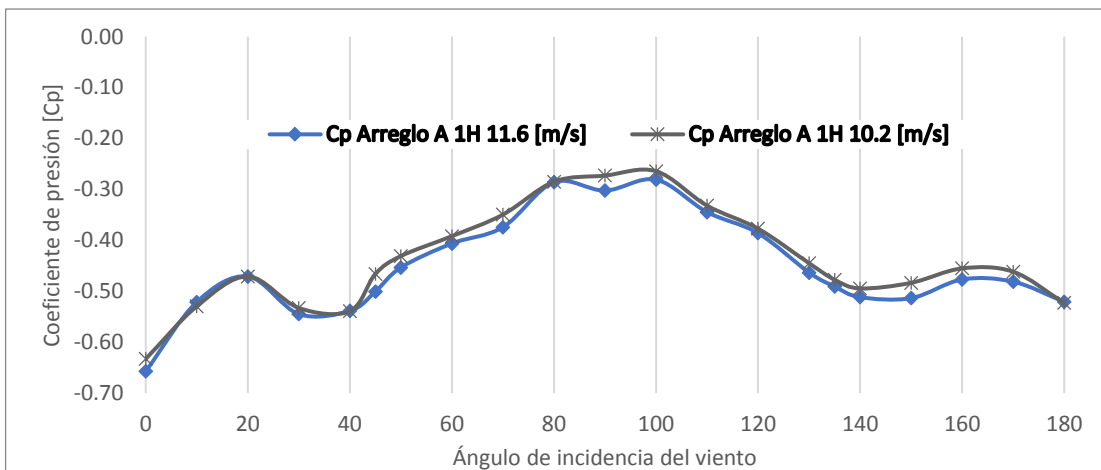
Figura A.11. Cp del Muro 4 ARREGLO A 1H variando el ángulo de incidencia del viento.
