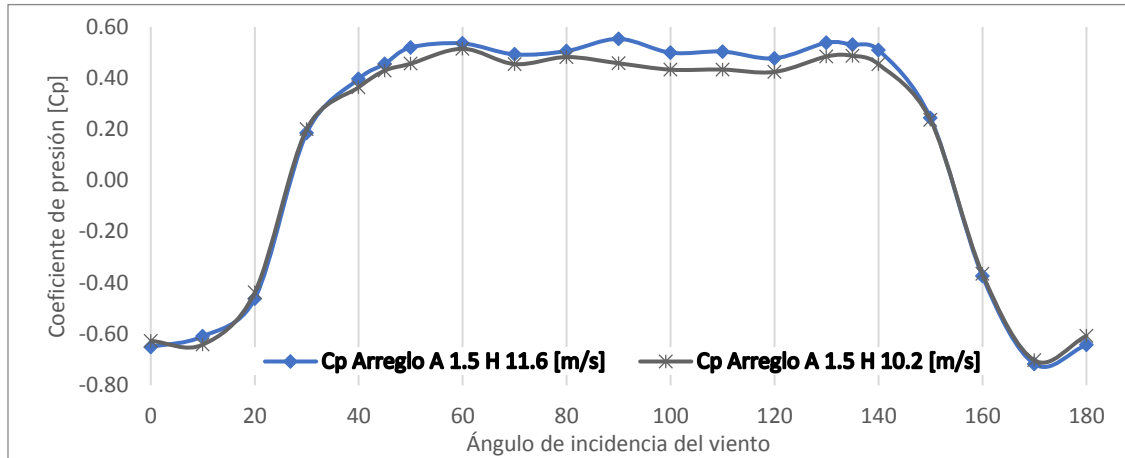
Figura A.12. Cp. del Muro 2 ARREGLO A 1.5H variando el ángulo de incidencia del viento.
