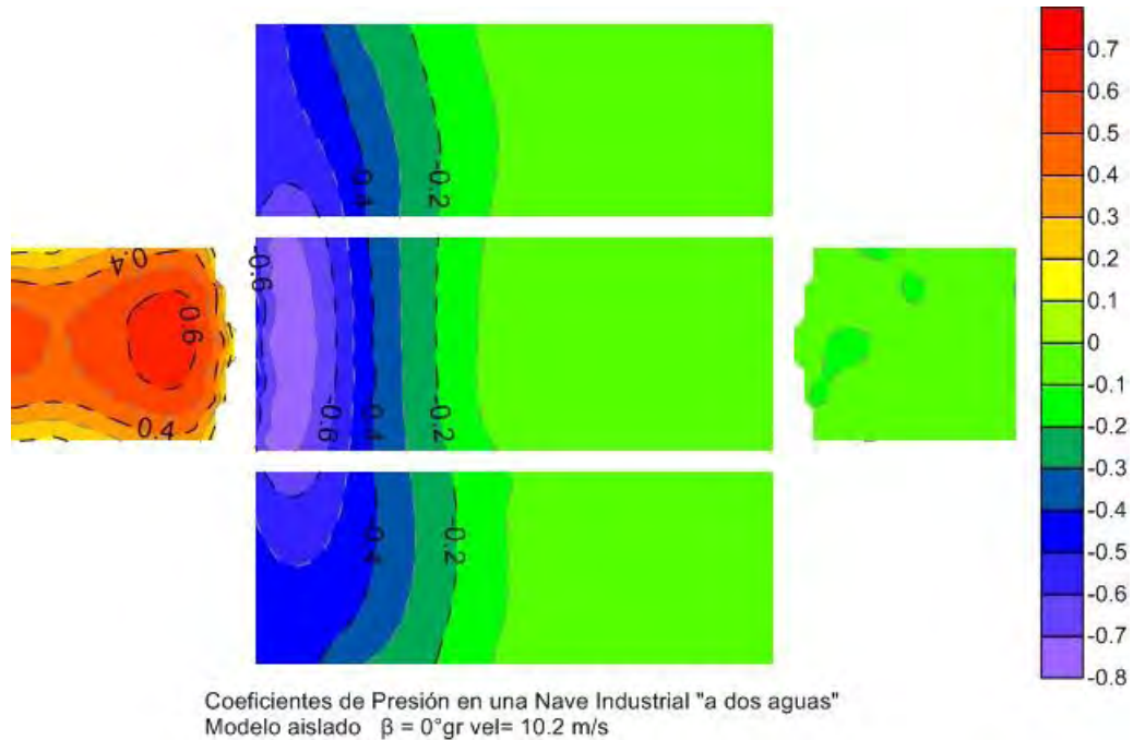
Figura 6.6. Mapa de contorno del Modelo Aislado con ángulo de incidencia de 0 gr y velocidad = 10.2 m/s
