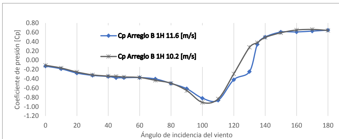
Figura A.2. Cp del Muro 3 del Modelo Aislado variando el ángulo de incidencia del viento.
