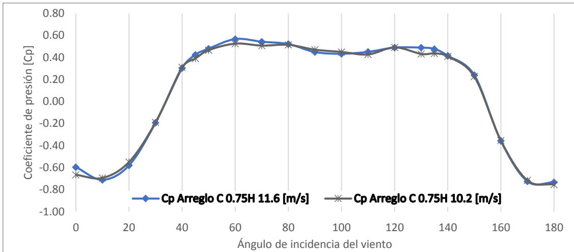
Figura A.30. Cp. del Muro 2 ARREGLO C 0.75H variando el ángulo de incidencia del viento.
