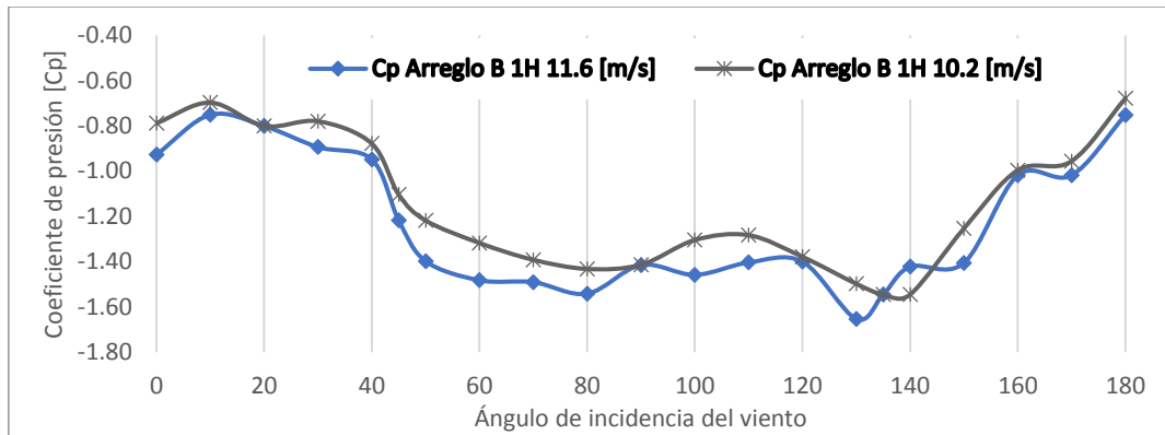
Figura 6.22. Cp de la cubierta del Arreglo B 1H variando el ángulo de incidencia del viento.
