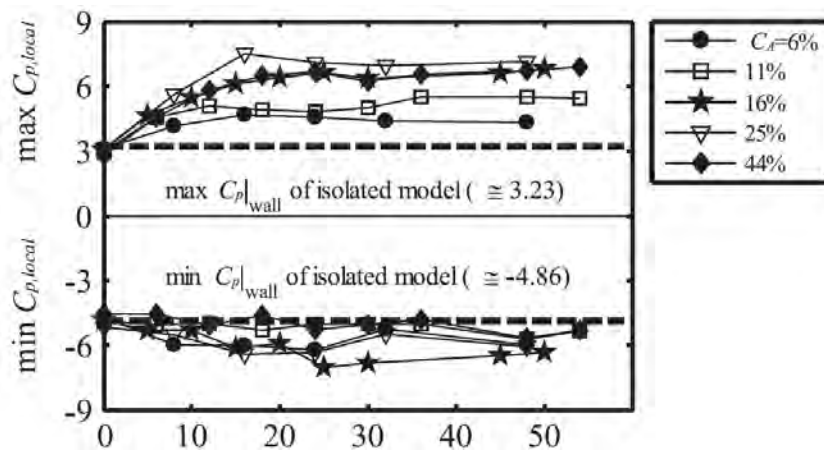
Figura 3.7. Gráfica con Cp pico (Kim, et al., 2015)
