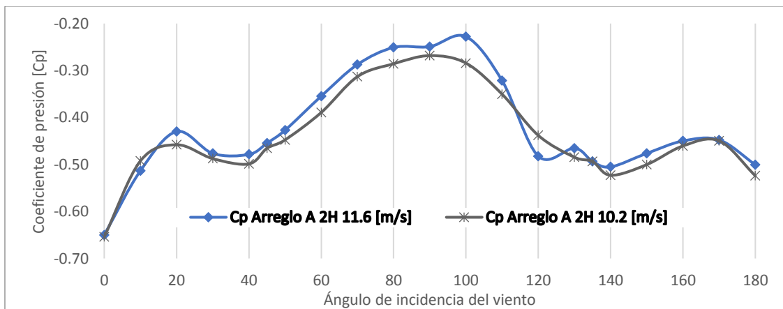
Figura A.17. Cp. del Muro 4 ARREGLO A 2H variando el ángulo de incidencia del viento.
