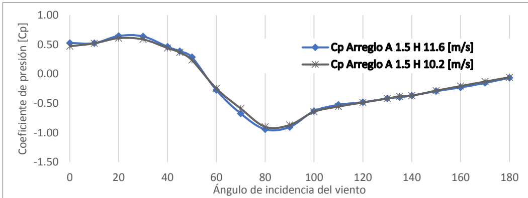
Figura 6.15. Cp del Muro 1 del Arreglo A 1.5H variando el ángulo de incidencia del viento.
