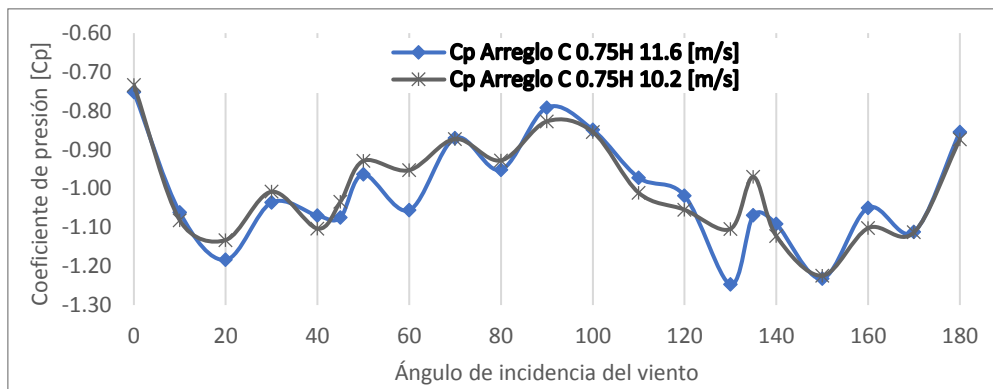
Figura 6.34. Cp cubierta Arreglo C 0.75H variando el ángulo de incidencia del viento.
