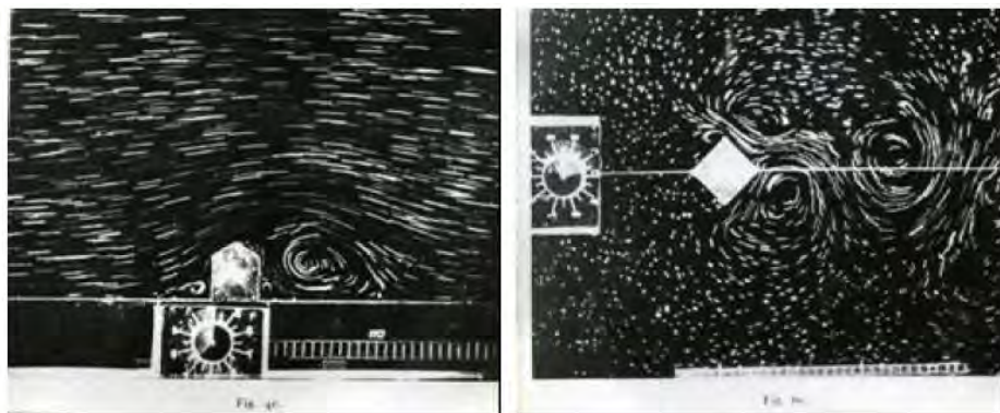
Figura 4.2. Imágenes de experimentos de fluidos desarrollados por Irminger (Geunrts, s.f.)
