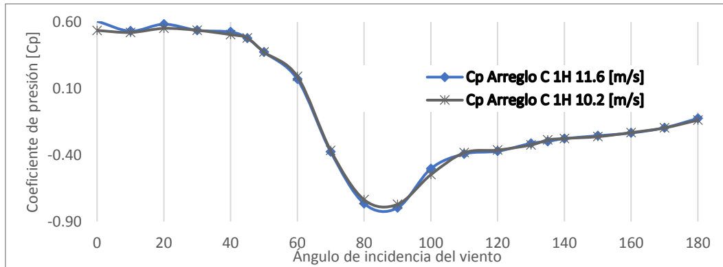
Figura 6.36. Cp del Muro 1 del Arreglo C 1H variando el ángulo de incidencia del viento.
