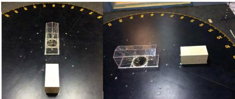
Figura 6.14. Arreglo A con una separación de 30 cm (1.5 H)
