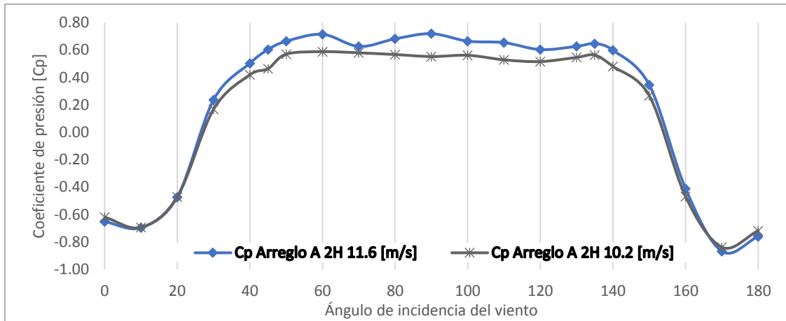
Figura A.15. Cp. del Muro 2 ARREGLO A 2H variando el ángulo de incidencia del viento.
