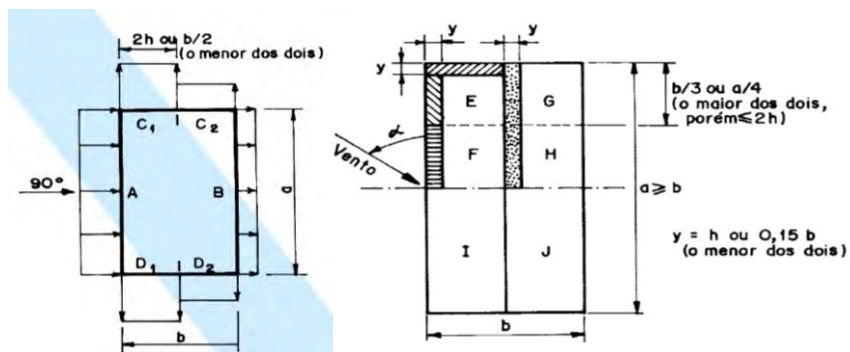
Figura 3.4. Coeficientes de presión para edificaciones a dos aguas. (NBR-6123, 1987)
