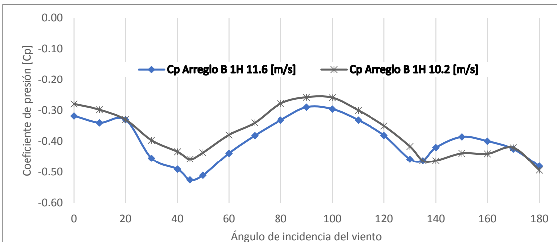
Figura A.20. Cp. del Muro 4 ARREGLO B 1H variando el ángulo de incidencia del viento.
