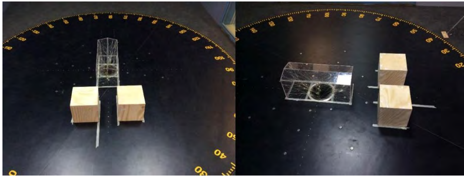
Figura 6.20. Arreglo B con separación de 20 cm (1 H), separación entre los obstáculos 15 cm.
