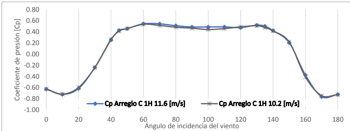
Figura A.33. Cp. del Muro 2 ARREGLO C 1H variando el ángulo de incidencia del viento.
