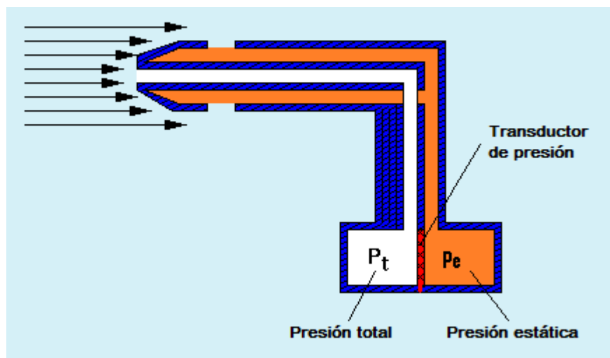
Figura 5.19. Figura esquemática de un tubo de Pitot.
