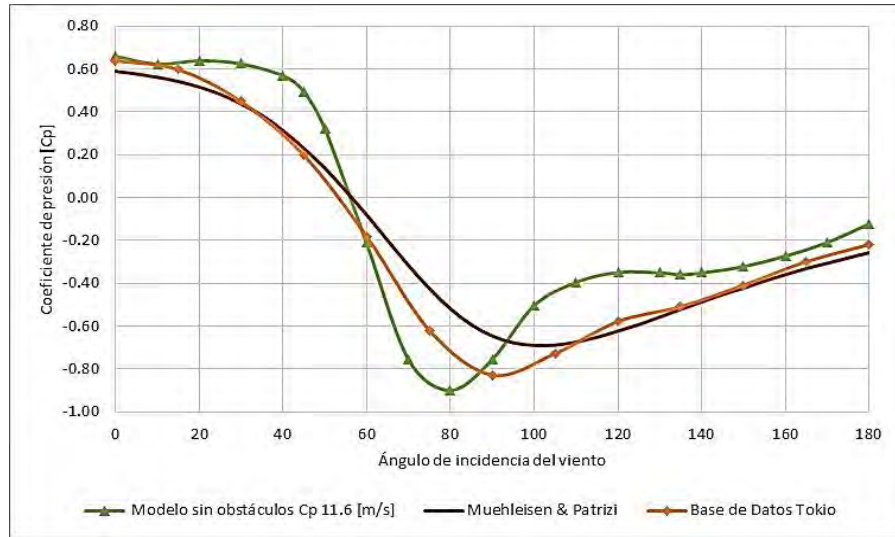
Figura 6.10. Resultados para el Muro 1 de las pruebas experimentales, Muehleisen y la Universidad de Tokio
