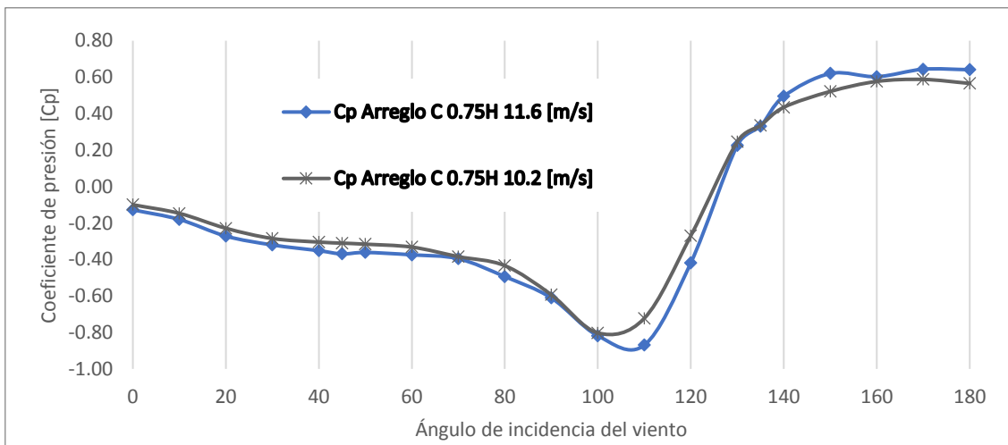
Figura A.31. Cp. del Muro 3 ARREGLO C 0.75H variando el ángulo de incidencia del viento.
