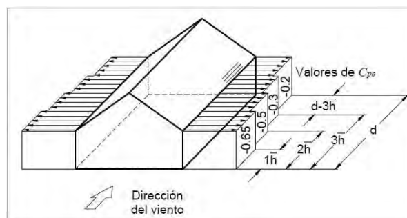
Figura 3.1. Coeficientes de presión para Nave Industrial (MOCDV, 2008)
