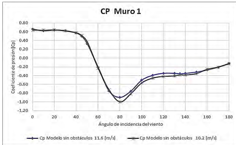
Figura 6.8 Cp del Muro 1 del Modelo Aislado variando el ángulo de incidencia del viento.
