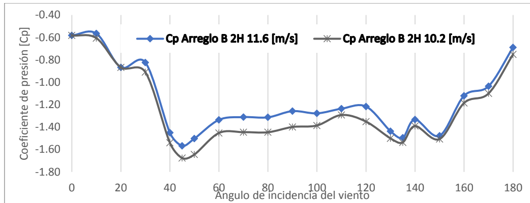
Figura 6.28. Cp de la cubierta del Arreglo B 2H variando el ángulo de incidencia del viento.
