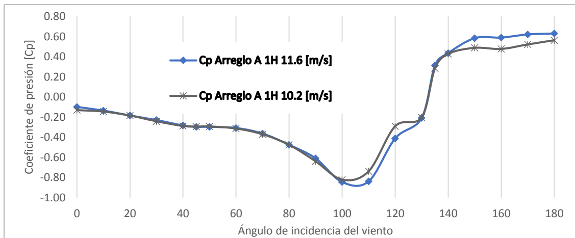
Figura A.10. Cp del Muro 3 ARREGLO A 1H variando el ángulo de incidencia del viento.
