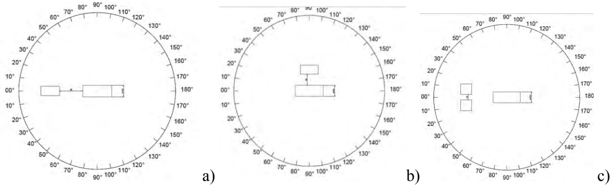
Figura 5.8. Arreglos de obstáculos para pruebas de modelo rígido: a) arreglo A, b) arreglo B y c) arreglo C.
