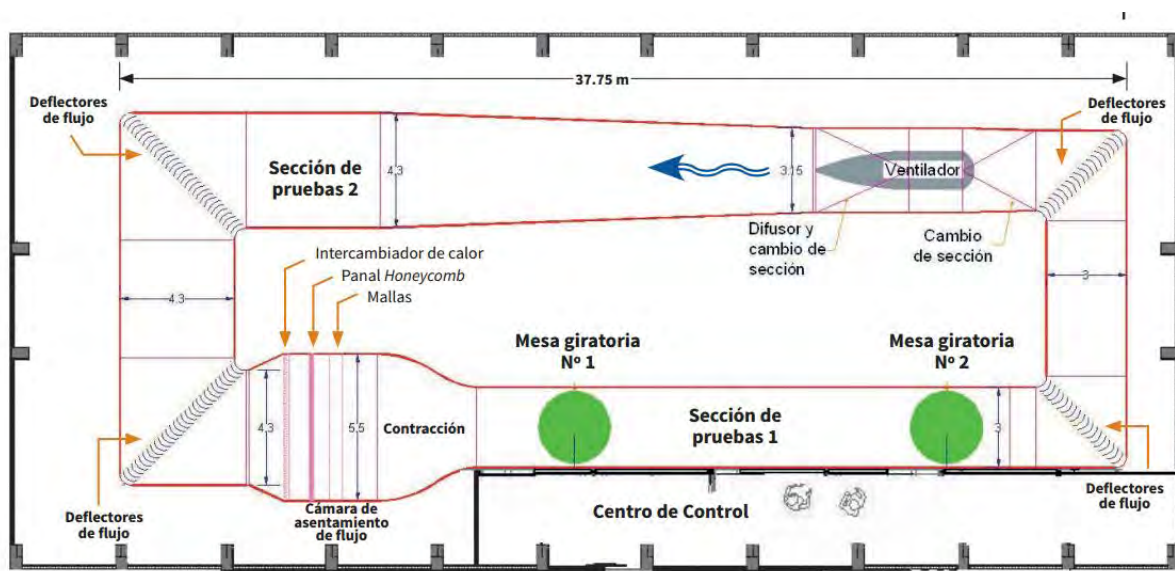
Figura 4.12. Diagrama del túnel de circuito cerrado de la UNAM.
