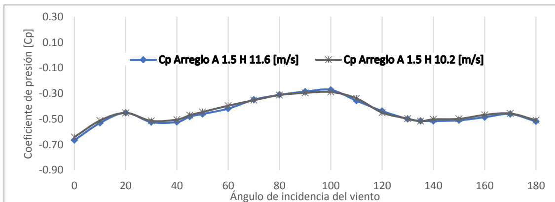
Figura A.14. Cp. del Muro 4 ARREGLO A 1.5H variando el ángulo de incidencia del viento.
