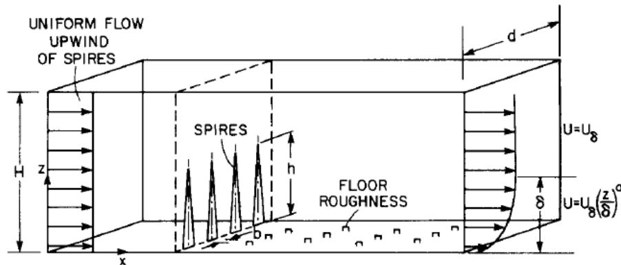
Figura 5.12 Generación de capa límite en túnel de viento con el diseño de (Irwin, 1980)
