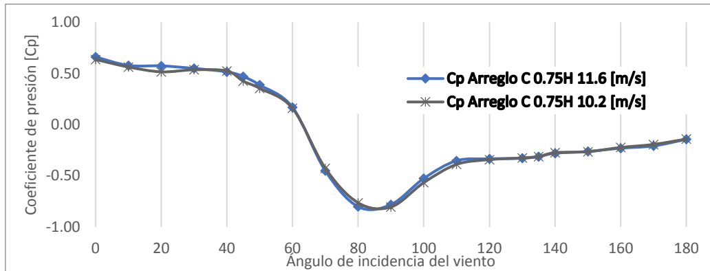
Figura 6.33. Cp Muro 1 Arreglo C 0.75H variando el ángulo de incidencia del viento.
