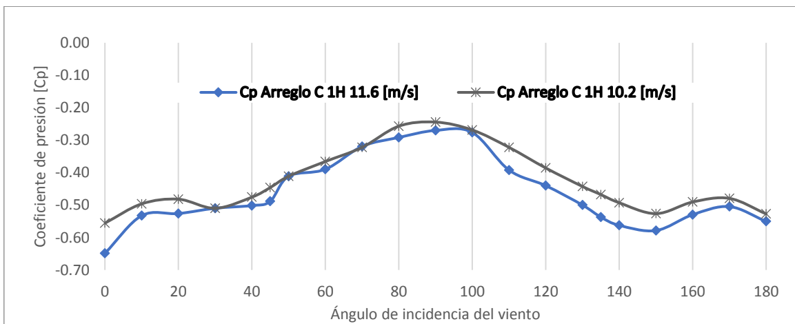
Figura A.35. Cp. del Muro 4 ARREGLO C 1H variando el ángulo de incidencia del viento.
