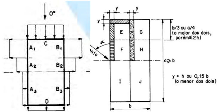
Figura 3.3. Coeficientes de presión para edificaciones a dos aguas. (NBR-6123, 1987)
