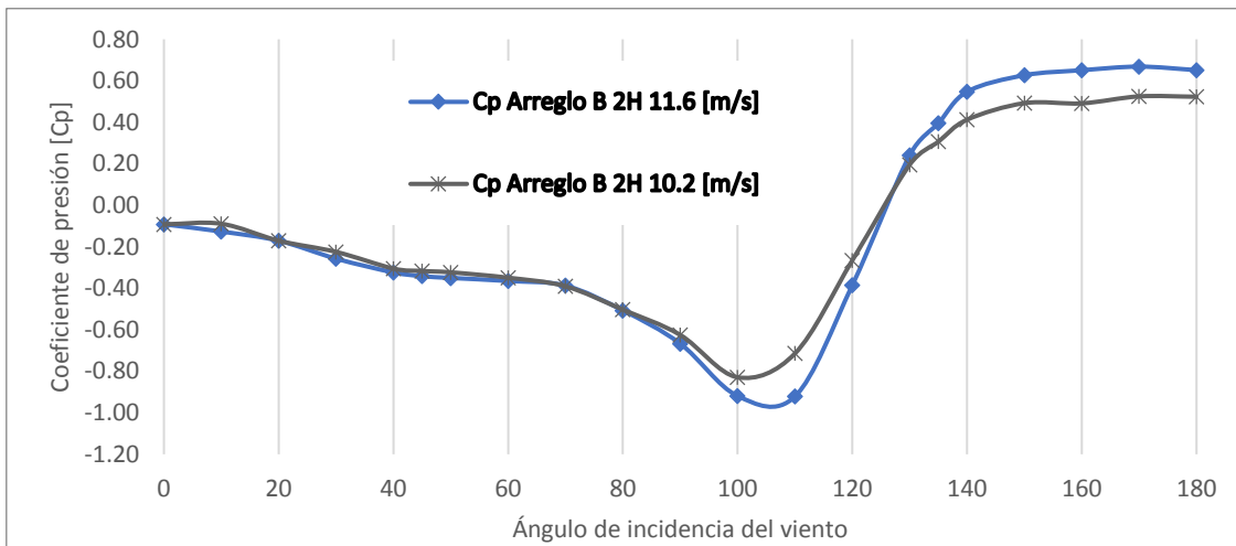
Figura A.25. Cp. del Muro 3 ARREGLO B 2H variando el ángulo de incidencia del viento.
