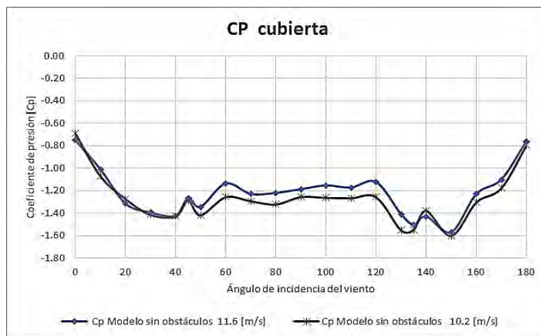
Figura 6.9 Cp de cubierta del Modelo Aislado variando ángulo de incidencia del viento.
