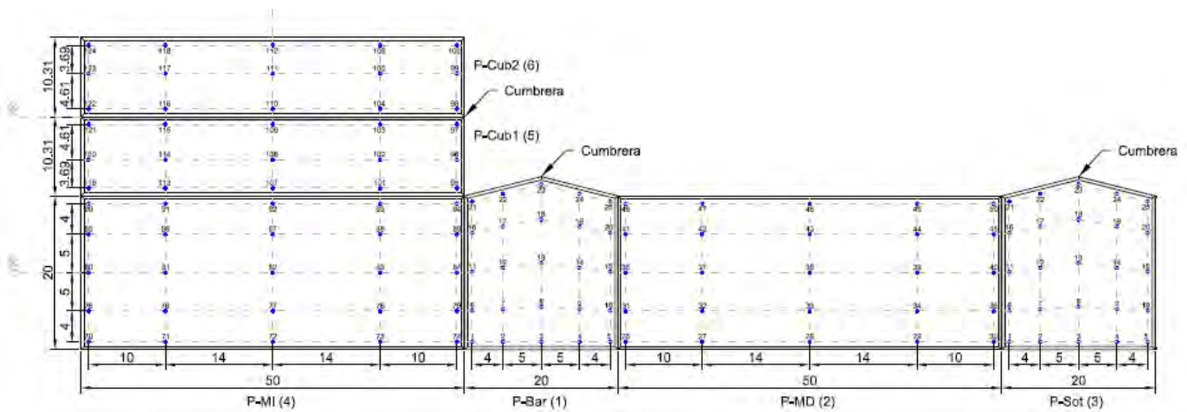
Figura 5.3. Distribución de los taps en el modelo de acrílico.
