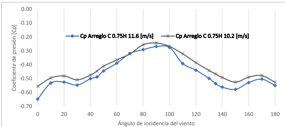
Figura A.32. Cp. del Muro 4 ARREGLO C 0.75H variando el ángulo de incidencia del viento.
