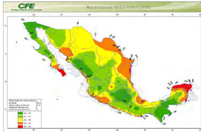
Figura 5.6. Mapa de Isotacas para periodo de Retorno de 200 años (MOCDV, 2008)
