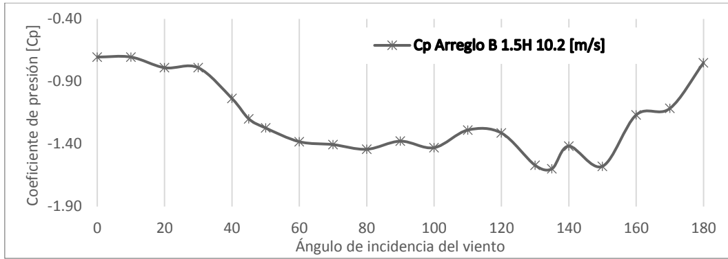
Figura 6.25. Cp cubierta Arrreglo B 1.5H variando el ángulo de incidencia del viento.
