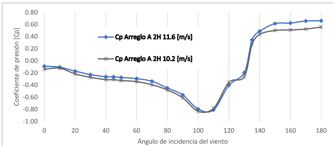
Figura A.16. Cp. del Muro 3 ARREGLO A 2H variando el ángulo de incidencia del viento.
