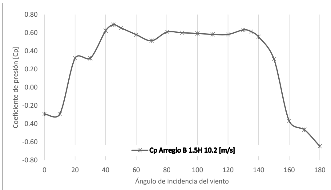
Figura A.21. Cp. del Muro 2 ARREGLO B 1.5H variando el ángulo de incidencia del viento.
