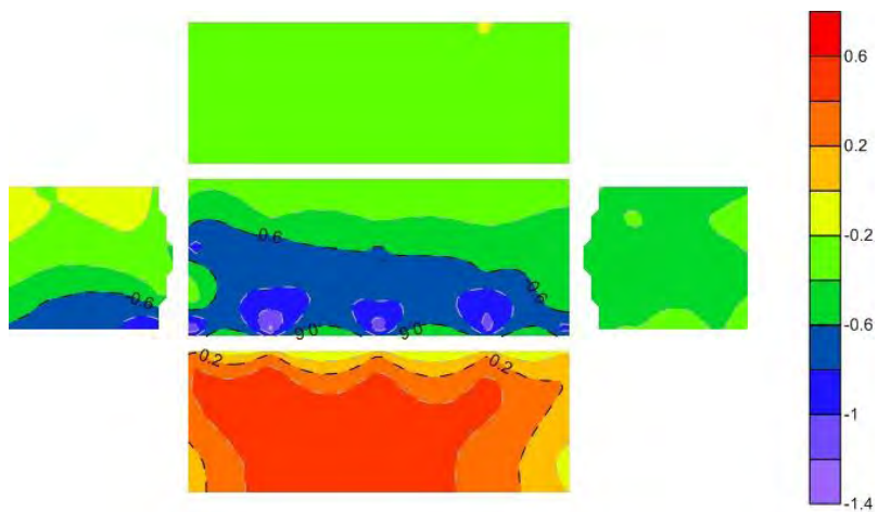
Figura A.6. Contorno de presión del Modelo Aislado con un ángulo de incidencia de 80°gr vel=10.2 m/s
