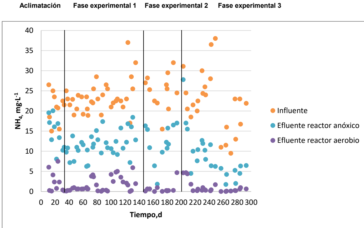
Figura 4.11 Valores obtenidos para nitrógeno amoniacal en el influente y efluentes de cada reactor.
