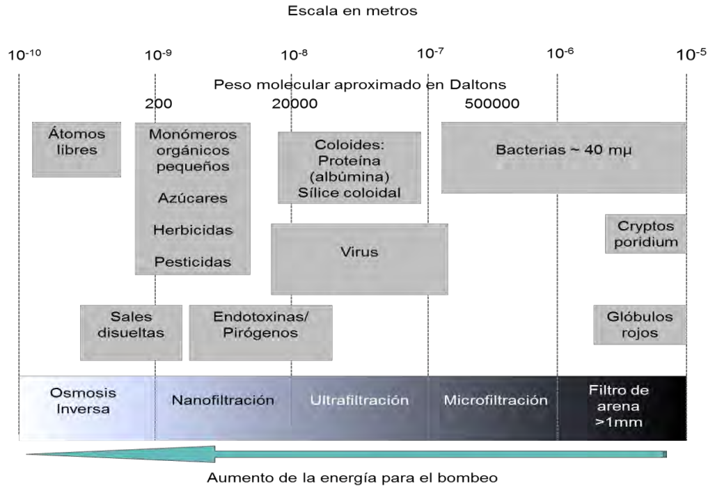
Figura 2.8 Comparación de los procesos de filtración de membranas (Judd and Jefferson, 2003).
