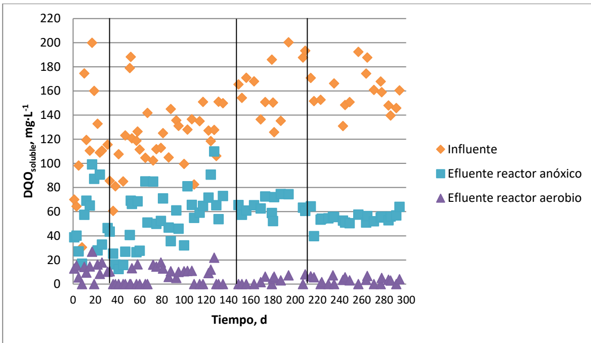
Figura 4.6 Valores de DQO soluble en el influente y efluente.
