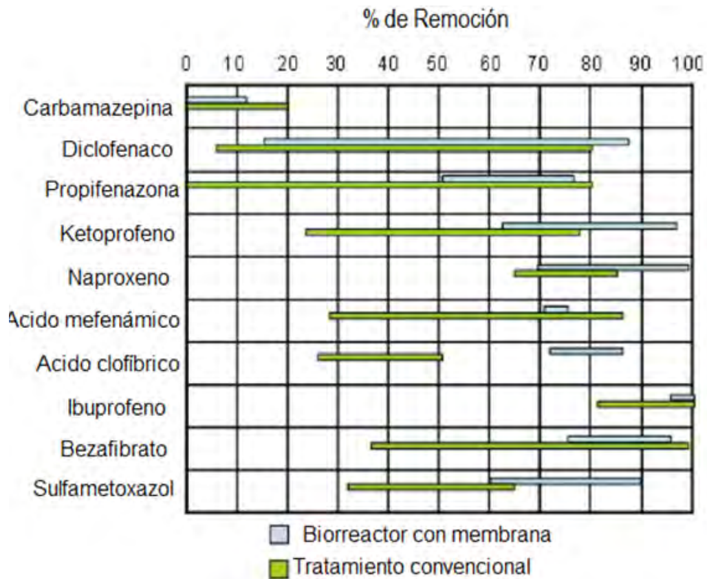
Figura 2.14 Remoción de fármacos en un biorreactor de membrana y un tratamiento convencional (Radjenovic et al., 2008).
