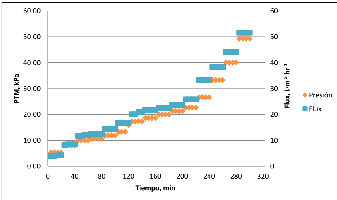
Figura 4.1 Comportamiento de la PTM y el flux con agua potable.
