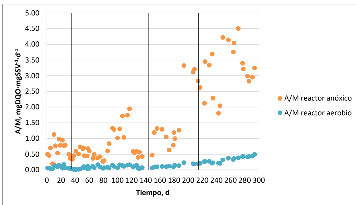
Figura 4.10 Variación de la relación A/M en cada reactor durante las diferentes fases.
