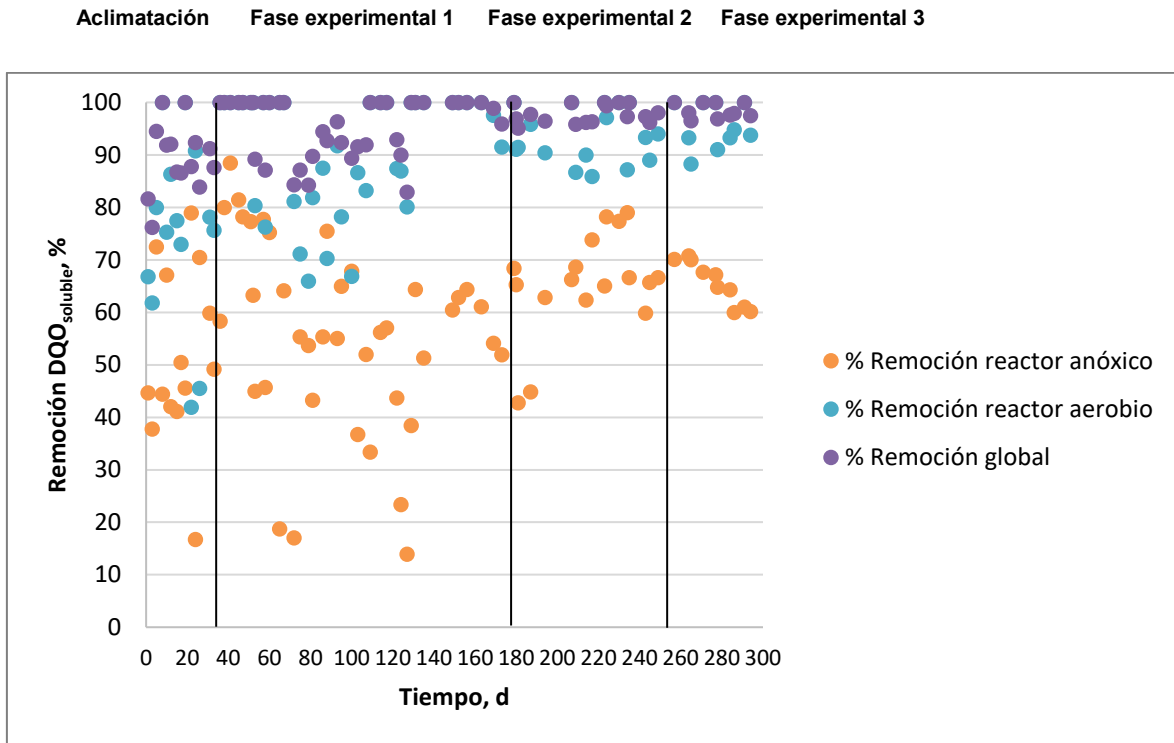
Figura 4.7 Remociones de DQO soluble en cada reactor y global en el sistema.
