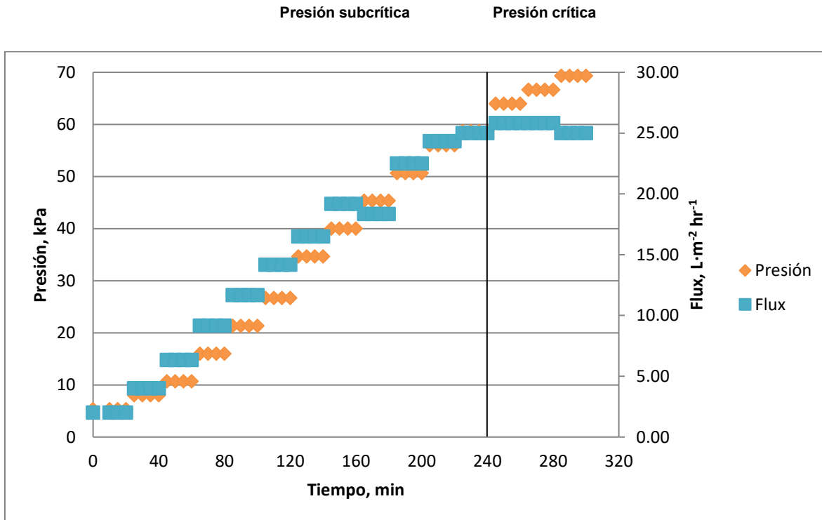
Figura 4.2 Comportamiento de la PTM y el flux con agua residual y biomasa.
