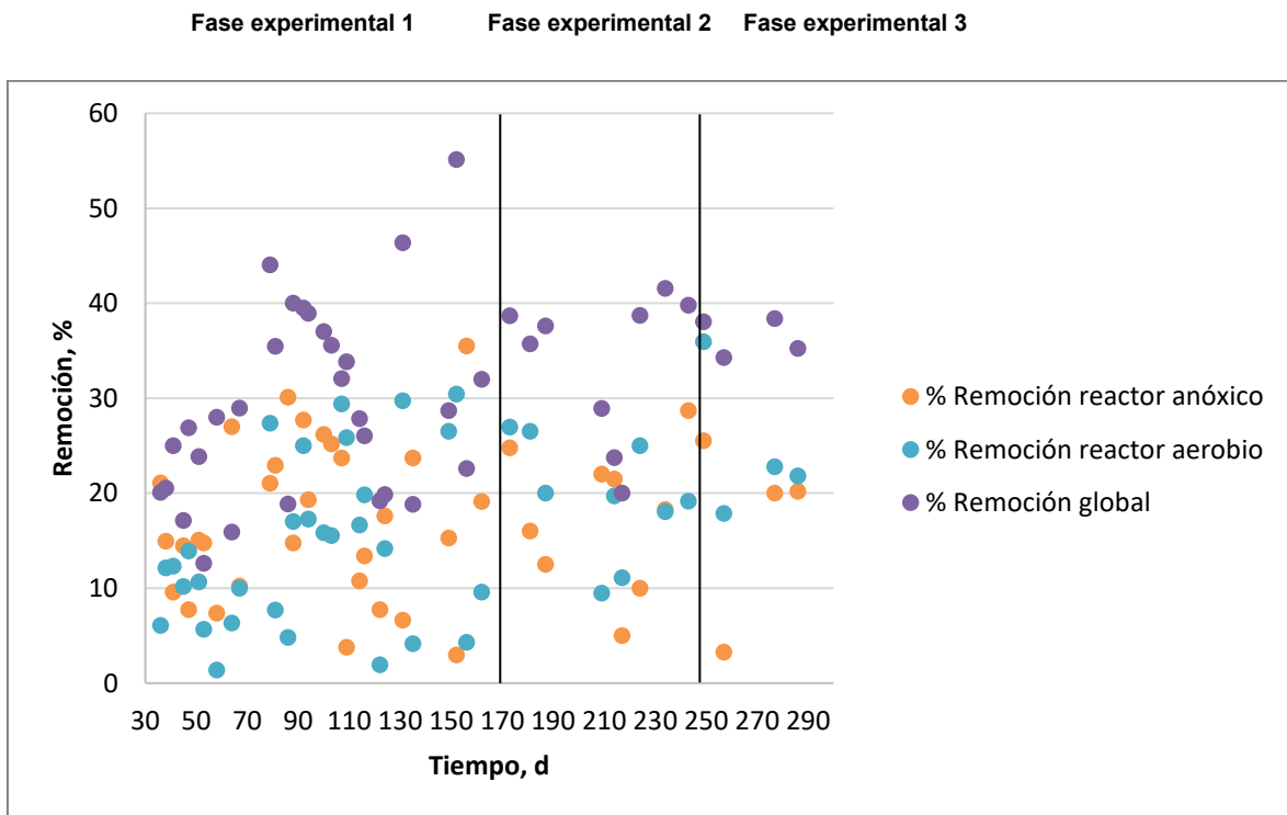
Figura 4.14 Remociones de P-PO 4 en cada reactor y global en el sistema.
