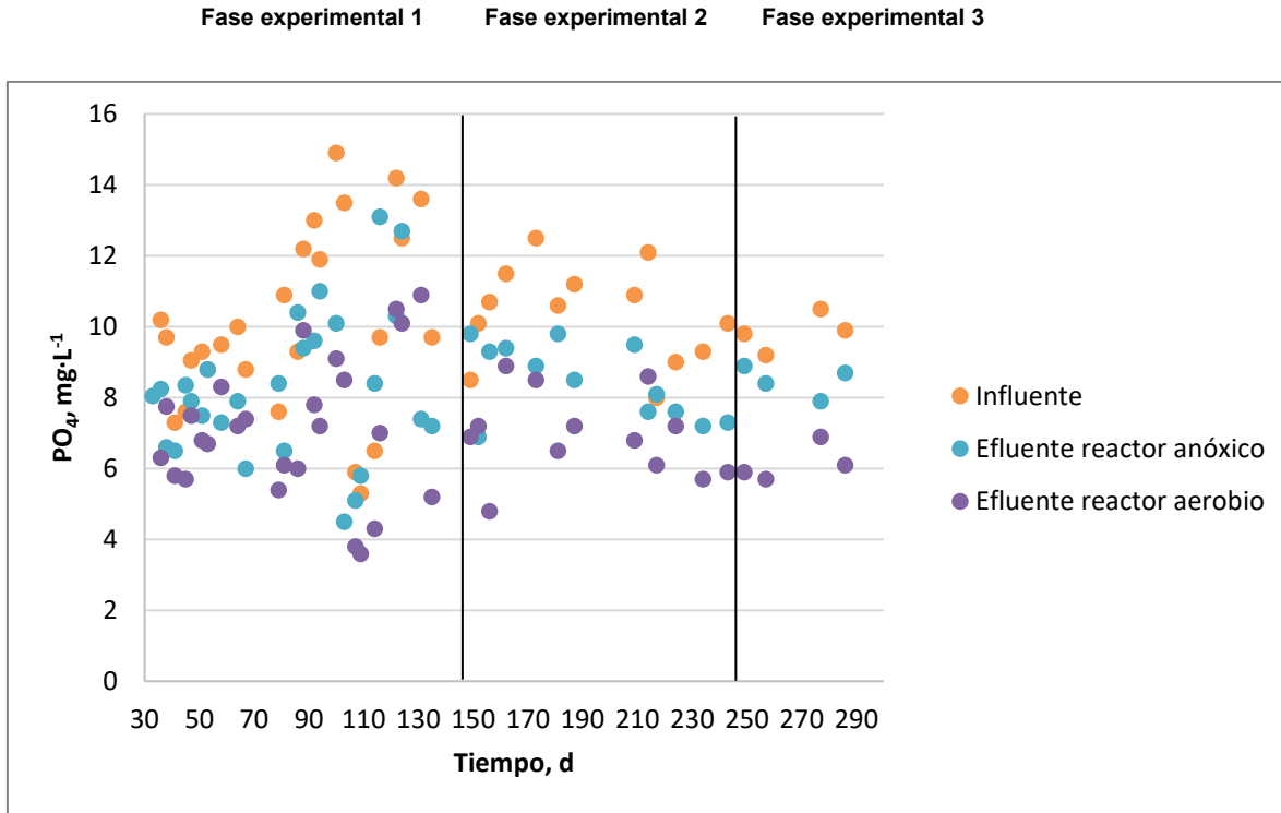
Figura 4.13 Valores de P-PO 4 en influente y efluente de cada reactor.
