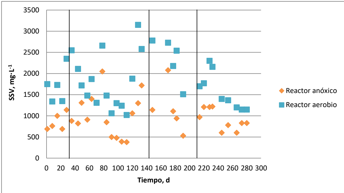
Figura 4.9 Valores de SSV en el reactor anóxico y aerobio.
