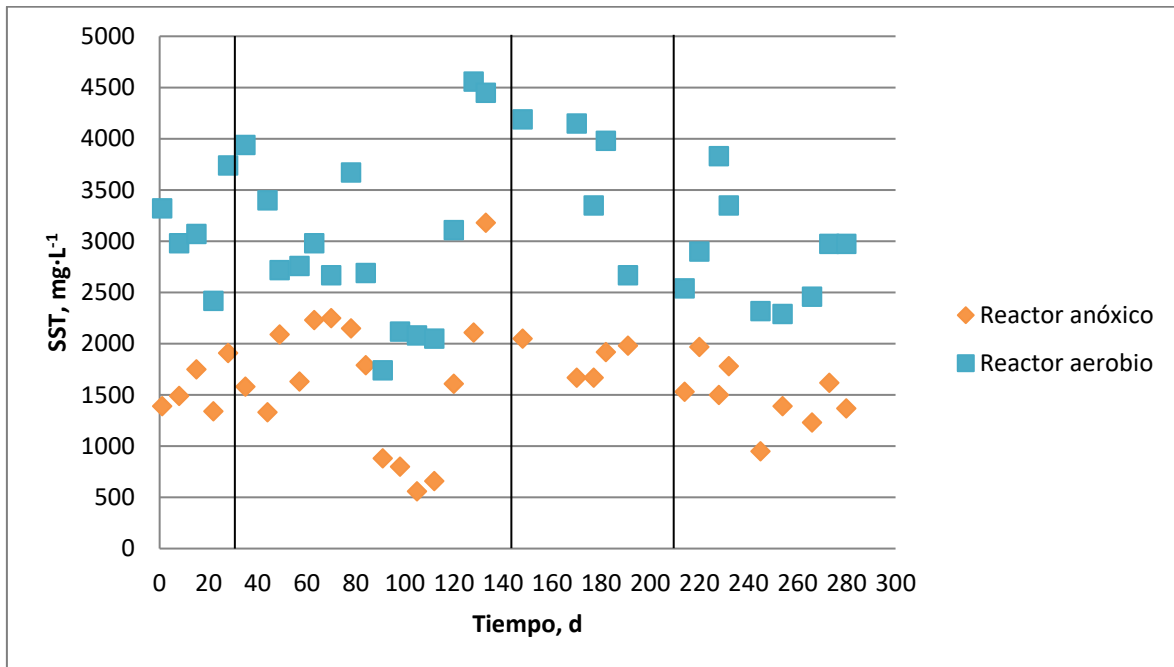
Figura 4.8 Valores de SST en el reactor anóxico y aerobio.
