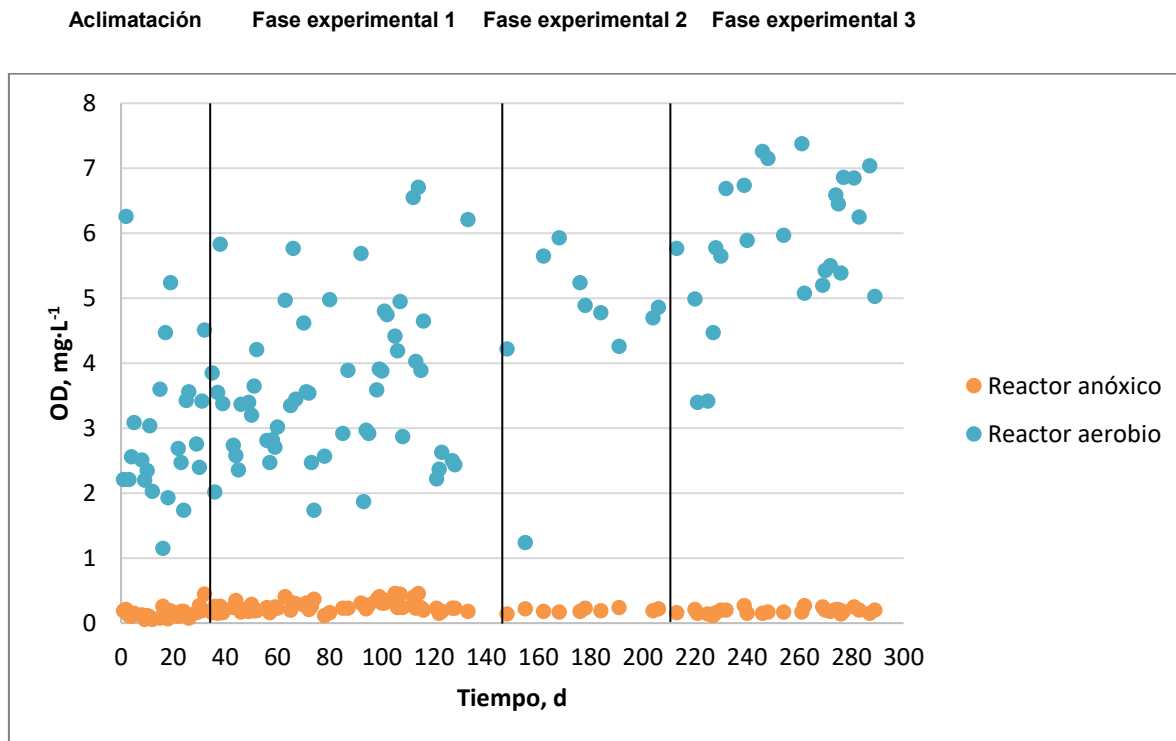
Figura 4.5 Valores de OD en cada reactor.
