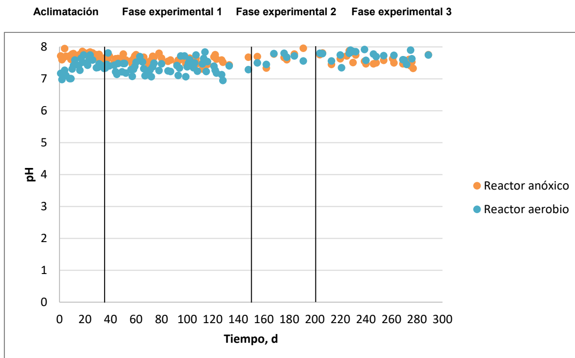
Figura 4.3 Valores de pH en el reactor anóxico y aerobio.
