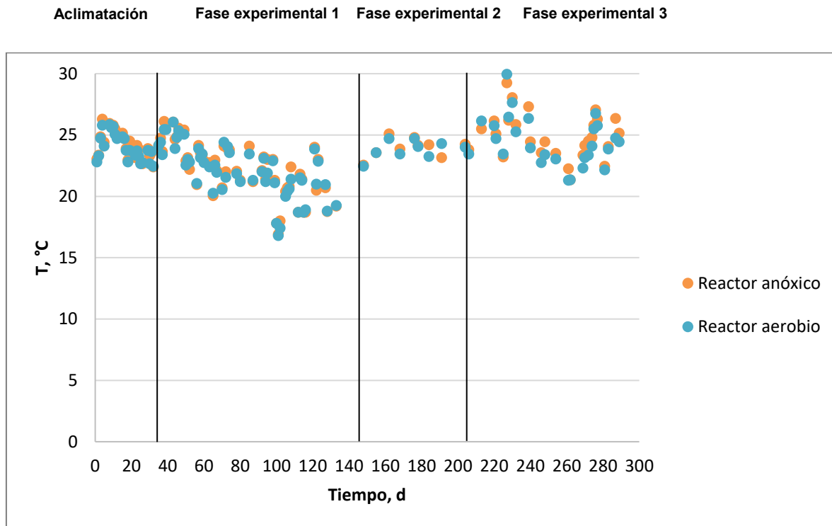
Figura 4.4 Valores de temperatura en el sistema experimental.
