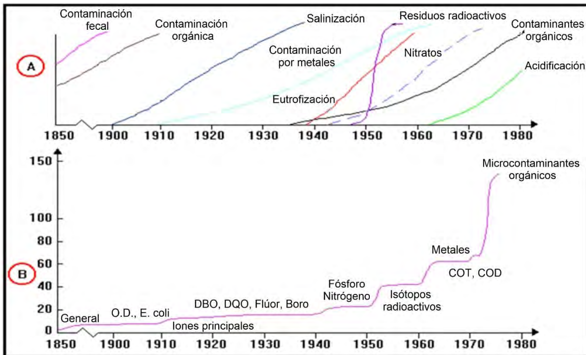
Figura 2.1 Evolución conceptual de los principales problemas de calidad del agua en América del Norte y Europa occidental (A) y los indicadores de calidad del agua (B).
