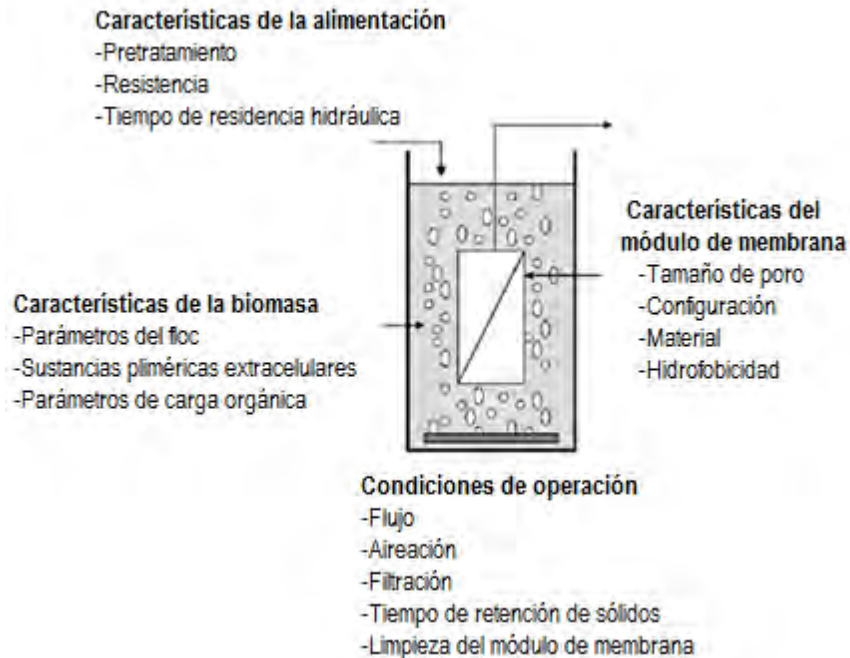
Figura 2.11 Factores de colmatación en los sistemas BRM.
