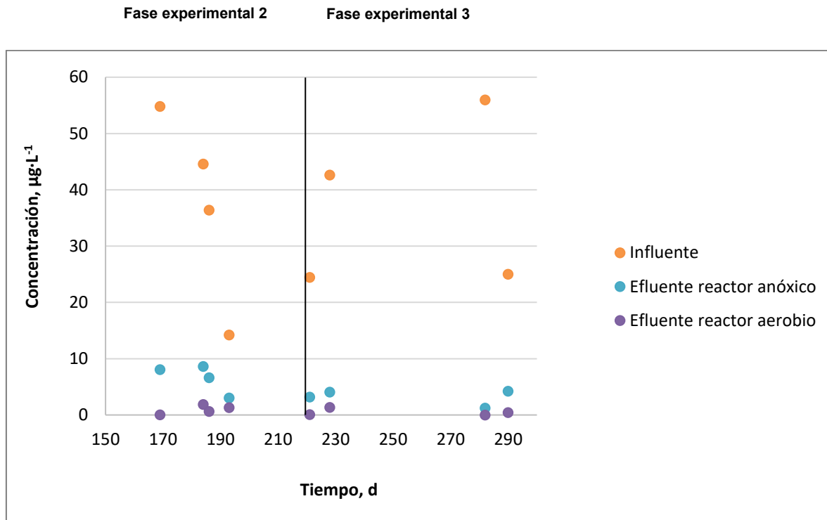
Figura 4.17 Valores de metoprolol en el influente y efluente de los reactores.
