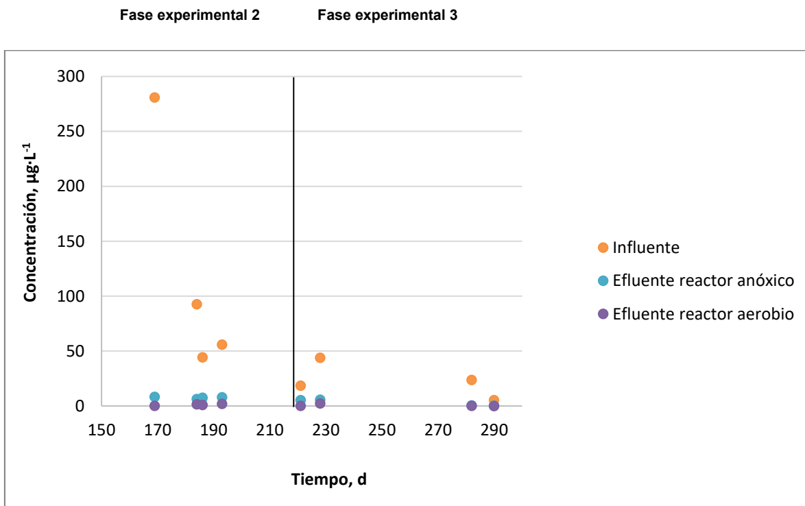
Figura 4.15 Valores de ácido mefenámico en el influente y efluente de los reactores.
