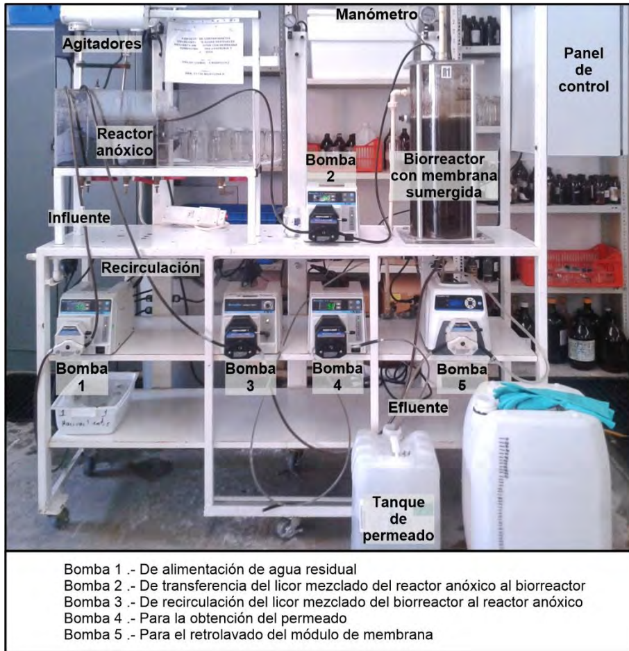
Figura 3.2 Sistema experimental en operación.
