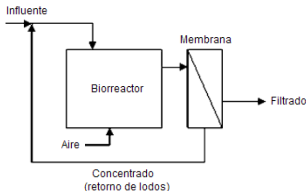
Figura 2.12 Biorreactor con membranas externa.
