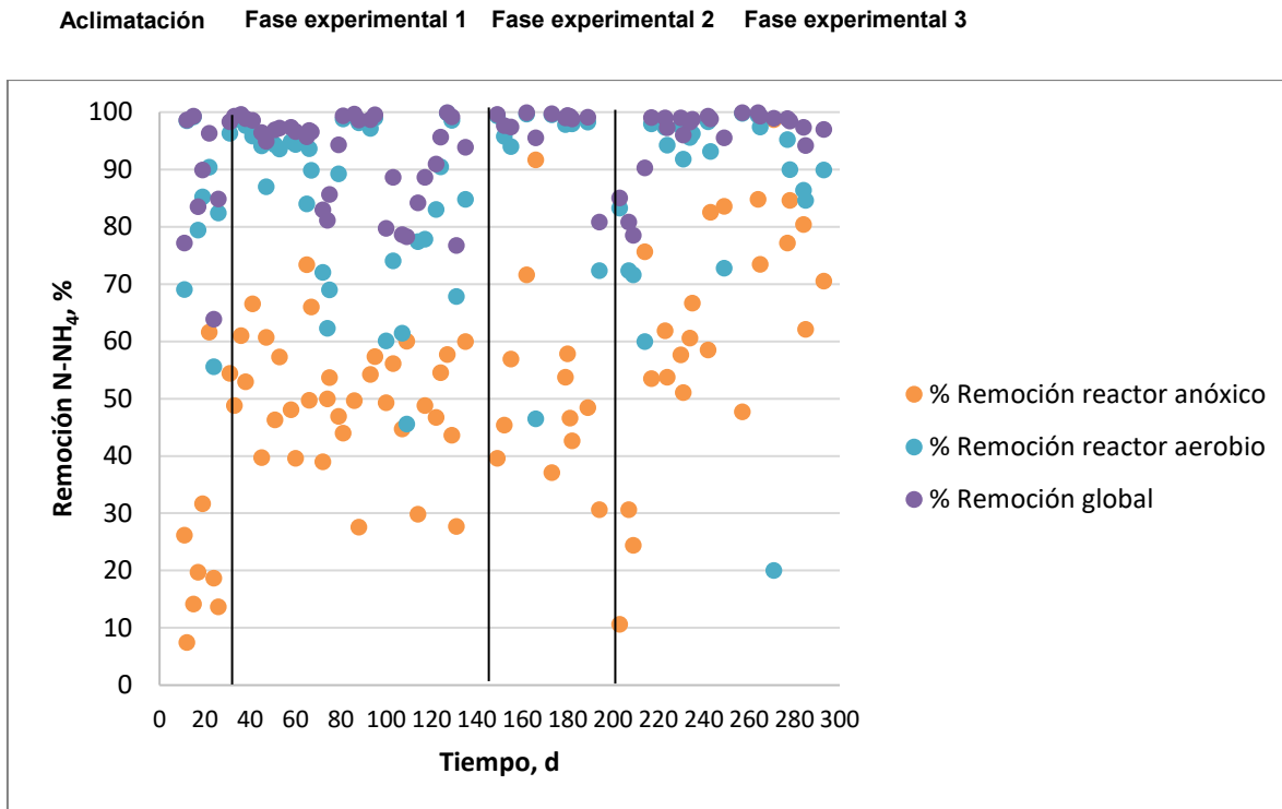
Figura 4.12 Remociones de \text{N-NH}_4 en cada reactor y global en el sistema.
