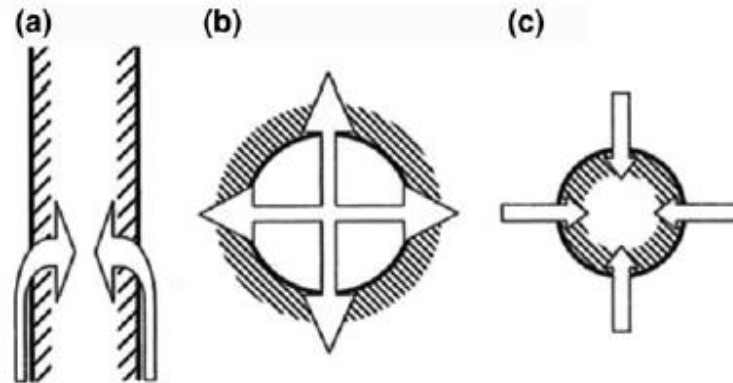
Figura 2.9 Esquema que muestra el flujo a través de la membrana: (a) placa y marco de hoja plana, (b) multitubular y (c) fibra hueca.
