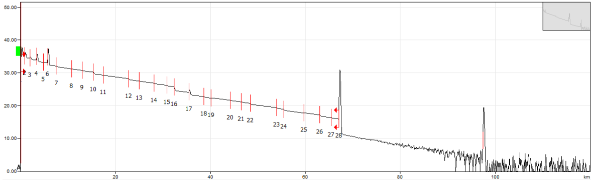
Figura 3.27. Trazo de referencia puerto 2 del OTH, monitoreo. Anillo DGTIC-CINVESTAV-UAM-DGTIC.
