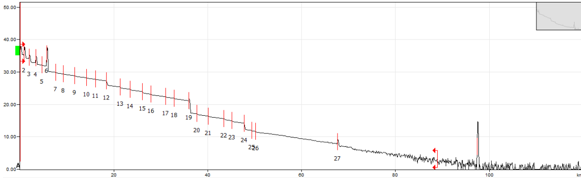
Figura 3.29. Trazo de referencia definitiva puerto 1 del OTH, monitoreo. Anillo DGTIC-UAM-CINVESTAV-DGTIC
