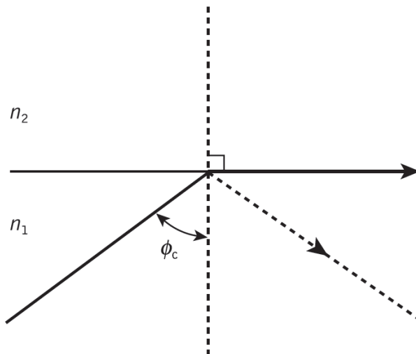
Figura 1.3. Ángulo crítico [7].
