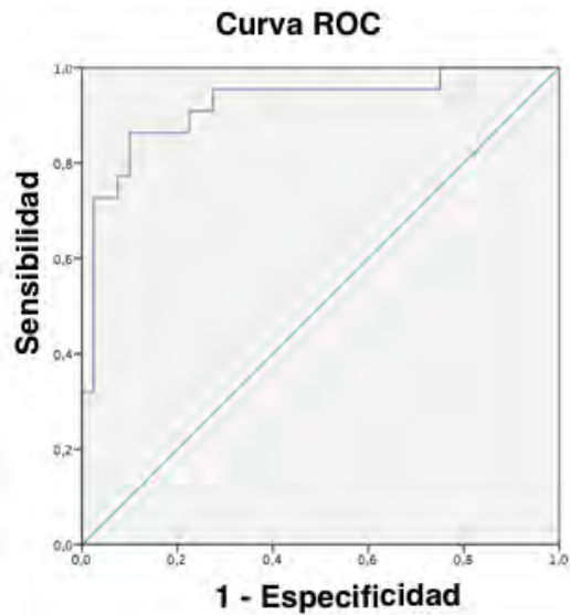
Figura 8: Curva ROC-AUC para anticuerpos anti-vimentina citrulinada.
