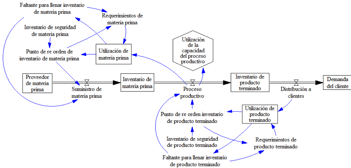
Figura B1.8. Construcción del modelo de simulación programado parte 2.
