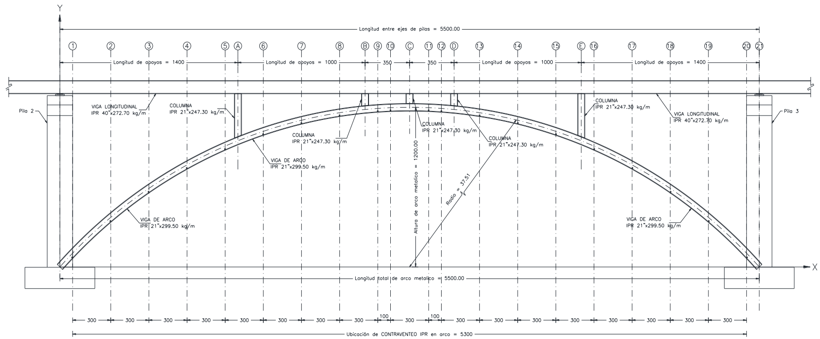
Figura 5.39 Elevación de contravento IPR de arco metálico.
