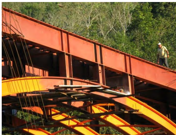
Figura 5.50 Trabajos finales de soldado en los atizadores.
