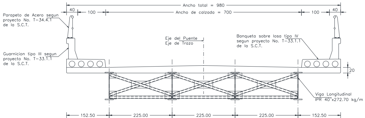
Figura 5.27 Sección transversal de contraenteo en vigas IPR 40"x272.70 kg/m (diafragma).
