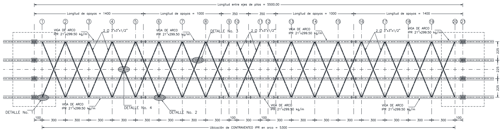
Figura 5.40 Planta de contravento IPR de arco metálico.
