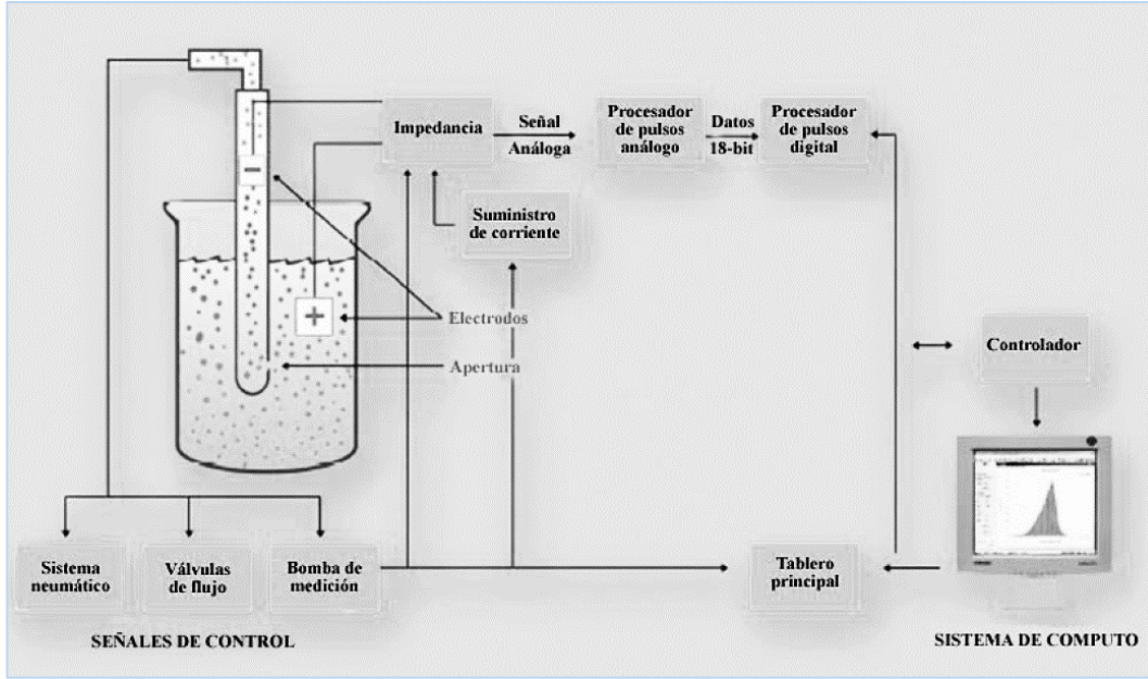
FIGURA 3 DIAGRAMA DEL FUNCIONAMIENTO DEL COULTER COUNTER
