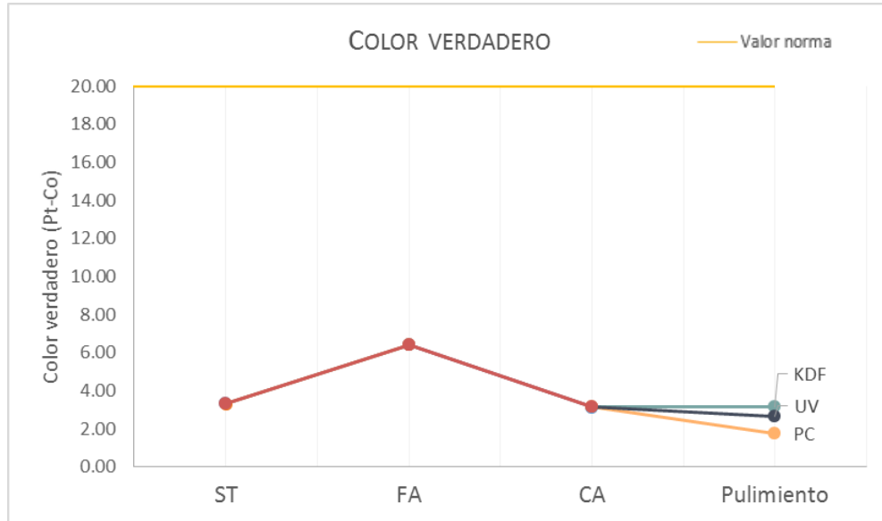
GRÁFICA 11 RESULTADOS DEL COLOR VERDADERO PARA LA PLANTA PILOTO
