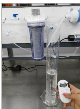
FIGURA 14 MEDICIÓN DEL GASTO DE LA BARRERA KDF
