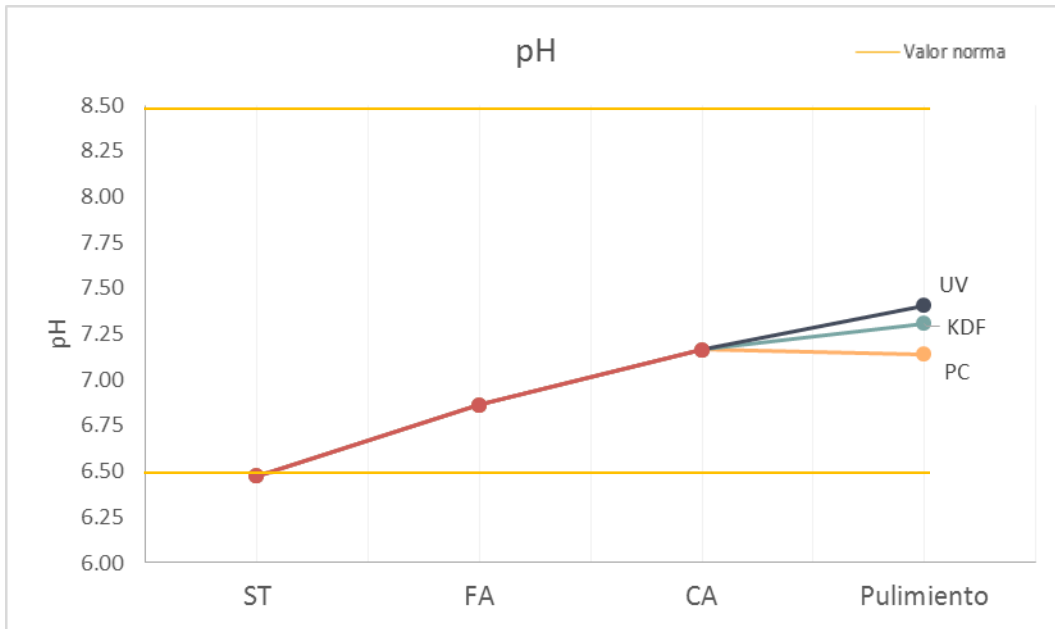
GRÁFICA 9 RESULTADOS DE pH EN LA PLANTA PILOTO
