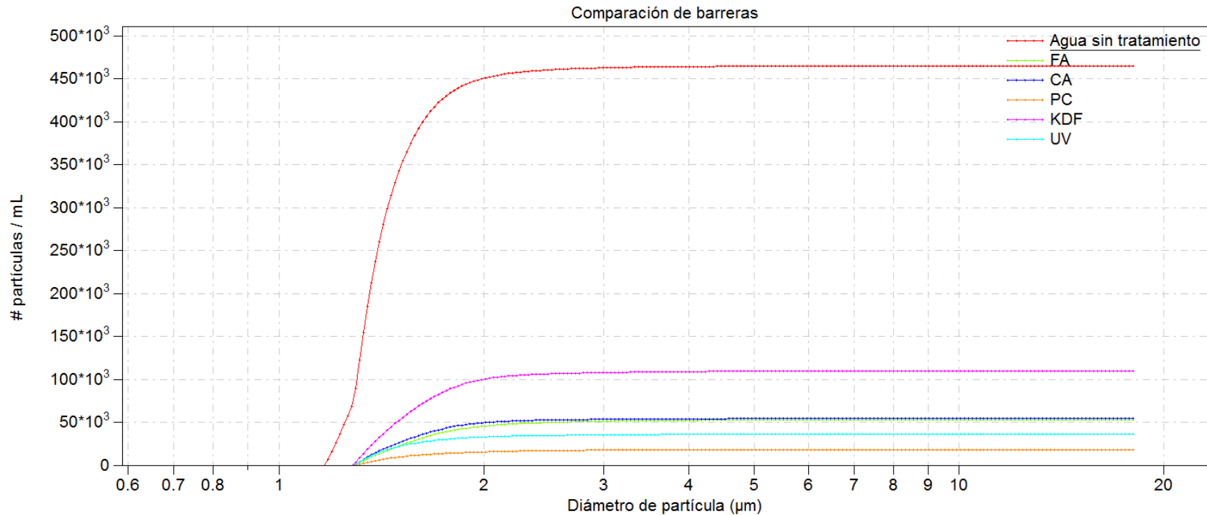
GRÁFICA 13 COMPARACIÓN DE LAS BARRERAS DE ACUERDO A SU DISTRIBUCIÓN DE PARTÍCULA
