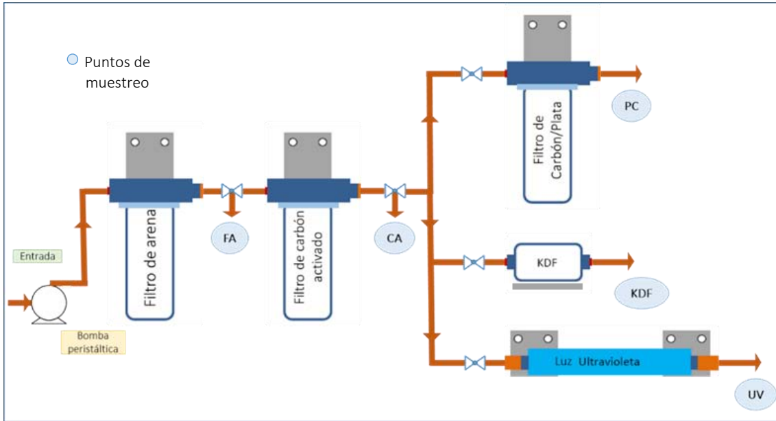
FIGURA 12 DIAGRAMA GENERAL DE LA PLANTA POTABILIZADORA PILOTO. FUENTE: ELABORACIÓN PROPIA.
