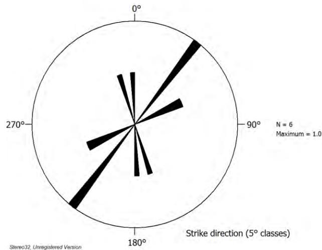
Figura 33. Familia de fracturas Museo de Arte Moderno y Altar a la Patria, Primera Sección del Bosque de Chapultepec.
