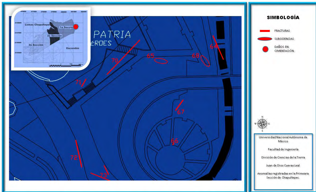
Figura 32. Fracturas lado sureste del Altar a la Patria, Primera Sección del Bosque de Chapultepec.
