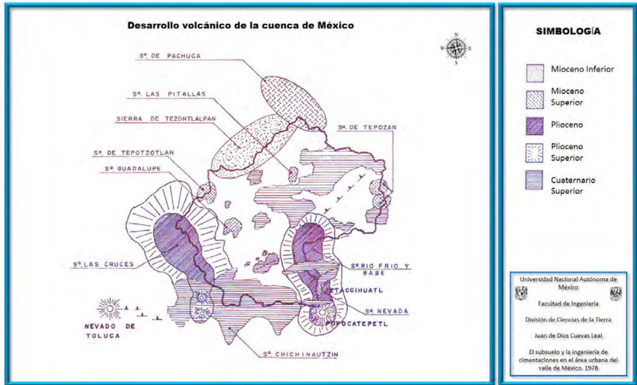
Figura 8. Desarrollo volcánico de la Cuenca del Valle de México. (tomada de: Sociedad Mexicana de Mecánica de Suelos, A. C., 1978).
