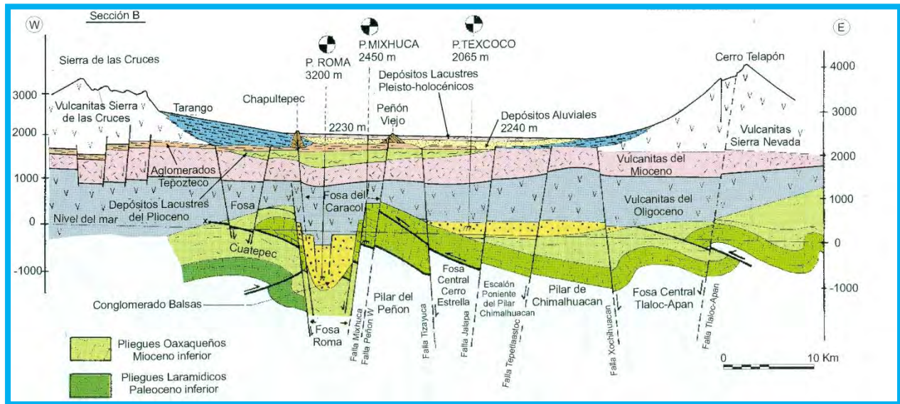
Figura 13. Sección geológica B de la Cuenca. (tomado de Mooser, 2005).
