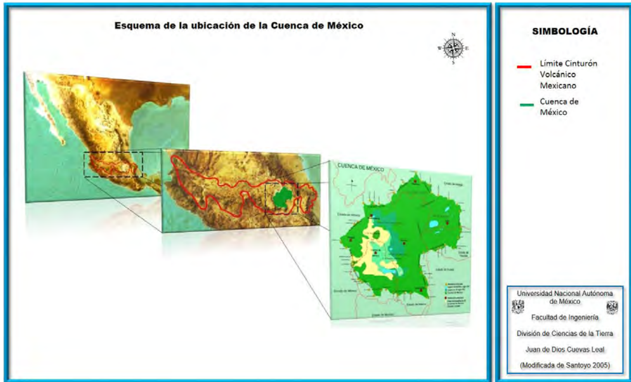
Figura 1. Ubicación de la Cuenca de México (modificada de Santoyo, 2005)
