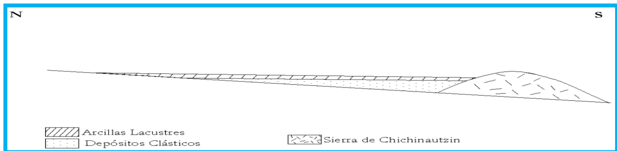
Figura 11. Sección geológica A de la Cuenca. (tomado de Mooser, 1986).
