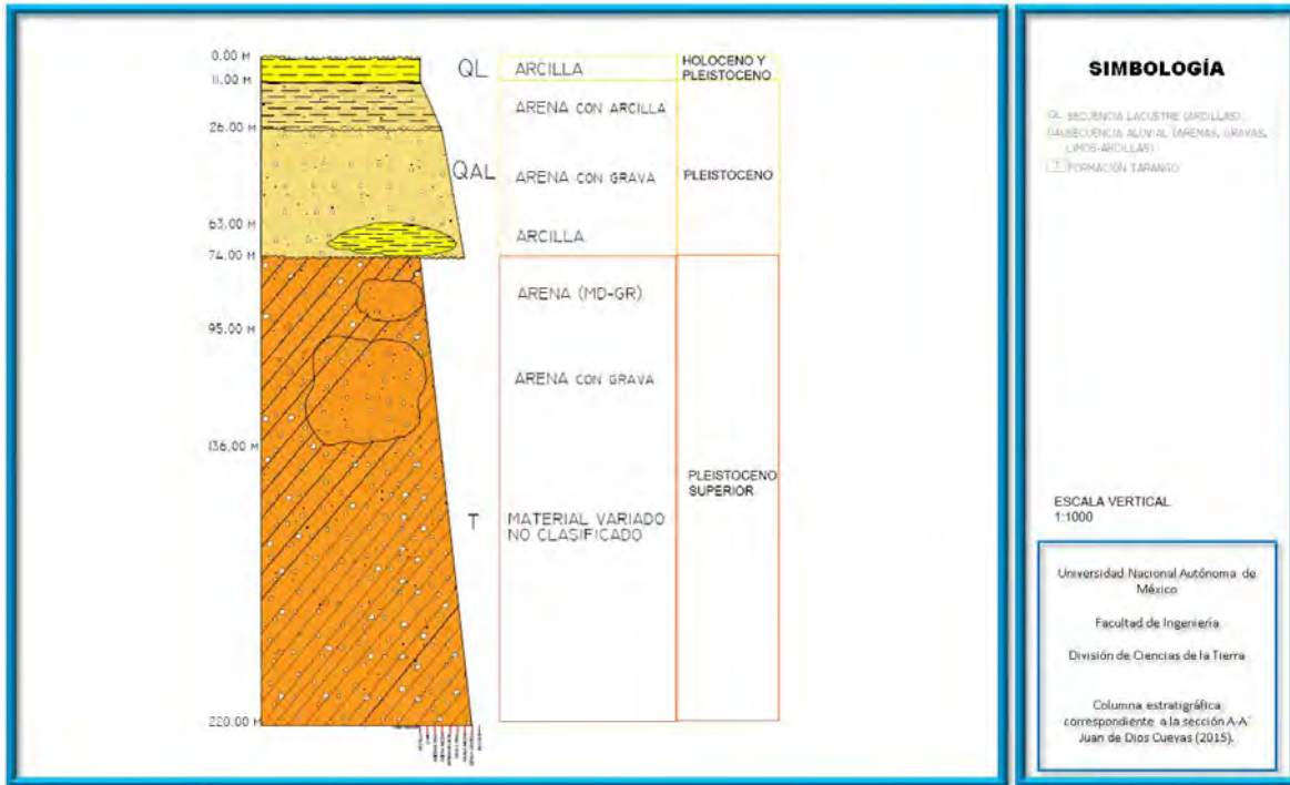
Figura 22. Columna estratigráfica correspondiente a la sección A-A'.
