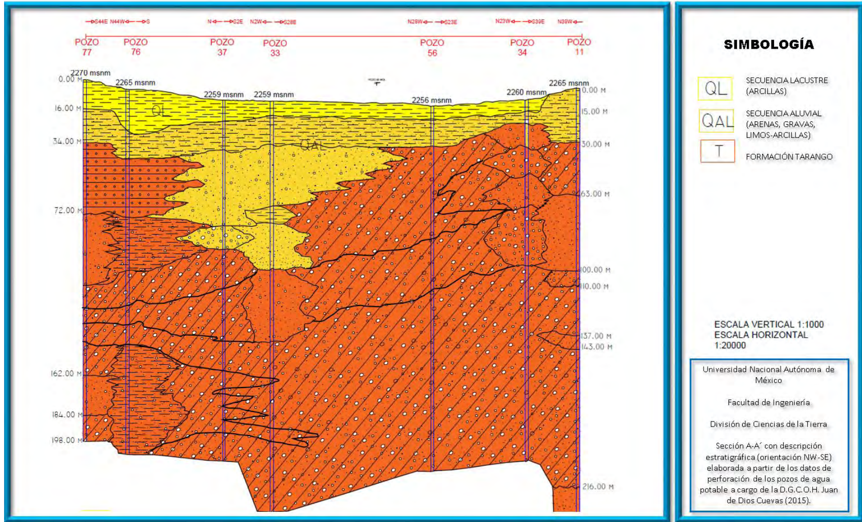
Figura 19. Sección A-A' con descripción de formaciones estratigráficas (orientación NW-SE) elaborada a partir de los datos de perforación de los pozos de agua potable a cargo de la D.G.C.O.H., 2015.
