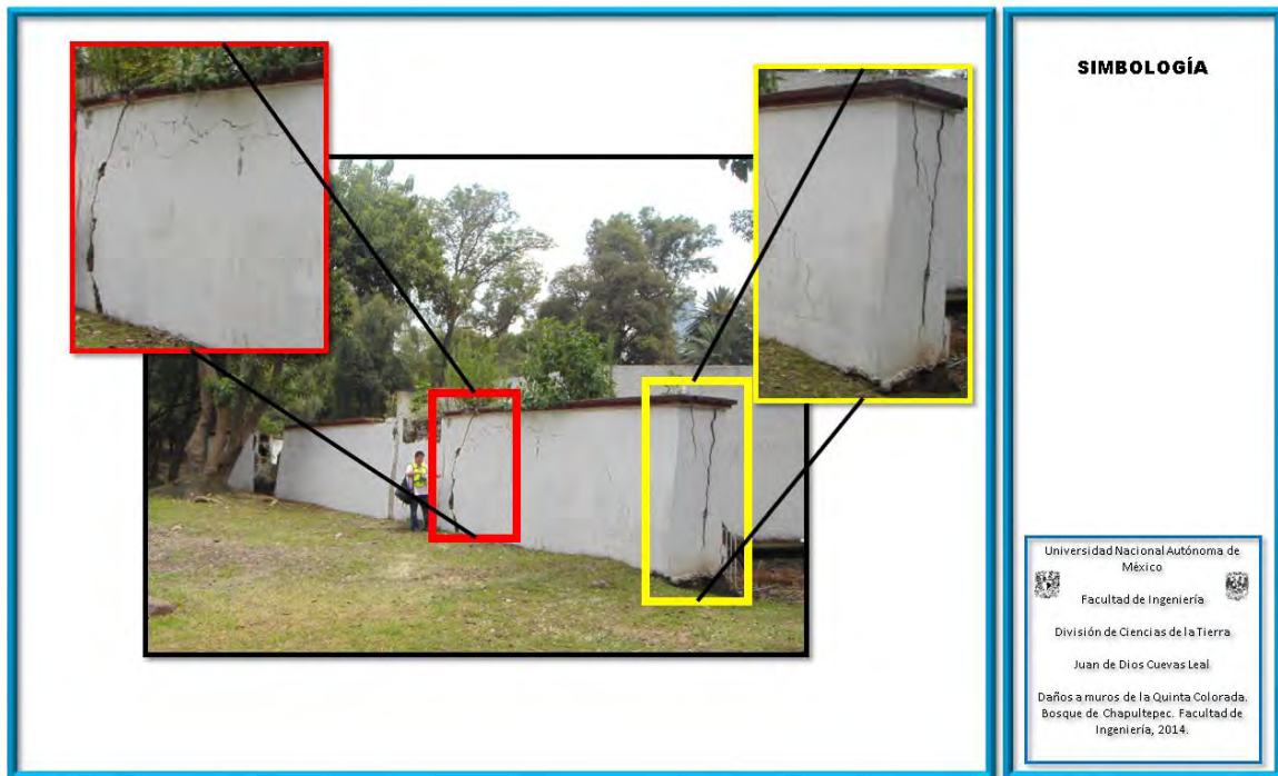
Fotografía 3. Daños a muros de la Quinta Colorada, Primera Sección del Bosque de Chapultepec. (Facultad de Ingeniería UNAM, 2014).
