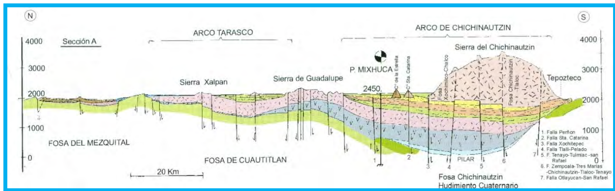
Figura 11. Sección geológica A de la Cuenca. (tomado de Mooser, 1986).
