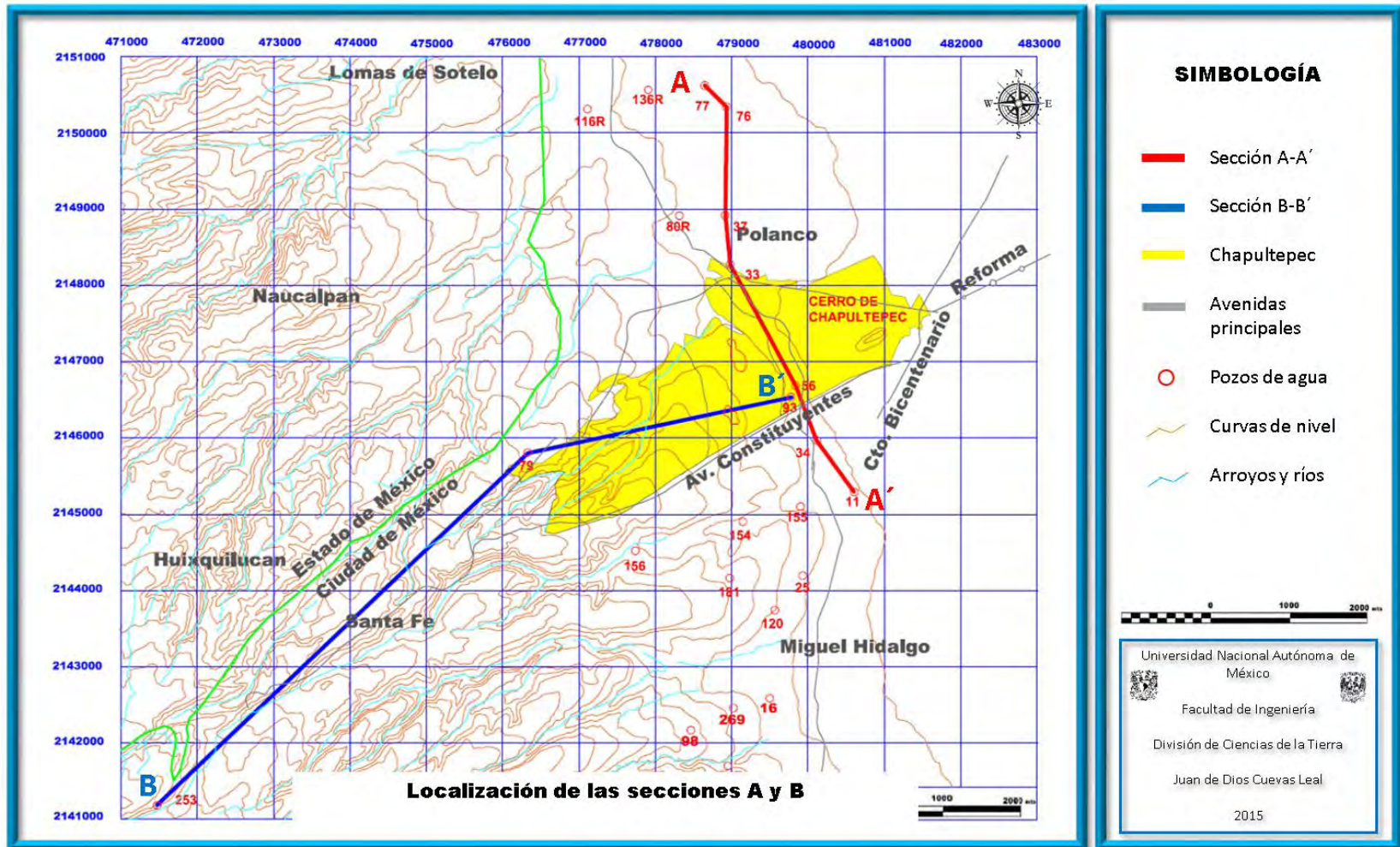
Figura 17. Ubicación de la Sección A (en color rojo) y la Sección B-B' (en color azul) en mapa con topografía.
