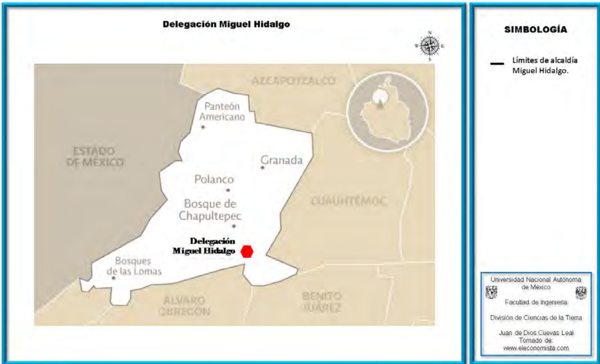
Figura 5. Límites de la delegación Miguel Hidalgo (tomada de www.eleconomista.com . Adaptada por Cuevas, 2016.)
