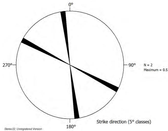
Figura 36. Familias de fracturas del lago de Chapultepec, Primera Sección del Bosque de Chapultepec.
