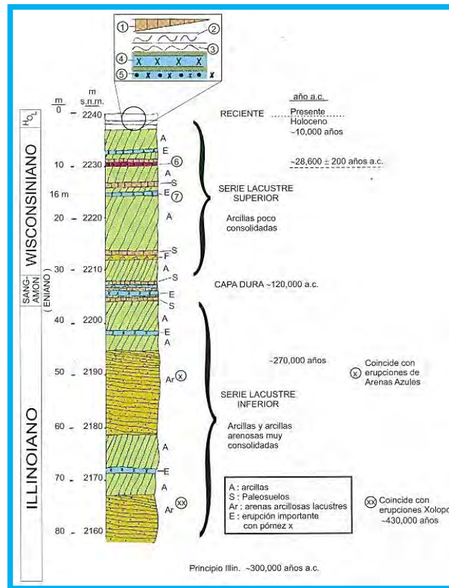
Figura 9. Erupciones volcánicas en los depósitos lacustres (tomado de Santoyo et al., 2005).
