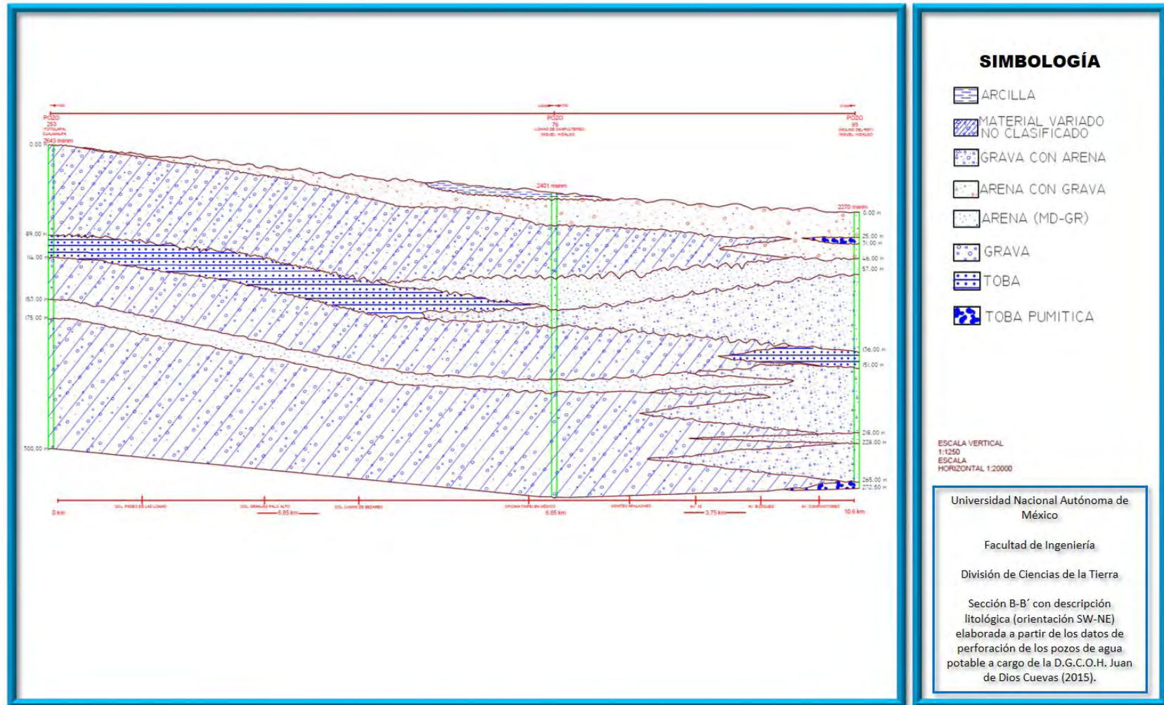
Figura 20. Sección B-B' con descripción estratigráfica (orientación SW-NE) elaborada a partir de los datos de perforación de los pozos de agua potable a cargo de la D.G.C.O.H.. 2015.
