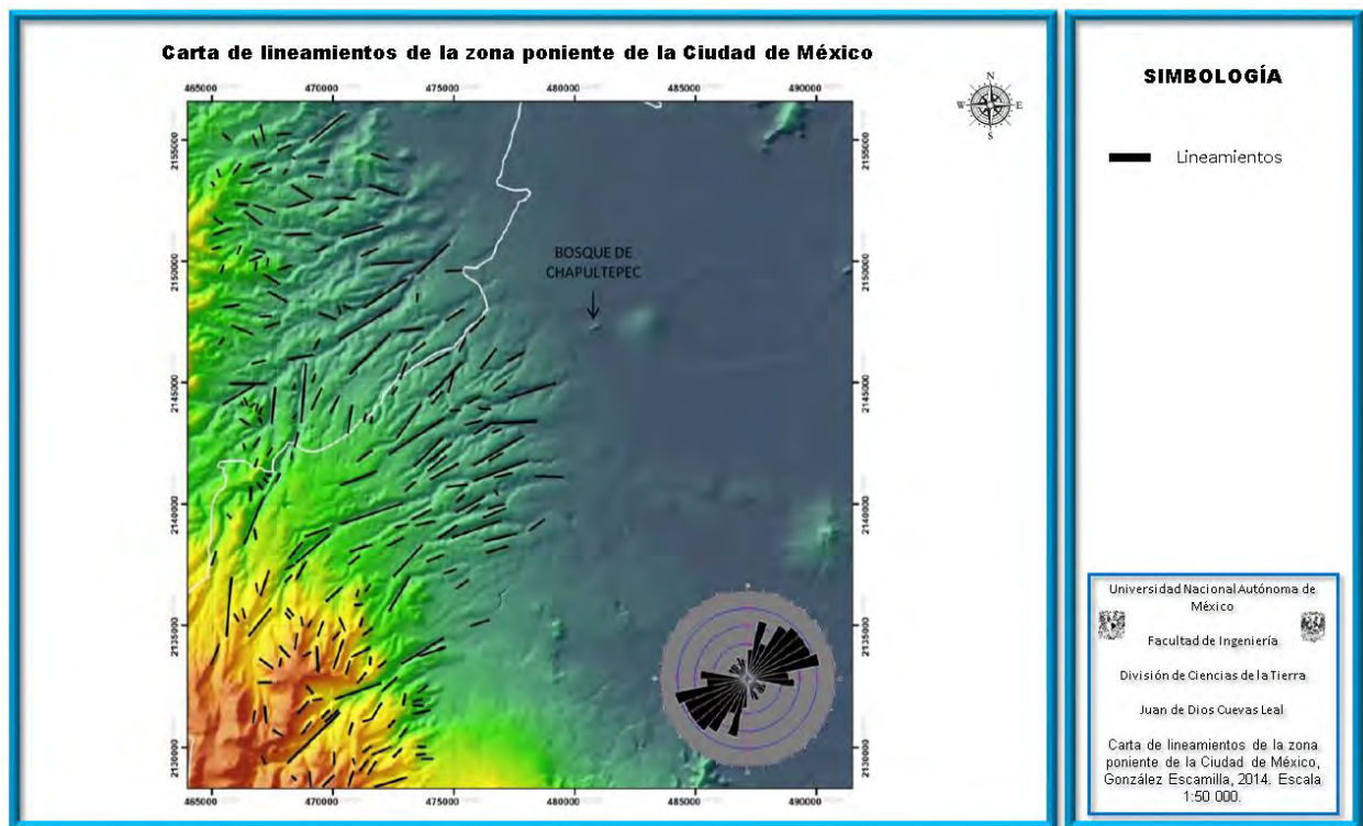
Figura 24. Carta de lineamientos de la zona poniente de la Ciudad de México. Escala 1:50 000 (González, 2014).
