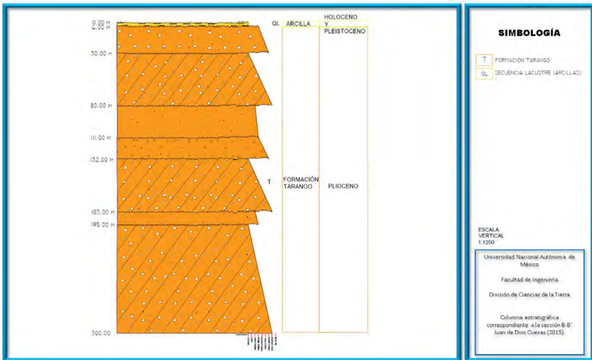
Figura 23. Columna estratigráfica correspondiente a la sección B-B'.
