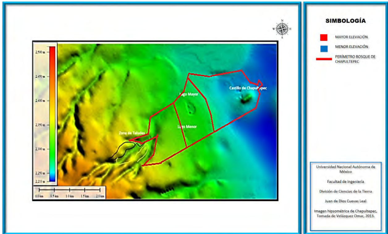
Figura 25. Imagen hipsométrica de Chapultepec (tomado de Velázquez, 2013).
