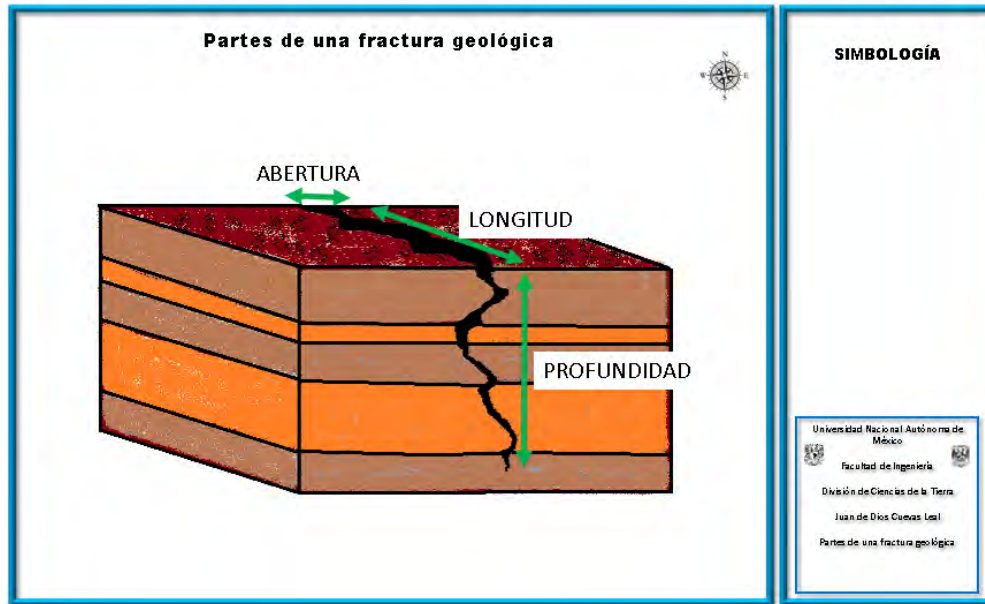
Figura 37. Componentes de una fractura geológica.
