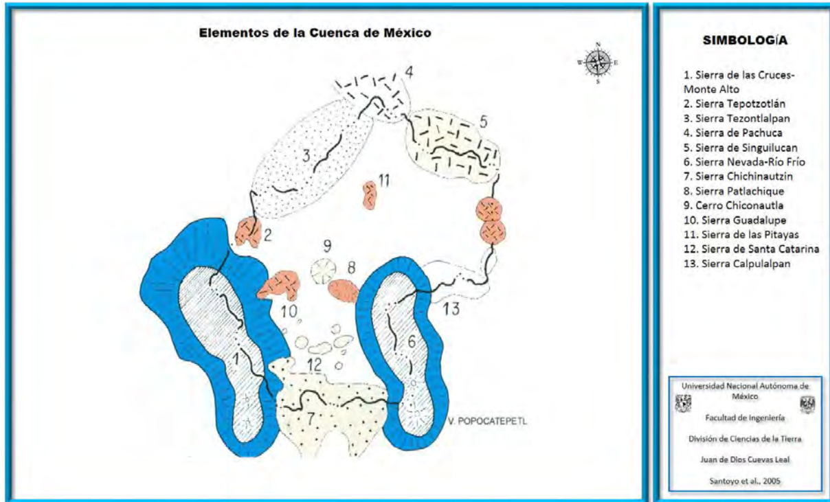
Figura 7. Elementos de la Cuenca de México (modificado de Santoyo et al., 2005).
