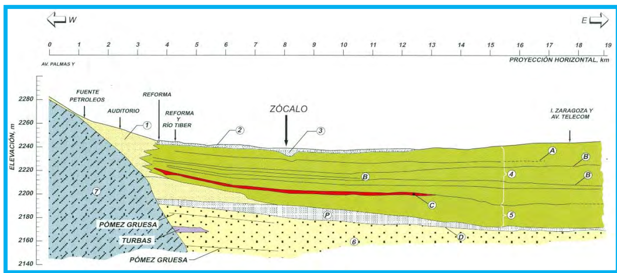
Figura 15. Sección geológica de la Cuenca dirección W-E. Secuencia pleistocénica de la Ciudad (tomado de Santoyo et al., 2005).
