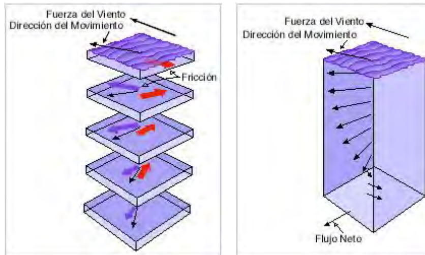
Figura 3: Efecto Coriolis
