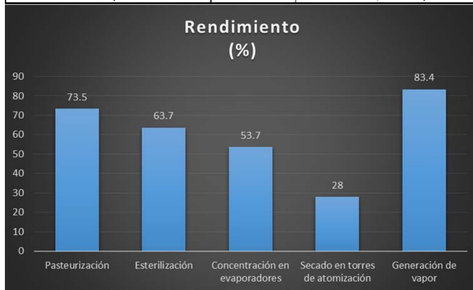
Imagen 18. Rendimiento energético por proceso térmico en una industria láctea.
