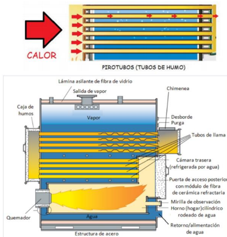
Imagen 6. Caldera Pirotubular de gas. Fuente: (Coakley, y otros, 2010), (Godos Fonseca, 2011)
