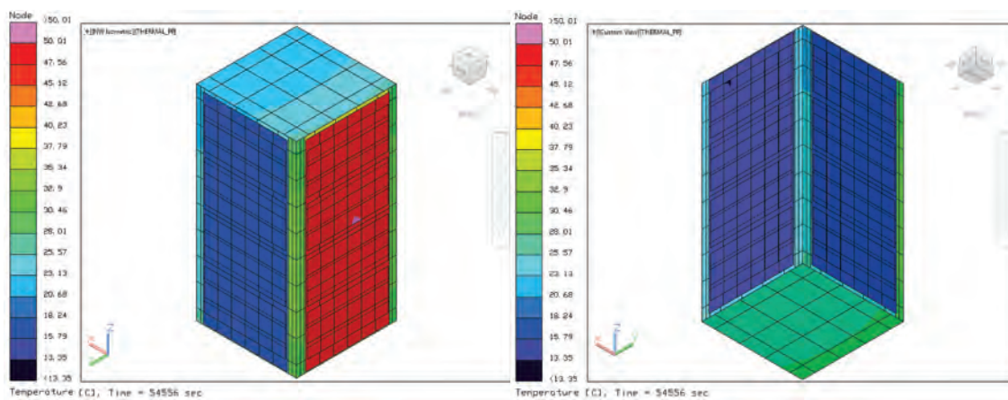
Figura 5.60: Temperaturas estructura y celdas CubeSat 2U caso caliente modificando posición
