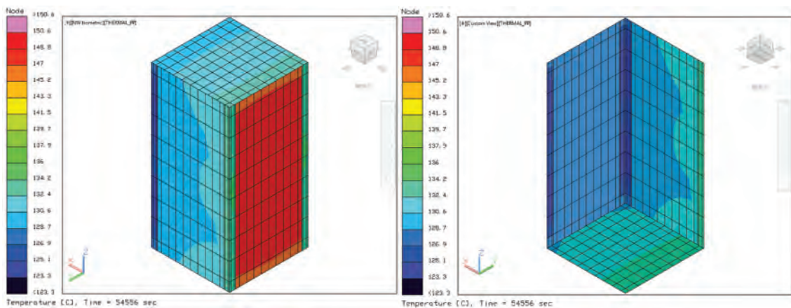
Figura 5.20: Temperaturas estructura CubeSat 2U considerando factor densidad 1.
