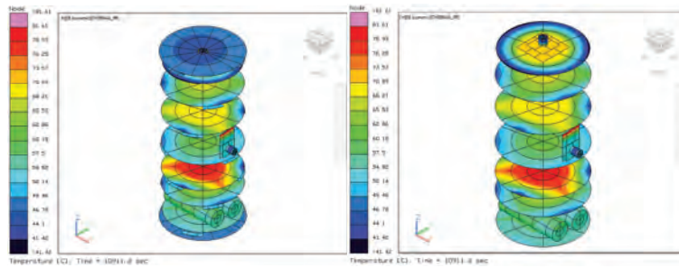
Figura 5.82: Temperatura componentes TubeSat 2U con pinturas caso caliente.
