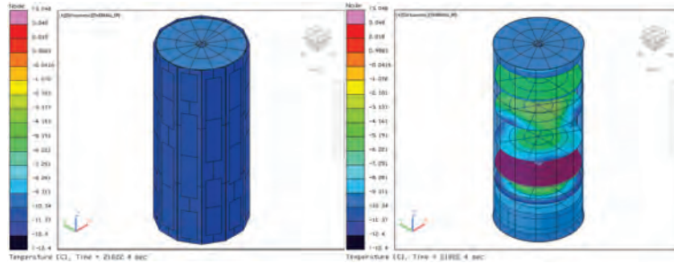
Figura 5.90: Temperatura TubeSat 2U con cajas caso frío.
