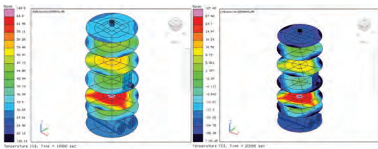
Figura 5.86: Temperatura componentes TubeSat 2U con pinturas caso frío.
