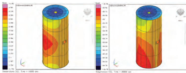
Figura 5.91: Temperatura estructura TubeSat 2U con cajas caso frío.
