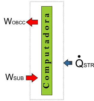
Figura 5.6: Diagrama de balance de energía del subsistema de computadora de abordó CubeSat.
