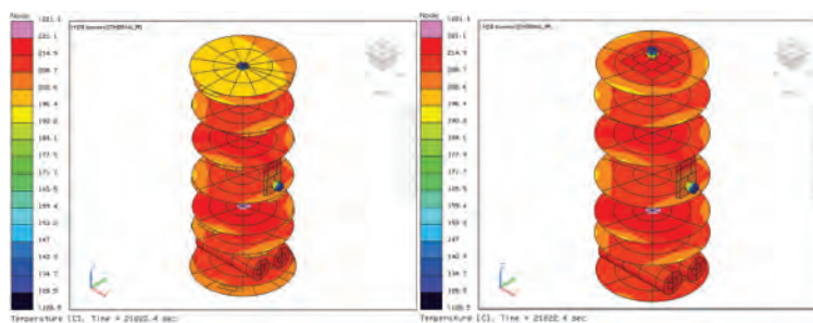
Figura 5.78: Temperatura componentes TubeSat 2U con separadores caso caliente.
