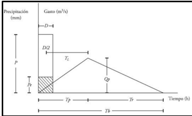
Ilustración 13 Ejemplo del Hidrograma Unitario Triangular, Domínguez 2015.
