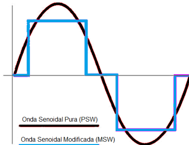
Imagen II.6: Señal de salida de los inversores Fuente: Energía Solar Fotovoltaica: Cálculo de una instalación aislada
