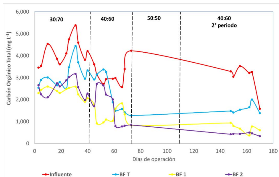
Figura 5.21. Comportamiento del carbón orgánico total (etapas I-IV)
