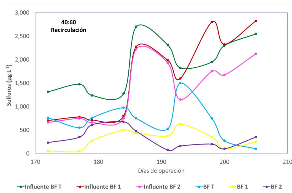
Figura 5.51. Comportamiento de los sulfuros (etapa V)
