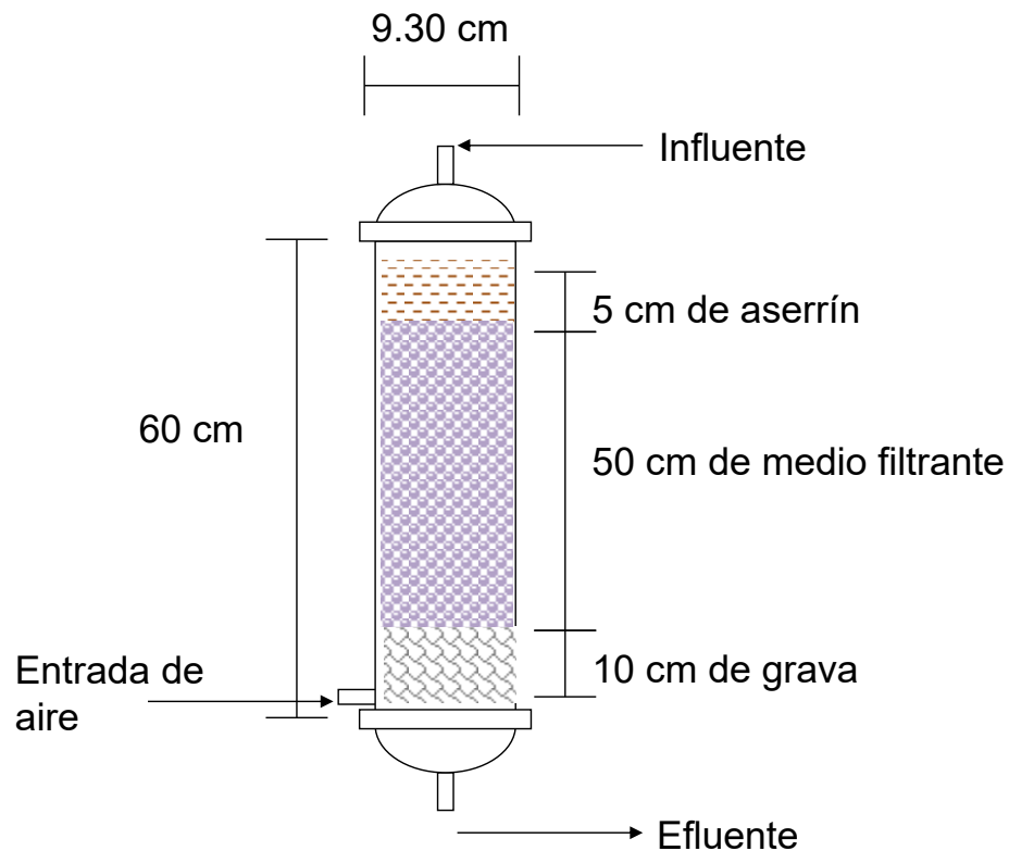
Figura 4.4 Configuración de los reactores
