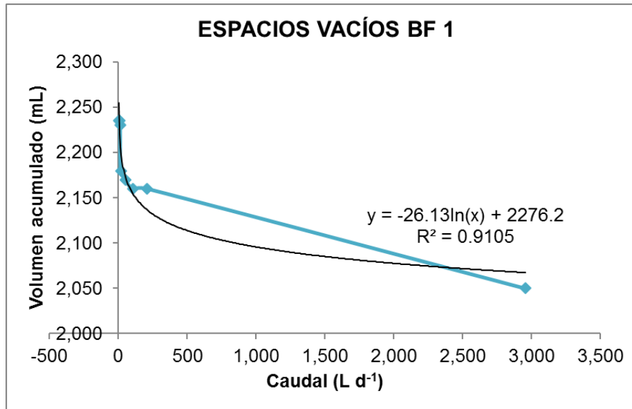
Figura 10.3. Curva de espacios vacíos contra caudal en el BF 1
