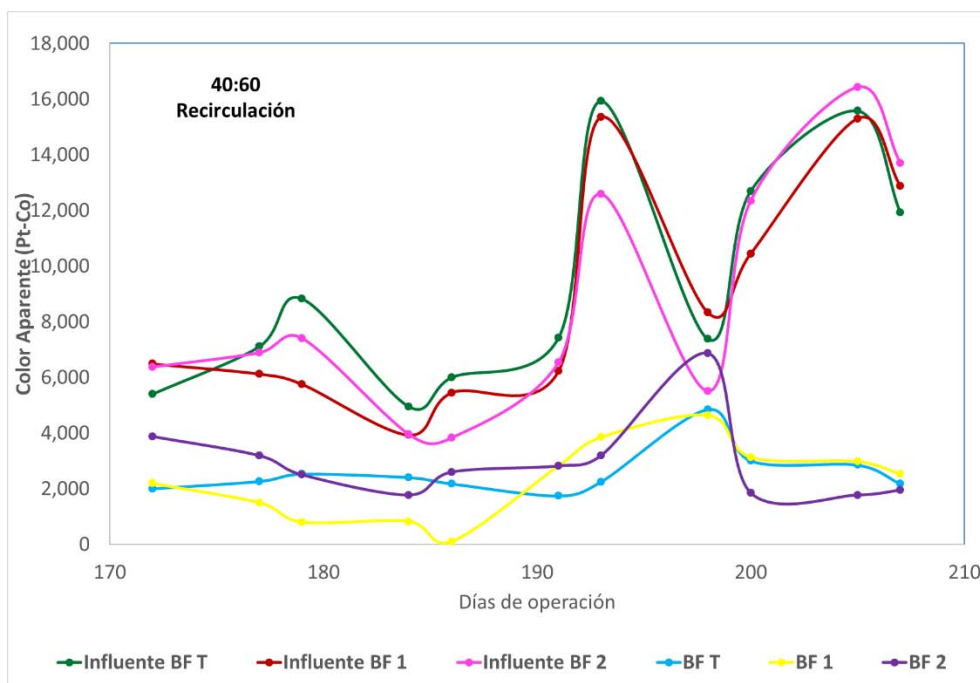
Figura 5.48. Comportamiento del color aparente (etapa V)
