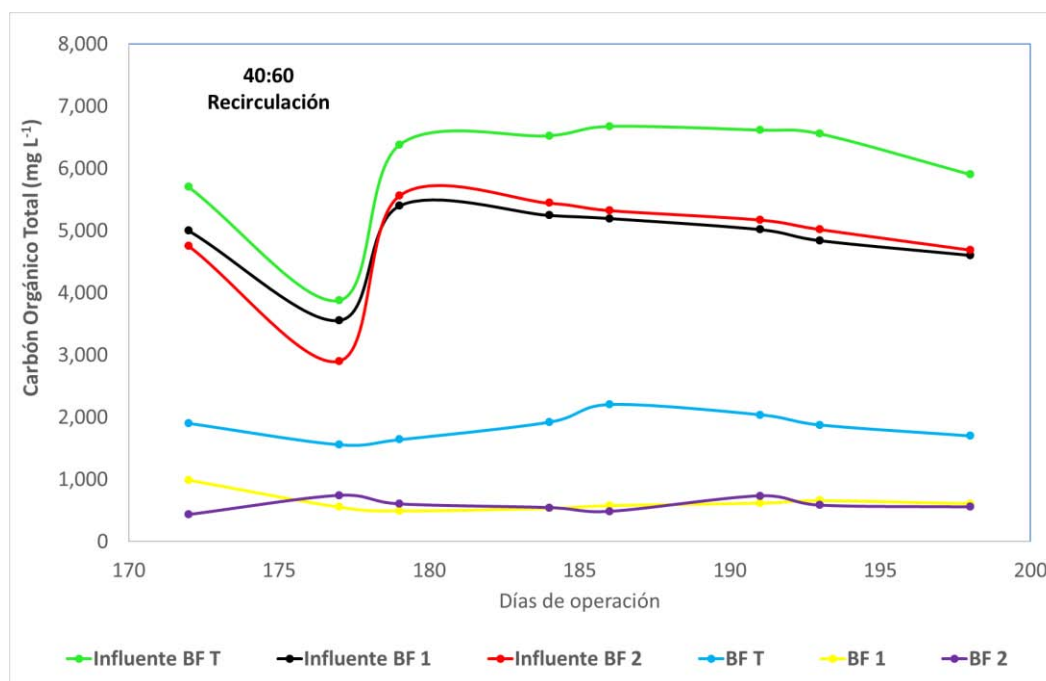
Figura 5.22. Comportamiento del carbón orgánico total (etapa V)
