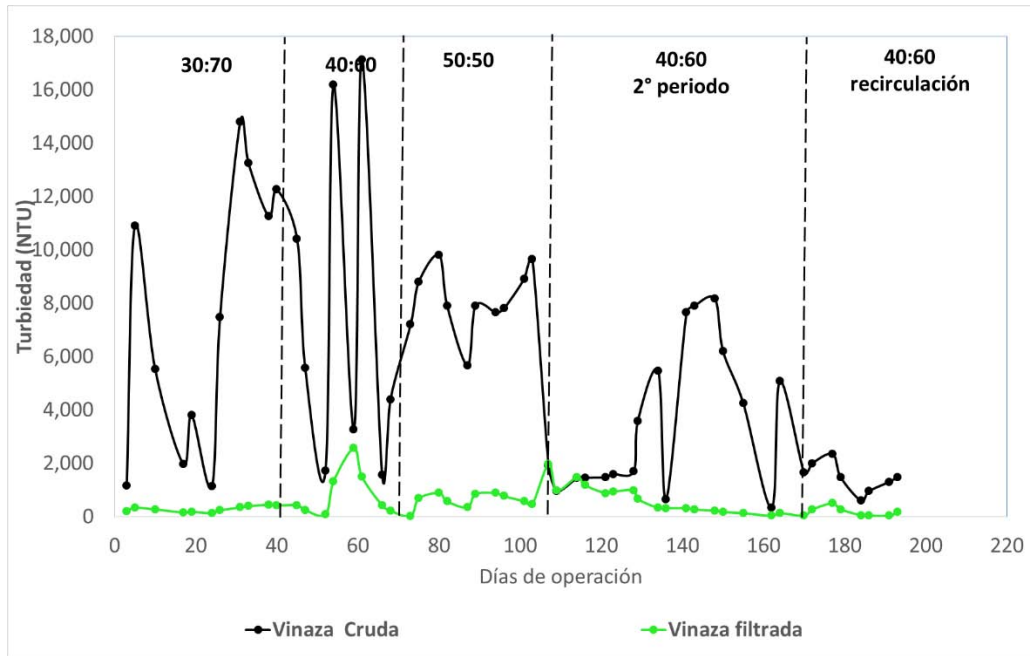
Figura 5.43. Comportamiento de la turbiedad (pretratamiento)
