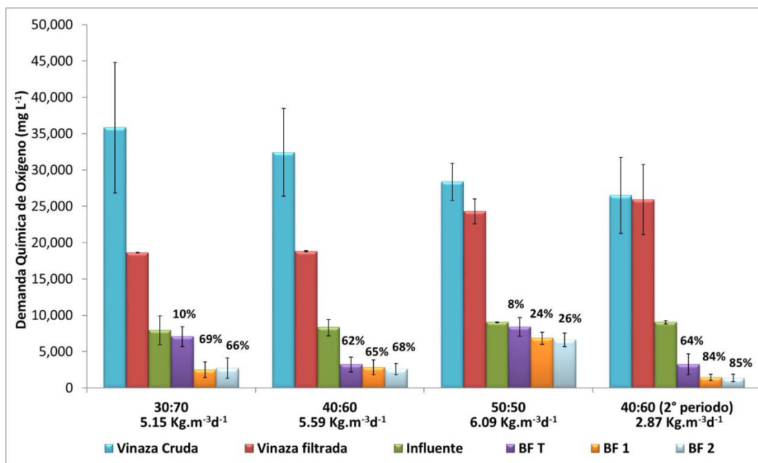
Figura 5.17. Comportamiento de la demanda química de oxígeno (promedio etapas I-IV)
