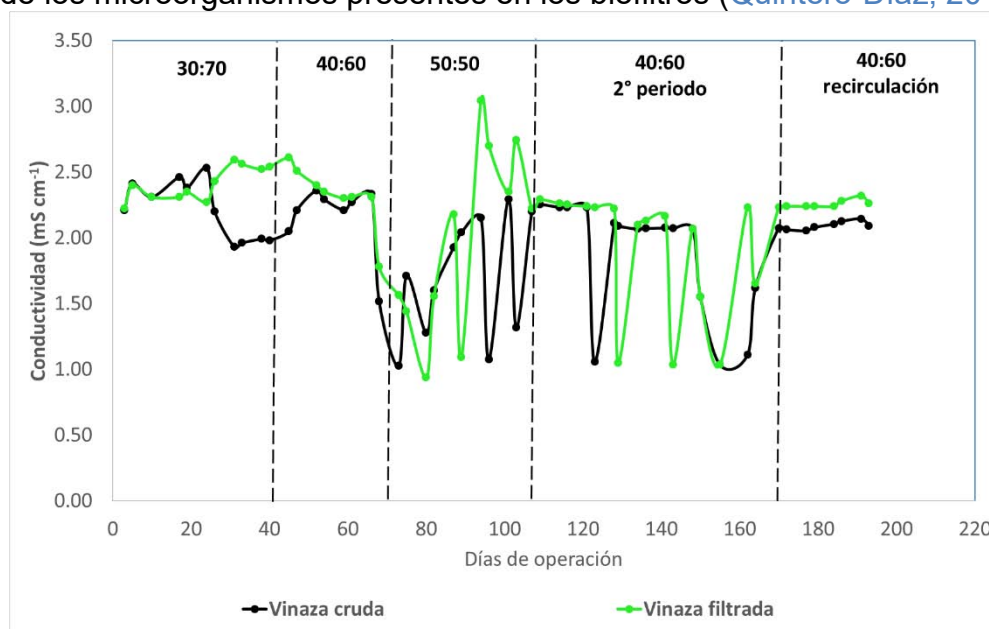
Figura 5.37. Comportamiento de la conductividad (pretratamiento)
