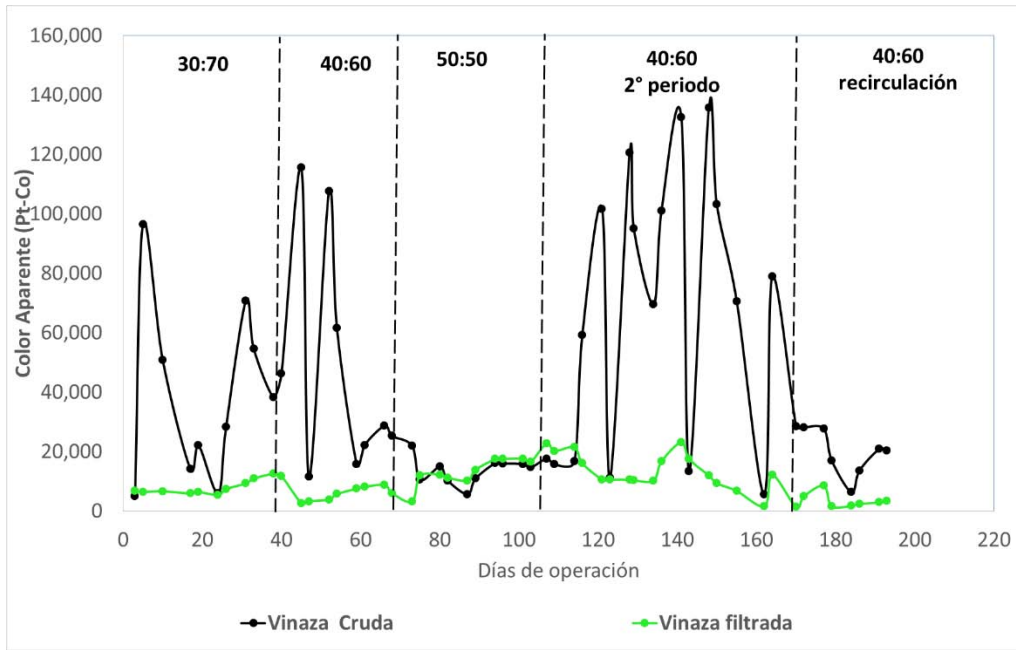
Figura 5.46. Comportamiento del color aparente (pretratamiento)
