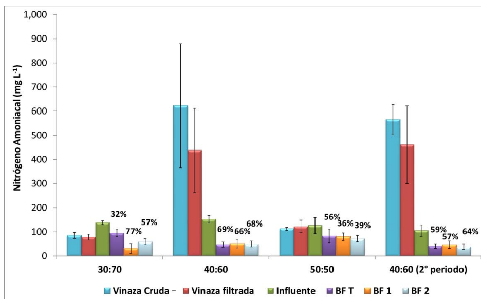
Figura 5.32. Comportamiento del nitrógeno amoniacal (promedio etapas I-IV)
