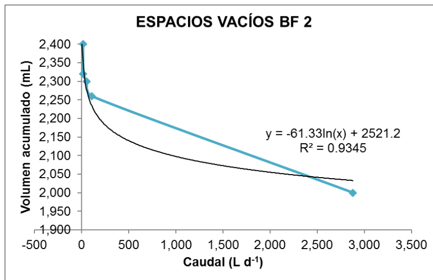
Figura 10.4. Curva de espacios vacíos contra caudal en el BF 2
