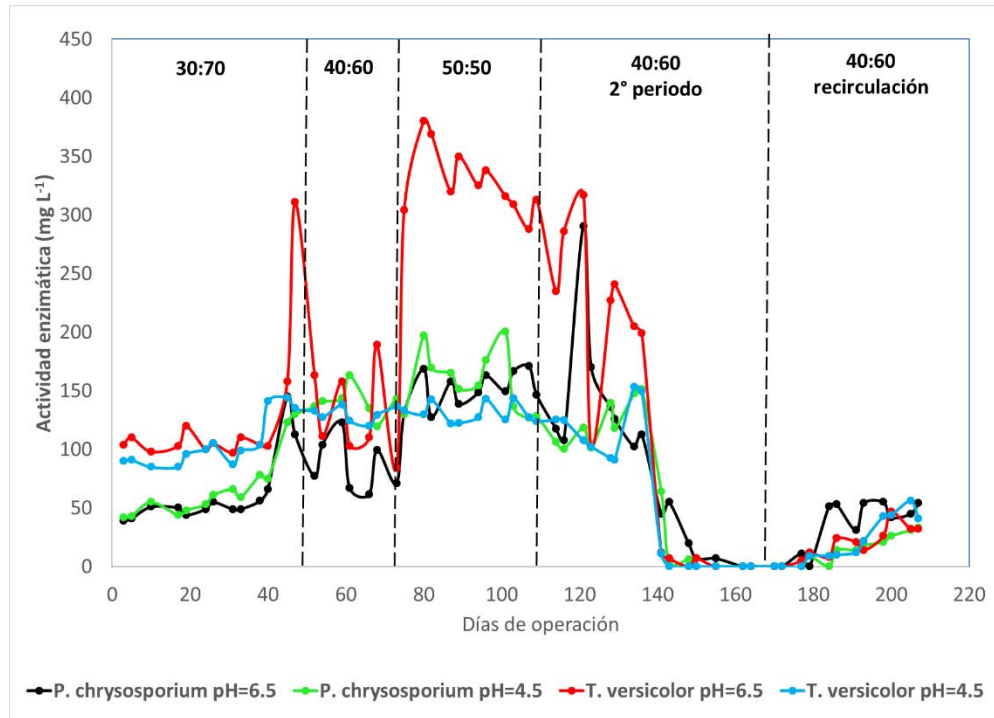
Figura 5.52. Comportamiento de las lacasas
