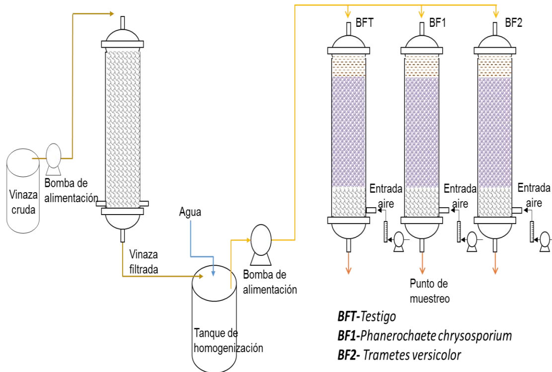
Figura 4.9 Tren de tratamiento de vinazas de tequila
