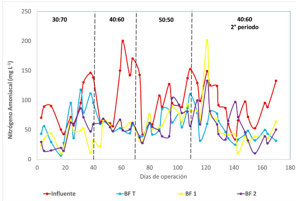
Figura 5.30. Comportamiento del nitrógeno amoniaco (etapas I-IV)
