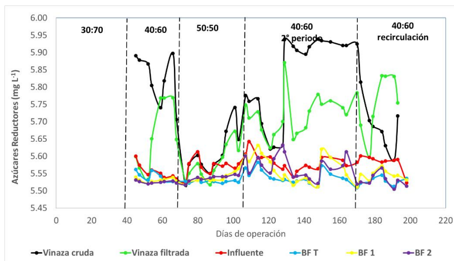
Figura 5.51. Comportamiento de los azúcares reductores (etapas I-V)
