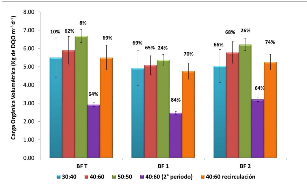
Figura 5.19. Cargas orgánicas volumétricas y porcentaje de remoción (etapas I-V)
