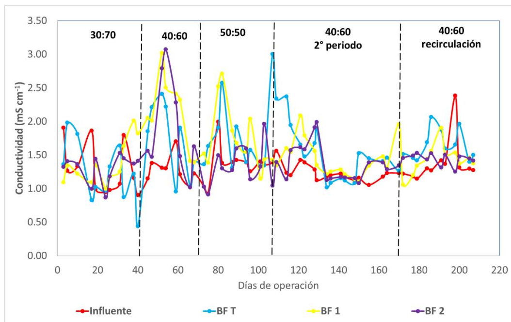
Figura 5.38. Comportamiento de la conductividad (etapas I-V)
