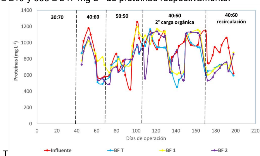
Figura 5.50. Comportamiento de las proteínas (etapas I-V)
