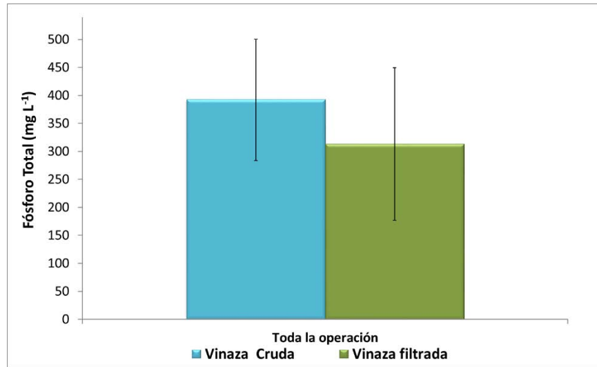
Figura 5.25. Comportamiento del fósforo total (pretratamiento)
