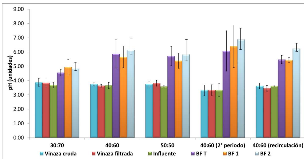
Figura 5.13. Comportamiento del pH (promedio de etapas I-V)
