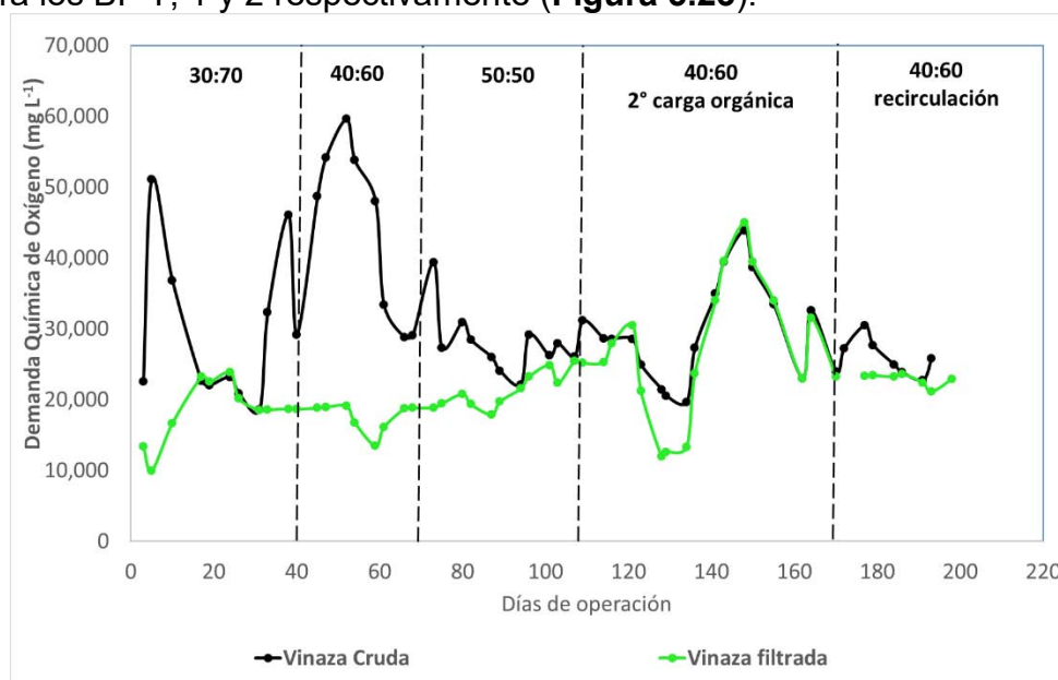
Figura 5.14. Comportamiento de la demanda química de oxígeno (pretratamiento)
