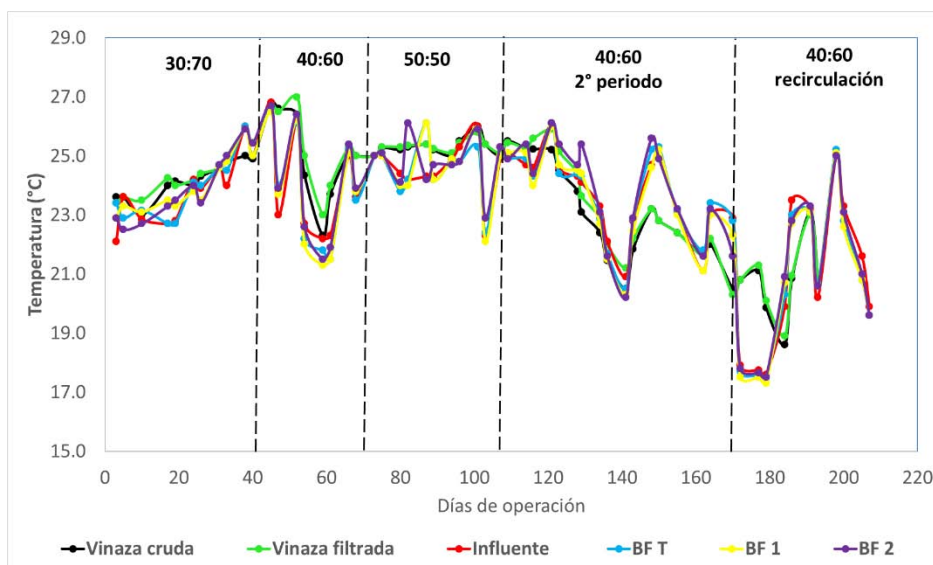
Figura 5.34. Comportamiento de la temperatura (etapas I-V)
