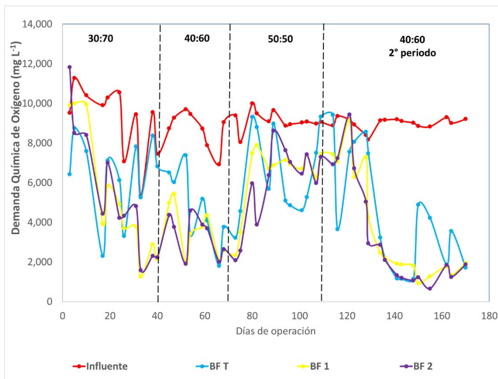
Figura 5.15. Comportamiento de la demanda química de oxígeno (etapas I-IV)
