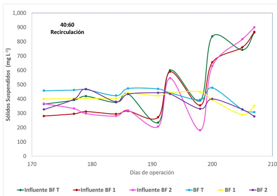
Figura 5.42. Comportamiento de los sólidos suspendidos (etapa V)
