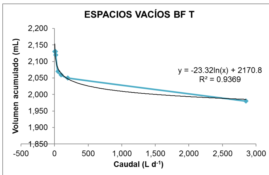
Figura 10.2. Curva de espacios vacíos contra caudal en el BF T
