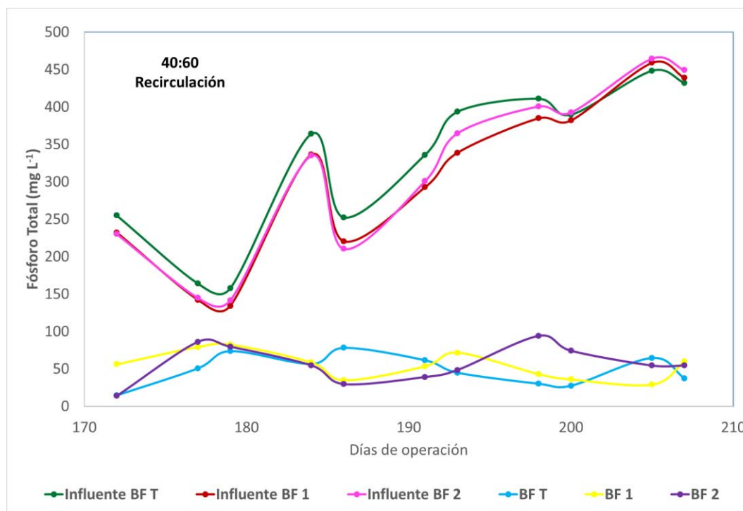
Figura 5.27. Comportamiento del fósforo total (etapa V)
