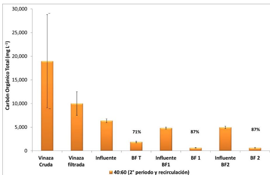
Figura 5.24 Comportamiento del carbón orgánico total (promedio etapa V)
