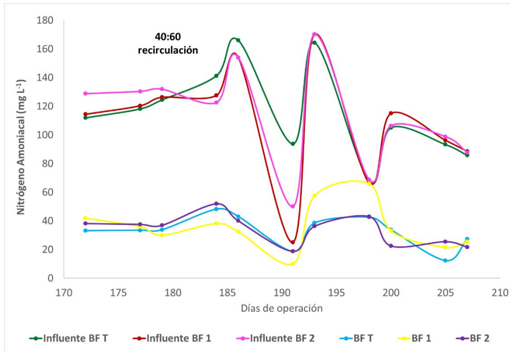
Figura 5.31. Comportamiento del nitrógeno amoniaco (etapa V)
