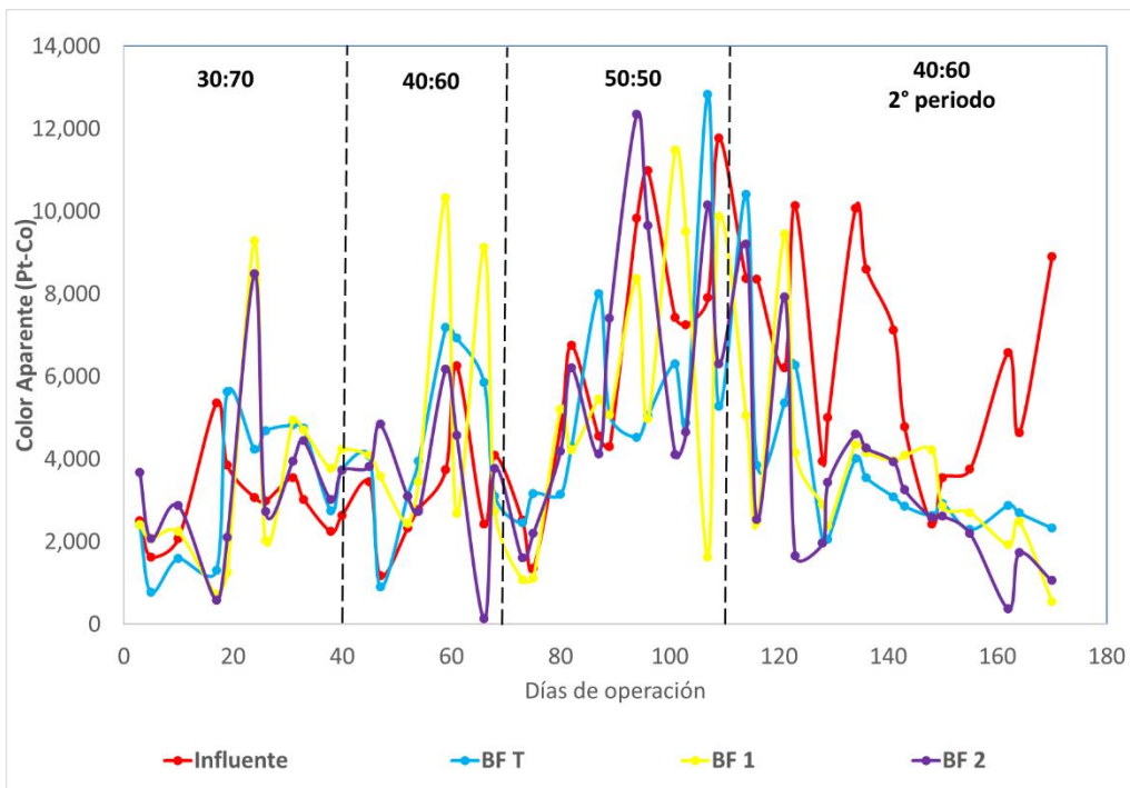
Figura 5.47. Comportamiento del color aparente (etapas I-IV)
