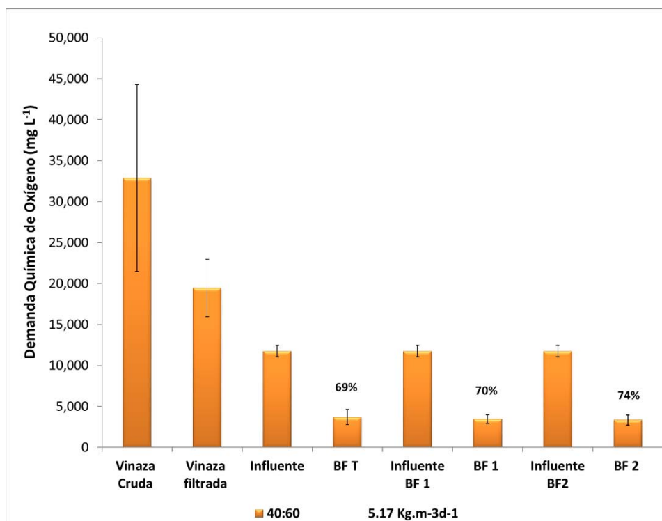
Figura 5.18. Comportamiento de la demanda química de oxígeno (promedio etapa V)
