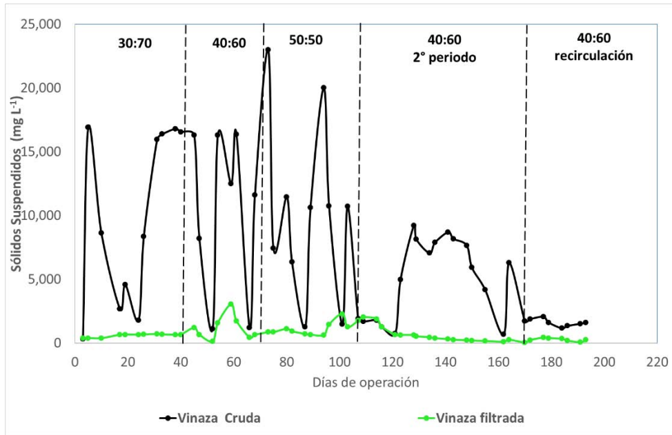
Figura 5.40. Comportamiento de los sólidos suspendidos (pretratamiento)
