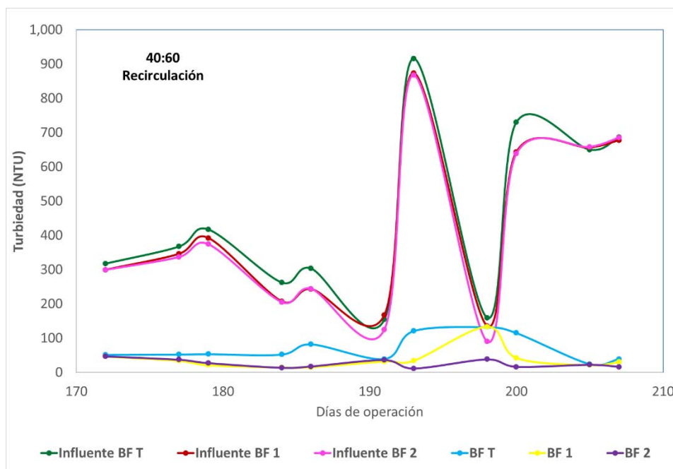
Figura 5.45. Comportamiento de la turbiedad (etapa V)
