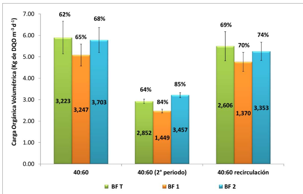
Figura 5.20. Cargas orgánicas volumétricas y porcentajes de remoción (etapas II, IV y V)
