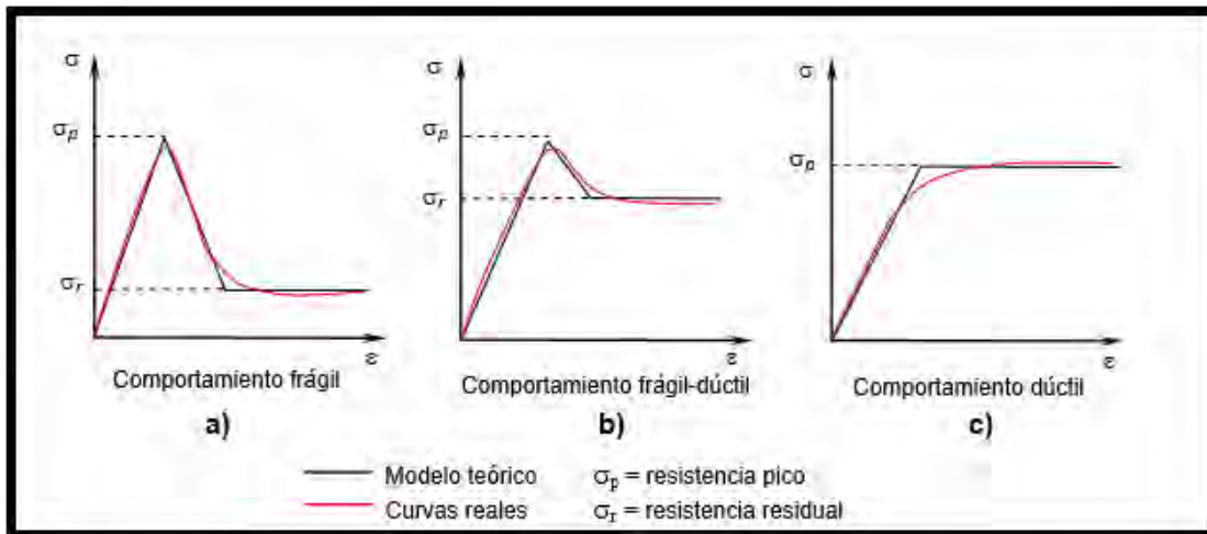
Figura 51. Comportamiento de las rocas según el tipo de esfuerzo-deformación. (Tomada de González de Vallejo, 2002)
