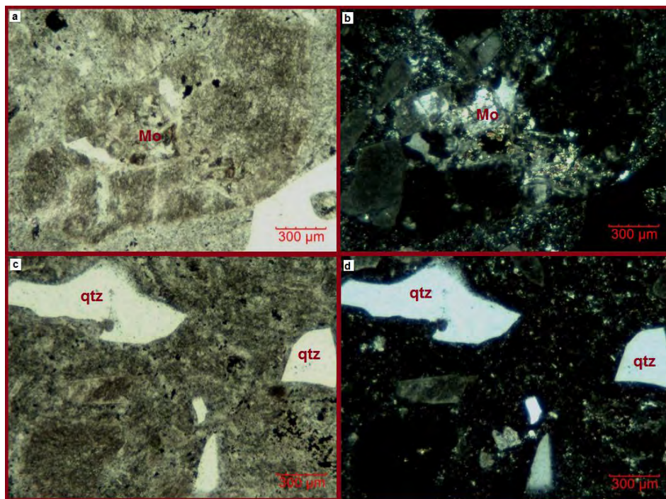
Figura 25. Vista al microscopio de la muestra SPA-5. a) Detalle de un cristal de muscovita de alto relieve, b) con colores de interferencia azulados propios de una alta birrefringencia en nícoles cruzados. c) Cristales subhedrales de cuarzo, d) con nícoles cruzados.
