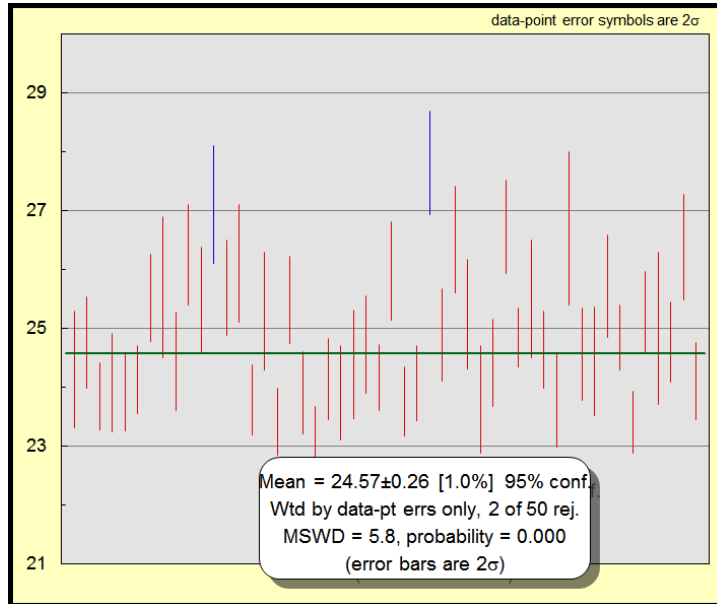
Figura 18. Gráfico TuffZirc con resultados para la muestra SPA-33A con un intervalo de edades de entre 23 y 29 Ma.
