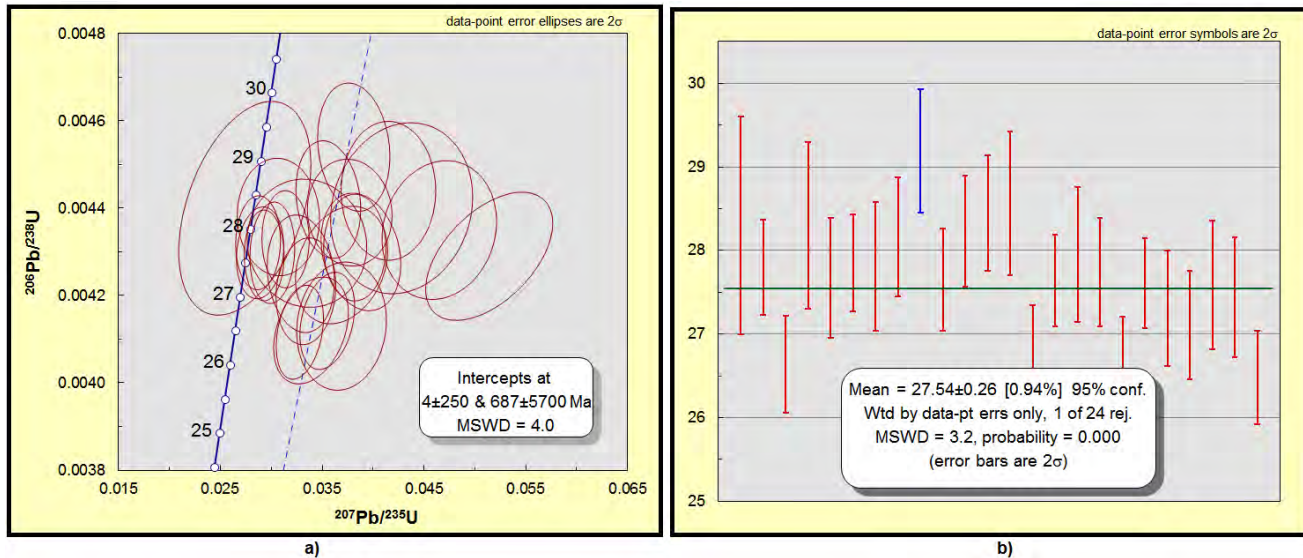
Figura 17. a) Gráfico de Wetherill con resultados discordantes para la muestra SPA-5. b) Gráfico TuffZirc de la misma muestra que configura una edad media ponderada de 27.54 \pm 0.26 Ma.
