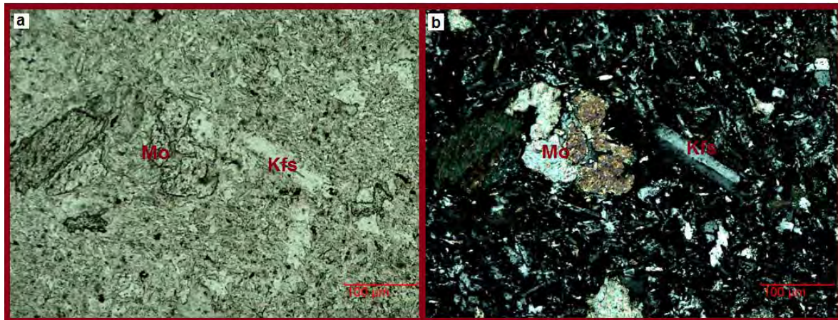
Figura 26. Muestra al microscopio de SPA-5. a) Imagen con nícoles alineados de un cristal de muscovita de alto relieve y uno de feldespato. b) Misma vista pero con nícoles cruzados donde se aprecia el maclado de Carlsbad del feldespato y los altos colores de interferencia de la muscovita
