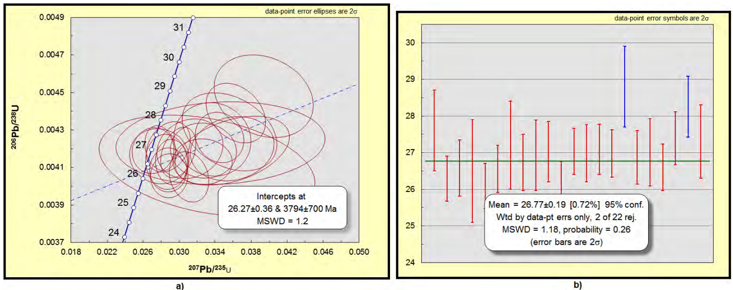
Figura 13 . a) Gráfico de Wetherill con resultados para la muestra SPA-28. A pesar de no estar tan concentrados, los datos muestran una marcada tendencia a la intersección. b) Gráfico TuffZirc de la misma muestra que configura una edad media ponderada de 26.77 Ma.
