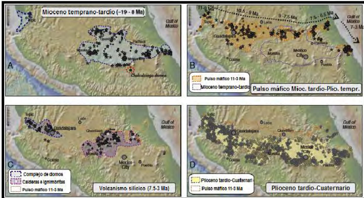
Figura 4. Secuencia de imágenes que representan la migración del arco magmático desde el Mioceno Temprano hasta su posición en el Cuaternario. Modificada de Ferrari et al, 2012
