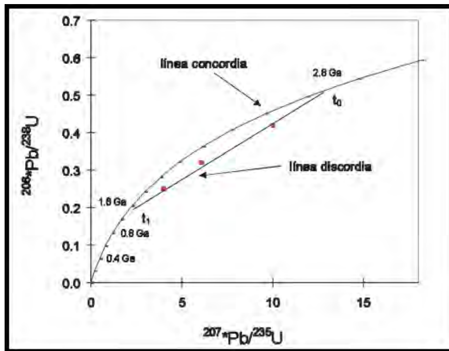
Figura 10. Ejemplo de un diagrama de concordia generada por los sistemas ^{238}\text{U} y ^{235}\text{U} . La línea de discordia interseca a la curva concordia en t_0 que representa la edad de cristalización de la roca, y en t_1 que indica la edad de algún evento de metamorfismo.
