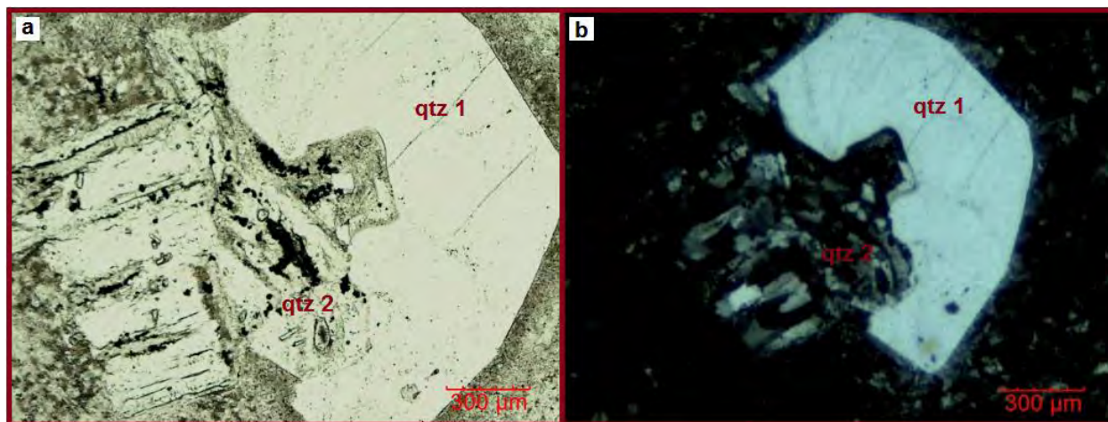
Figura 36. Cristales de cuarzo de la lámina SPA-28; qtz 1: cuarzo con extinción recta, qtz 2: cuarzo con extinción ondulante. a) Nicoles paralelos. b) Nicoles cruzados
