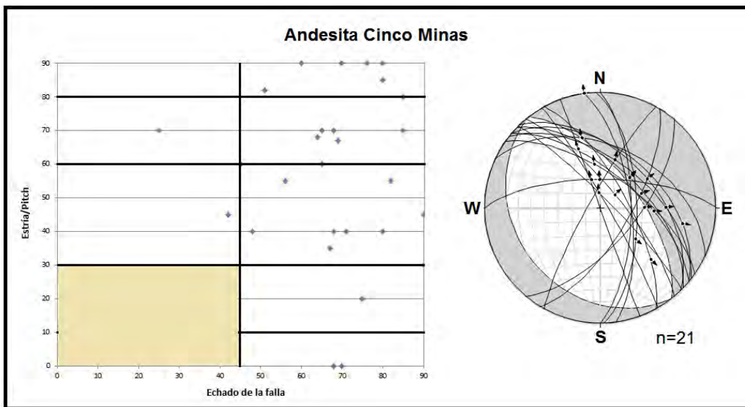
Figura 54. Gráfica dip vs pitch y diagrama de mecanismo focal de la Andesita Cinco Minas
