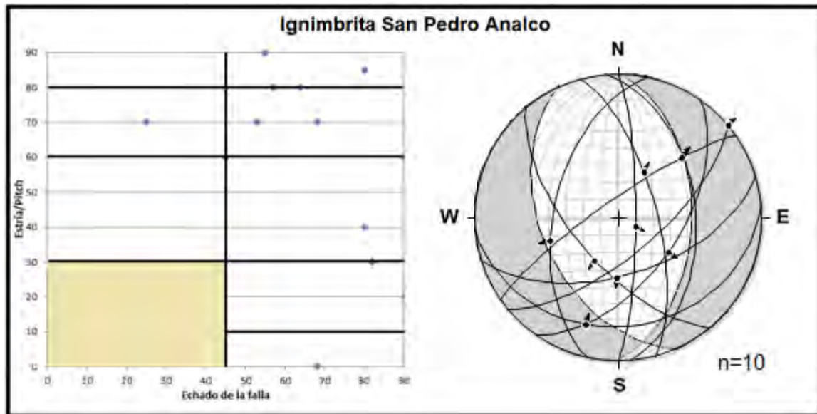
Figura 55. Gráfica dip vs pitch y diagrama de mecanismo focal de la Ignimbrita San Pedro Analco.
