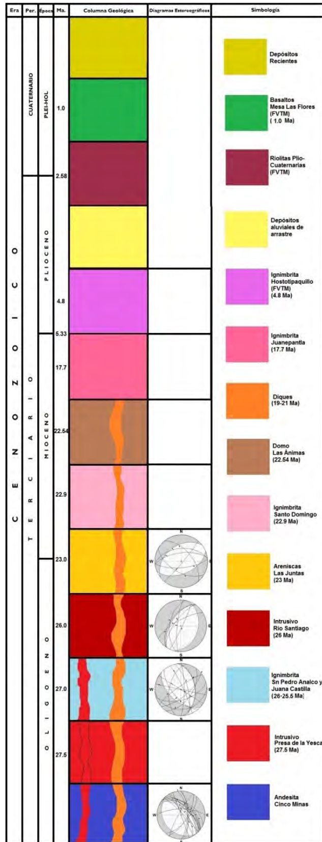
Figura 46. Columna Geológica elaborada de la región
