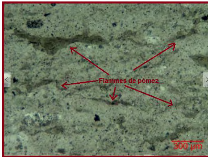
Figura 31. Detalle de las pómez aplastadas en forma de fiamme a nivel microscópico de la muestra SPA-7
