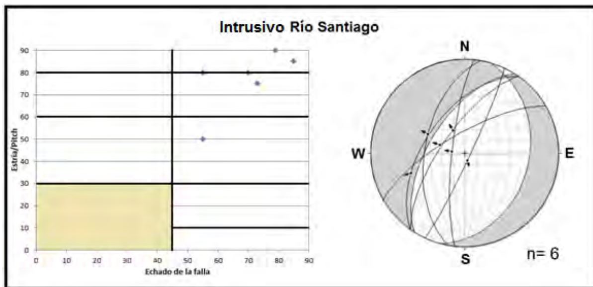
Figura 56. Gráfica dip vs pitch y diagrama de mecanismo focal del Intrusivo Río Santiago.
