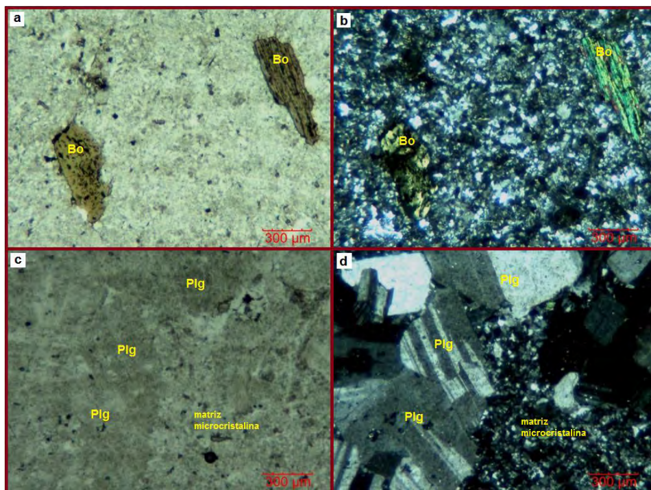
Figura 35. Lámina delgada de SPA-31. a) Se observan dos cristales de biotita de color pardo. b) Misma biotita con nicoles cruzados donde se aprecian colores de interferencia entre verdes y amarillos. c) Plagioclasas inmersas en una matriz microcristalina. d) Las mismas plagioclasas vistas con nicoles cruzados con maclado polisintético.
