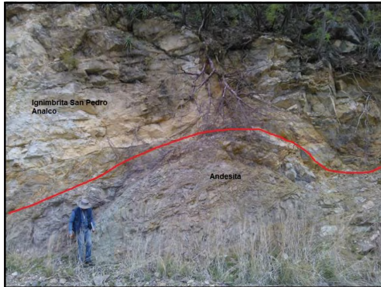
Figura 27. Afloramiento donde la ignimbrita San Pedro Analco cubre a la Andesita Cinco Minas.
