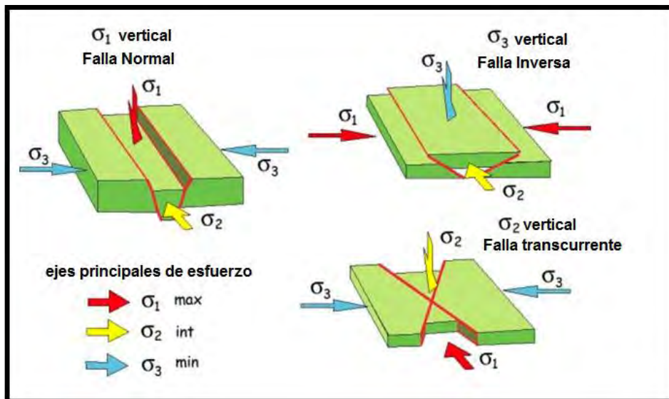
Figura 50. Tipos de fallas generadas según orientación de esfuerzos.
