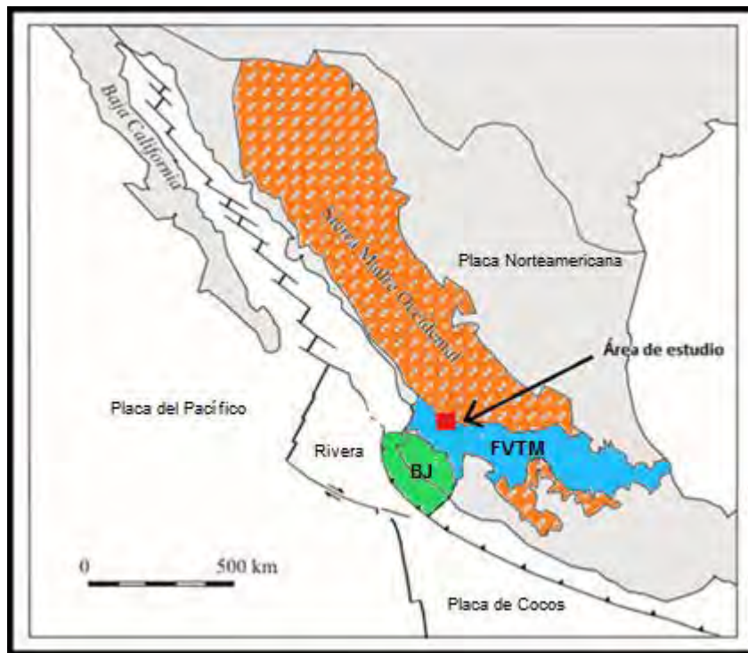
Figura 2. Ubicación de las tres provincias mayores: Sierra Madre Occidental (SMO), Faja Volcánica Trans-Mexicana (FVTM) y el Bloque Jalisco (JB), así como de la zona de estudio. Modificada de Ferrari et al, 2000
