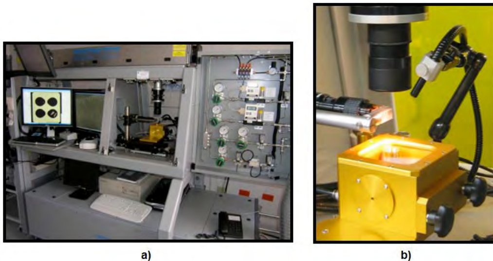
Figura 7. a) Laser Resonetics Resolution M-50 del Laboratorio de Estudios Isotópicos del CGEO. b) Detalle del mismo dispositivo donde se emite el haz de Ar sobre los zircones.
