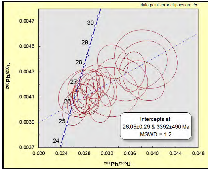
Figura 14. Gráfico de Wetherill con resultados para la muestra SPA-31. Tendencia de los datos a una intersección en 26.05 \pm 0.29 Ma.
