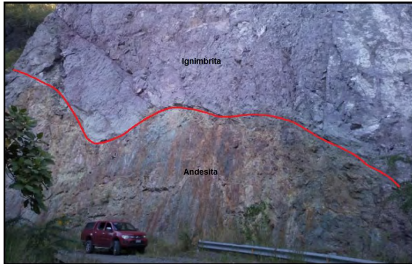
Figura 23. Imagen que muestra la posición estratigráfica de la andesita con respecto a otras unidades. (en este caso, respecto a una ignimbrita) La andesita es la roca más antigua.
