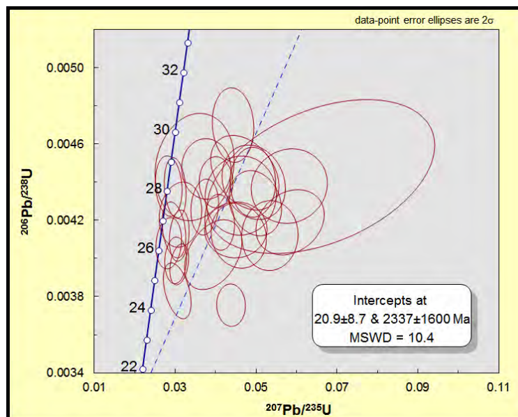
Figura 15. Gráfico de Wetherill con resultados para la muestra SPA-18C. Buena parte de los datos son discordantes y con una gran dispersión, por lo que la intersección de la concordia cae muy lejos de los datos.
