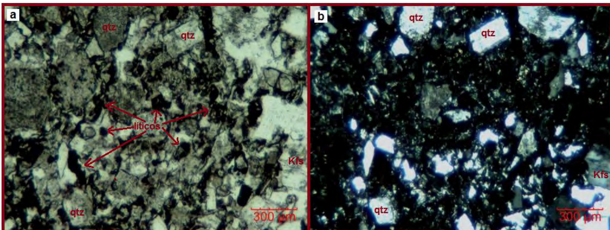
Figura 40. a) Líticos oxidados, cuarzos y feldespato potásico en nícoles paralelos de la muestra SPA-33A. b) Nícoles cruzados de SPA-33A.
