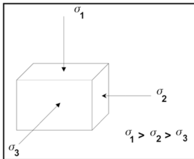
Figura 49. Ejes principales de esfuerzo
