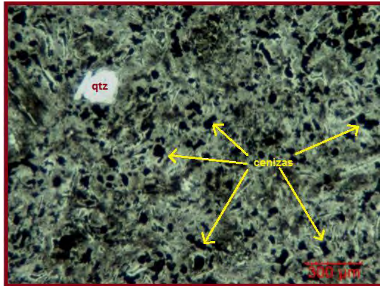
Figura 29. Imagen vista con al microscopio de la muestra SPA-14. Se observa un elevado número de vidrios de ceniza con formas totalmente amorfas. En la parte izquierda se puede apreciar un cristal de cuarzo.
