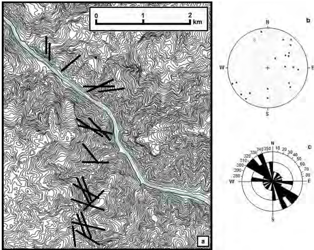
Figura 59. a) Mapa del área de afloramiento de los diques máficos. b) Diagrama estereográfico de polos de cada uno de los planos de intrusión de los diques. c) Roseta estructural que marca la orientación de los diques.
