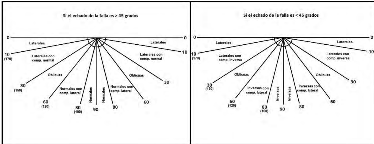
Figura 53. Criterios para la nomenclatura de las fallas basado en el ángulo de echado y en el del pitch de las estrías
