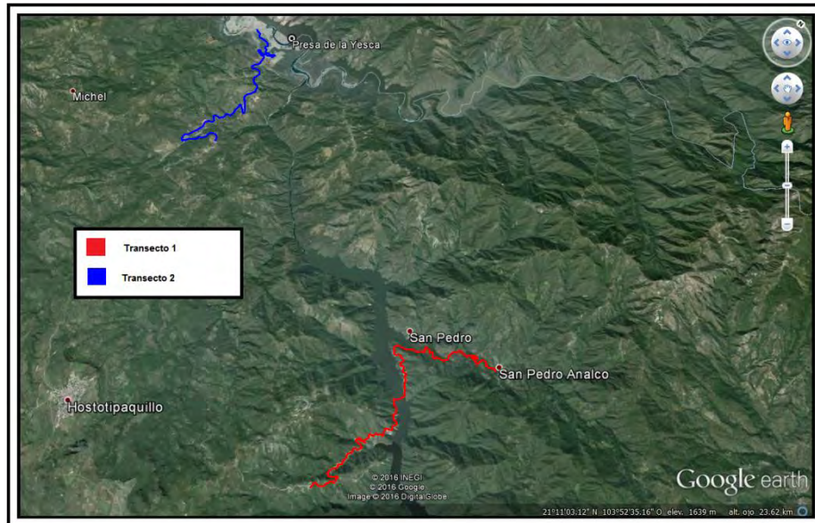
Figura 6. Se muestra la ubicación de cada uno de los transectos trabajados durante las temporadas de campo. Imagen satelital tomada de Google Earth
