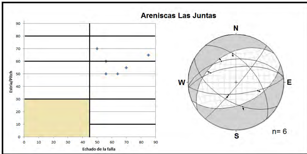
Figura 57. Gráfica dip vs pitch y diagrama de mecanismo focal de las Areniscas Las Juntas
