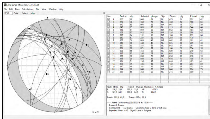
Figura 8. Captura de pantalla del software FaultKin durante el procesamiento de los datos de este trabajo
