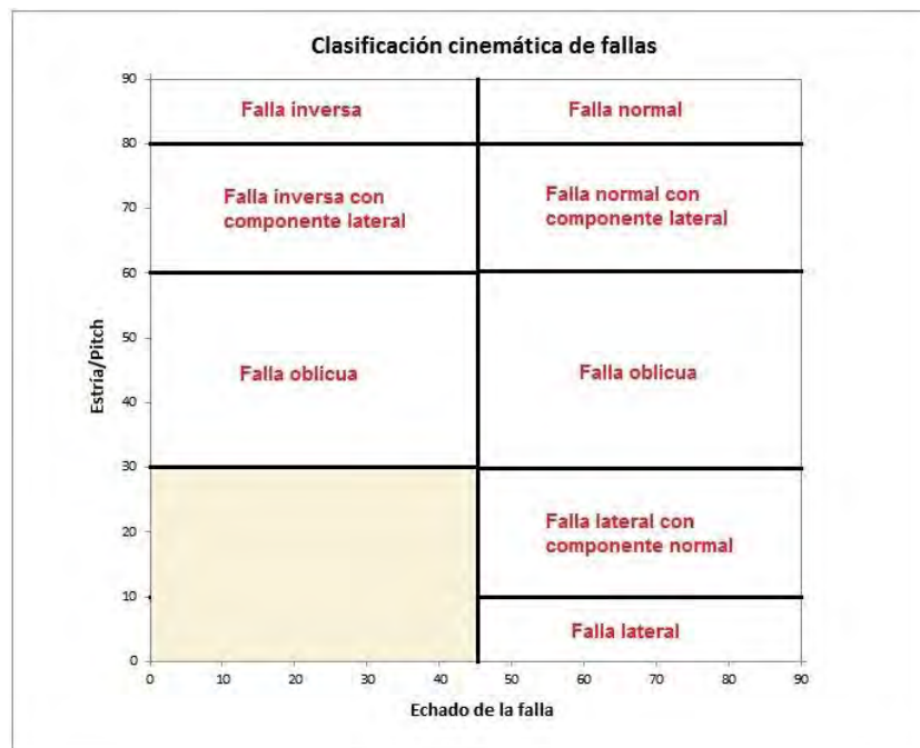
Figura 52. Diagrama elaborado para definir el tipo de cada una de las fallas estudiadas.
