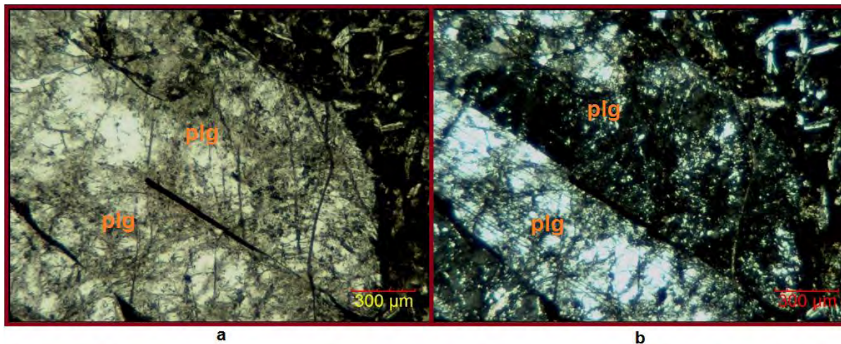
Figura 20. a) Vista al microscopio de la andesita SPA-32A, en donde se observa en detalle uno de los abundantes cristales de plagioclasa. b) Misma vista de la plagioclasa con nicoles cruzados
