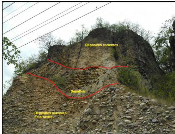
Figura 45. Imagen que muestra el orden cronológico del depósito de las últimas tres unidades descritas.
