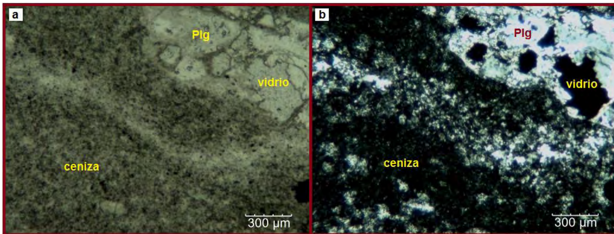
Figura 44. Lámina delgada de la muestra SPA-36 a) Se observa abundante ceniza como matriz y un cristal de plagioclasa b) Nícoles cruzados de SPA-36.
