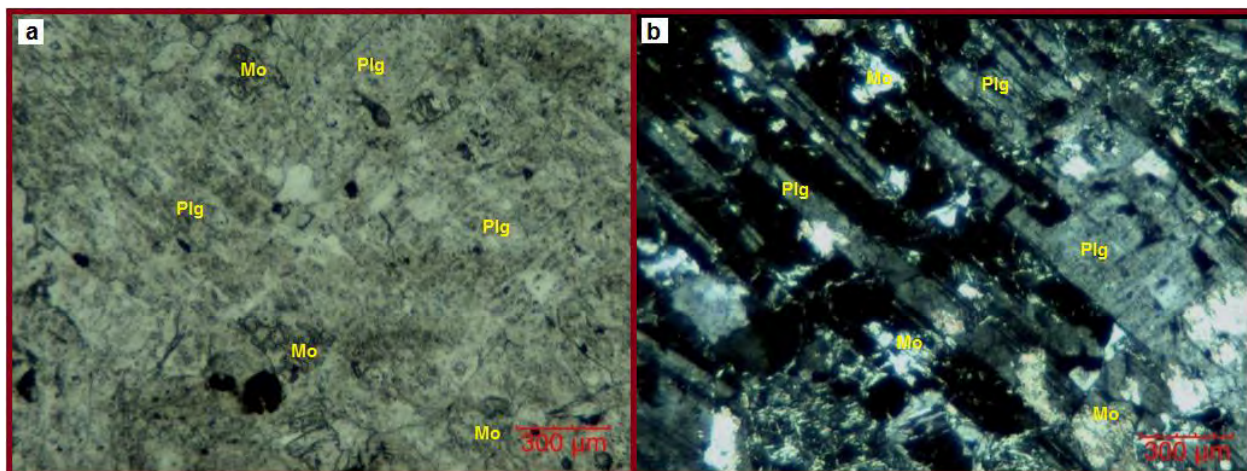
Figura 32. a) Pequeños cristales de mica blanca de grano fino que alteran a un fenocristal de plagioclasa de la lámina SPA-34. b) Misma lámina con nícoles cruzados donde se aprecia el maclado polisintético de las plagioclasas
