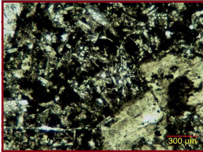
Figura 21. Detalle de la matriz traquítica de la andesita por la presencia de numerosos microlitos de plagioclasa.
