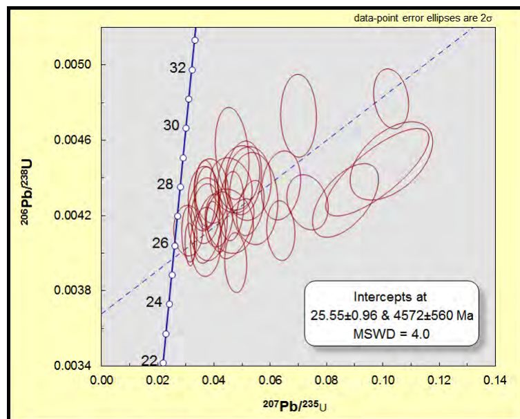
Figura 16. Gráfico de Wetherill con resultados para la muestra SPA-7.
