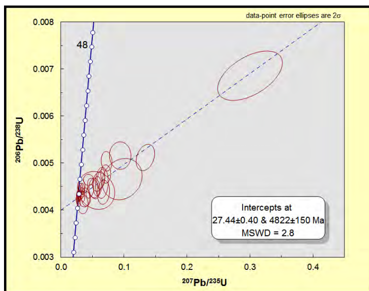
Figura 12. Gráfico de Wetherill con resultados para la muestra SPA-22. Presenta una alta concentración de datos concordantes en la intersección. Solo se observa un dato demasiado aislado.
