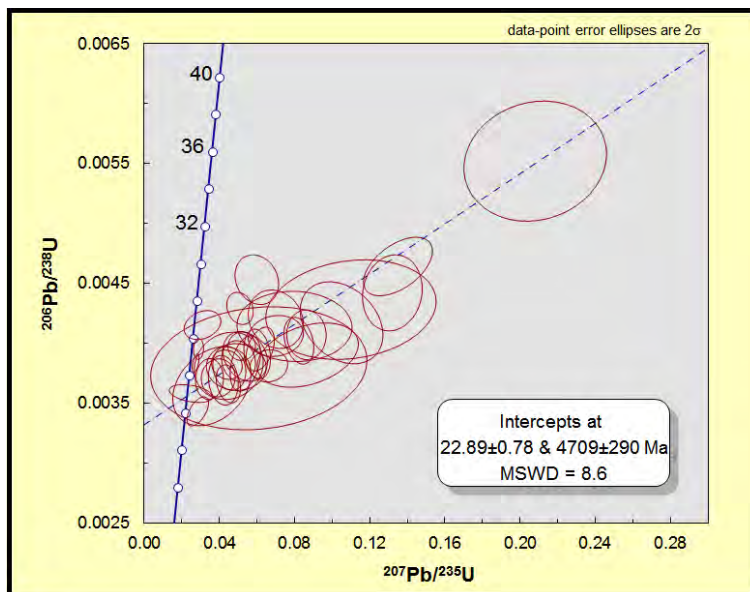
Figura 11. Gráfico de Wetherill con resultados para la muestra SPA-2. La mayoría de los datos presentan edades concordantes.
