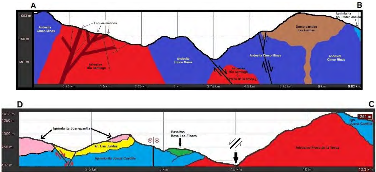
Figura 48. Secciones estructurales de los transectos trabajados durante las jornadas de campo
