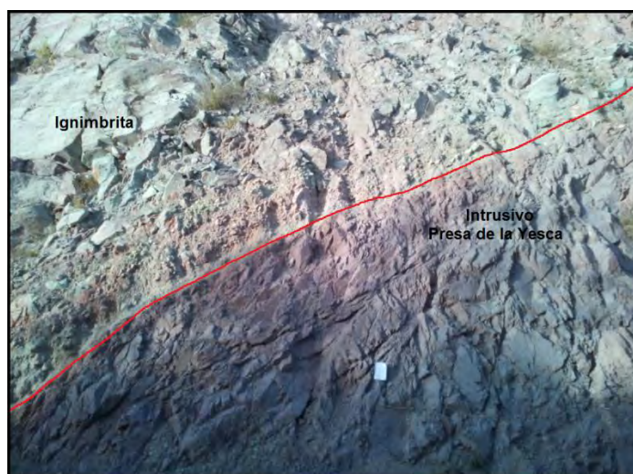
Figura 24. Contacto por plano de falla entre el Intrusivo Presa de la Yesca y una ignimbrita en color verde más reciente.
