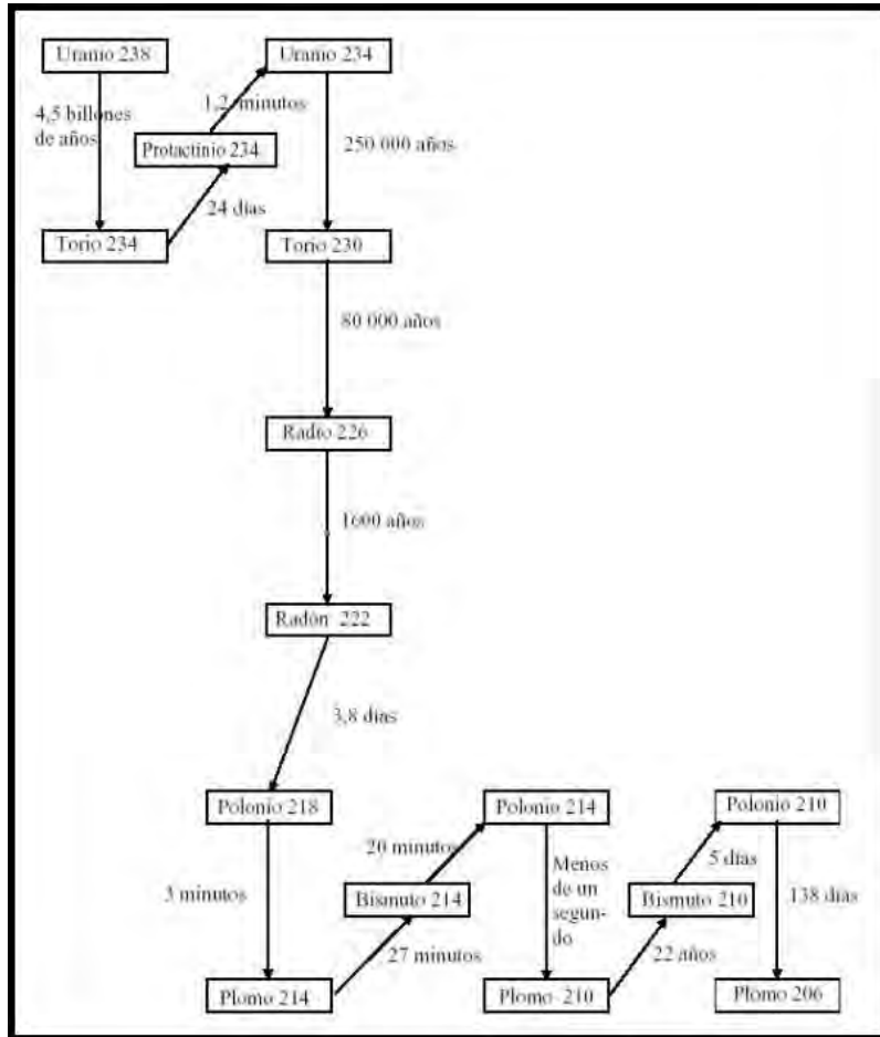
Figura 9. Serie de desintegración del ^{238}\text{U} con los tiempos de vida media en cada paso. Tomada de Cánovas-Picón, 2007
