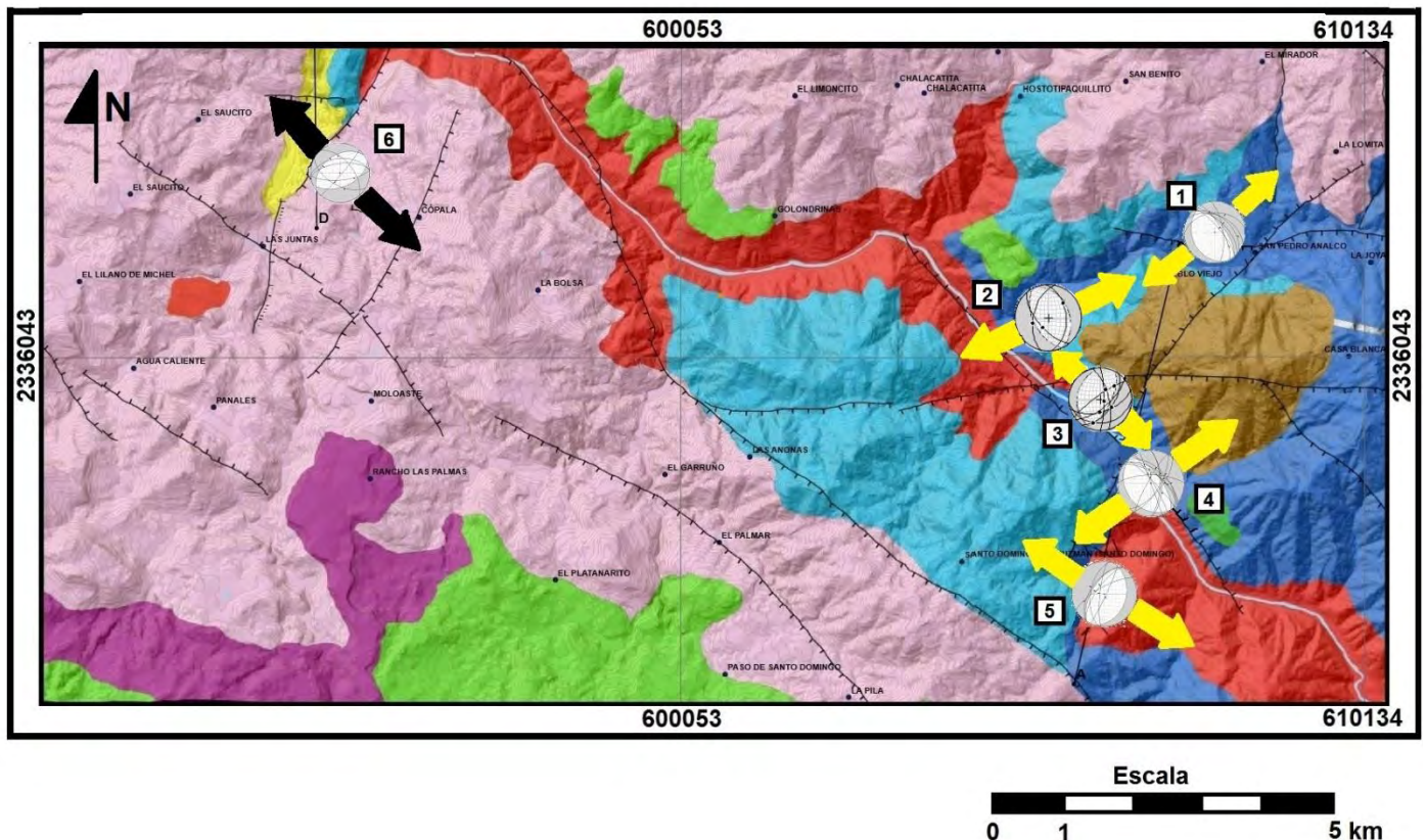
Figura 58. Detalle del mapa del área de estudio con la ubicación de los mecanismos focales. Los diagramas 1 y 4 superpuestos corresponden al diagrama de la Andesita Cinco Minas mostrado en la sección de análisis de este capítulo, mientras que los diagramas 2 y 3 generan al diagrama analizado de la Ignimbrita San Pedro Analco. Los diagramas 5 y 6 del Intrusivo Río Santiago y de las Areniscas Las Juntas, respectivamente, son los mismos presentados en el análisis cinemático.
