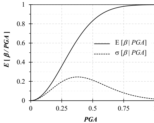
Figura 1.14. Ejemplo de una función de vulnerabilidad sísmica
