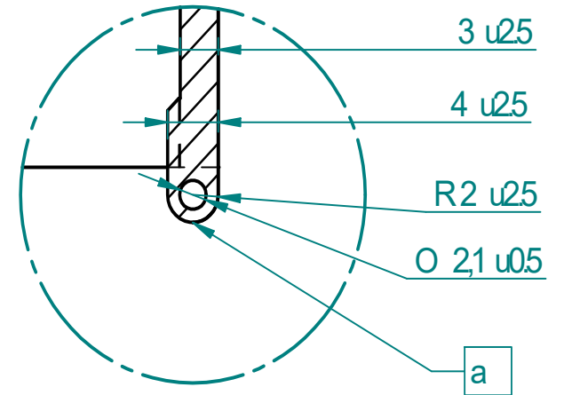
DETALE B
