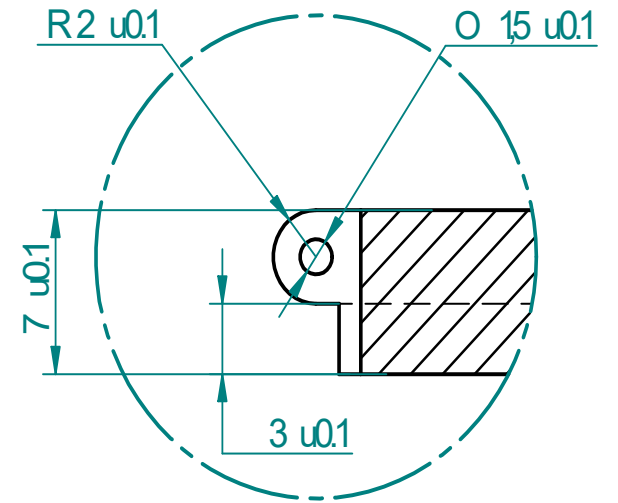
DETAL B
