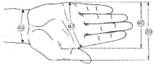
Figura 3.2.2 Medidas principales de la mano (Según Norma DIN 33.402 segunda parte)
