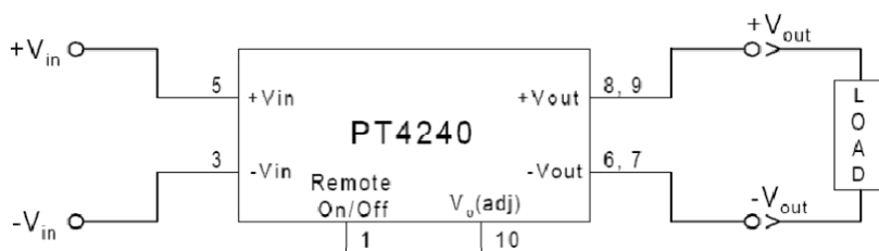
Figura 2.8.4 Regulador de voltaje del tipo aislado
