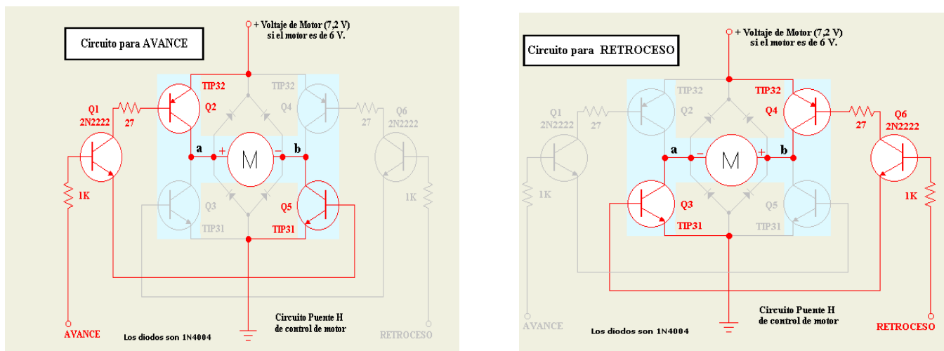
Figura 2.8.2 .Funcionamiento del Puente H (Avance y Retroceso)
