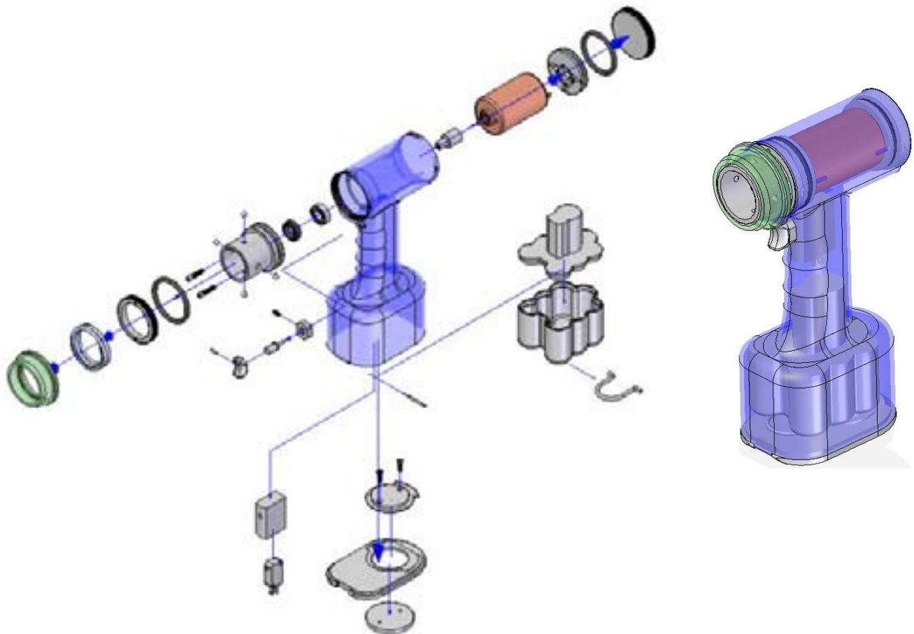
Figura T2 Explosivo del Prototipo Rápido
