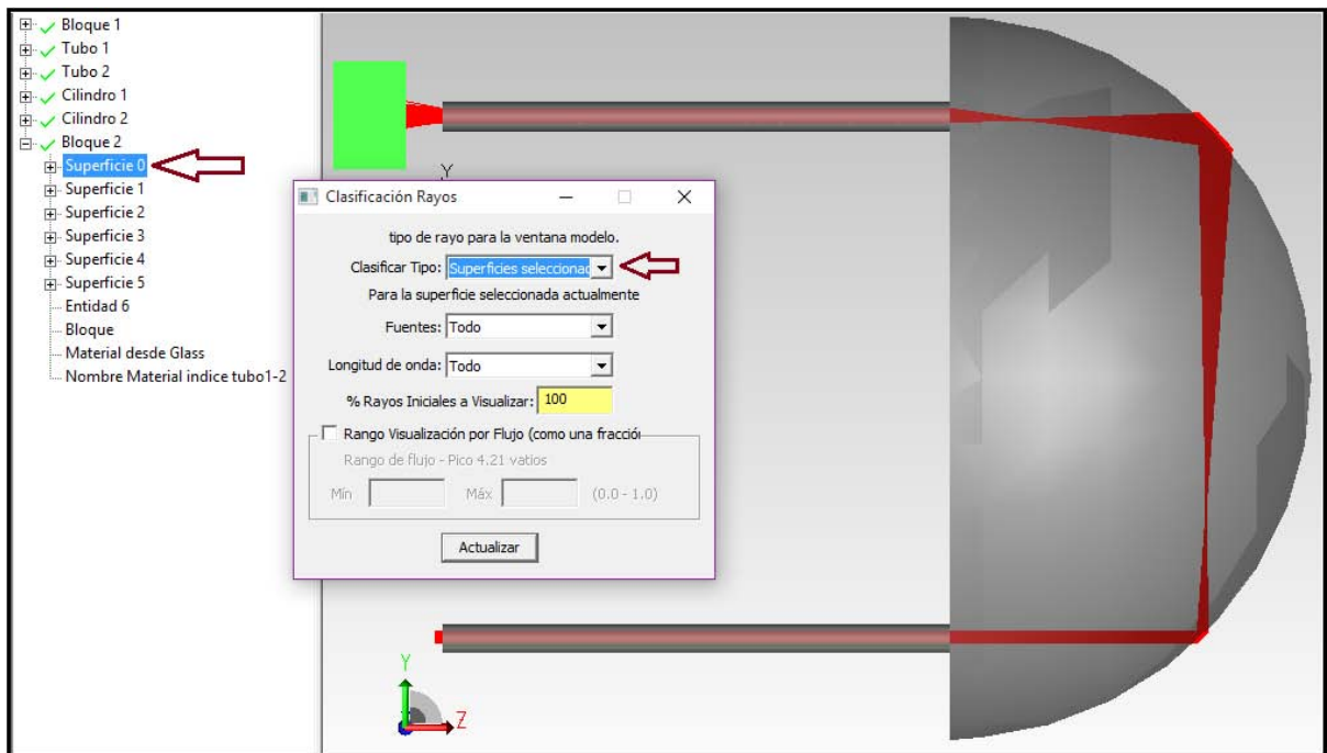
Figura 7.24. MODELO DEL TRANSDUCTOR CON SUPERFICIE SELECCIONADA PARA LA DETERMINACION DEL FLUJO RADIANTE A LA SALIDA DELA FIBRA OPTICA F2
