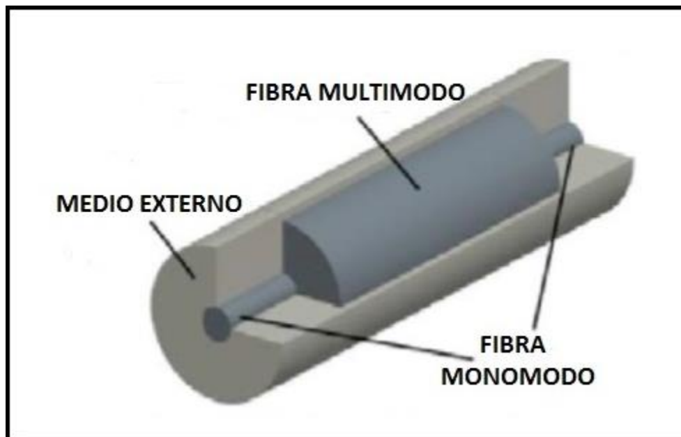
Figura 4.9. SENSOR REFRACTOMÉTRICO CON ESTRUCTURA MONOMODO-MULTIMODO-MONOMODO
