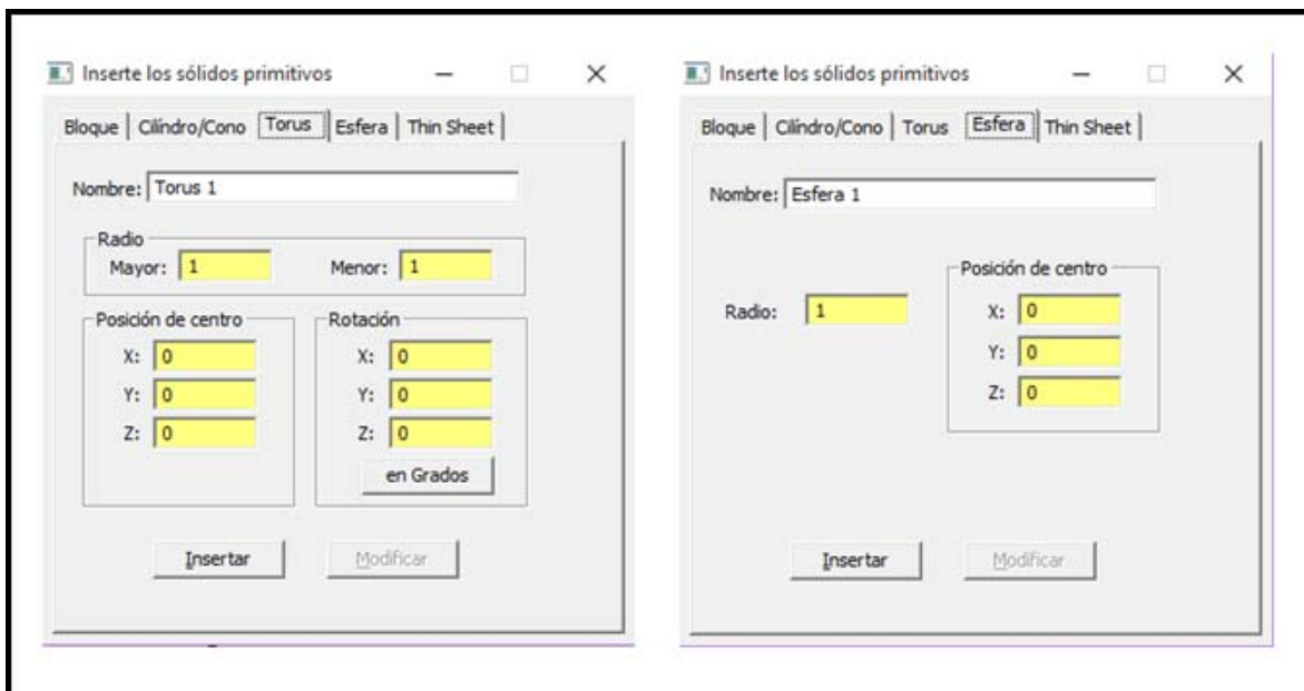
Figura 7.7. PANTALLA CON LAS ESPECIFICACIONES DE UN SOLIDO PRIMITIVO EN LA PESTAÑA TORUS Y ESFERA
