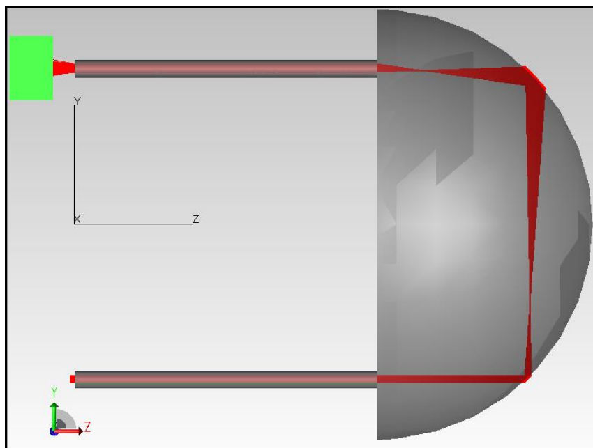
Figura 7.22. TRAZADO DE RAYOS EN EL TRANSDUCTOR DE LA FIGURA 7.21
