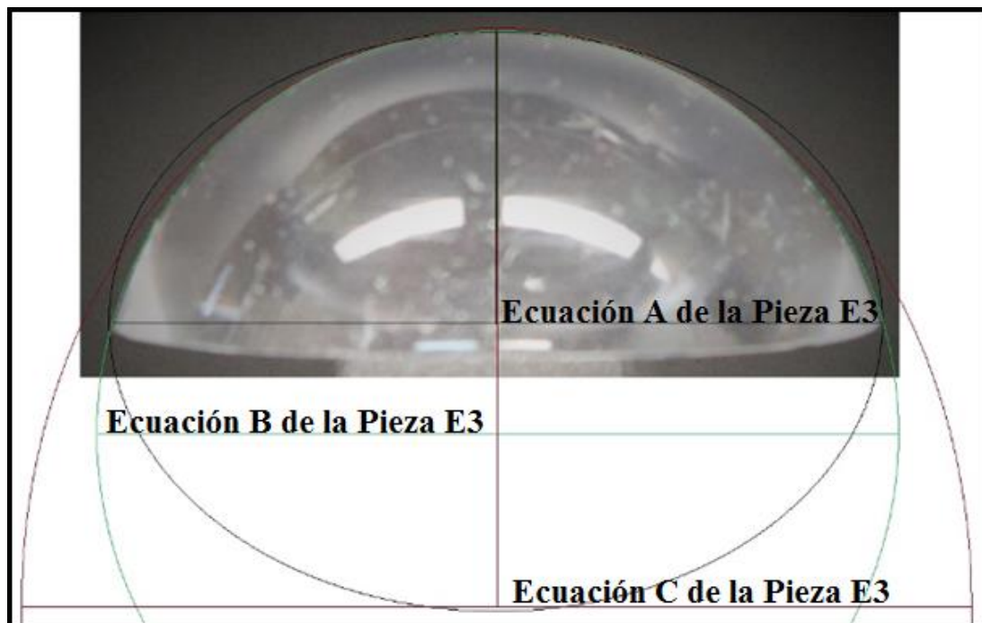
Figura 9.1. VARIANTES DE APROXIMACION DE SUPERFICIE CON TRES ELIPSOIDES DIFERENTES DE LA PIEZA E3
