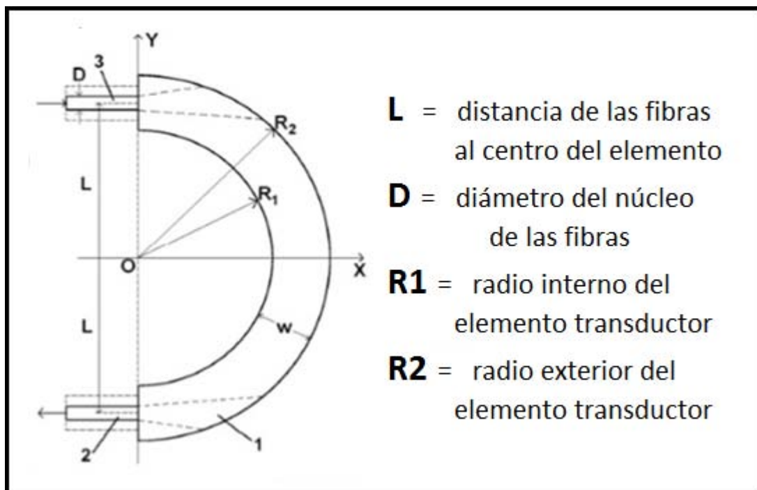
Figura 4.8. SENSOR REFRACTOMÉTRICO CON ELEMENTO DE DETECCIÓN SEMICILÍNDRICO
