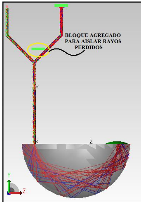
Figura 7.44. MODELO DEL TRANSDUCTOR EN EL MODO DE REFLEXION CON UN ACOPLADOR DIRECCIONAL DE FIBRA OPTICA Y UN BLOQUE AGREGADO QUE ABSORBE LOS RAYOS QUE SALEN DEL ACOPLADOR
