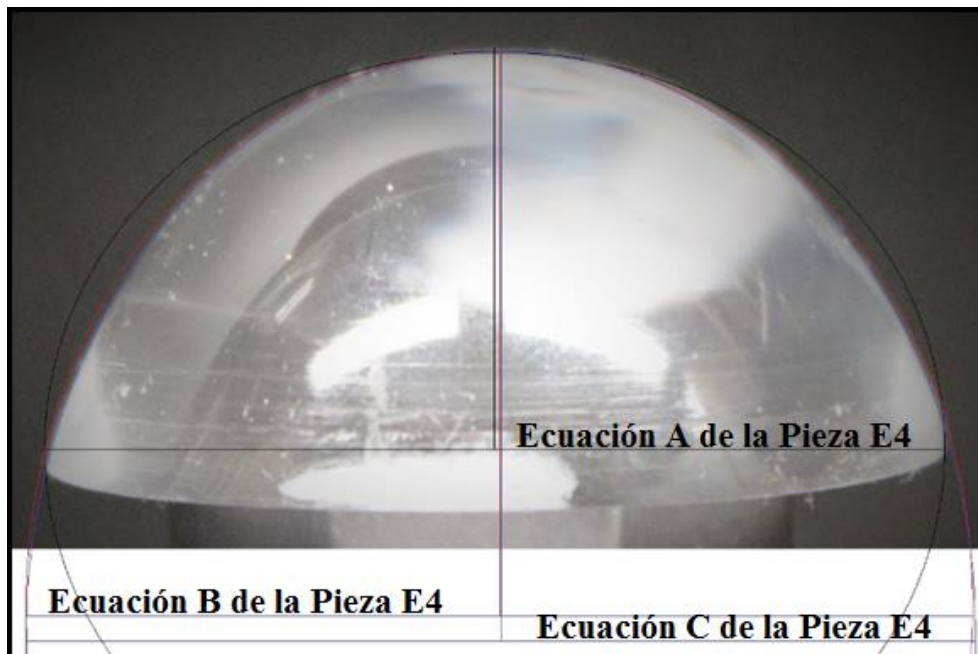
Figura 9.9. VARIANTES DE APROXIMACION DE SUPERFICIE CON TRES ELIPSOIDES DIFERENTES DE LA PIEZA E4
