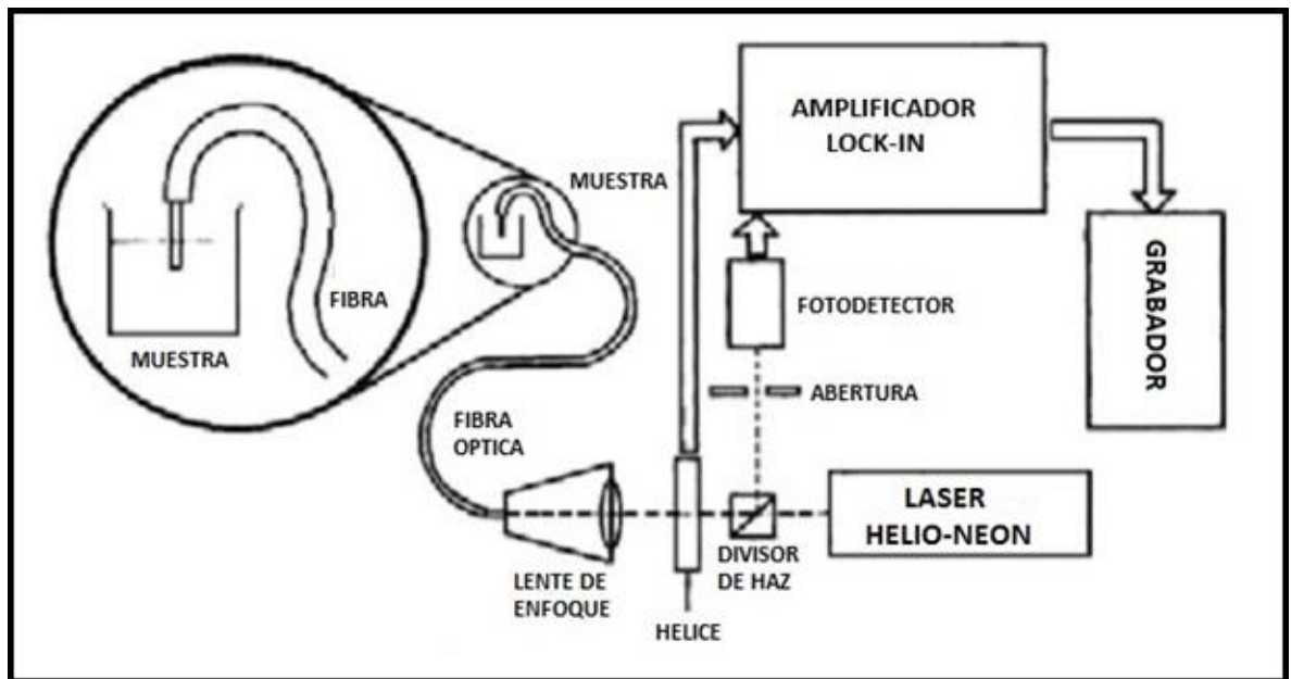
Figura 4.4. SISTEMA DE SENSADO REFRACTOMÉTRICO DE FIBRA ÓPTICA
