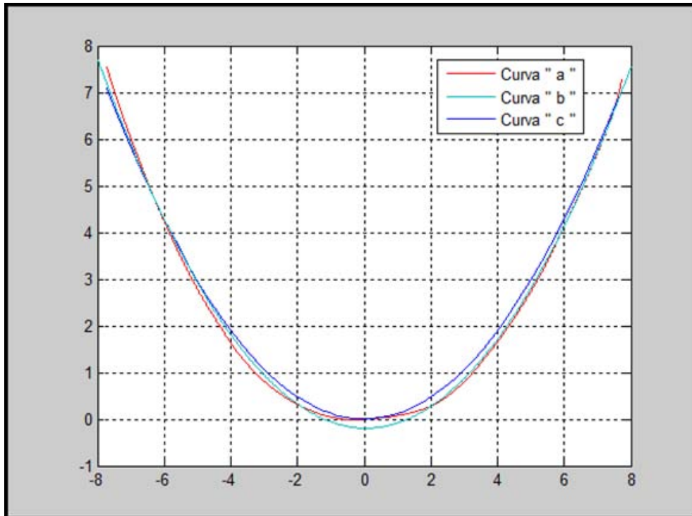
FIGURA 1 CONTORNOS DEL TRANSDUCTOR: a) OBTENIDO MEDIANTE DIGITALIZACION DE FOTOGRAFIA b) OBTENIDO MEDIANTE COMANDO POR DEFECTO DE MATLAB c) OBTENIDO MEDIANTE UN PROGRAMA DE MATLAB
