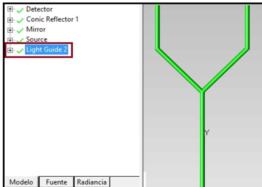
Figura 7.42. PANTALLA E IMAGEN DE LA UNION DE DOS GUIAS DE LUZ EN UNA SOLA (MODELO DE UN ACOPLADOR DIRECCIONAL DE FIBRA OPTICA)
