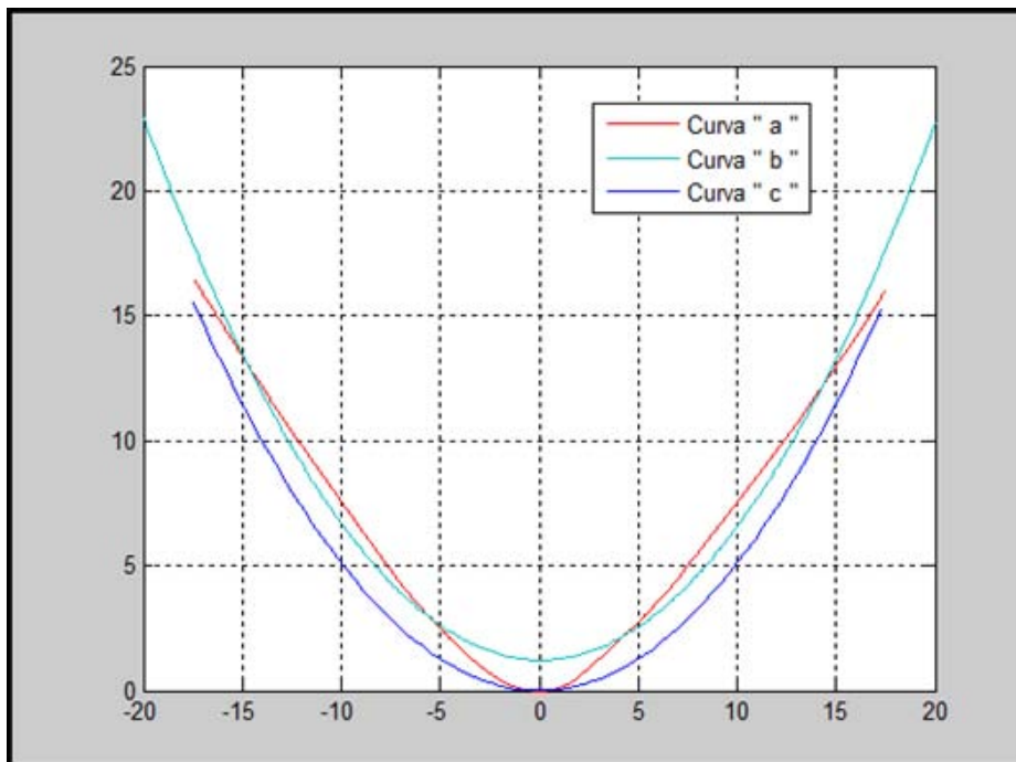
FIGURA 28. CONTORNOS DEL TRANSDUCTOR: a) OBTENIDO MEDIANTE DIGITALIZACION DE FOTOGRAFIA b) OBTENIDO MEDIANTE COMANDO POR DEFECTO DE MATLAB OBTENIDO MEDIANTE UN PROGRAMA DE MATLAB
