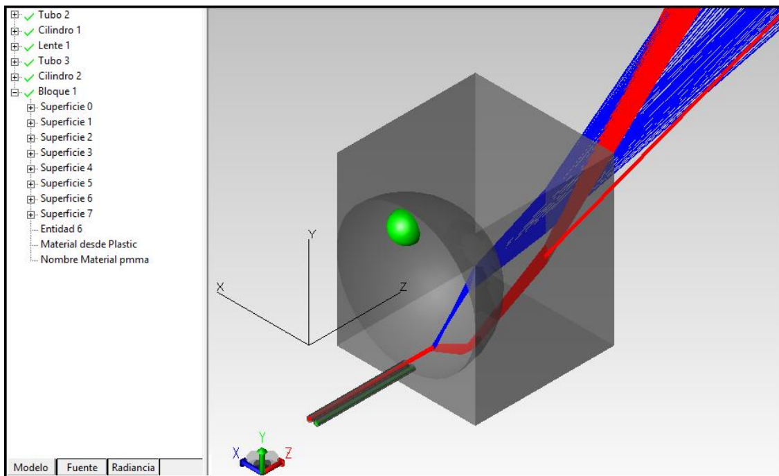
Figura 7.19. PANTALLA E IMAGEN DEL TRAZADO DE RAYOS EN BLOQUE CON CAVIDAD ESFERICA
