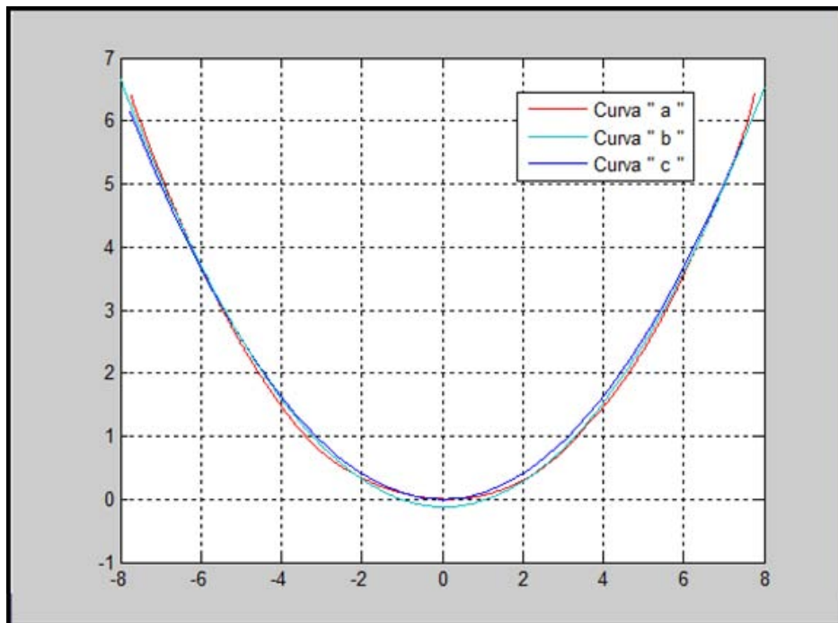
FIGURA 4. CONTORNOS DEL TRANSDUCTOR: a) OBTENIDO MEDIANTE DIGITALIZACION DE FOTOGRAFIA b) OBTENIDO MEDIANTE COMANDO POR DEFECTO DE MATLAB c) OBTENIDO MEDIANTE UN PROGRAMA DE MATLAB
