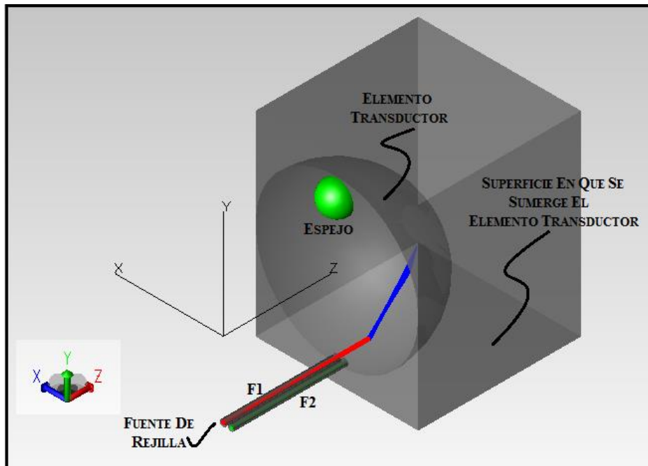
Figura 7.11. MODELO DEL TRANSDUCTOR CON FUENTE DE REJILLA, F1, F2, ESPEJO, ELEMENTO TRANSDUCTOR Y SUPERFICIE DONDE SE SUMERGE AL ELEMENTO
