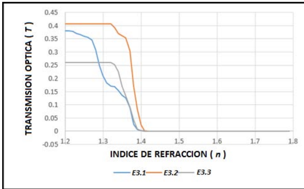
Figura 9.8. TRANSMISION OPTICA T Vs. INDICE DE REFRACCION n PARA TRANSDUCTOR E3
