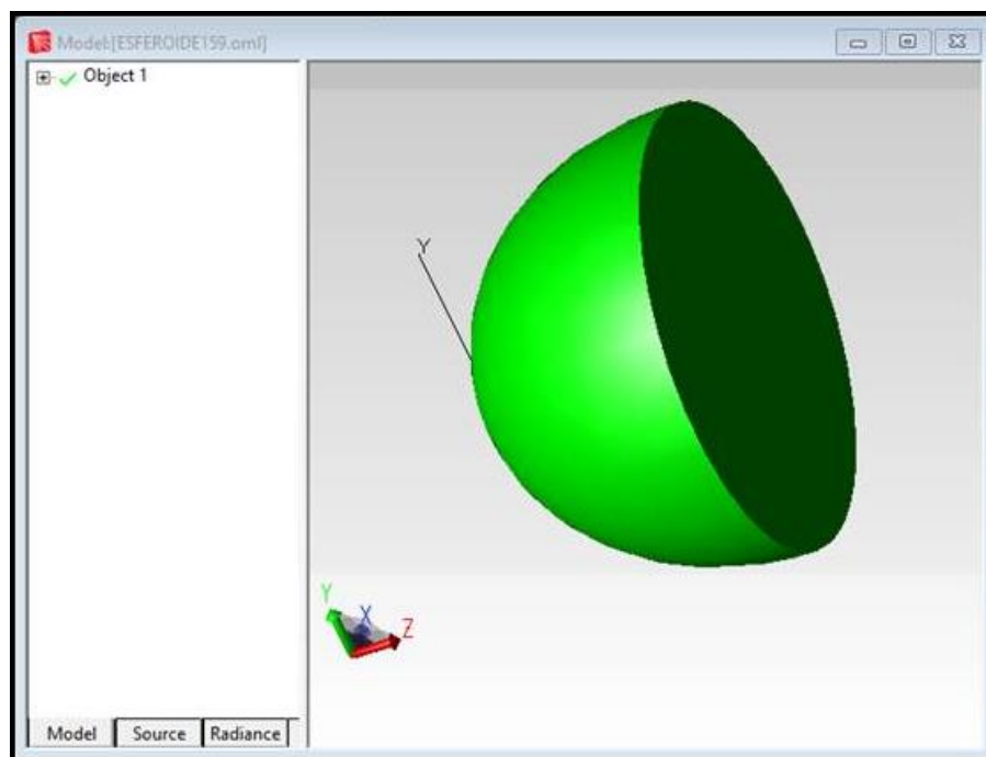
Figura 7.47. ELIPSOIDE CON DIAMETRO 15.90 mm CREADO EN AUTOCAD CON ARCHIVO SAT (ACIS) Y ABIERTO EN TRACEPRO
