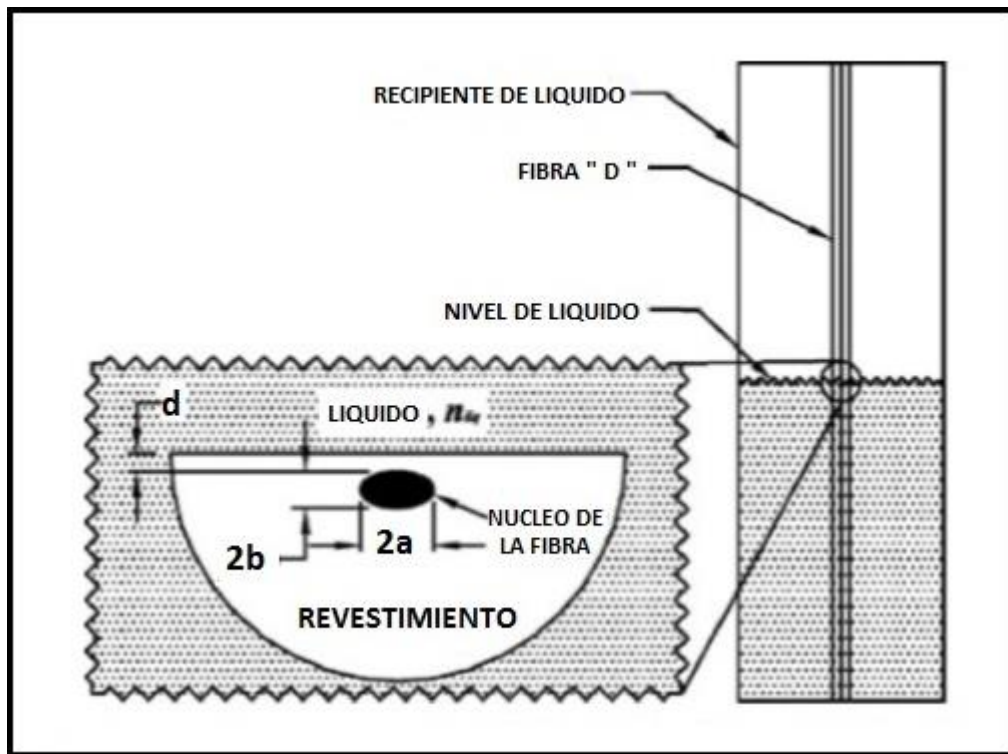
Figura 4.5. SISTEMA DE SENSADO DE NIVEL DE LÍQUIDO DE FIBRA ÓPTICA EN FORMA "D"
