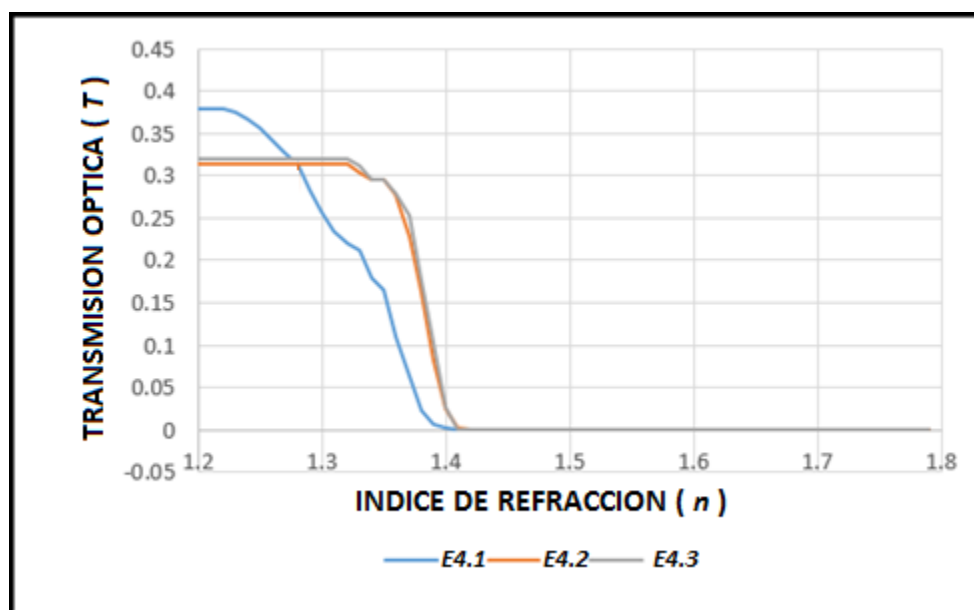
Figura 9.14. TRANSMISION OPTICA T Vs. INDICE DE REFRACCION n PARA TRANSDUCTOR E4
