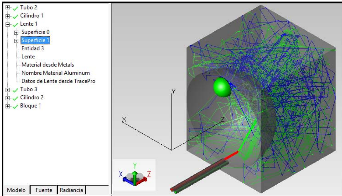
Figura 7.20. PANTALLA E IMAGEN DEL TRAZADO DE RAYOS EN BLOQUE CON CAVIDAD ESFERICA
