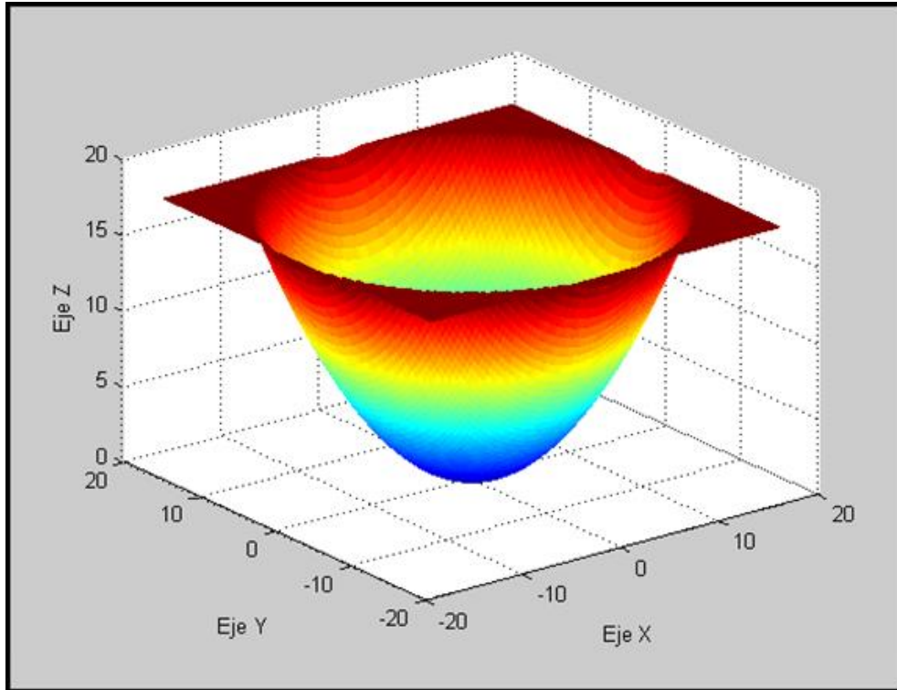
FIGURA 29. Pieza P10 en 3D
