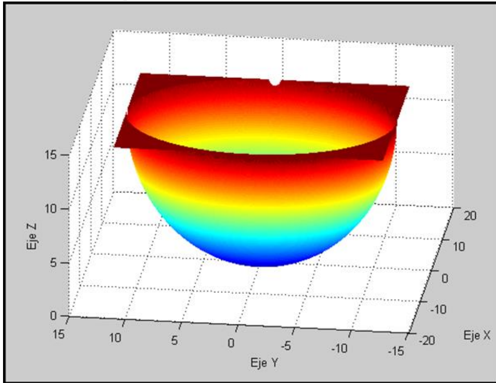
FIGURA 17. Pieza E6 en 3D
