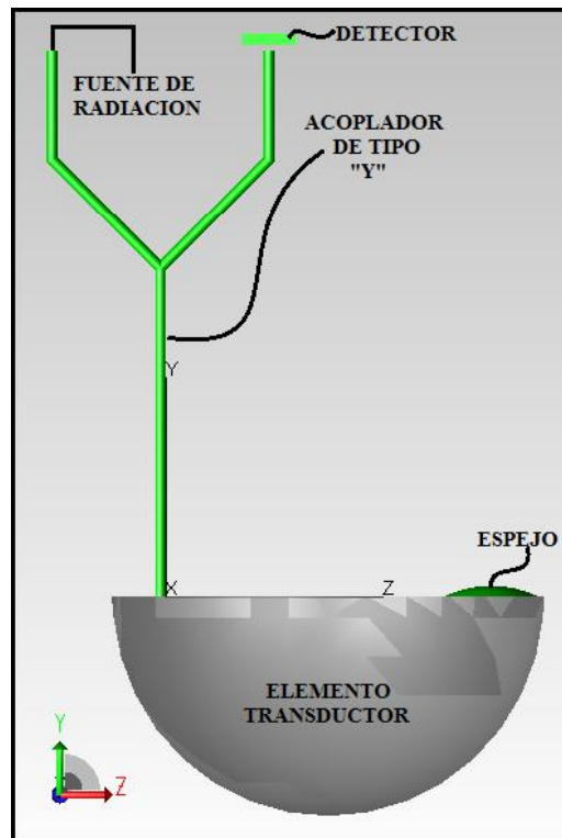
Figura 7.39. MODELO DEL TRANSDUCTOR EN EL MODO DE REFLEXION CON UN ACOPLADOR DIRECCIONAL DE FIBRA OPTICA TIPO "Y", FUENTE DE RADIACION, UN ESPEJO Y UN FOTODETECTOR
