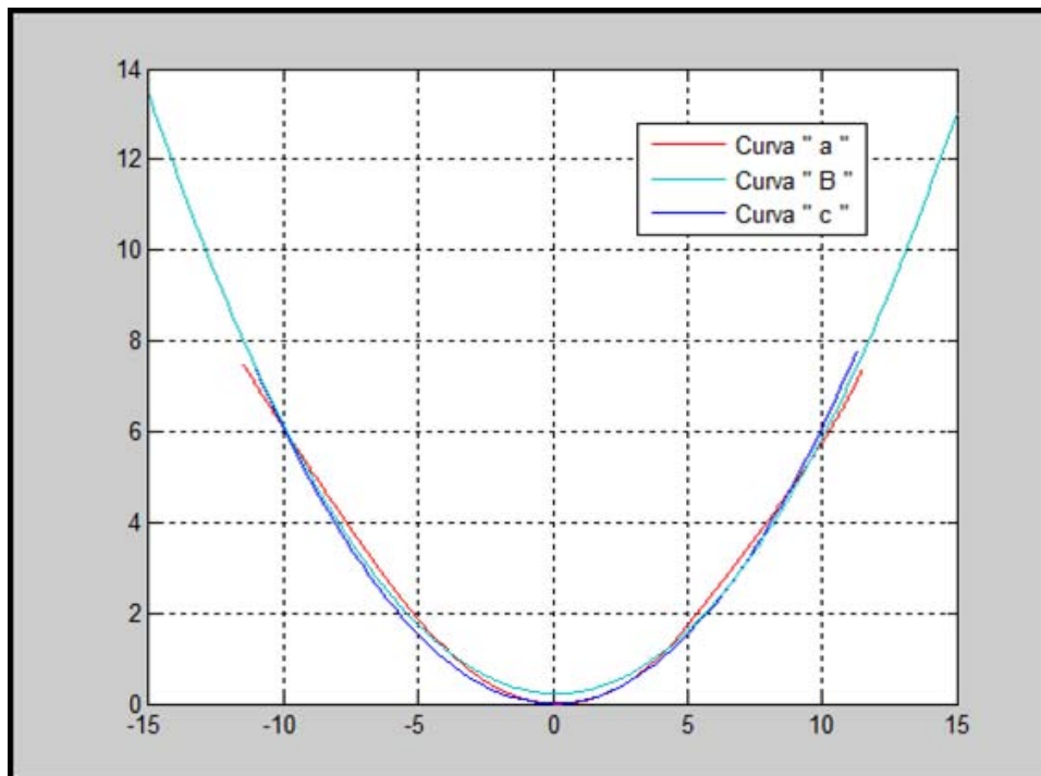
FIGURA 10. CONTORNOS DEL TRANSDUCTOR: a) OBTENIDO MEDIANTE DIGITALIZACION DE FOTOGRAFIA b) OBTENIDO MEDIANTE COMANDO POR DEFECTO DE MATLAB OBTENIDO MEDIANTE UN PROGRAMA DE MATLAB
