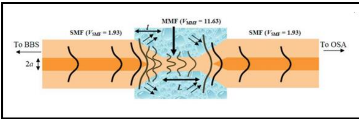
Figura 4.6. DIAGRAMA DE SENSOR REFRACTOMÉTRICO DE FIBRA ÓPTICA ESTRECHA
