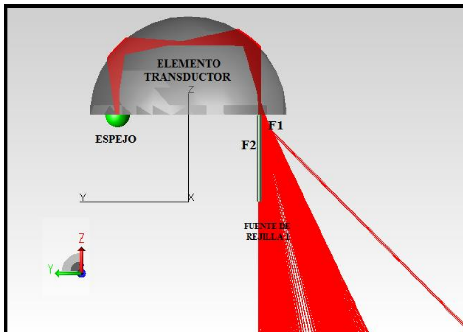
FIGURA 7.10. MODELO DEL TRANSDUCTOR CON FUENTE DE REJILLA, F1, F2, ESPEJO Y ELEMENTO TRANSDUCTOR; PLANO YZ
