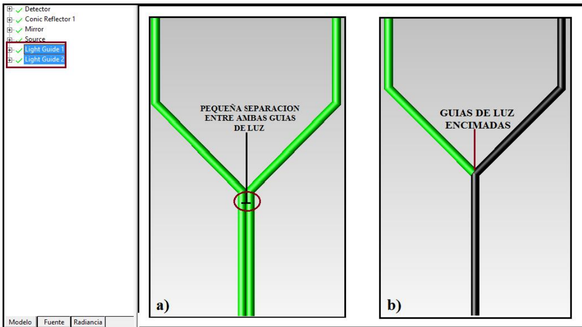
Figura 7.41. PANTALLA E IMAGEN DE MODELOS DE DOS GUIAS DE LUZ PARALELAS: a) DOS GUIAS DE LUZ CON PEQUEÑA SEPARACION, b) GUIA DE LUZ ENCIMADA UNA EN LA OTRA
