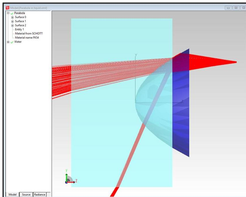
Figura 7.50. PARABOLOIDE DENTRO DEL BLOQUE (REPRESENTA EL AGUA) Y TRAYECTORIAS DE HACES DE LUZ
