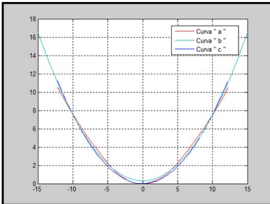
FIGURA 19. CONTORNOS DEL TRANSDUCTOR: a) OBTENIDO MEDIANTE DIGITALIZACION DE FOTOGRAFIA b) OBTENIDO MEDIANTE COMANDO POR DEFECTO DE MATLAB OBTENIDO MEDIANTE UN PROGRAMA DE MATLAB
