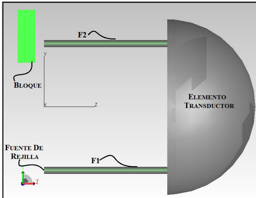
Figura 7.21. MODELO DEL TRANSDUCTOR EN EL MODO DE TRANSMISION CON FUENTE DE REJILLA, DOS FIBRAS OPTICAS F1 Y F2, ELEMENTO TRANSDUCTOR Y BLOQUE
