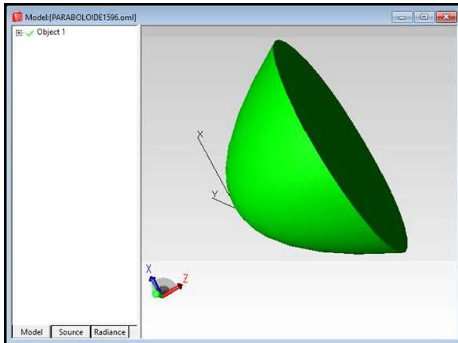
Figura 7.48. PARABOLOIDE CON DIAMETRO 15.96 mm CREADO EN AUTOCAD CON ARCHIVO SAT (ACIS) Y ABIETO EN TRACEPRO
