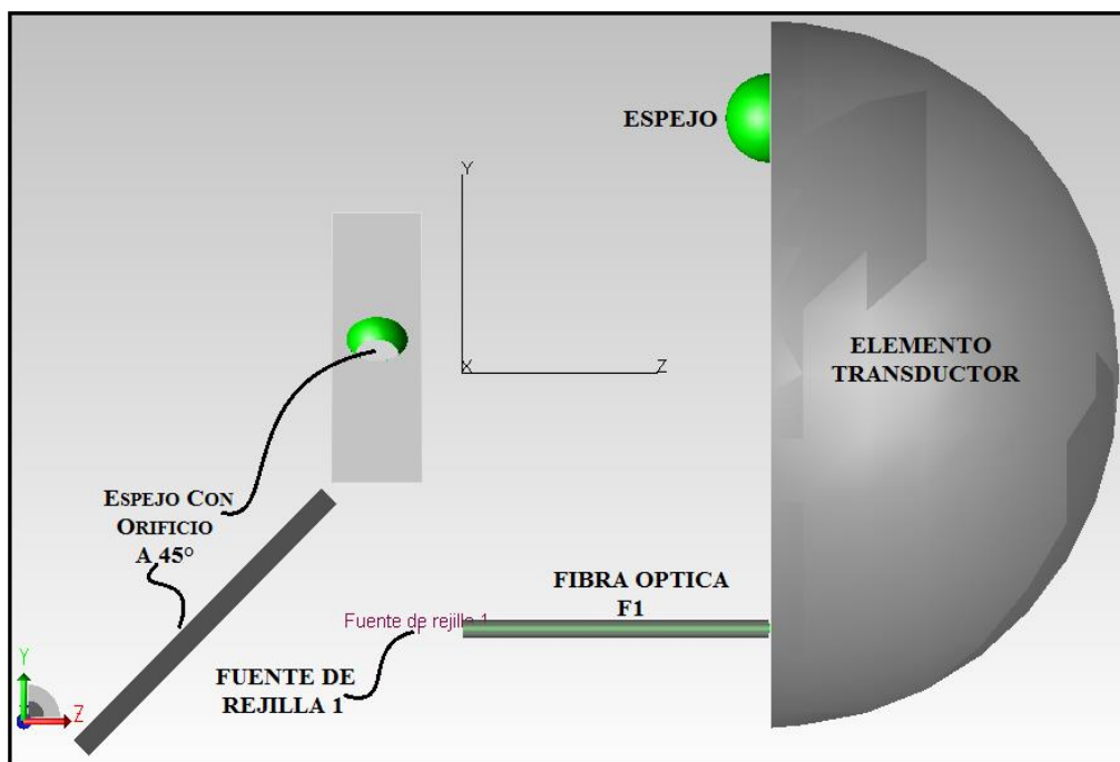
Figura 7.29. MODELO DEL TRANSDUCTOR EN EL MODO DE REFLEXION CON UN DIVISOR DEL HAZ (UN ESPEJO INCLINADO A 45°)
