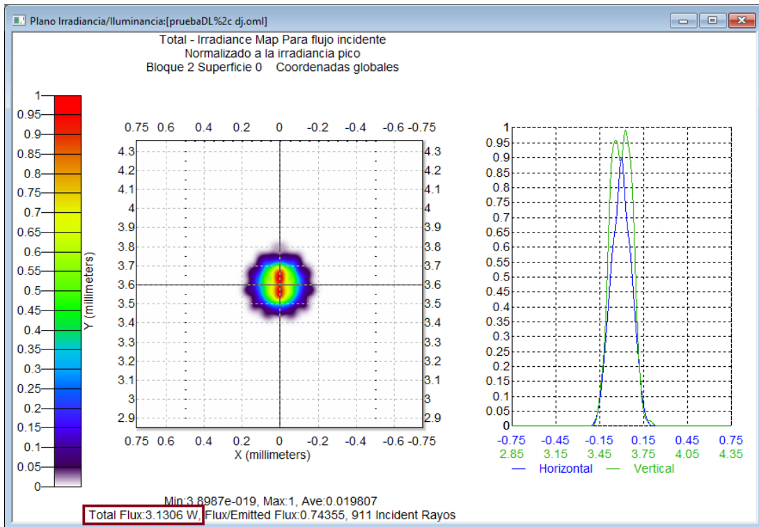
Figura 7.26. PANTALLA CON DISTRIBUCION DE FLUJO RADIANTE A LA SALIDA LA FIBRA OPTICA F2
