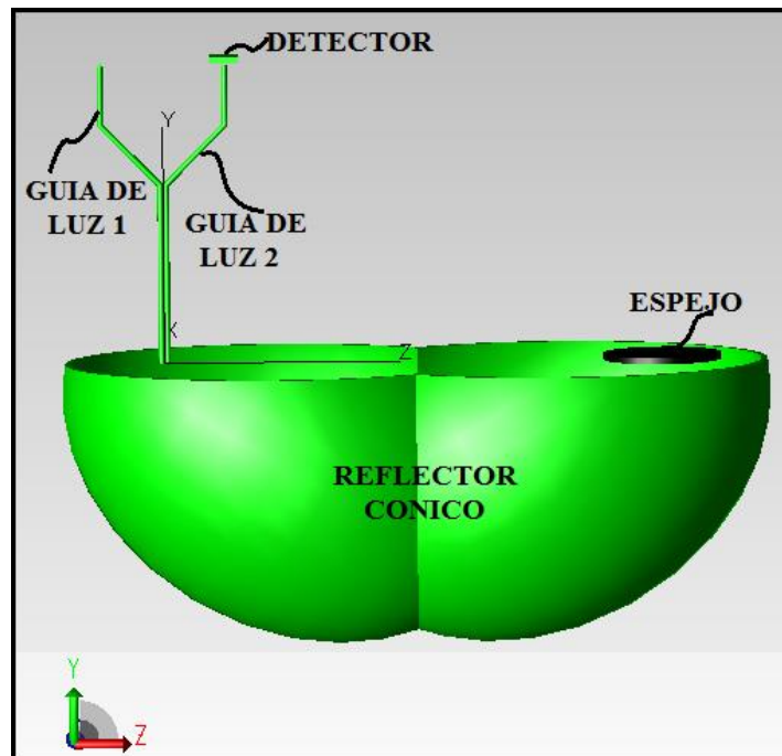
Figura 7.40. MODELO DEL TRANSDUCTOR EN EL MODO DE REFLEXION CON DOS FIBRAS OPTICAS PARALELAS
