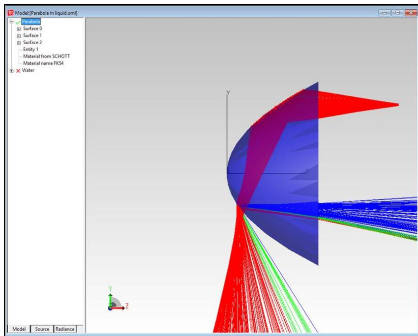
Figura 7.49. TRAZADO DE RAYOS DEL PARABOLOIDE
