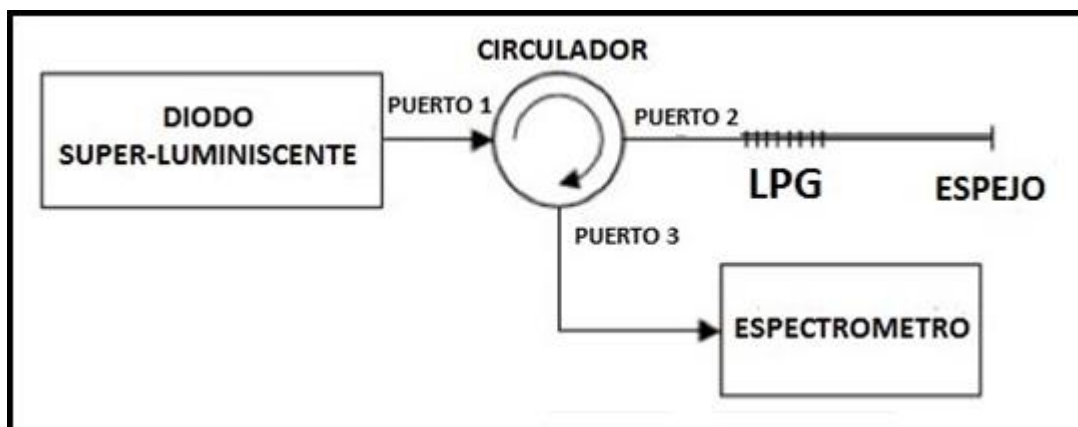
Figura 4.7. SISTEMA DE SENSADO REFRACTOMÉTRICO ÓPTICO DE REJILLAS DE PERIODO LARGO
