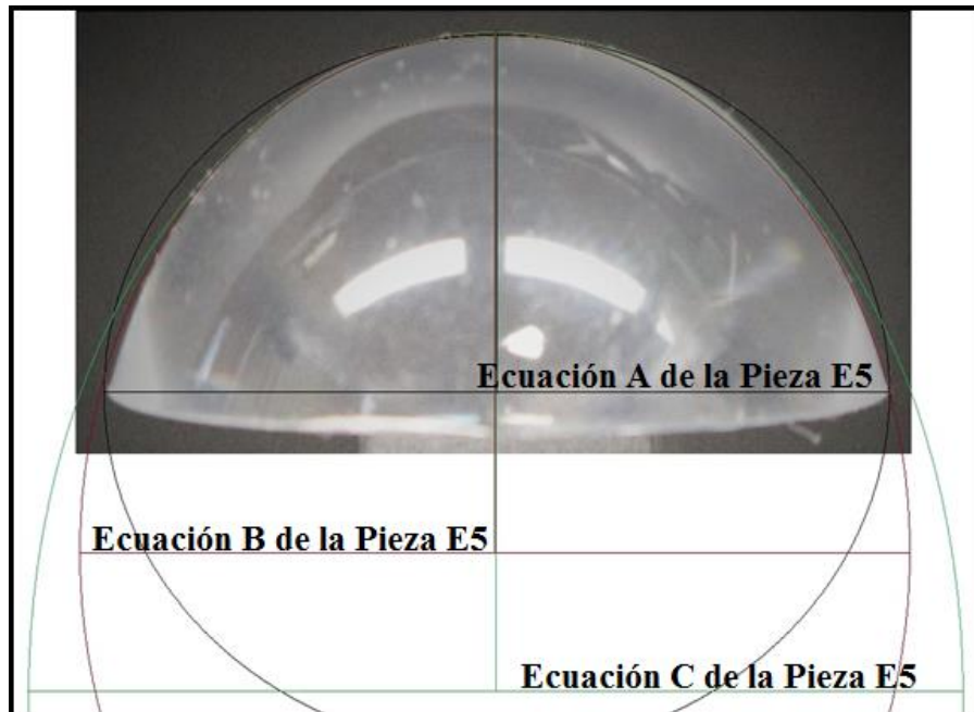
Figura 9.15. VARIANTES DE APROXIMACION DE SUPERFICIE CON TRES ELIPSOIDES DIFERENTES DE LA PIEZA E5
