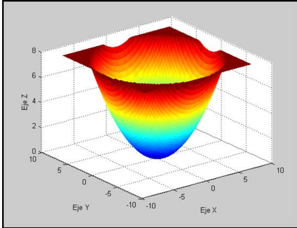
FIGURA 8. Pieza P3 en 3D
