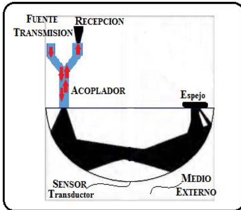
Figura 7.2. SENSOR TRANSDUCTOR CON ACOPLADOR Y UNA FIBRA OPTICA
