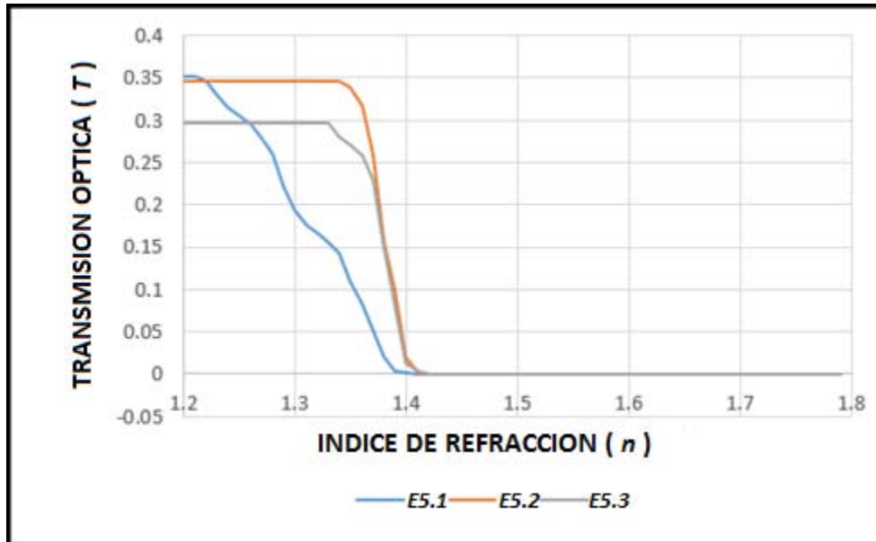
Figura 9.21. TRANSMISION OPTICA T Vs. INDICE DE REFRACCION n PARA TRANSDUCTOR E5
