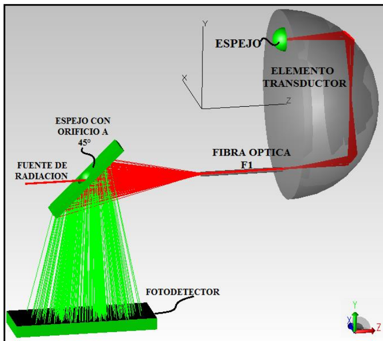
Figura 7.35. MODELO DEL TRANSDUCTOR COMPLETO EN MODO DE REFLEXION CON ESPEJO (INCLINADO A 45°), FIBRA OPTICA F1, ELEMENTO TRANSDUCTOR, ESPEJO Y FOTODETECTOR
