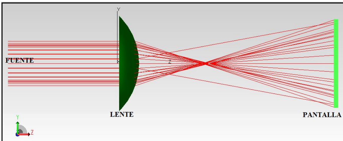
Figura 7.3. PRUEBA DE UN LENTE, UNA FUENTE Y UNA PANTALLA
