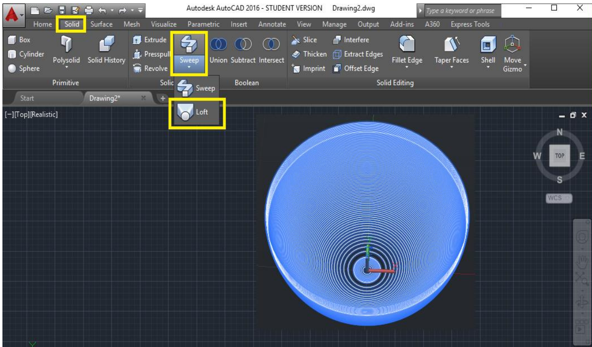
Figura 8.11. MODELADO DE UNA ELIPSOIDE: SELECCIÓN DE CADA CÍRCULO ELEMENTAL CON EL COMANDO LOFT
