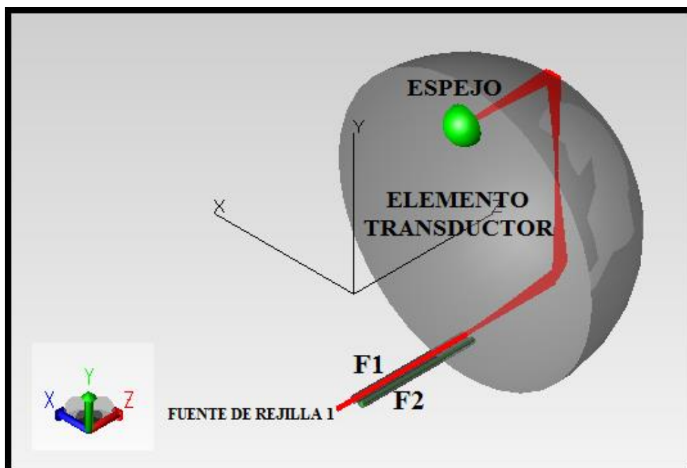
Figura 7.9. MODELO DEL TRANSDUCTOR CON LA FUENTE DE REJILLA 1, FIBRA DE TRANSMISION F1, FIBRA DE RECEPCION F2, ESPEJO Y ELEMENTO TRANSDUCTOR
