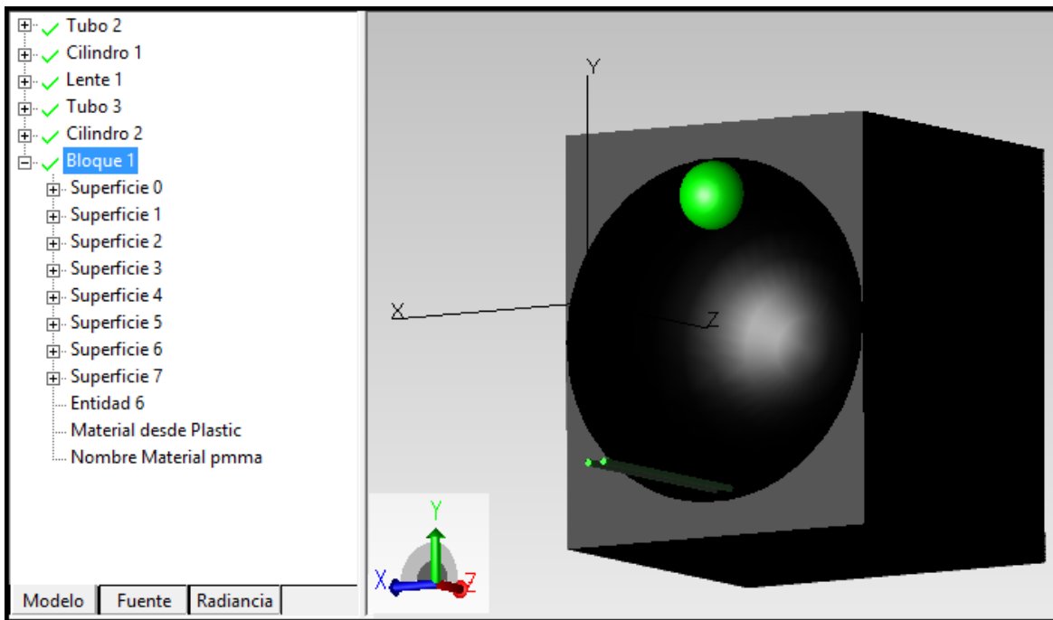
Figura 7.18. PANTALLA E IMAGEN DEL BLOQUE CON CAVIDAD ESFERICA
