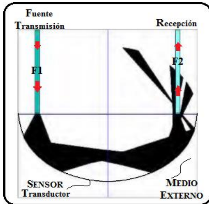
Figura 7.1. SENSOR TRANSDUCTOR CON DOS FIBRAS OPTICAS
