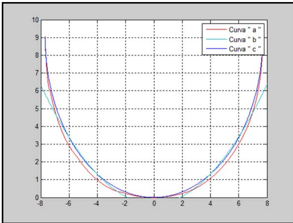
Figura 1. CONTORNOS DEL TRANSDUCTOR: a) OBTENIDO MEDIANTE DIGITALIZACION DE FOTOGRAFIA b) OBTENIDO MEDIANTE COMANDO POR DEFECTO DE MATLAB c) OBTENIDO MEDIANTE UN PROGRAMA DE MATLAB
