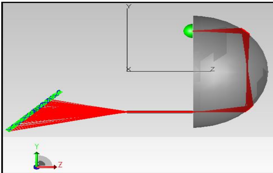
Figura 7.31. TRAZADO DE RAYOS DEL MODELO DEL TRANSDUCTOR EN EL MODO DE REFLEXION
