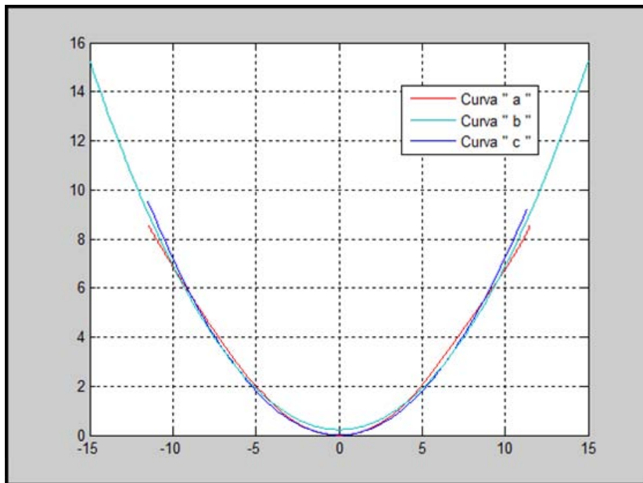
FIGURA 13. CONTORNOS DEL TRANSDUCTOR: a) OBTENIDO MEDIANTE DIGITALIZACION DE FOTOGRAFIA b) OBTENIDO MEDIANTE COMANDO POR DEFECTO DE MATLAB OBTENIDO MEDIANTE UN PROGRAMA DE MATLAB
