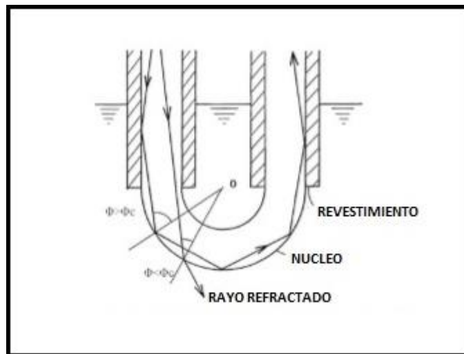
Figura 4.3. SENSOR REFRACTOMÉTRICO DE FIBRA ÓPTICA EN FORMA DE "U"
