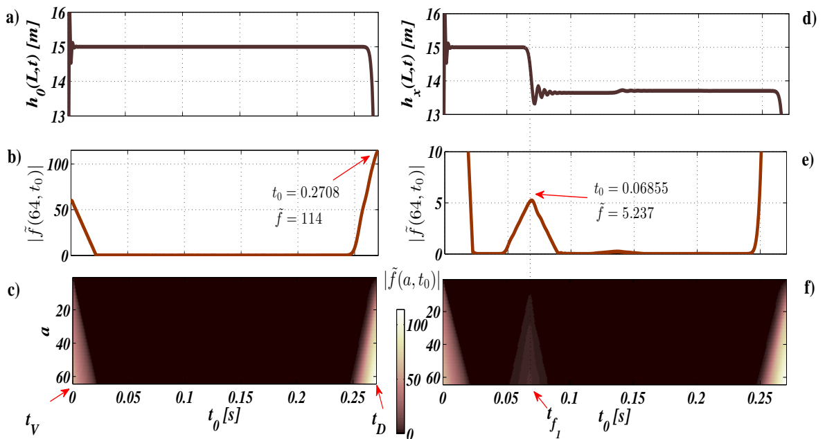
Figura 4.7: Comparación de TO aplicada a la onda de presión en condiciones normales y en presencia de fuga, a) onda de presión h_0(L, t) , obtenida mediante simulación, en condiciones normales, en el intervalo (0, 0.2688) [s] b) gráfica del valor absoluto de TO con una onduleta madre Haar y una escala a = 64 aplicada a h_0(L, t) c) TO de la onda de presión sin fuga con escalas de 0 \leq a \leq 64 , d) onda de presión h_x(L, t) , obtenida mediante simulación, en presencia de fuga 25% del gasto nominal en el intervalo (0, 0.2688) [s], e) gráfica del valor absoluto de TO con una escala a = 64 aplicada a h_x(L, t) , f) TO de la onda de presión en presencia de fuga con escalas de 0 \leq a \leq 64 .
