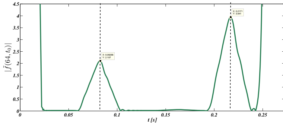
Figura 4.15: TO con un escalamiento de a = 64 y un corrimiento 0 \leq t_0 \leq t_D = 0.2708 [s], aplicada a la presión en el extremo del ducto con fricción y con dos fugas presentes. La primera del 10% la magnitud del flujo de salida y ubicada a 60 [m] de la válvula; la segunda, del 20% y a 160 [m].
