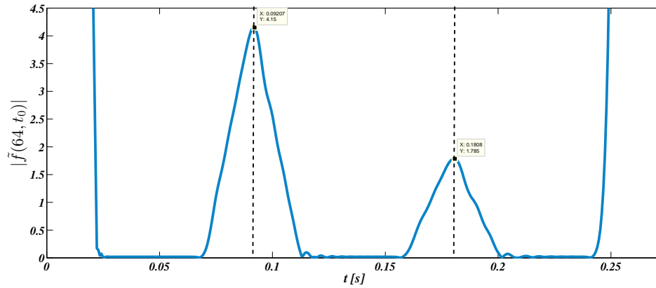
Figura 4.13: TO con un escalamiento de a = 64 y un corrimiento 0 \leq t_0 \leq t_D = 0.2708 [s], aplicada a la presión en el extremo del ducto con fricción y con dos fugas presentes. La primera del 10% la magnitud del flujo de salida y ubicada a 66.67 [m] de la válvula; la segunda, del 20% y a 133.33 [m].
