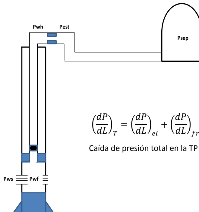
Fig. 1.8 Pozouyente necesario para tener flujo multifasico vertical
