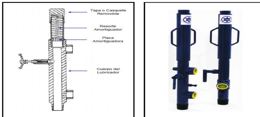
Fig. 2.12 Partes internas y externas típicas de un lubricador
