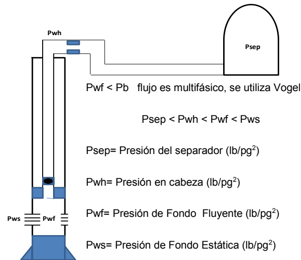
Fig. 1.1 Esquema pozo Fluuyente
