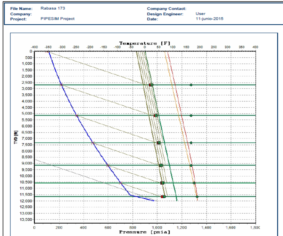
Fig. 5.10 Espaciamiento de Válvulas de BNC programa PIPESIM
