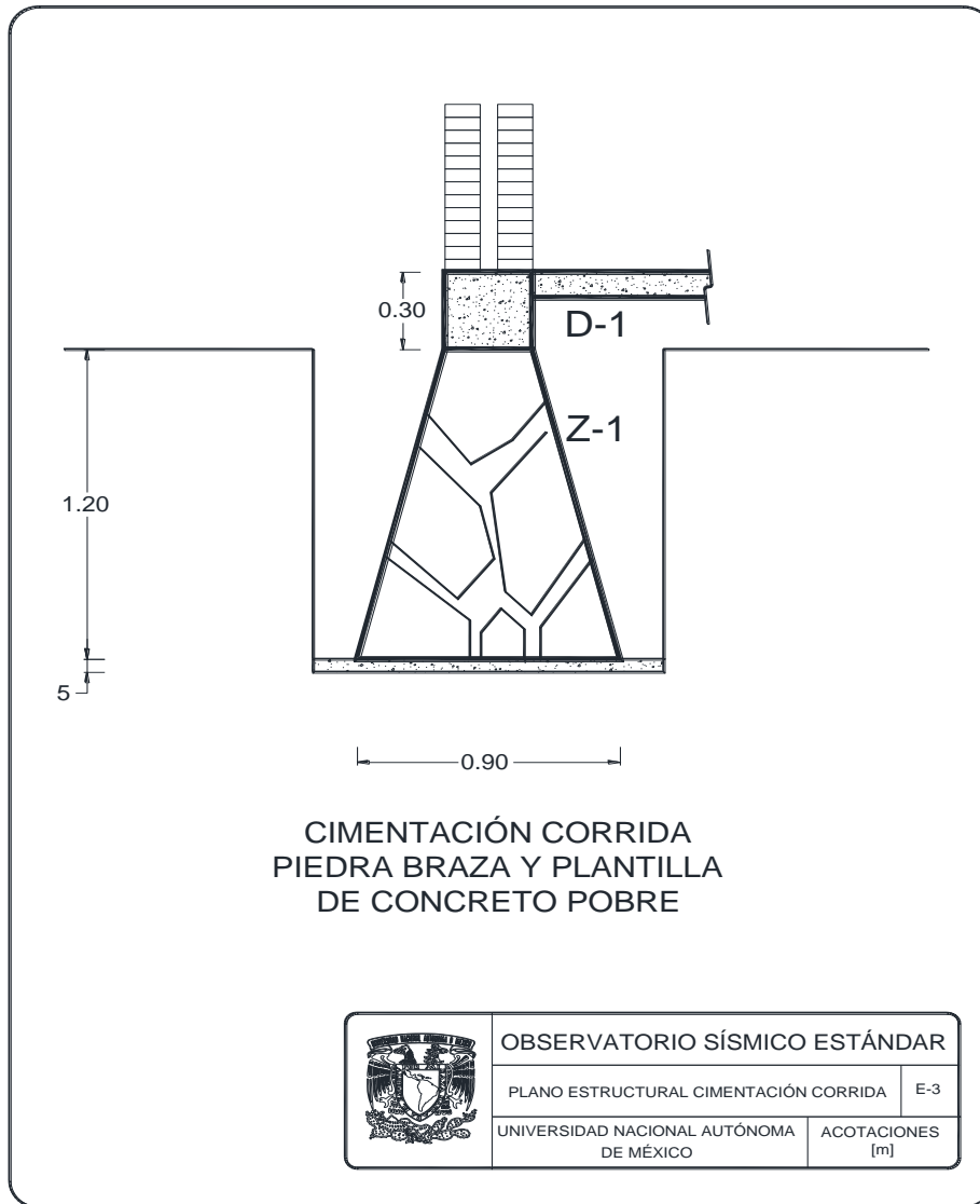
Figura 3.2 Cimentación corrida
