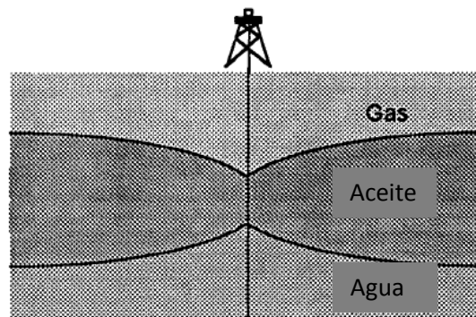
Figura 34. Contactos del acuñamiento de gas/aceite y aceite/agua, en un pozo productor (modificada de Ander et al, 1997).
