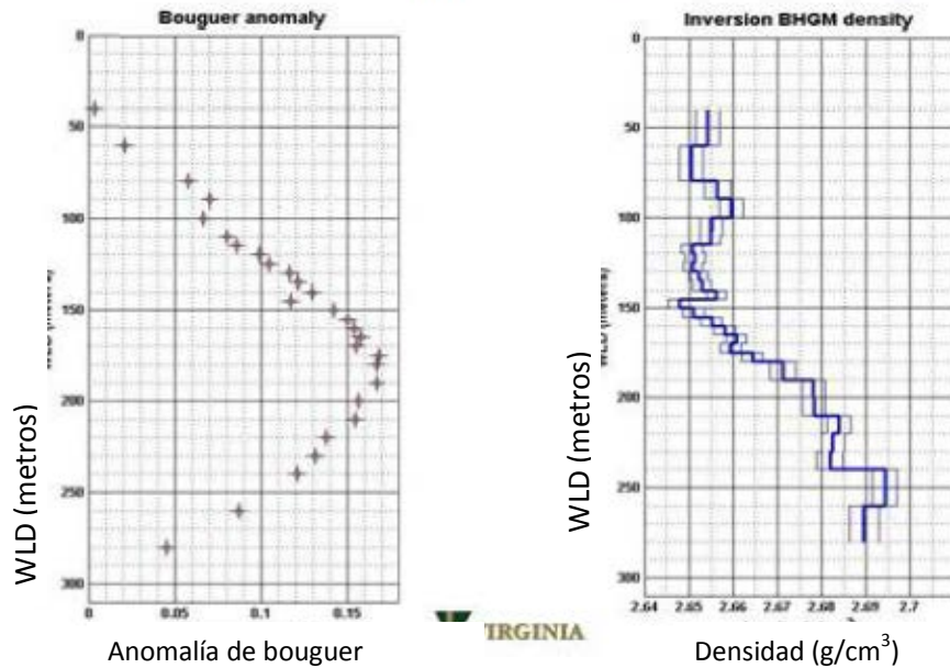
Figura 41. Mediciones de gravimetría de pozo y densidad aparente medidas en el pozo CN-08-128 en un yacimiento de la mina de Virginia. El pozo no se extiende lo suficiente por debajo del depósito, para medir de manera completa la anomalía de gravedad (modificada de Nind et al, 2013).
