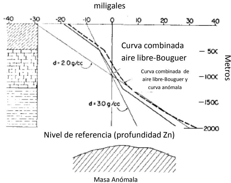
Figura 15. Curvas combinadas de aire libre, Bouguer y masa anómala. La escala de gravedad ha sido duplicada con respecto a las figuras previas y con referencia a g_0 que se desplaza a la izquierda. También muestra las curvas de Bouguer y aire libre para la densidad promedio de la formación con un valor de 2.0 y 3.0 \text{gr/cm}^3 (modificada de Smith, 1950).
