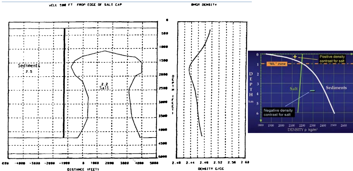
Figura 32. (Izquierda) efecto en la densidad medida con el gravímetro de pozo debida a un domo salino (Smolen, 1996, cortesía de Edcon), (derecha) variación típica de densidad contra profundidad para sedimentos y sal (Saad, 2006).
