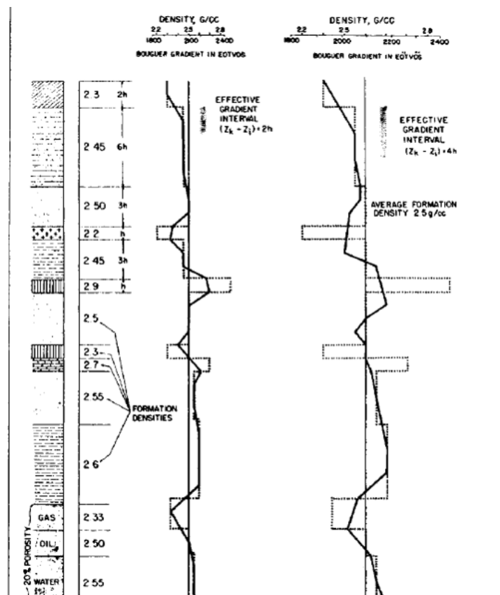
Figura 25. Densidad obtenida mediante mediciones de BHGM para dos espaciamientos entre estaciones (modificada de Smith, 1950).
