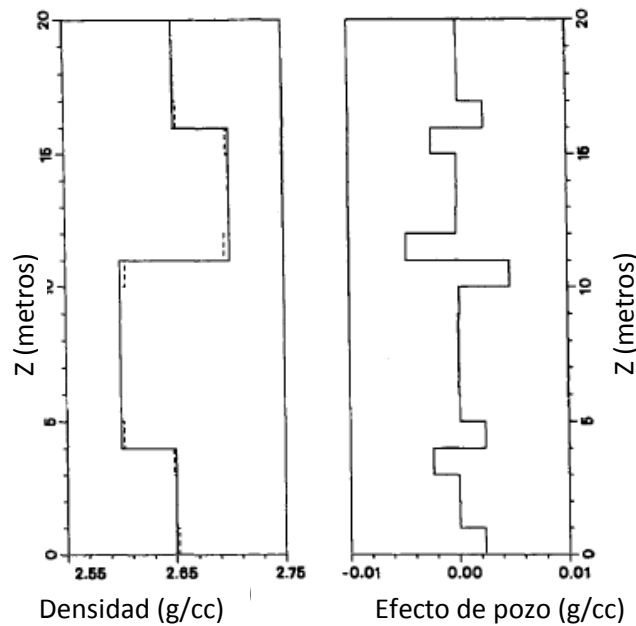
Figura 23. Densidad de la formación (izquierda), densidad aparente (línea discontinua) y efecto de pozo (derecha) para un diámetro de 20cm, espaciamiento de estación igual a 1m y una densidad de lodo de 2.7\text{gr/cm}^3 . El fondo del pozo está en z=0 (modificada de Sezginer, 1991).
