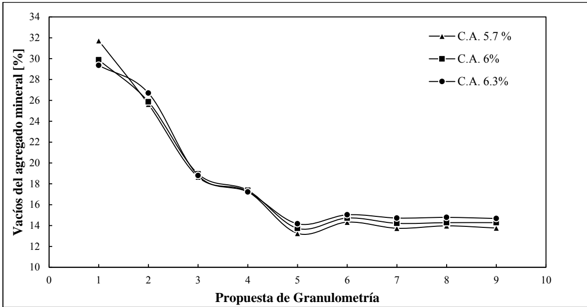
Figura 4.7. Vacíos del agregado mineral
