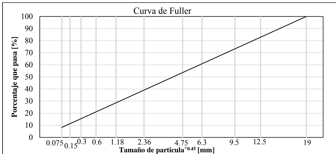
Figura 3.1. Gráfica de la curva de Fuller con n=0.45
