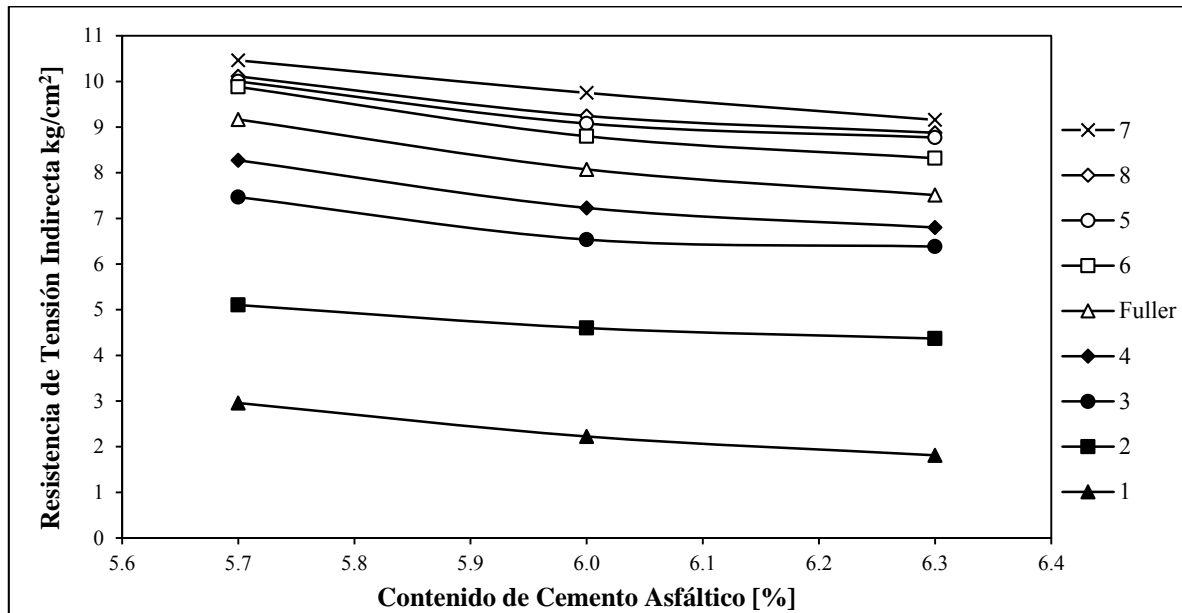
Figura 4.16. Variación del contenido de ligante y la RTI
