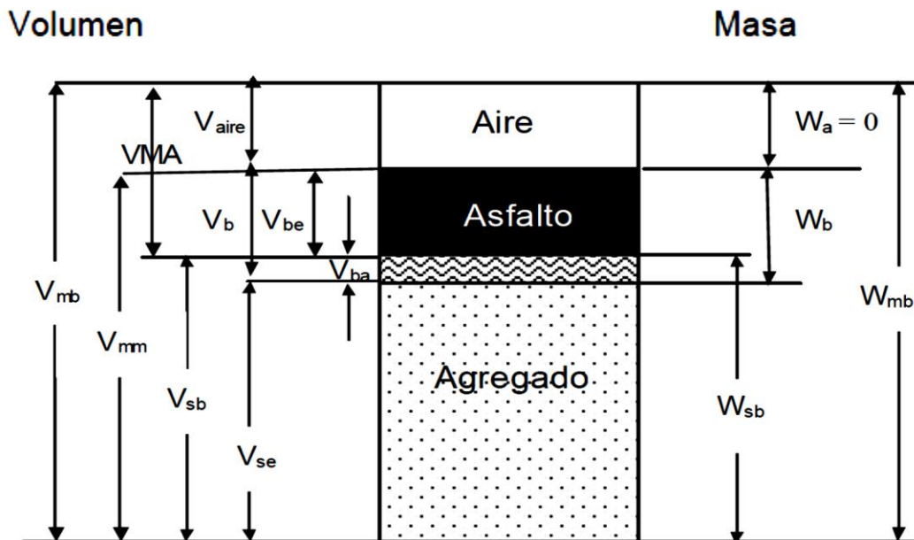
Figura 2.27. Diagrama de fases de una mezcla asfáltica compactada
