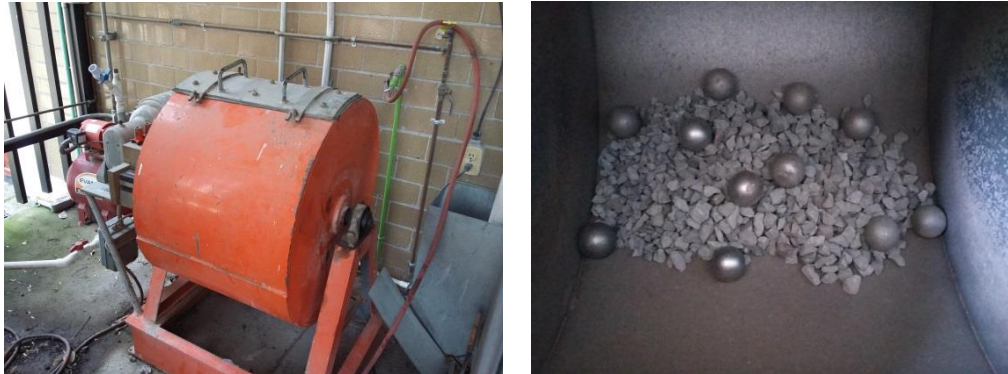
Figura 2.13. Cilindro y esferas para el ensayo de Los Ángeles
