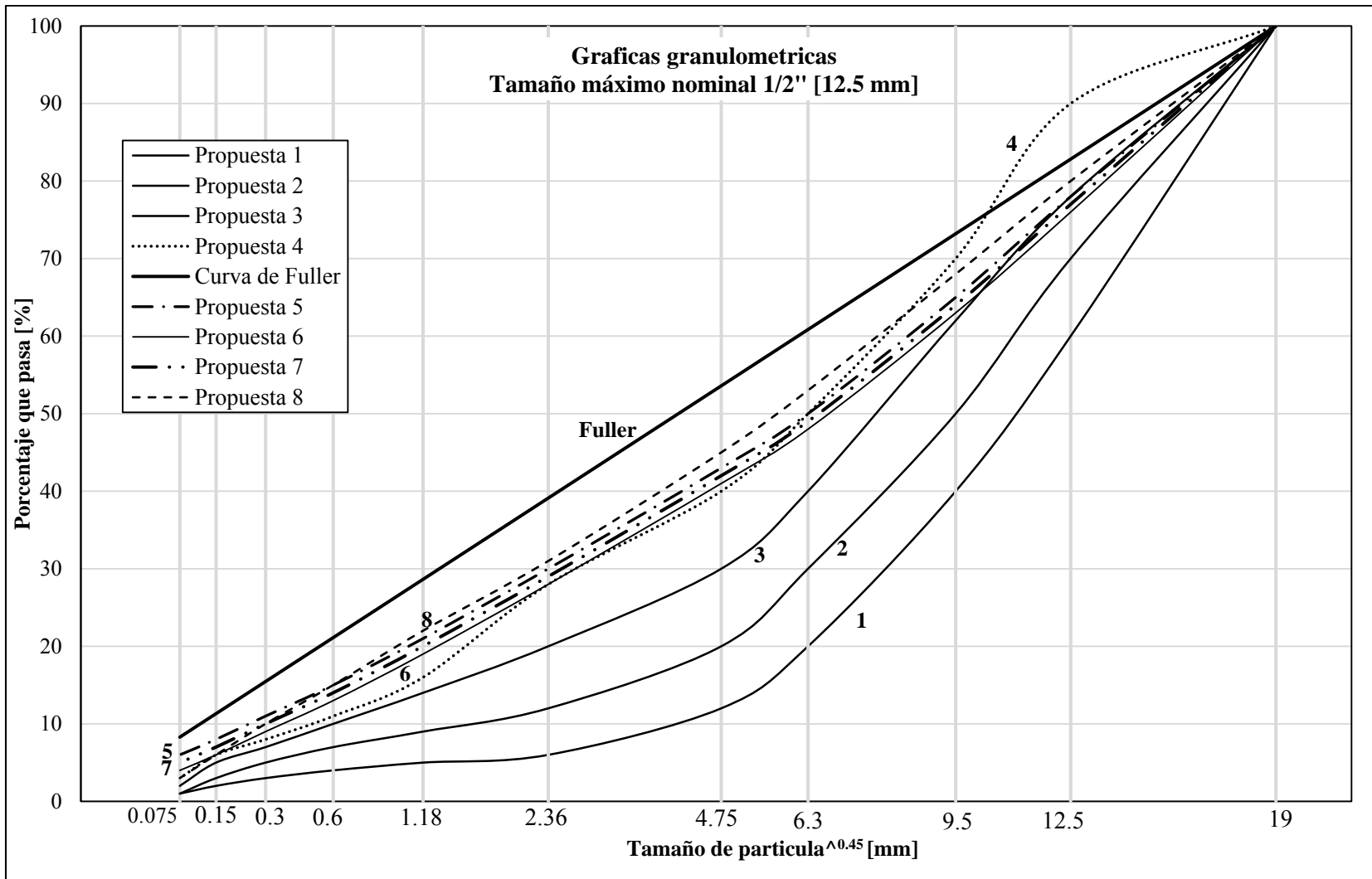
Figura 3.2. Granulometrías propuestas
