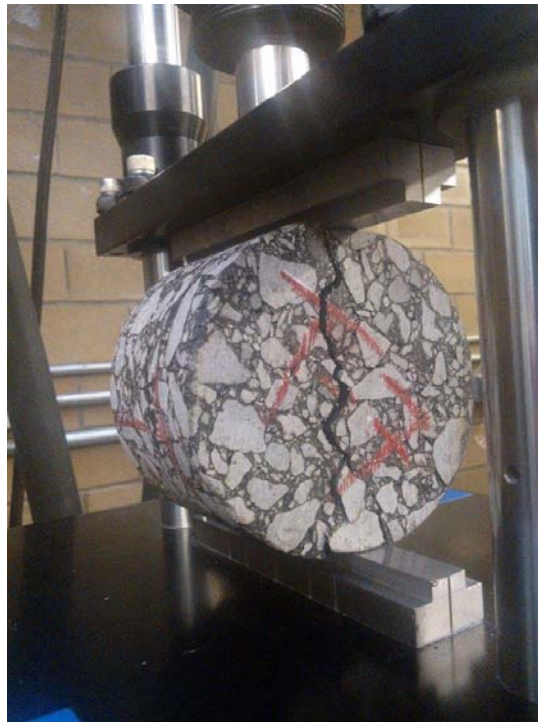
Figura 4.3. Especimen fallado
