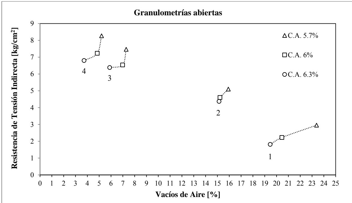
Figura 4.13. Correspondencia de %Va y RTI para granulometrías abiertas
