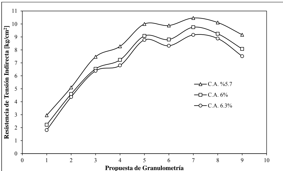
Figura 4.12. Relación entre la tensión indirecta del concreto asfáltico, la granulometría y el contenido de cemento asfáltico
