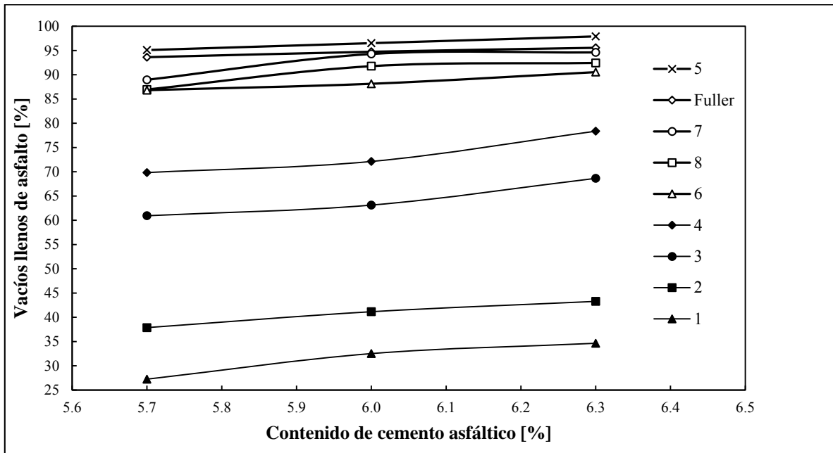
Figura 4.11. Vacíos llenos de asfalto y contenido de cemento asfáltico
