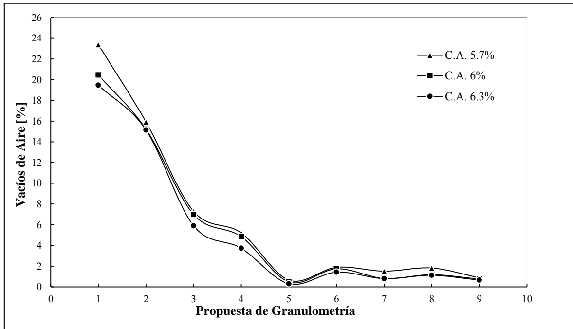
Figura 4.6. Vacíos de aire
