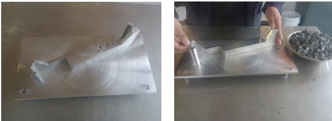
Figura 2.12. Dispositivo para partículas alargadas y planas (Josephia, R., 2015)
