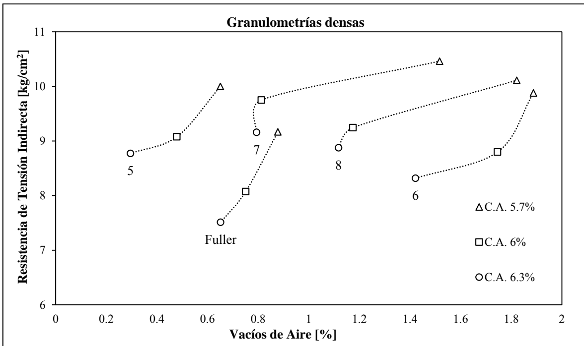
Figura 4.14. Correspondencia de %Va y RTI para granulometrías densas
