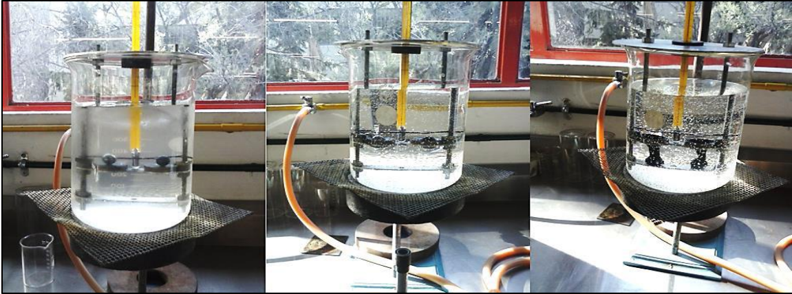
Figura 2.20. Ensayo de punto de reblandecimiento (Martínez, O., 2014)
