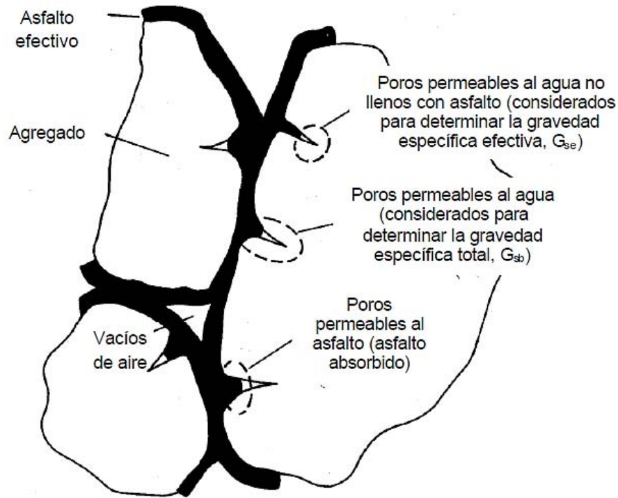
Figura 2.28. Ilustración del volumen de aire, volumen de cemento asfáltico efectivo y volumen de cemento asfáltico absorbido en una mezcla asfáltica compactada
