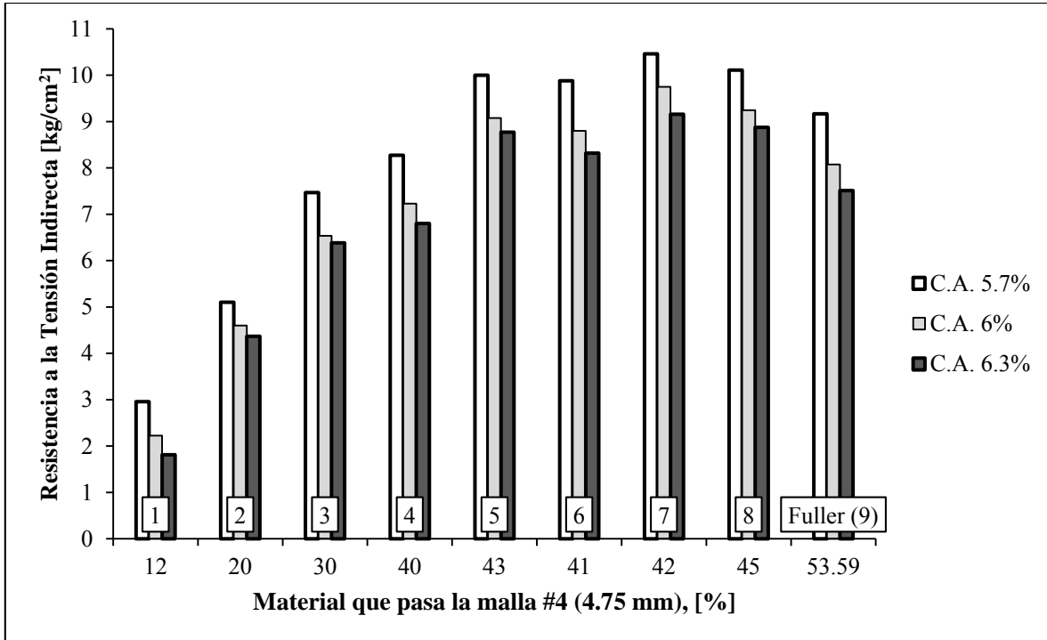
Figura 4.15. Resistencia de Tensión Indirecta y contenido de arena-fino
