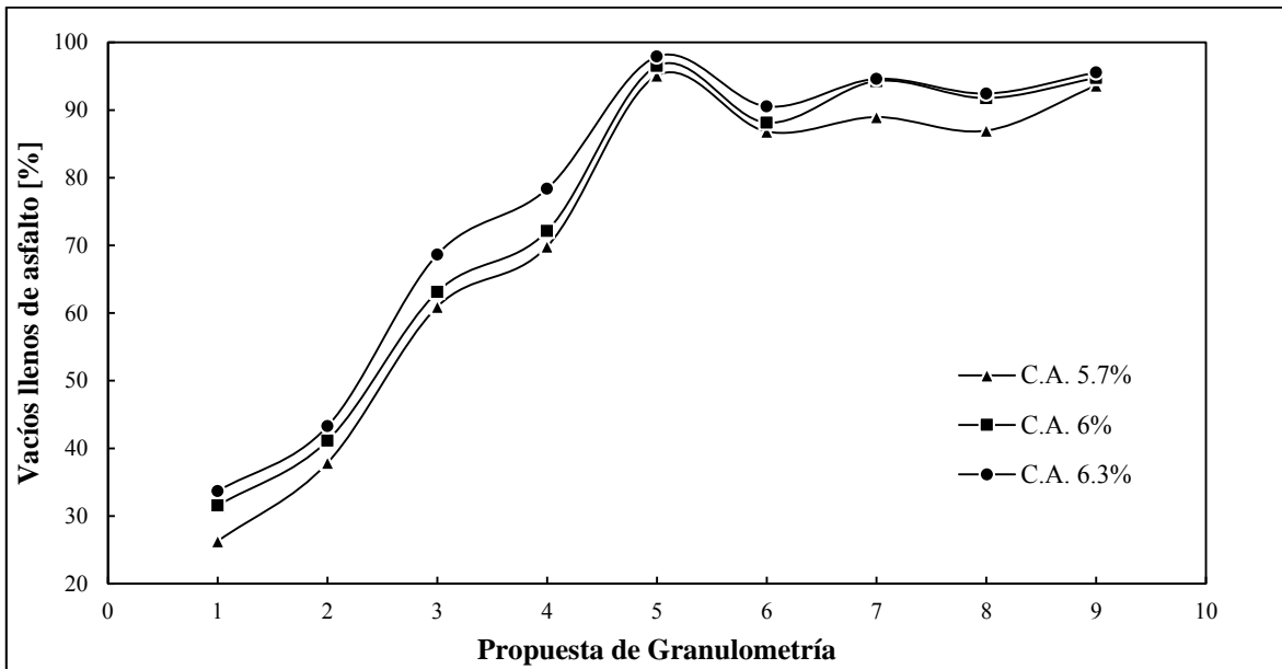
Figura 4.8. Vacíos llenos de asfalto
