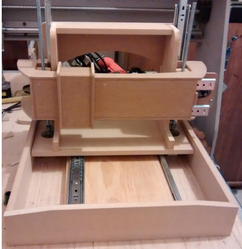
Ilustración 51. Ensamble del carro de Y y la estructura fija del prototipo de Bio-impresora 3D.
