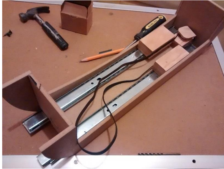
Ilustración 49. Montaje de guías lineales y banda dentada en el carro de Z de la bio-impresora.
