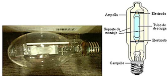
Figura 1-15 Lámpara de haluro metálico
