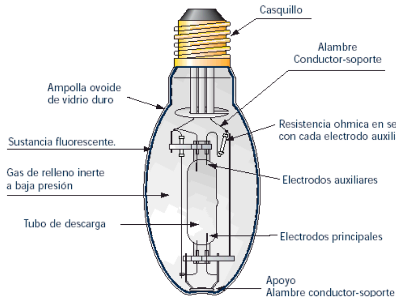
Figura 2.5 Lámpara de vapor de mercurio.
