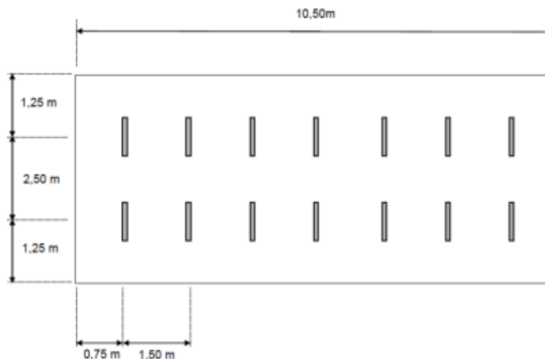
Figura 3.5 Luminarias resultantes
