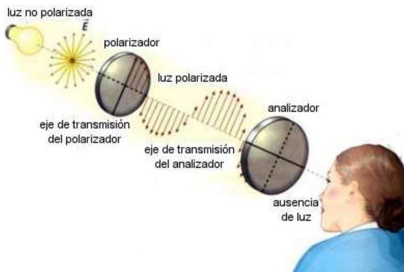
Figura 1.15 Polarización de la luz
