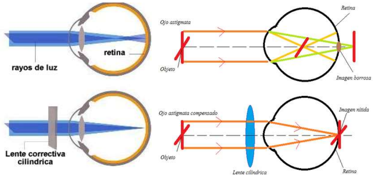
Figura 1.6 Lentes para astigmatismo.
