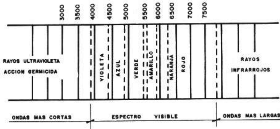
Figura 1.17 Espectro visible para el ojo humano
