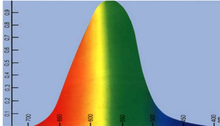
Figura 1.8 sensibilidad del ojo a los colores
