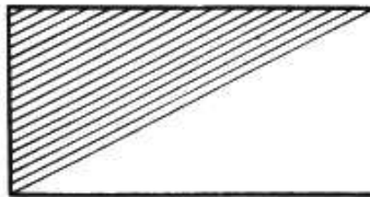
Figura 1.20 Se observa un objeto con contraste.
