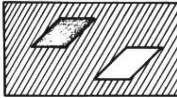
Figura 1.19 Se observan objetos de diferente brillantes.
