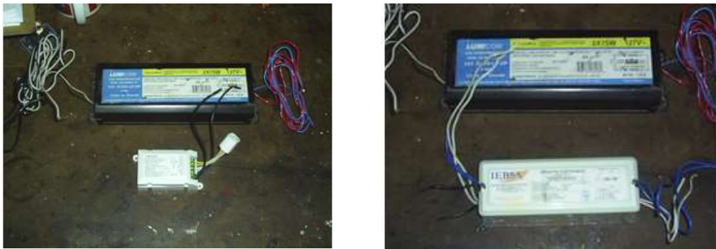
Figura 2.10 Diferencia de tamaño de un balastro electromagnético a un electrónico
