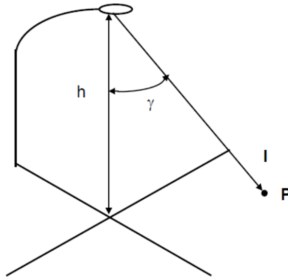
Figura 3.7 Esquema de una columna con artefacto para alumbrado exterior
