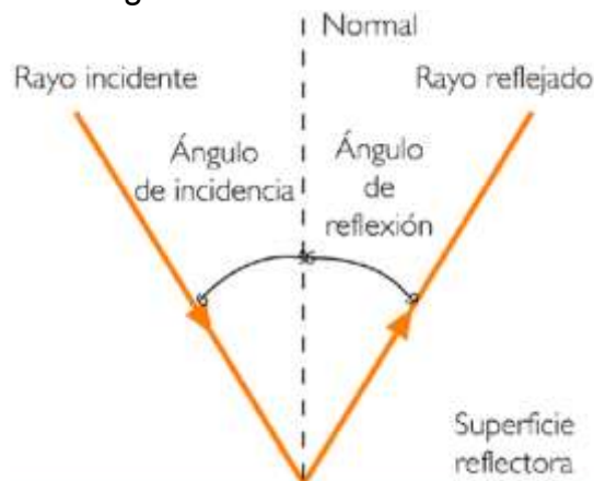
Figura 1.10 Rayo incidente Y rayo reflejado
