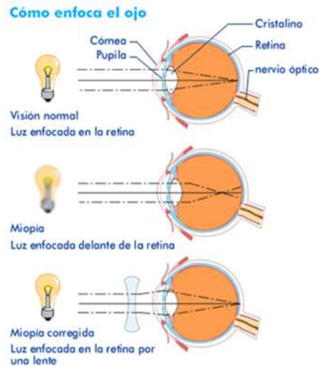
Figura 1.4 Miopía y su corrección
