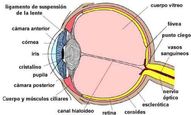
Figura 1.1 Conformado del ojo humano
