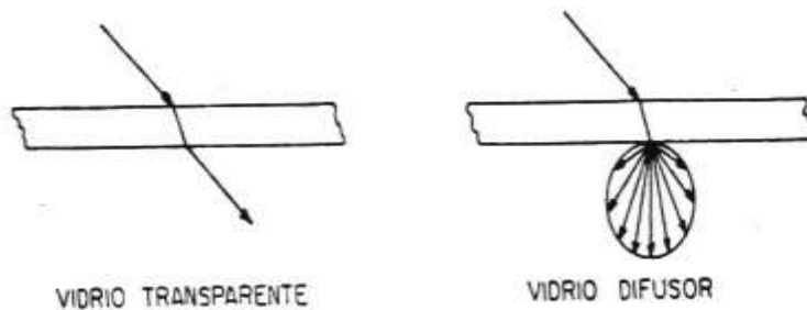
Figura 1.13 Transmisión de la luz.
