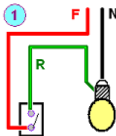
Figura 2.23 Apagador de paso
