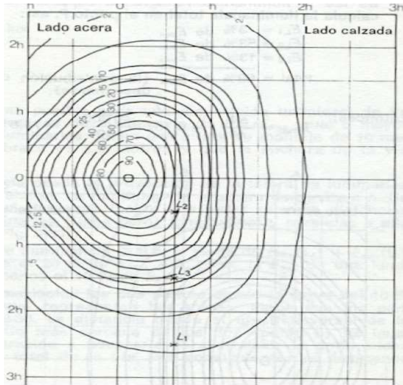
Figura 3.8 Diagrama isolux
