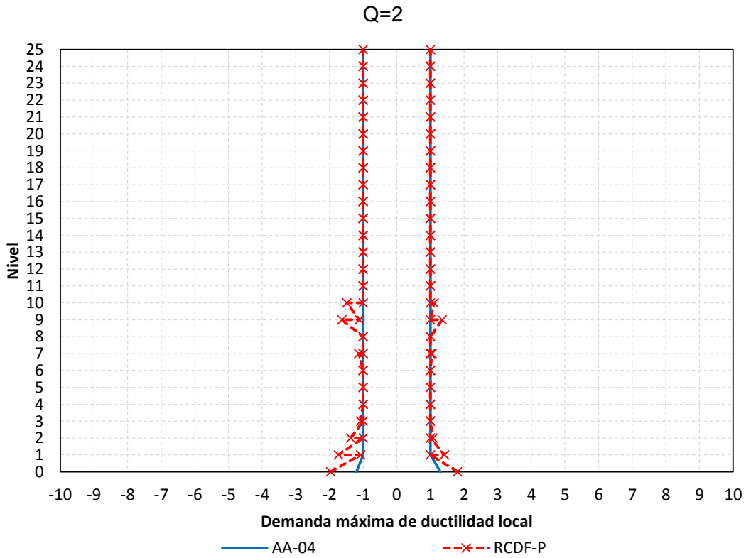
Figura 5.22 Comparación de demandas máximas de ductilidad en columnas de los análisis paso a paso, diseños para Q=2 y 4 con el Apéndice A ( T_s=2 s) de las NTC-Sismo del RCDF-04 y NTC-Sismo ( T_s=2 s) del RCDF-P, edificio de 25 niveles
