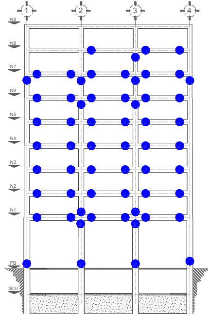
Figura 4.67 Distribución de articulaciones plásticas del análisis estático no lineal ( Push-over ) para la condición de distorsiones máximas permisibles (colapso) de acuerdo al RCDF-P, T_s = 2 s, edificio 9 niveles con Q=4
