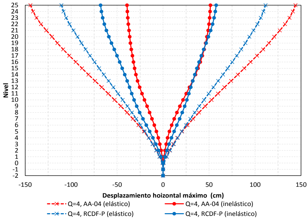
Figura 5.10 Comparación de desplazamientos horizontales máximos de los análisis paso a paso (elástico e inelástico), diseños para Q= 2 y 4 con el Apéndice A ( T_s = 2 s) de las NTC-Sismo del RCDF-04 y NTC-Sismo ( T_s = 2 s) del RCDF-P, edificio de 25 niveles
