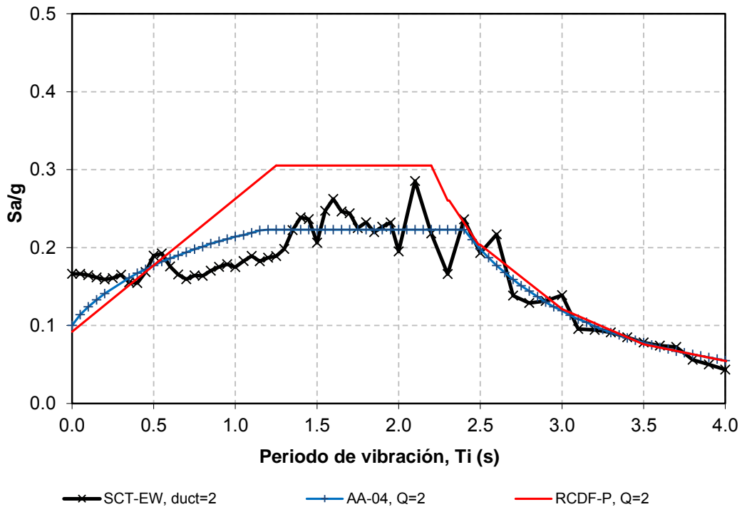
Figura 3.2 Comparación de espectros inelásticos ( Q= 2 ) de diseño del Apéndice A ( T_s= 2 s) de las NTC-Sismo del RCDF-04 y NTC-Sismo del RCDF-P, y espectro de respuesta inelástica ( \mu= 2 ) del acelerograma SCT-EW del sismo de 1985
