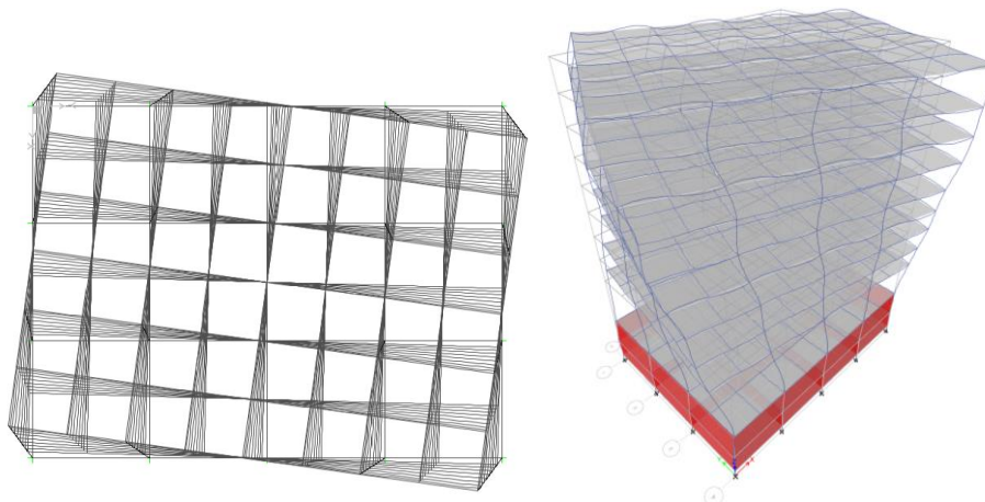
Figura 3.14 Vista en planta y elevación de la deformada del tercer modo de vibrar del edificio de 9 niveles
