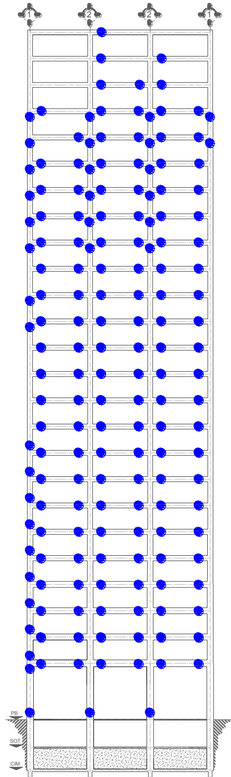
Figura 4.135 Distribución de articulaciones plásticas del análisis estático no lineal ( Push-over ) para la condición de distorsiones máximas permisibles de acuerdo al RCDF-P, T_s = 2 s, edificio 9 niveles con Q=4
