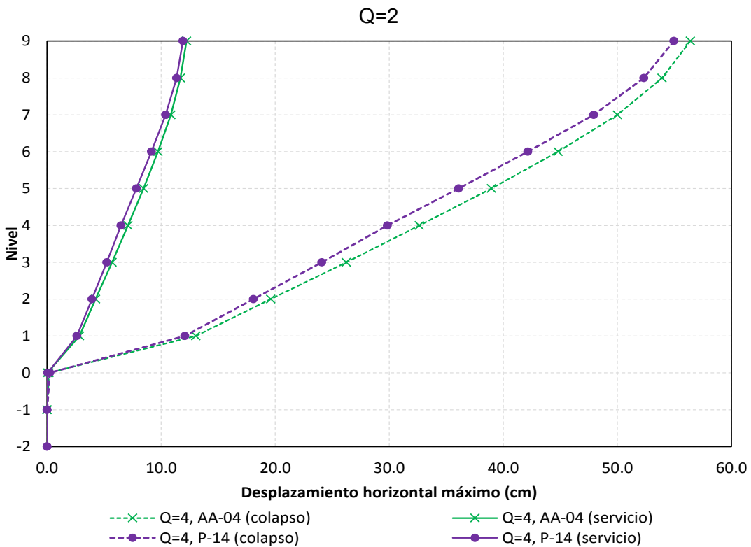
Figura 5.3 Comparación de desplazamientos horizontales máximos de las condiciones de servicio y de colapso, análisis dinámico modal con los espectros de diseño (Q= 2 y 4) del Apéndice A ( T_s= 2 s) de las NTC-Sismo del RCDF-04 y NTC-Sismo ( T_s= 2 s) del RCDF-P, edificio de 9 niveles
