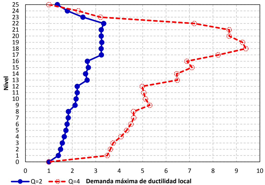
Figura 4.137 Demandas máximas de ductilidad local en vigas del análisis estático no lineal ( Push-over ) para la condición de distorsiones máximas permisibles de acuerdo al RCDF-P, T_s = 2 s, edificio 25 niveles con Q=2 y 4
