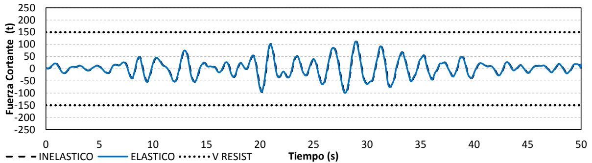
Figura 4.32 Historias de fuerzas cortantes en el extremo inferior de la columna 1 (comportamientos elástico e inelástico), diseño para Q=2 con el Apéndice A de las NTC-Sismo del RCDF-04, edificio de 9 niveles
