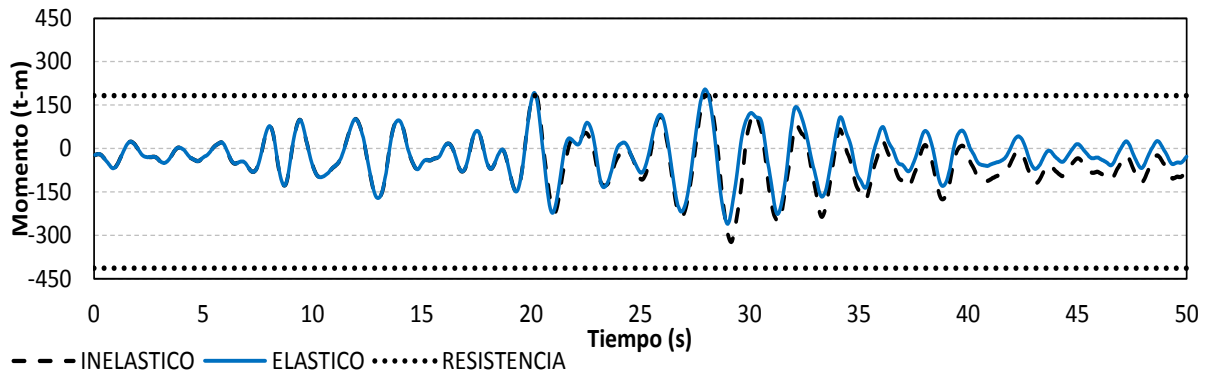
Figura 4.39 Historias de momentos flexionantes en el extremo izquierdo de la viga 1 (comportamientos elástico e inelástico), diseño para Q=4 con las NTC-Sismo de la propuesta RCDF-P, edificio de 9 niveles
