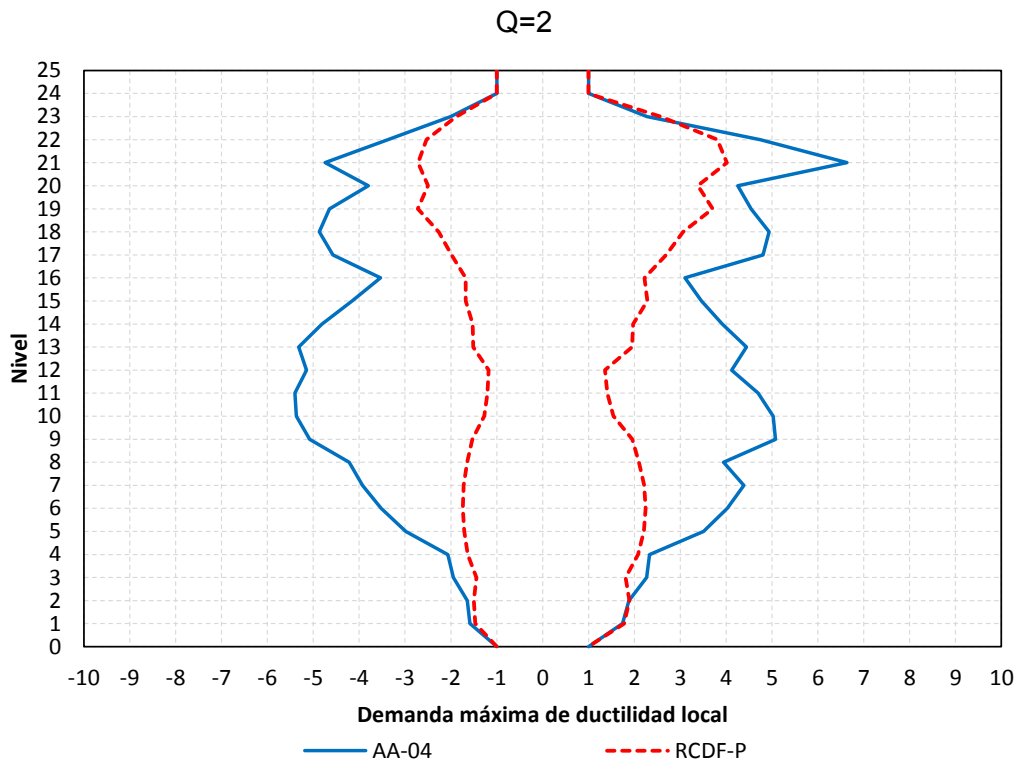
Figura 5.20 Comparación de demandas máximas de ductilidad local en vigas de los análisis paso a paso, diseños para Q=2 y 4 con el Apéndice A ( T_s=2 s) de las NTC-Sismo del RCDF-04 y NTC-Sismo ( T_s=2 s) del RCDF-P, edificio de 25 niveles
