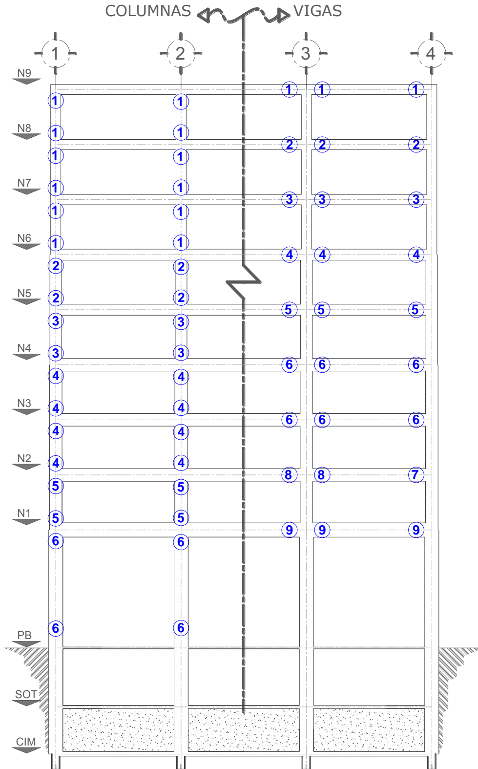
Figura 3.45 Ubicación de los tipos de armados de vigas y columnas del eje C, edificio de 9 niveles, Q=2 , Apéndice A de las NTC-Sismo del RCDF-04
