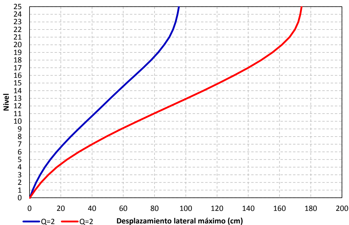
Figura 4.128 Desplazamientos horizontales máximos de los análisis estáticos no-lineales, diseños para Q=2 y 4 con el Apéndice A ( T_s=2 s) de las NTC-Sismo del RCDF-04, edificio 25 niveles
