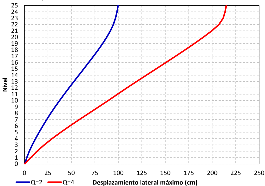
Figura 4.129 Desplazamientos horizontales máximos de los análisis estáticos no-lineales, diseños para Q=2 y 4 con las NTC-Sismo ( T_s=2 s) de la propuesta RCDF-P, edificio 25 niveles
