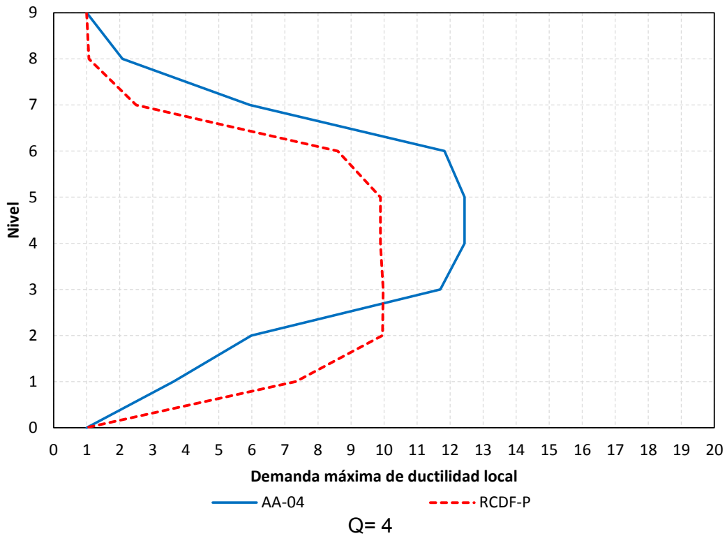
Figura 5.31 Comparación de demandas máximas de ductilidad en vigas, análisis estático no-lineal ( Push-over ), diseños para Q= 2 y 4 con el Apéndice A ( T_s= 2 s) de las NTC-Sismo del RCDF-04 y NTC-Sismo ( T_s= 2 s) del RCDF-P, edificio de 9 niveles
