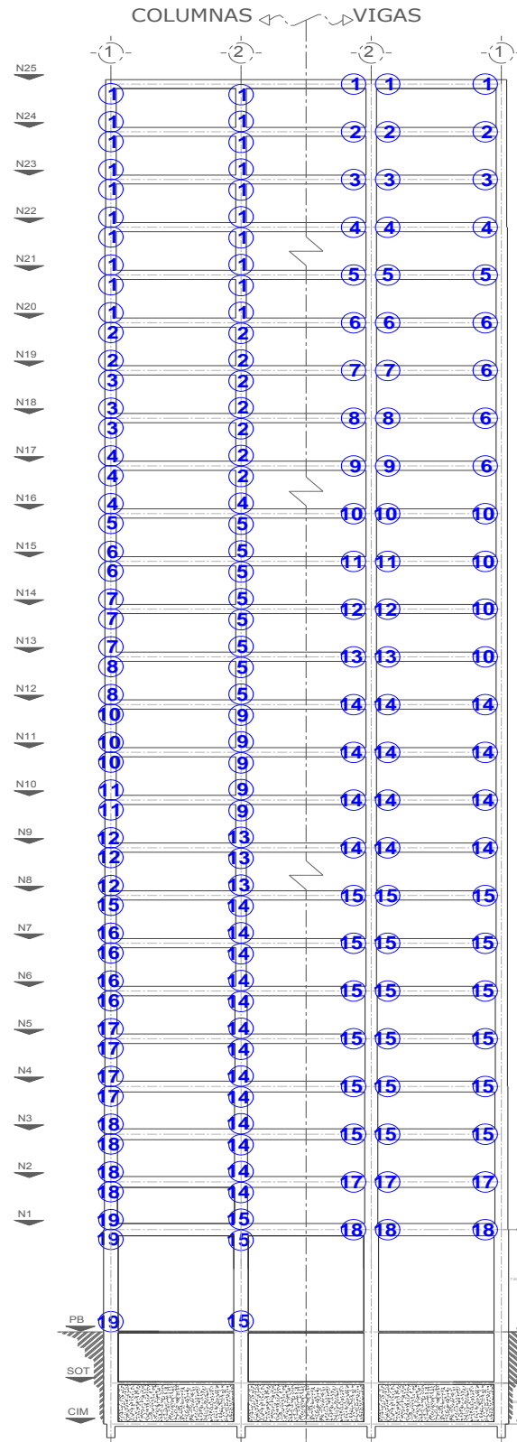
Figura 3.79 Ubicación de los tipos de armados de vigas y columnas del eje C, edificio de 25 niveles, Q= 2, NTC-Sismo del RCDF-04 y NTC-Sismo del RCDF-P
