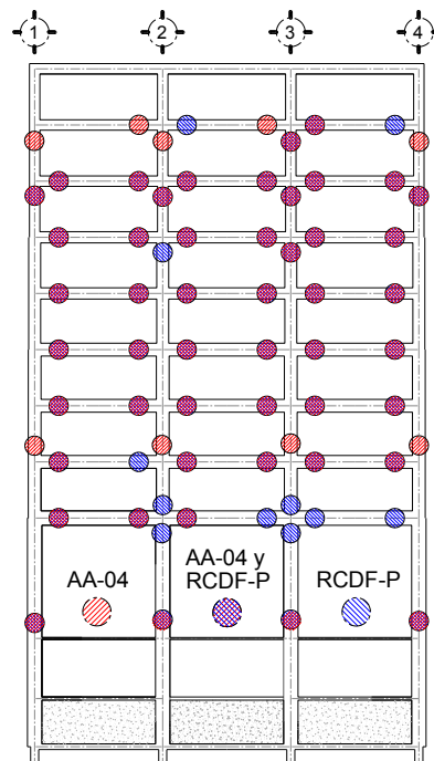
Figura 5.29 Comparación de las distribuciones de articulaciones plásticas, análisis estático no-lineal ( Push-over ), diseños para Q= 2 y 4 con el Apéndice A ( T_s= 2 s) de las NTC-Sismo del RCDF-04 y NTC-Sismo ( T_s= 2 s) del RCDF-P, edificio de 9 niveles
