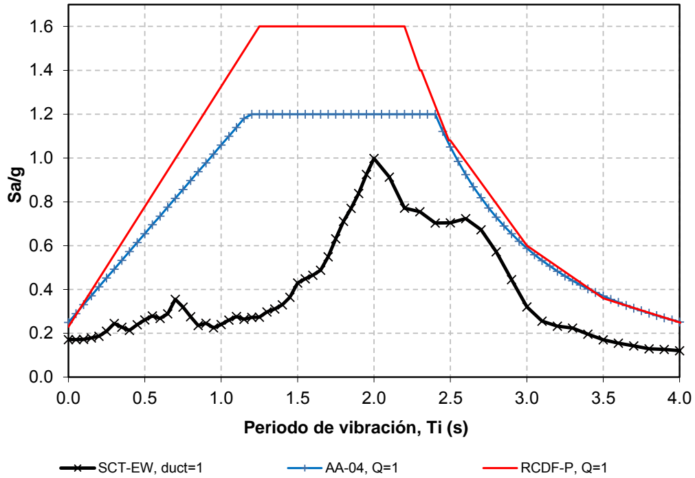
Figura 3.1 Comparación de espectros elásticos de diseño del Apéndice A ( T_s= 2 s) de las NTC-Sismo del RCDF-04 y NTC-Sismo del RCDF-P, y espectro de respuesta elástica del acelerograma SCT-EW del sismo de 1985
