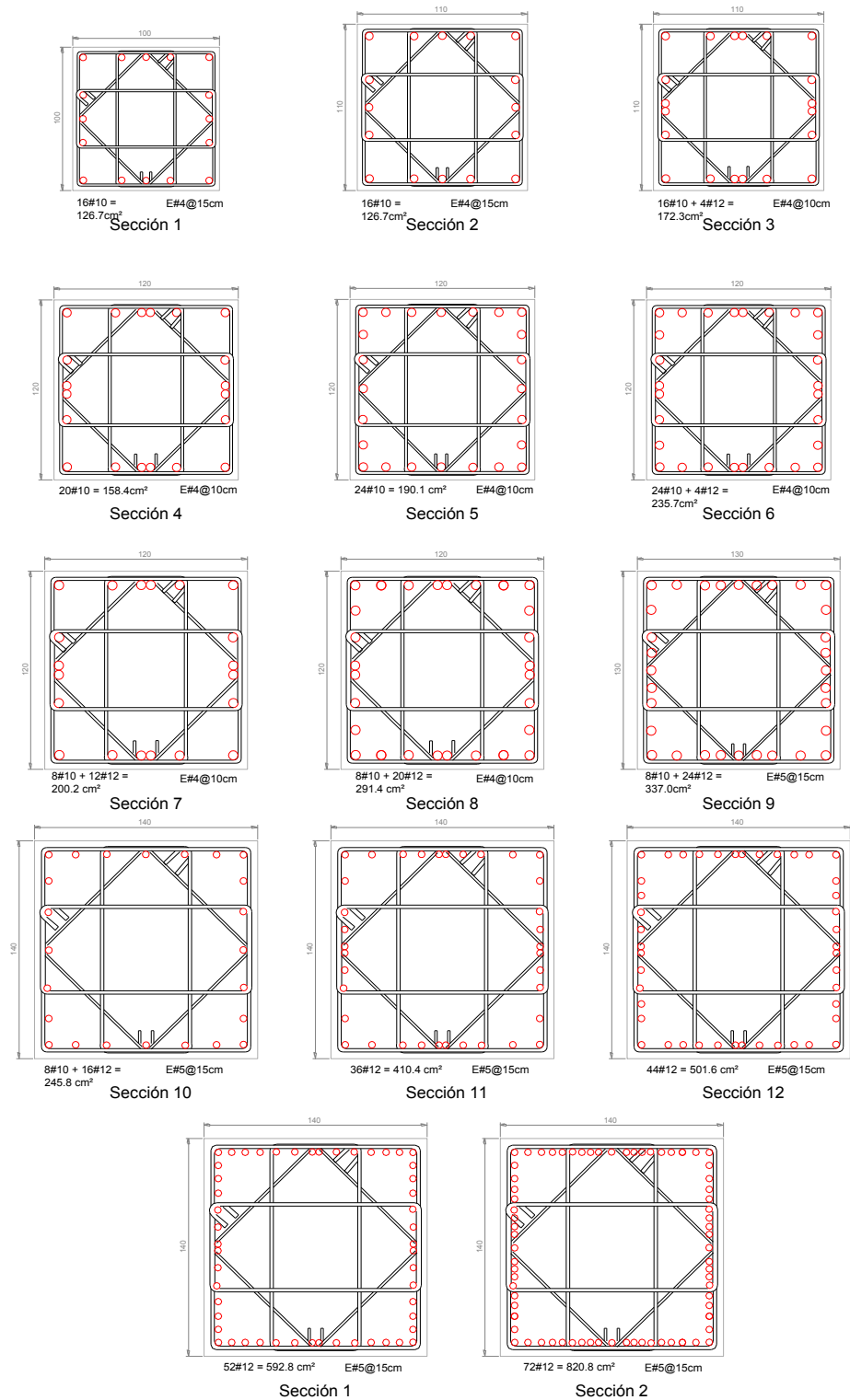
Figura 3.74 Armados longitudinal y transversal propuestos de las columnas del eje C, edificio de 25 niveles, Q= 2, Apéndice A de las NTC-Sismo del RCDF-04
