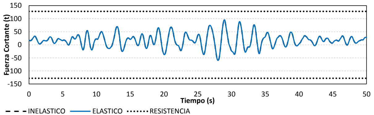
Figura 4.41 Historias de fuerzas cortantes en el extremo izquierdo de la viga 1 (comportamientos elástico e inelástico), diseño para Q=2 con las NTC-Sismo de la propuesta RCDF-P, edificio de 9 niveles
