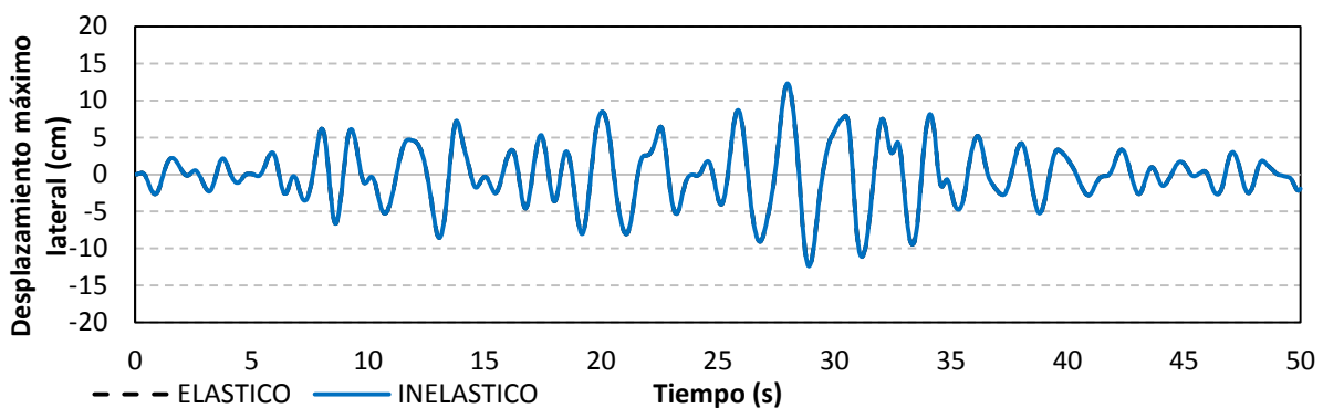
Figura 4.9 Historia de desplazamientos laterales de azotea de los análisis sísmicos paso a paso (elásticos e inelásticos) con el registro SCT-EW-85, diseño para Q=2 con la propuesta de NTC-Sismo ( T_s=2 s) del RCDF-P, edificio de 9 niveles
