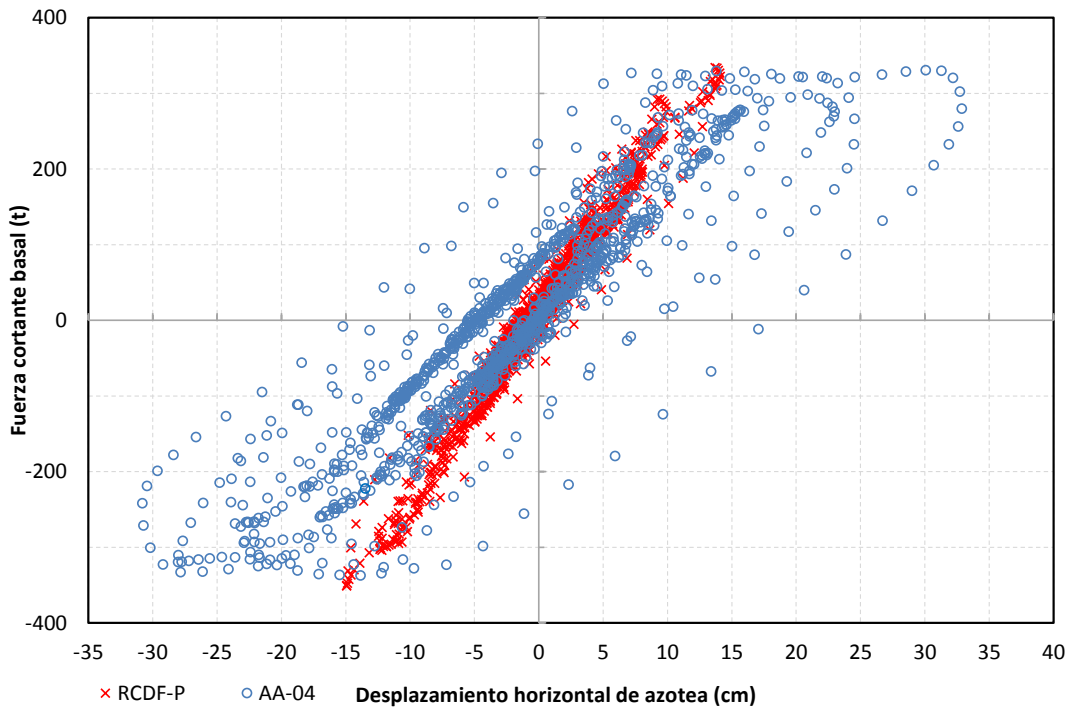
Figura 5.15 Comparación de relaciones fuerza cortante basal-desplazamiento horizontal de azotea de los análisis paso a paso, diseños para Q= 2 y 4 con el Apéndice A ( T_s= 2 s) de las NTC-Sismo del RCDF-04 y NTC-Sismo ( T_s= 2 s) del RCDF-P, edificio de 9 niveles
