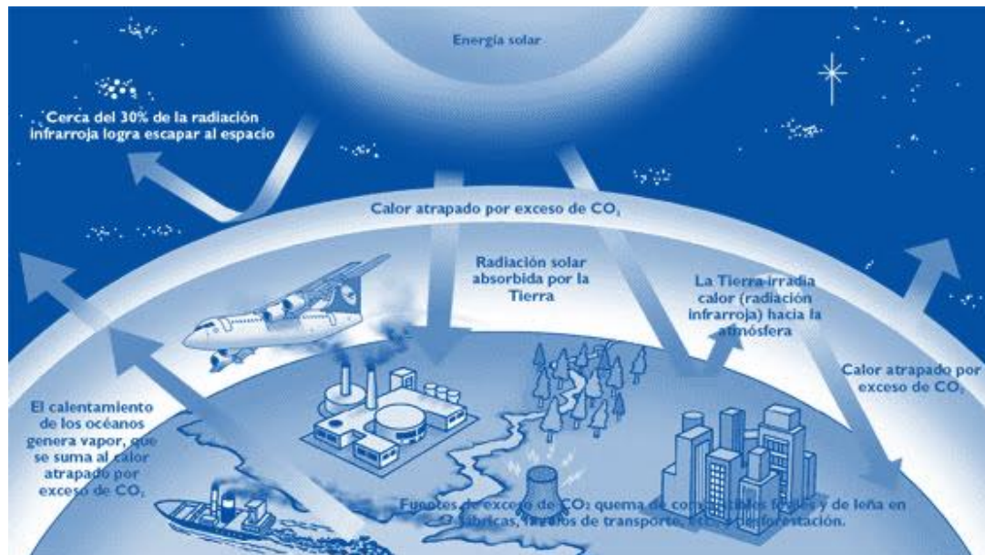
Figura 12. Principales interacciones de la atmósfera con la radiación electromagnética. (ITC, 2004).
