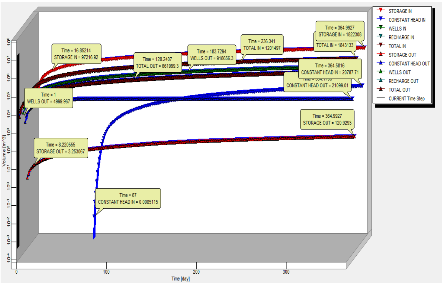
Fig.102 Variaciones de volumen para un año
