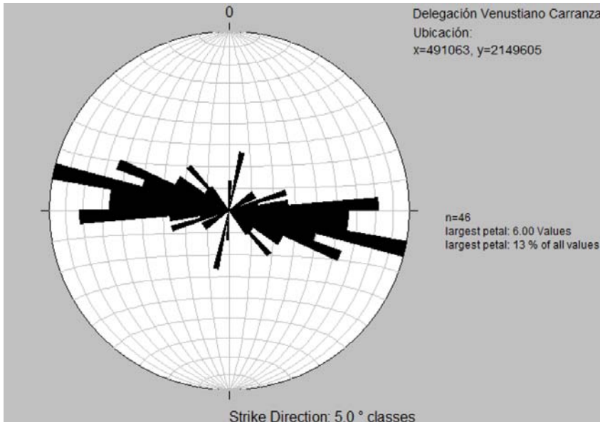
Fig. 39. Roseta de rumbos de fracturas medidas en el afloramiento del Peñon de los Baños. (Palma, 2012)
