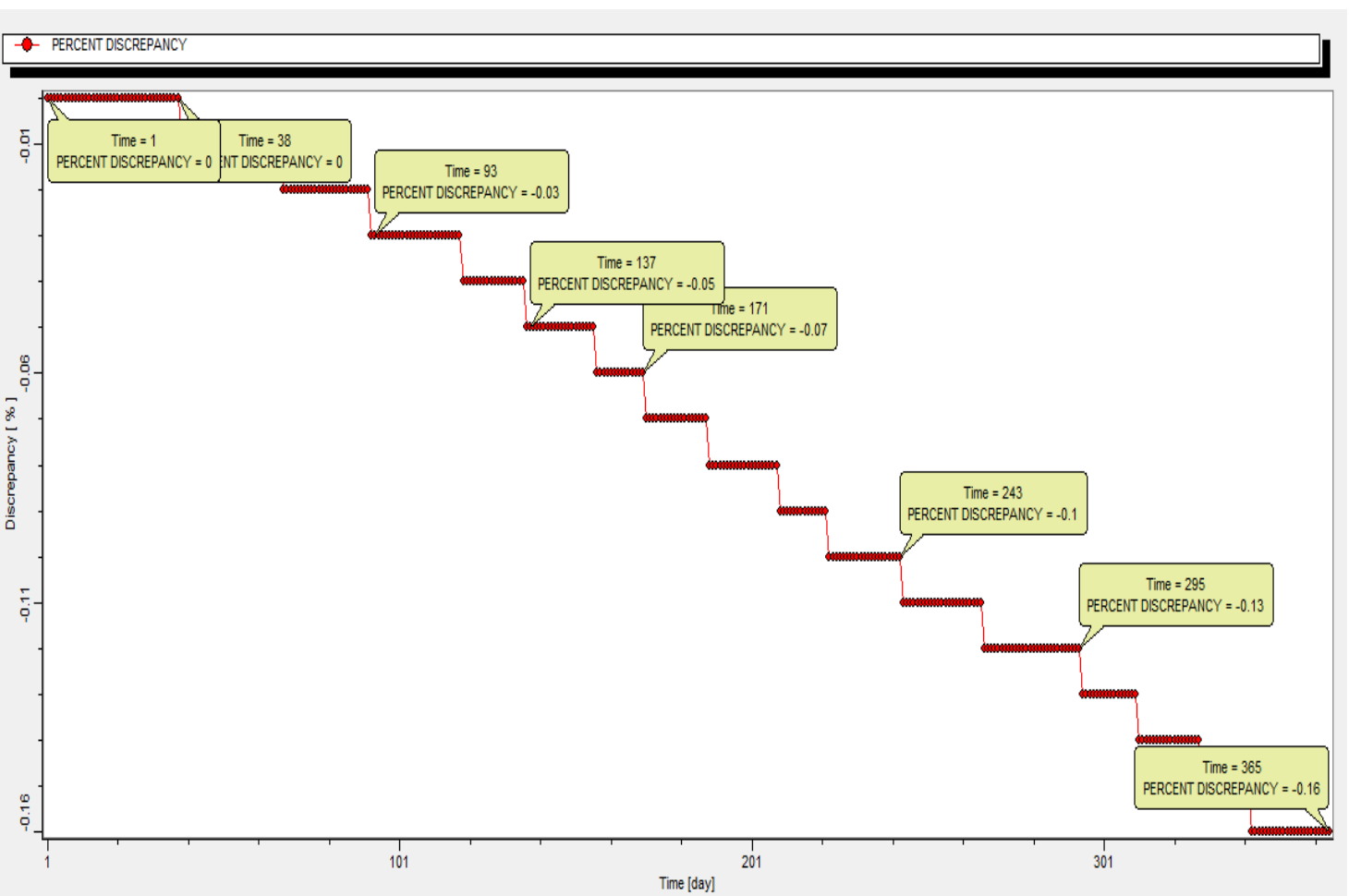
Fig.100 Porcentaje de error por día
