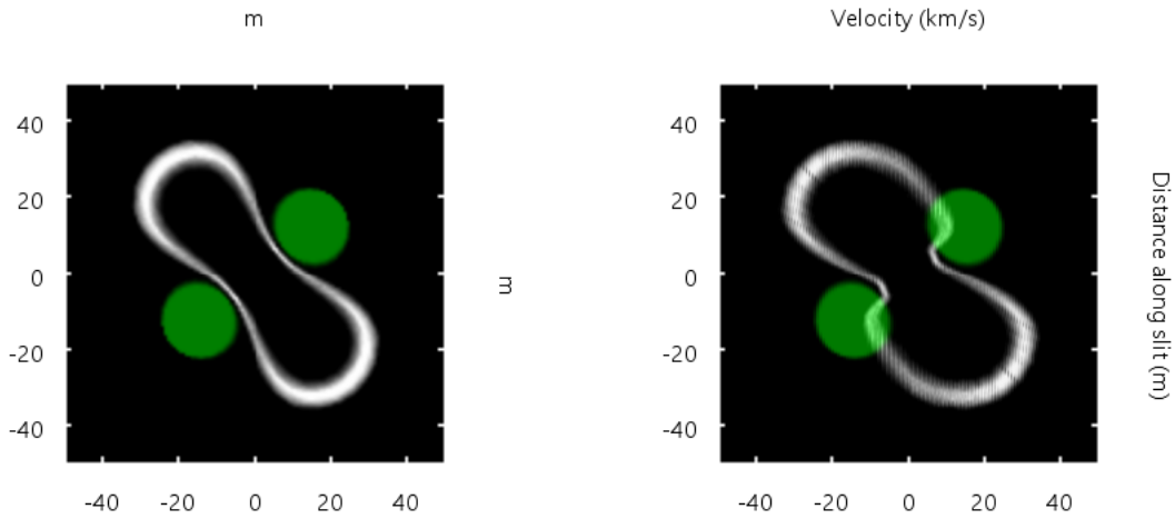
(a) Imagen directa del modelo de la figura 6.2a. (b) Diagrama PV del modelo de la figura 6.2a.
