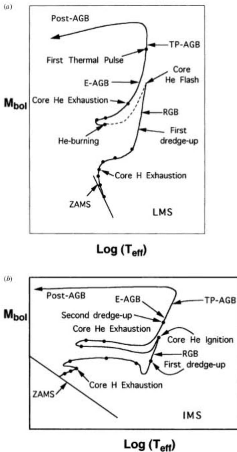
Figura 2.1: Evolución en el diagrama H-R para una estrella (a) de 1 M_{\odot} y (b) de 5 M_{\odot} . Adaptado de [8].
