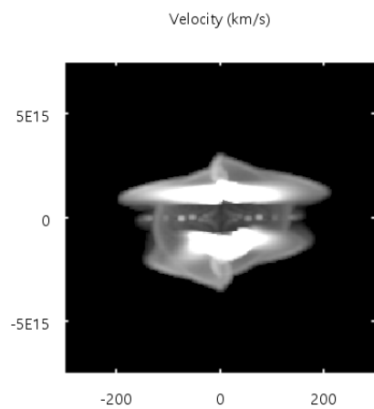
(c) Diagrama PV de la nebulosa de la figura 8.1a.
