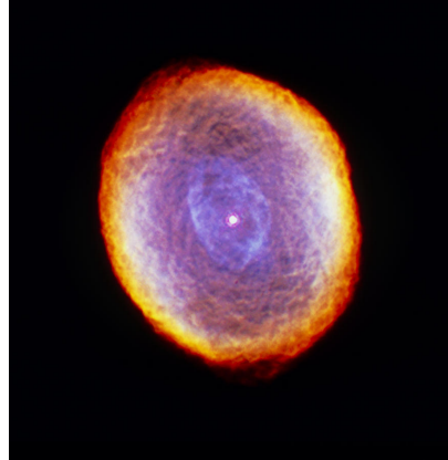
(b) Nebulosa elíptica IC418.
