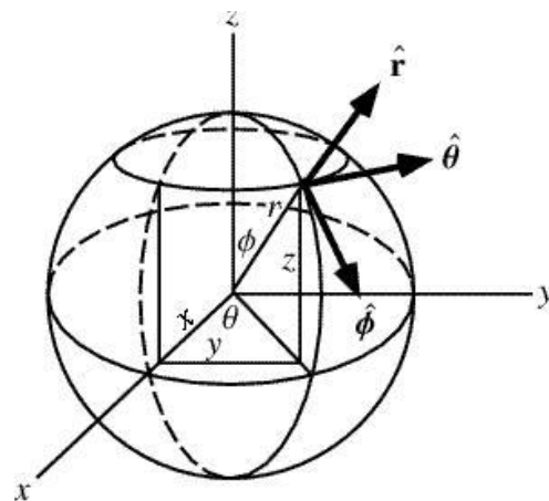
Figura 6.6: Sistema de coordenadas esférico. La dirección radial está representada por el vector unitario \hat{r} y la dirección poloidal por el vector \hat{\phi} .
