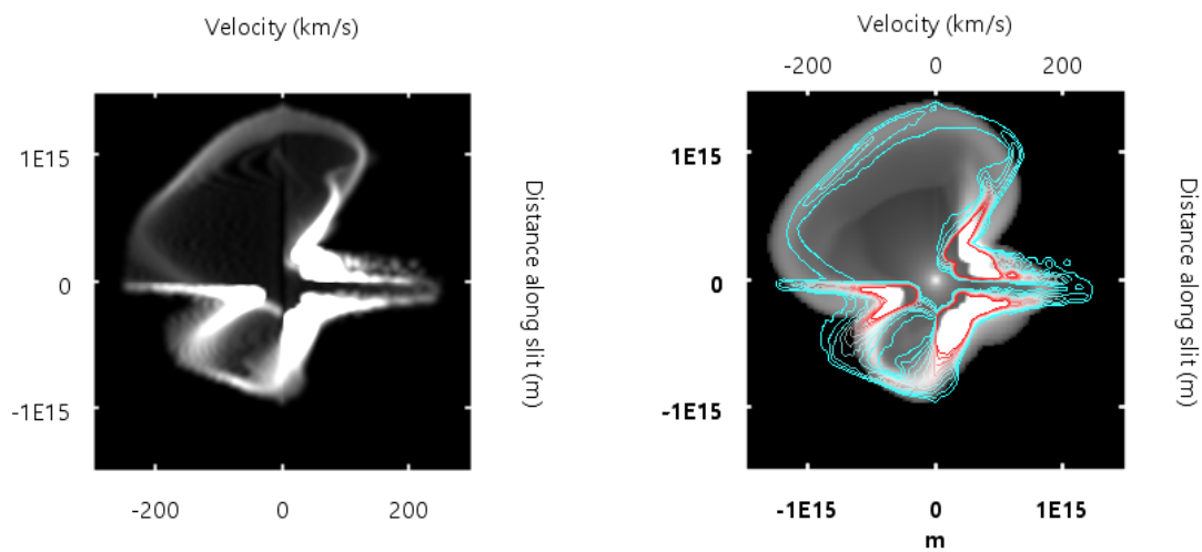
(c) Diagrama PV de la nebulosa de la figura 8.8a.
