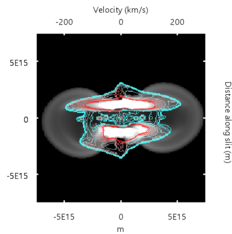
(d) Combinación del corte transversal (representado en escala de grises) de la figura 8.1b y del diagrama PV (simbolizado por los contornos) de la figura 8.1c.
