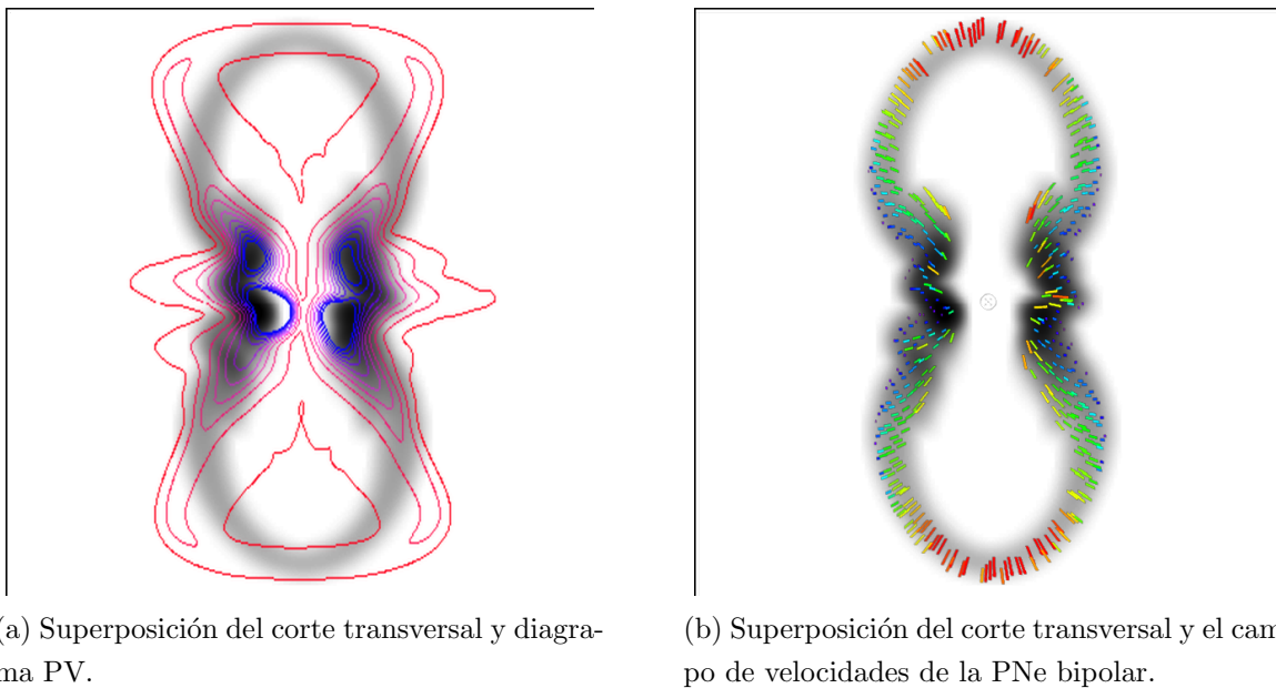
Figura 8.6: Superposición del corte transversal con el diagrama PV y con el campo de velocidades de la PNe bipolar.
