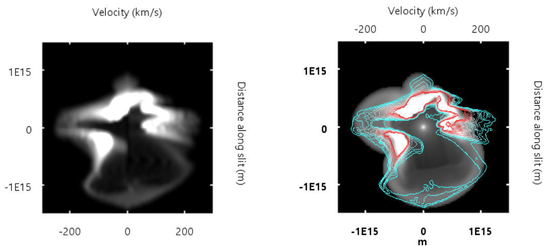
(c) Diagrama PV de la nebulosa de la figura 8.7a.
