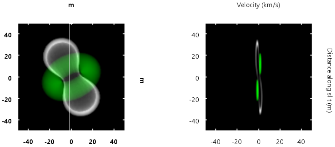
(a) Modelo geométrico generado con el módulo 3D de SHAPE .
