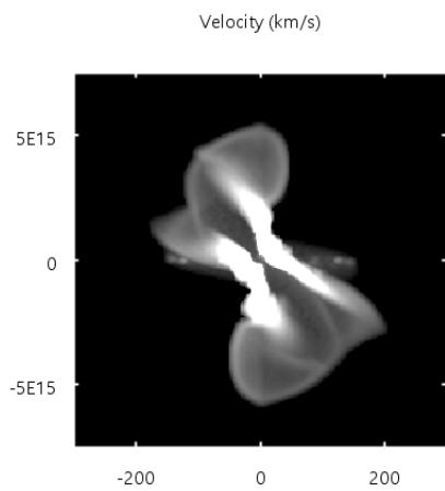
(c) Diagrama PV de la nebulosa de la figura 8.3a.
