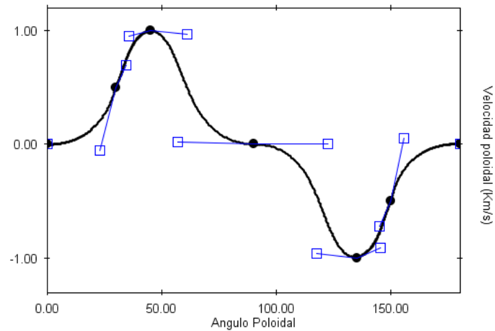
Figura 6.5: Representación gráfica de la velocidad poloidal como función del ángulo poloidal \theta . La forma de la curva se ha generado de forma interactiva. \theta = 90 corresponde al ecuador, \theta = 0 y \theta = 180 corresponde a los polos. La velocidad está normalizada al valor máximo V_{max} = 10km/s .
