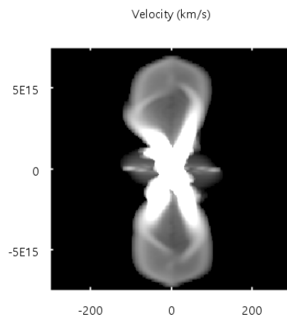
(c) Diagrama PV de la nebulosa de la figura 8.2a.
