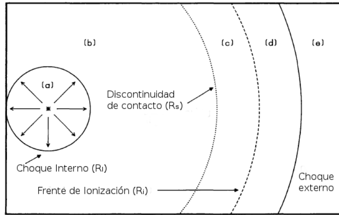
Figura 3.1: Diagrama del modelo de vientos estelares interactuantes (ISW). Las regiones del modelo son: (a) Viento rápido no chocado. (b) Viento rápido chocado ó burbuja caliente. (c) Fracción ionizada de la cáscara. (d) Fracción neutra de la cáscara. (e) Viento AGB no perturbado. Figura adaptada de [93].
