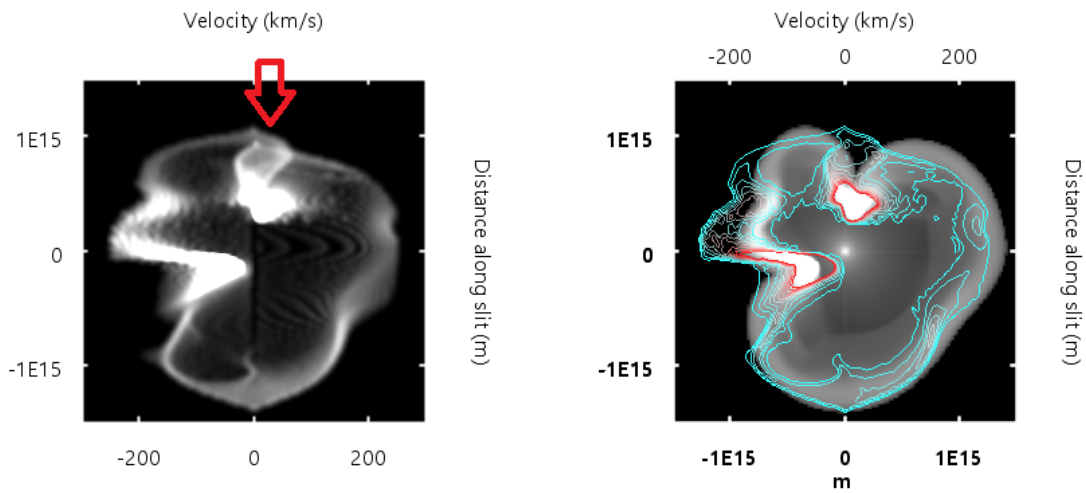
(c) Diagrama PV de la nebulosa de la figura 8.9a.
