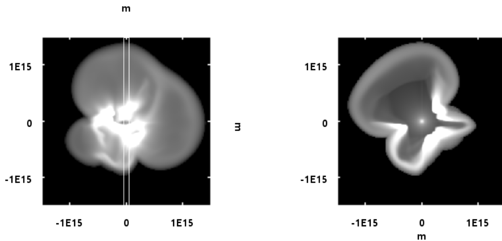
(a) Modelo hidrodinámico tridimensional. La posición de la rendija es señalada por las dos líneas verticales.
