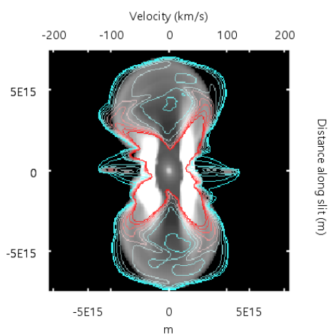
(d) Combinación del corte transversal de la figura 8.2b y del diagrama PV de la figura 8.2c.
