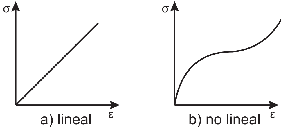
Figura 2.4: Estas curvas representan la respuesta de esfuerzo-deformación en un ensayo tracción uniaxial. (a) representa la respuesta de un material isotrópico Hookeano lineal, (b) muestra un comportamiento típico de los elastómeros, en la que se hace hincapié en que no se puede describir como una función lineal.
