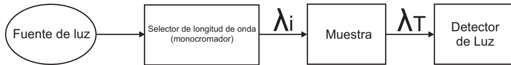
Figura 2.11: Estructura de un espectrofotómetro. \lambda_i es la longitud incidente y \lambda_T es la longitud transmitida [19].
