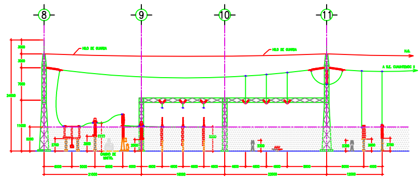
CORTE B-B
