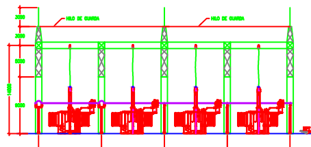
CORTE C-C
