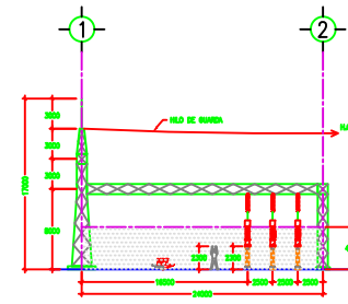
CORTE F-F
