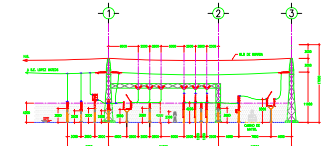
CORTE D-D
