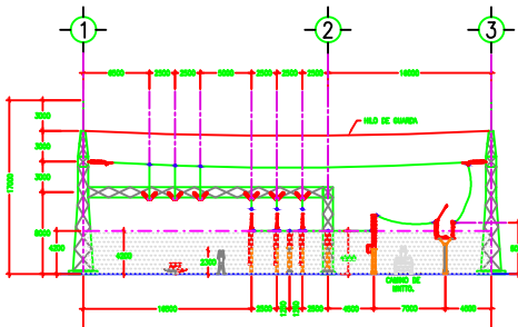
CORTE E-E
