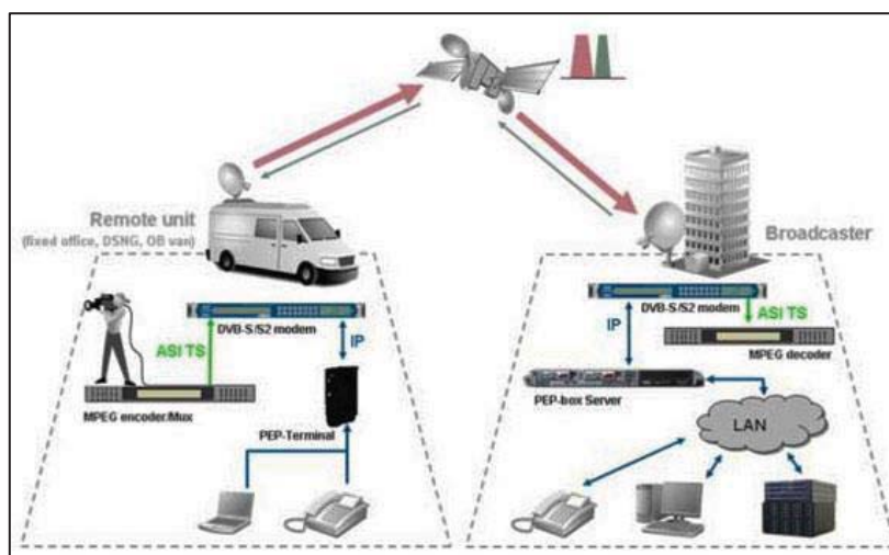
Fig. 3-2. Diagrama típico usando DVB-DSGN 69
