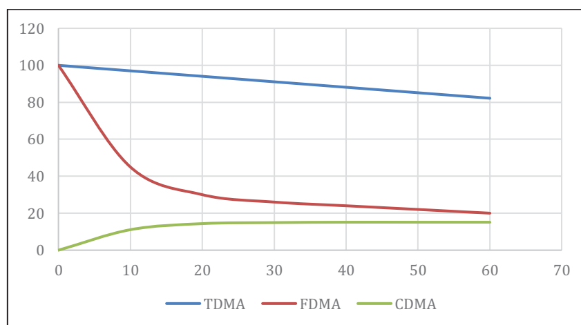
Fig. 1-9. Throughput vs Nº Estaciones CDMA.
