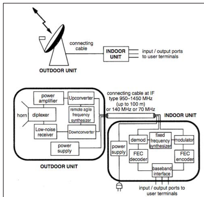
Fig. 2-2. Diagrama de una estación VSAT. [2]
