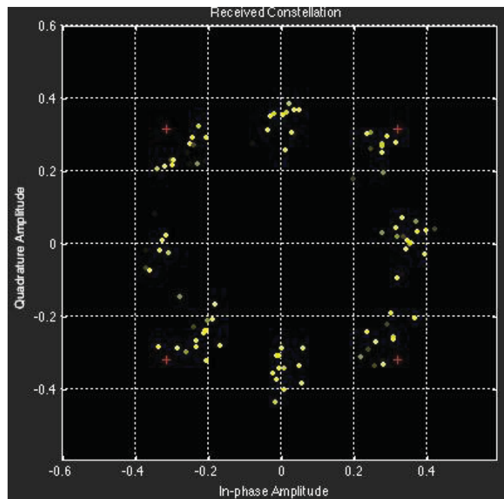
Fig. 4-7. Constelación recibida, 8PSK
