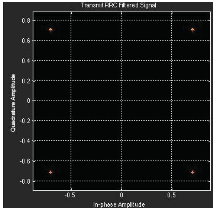
Fig. 4-2. Información en modo de constelación QPSK antes de pasar por el HPA.
