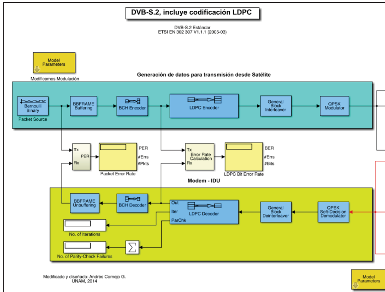
Fig. A2.-1. Modelo Simulink ®, DVB-S2 con codificación LDPC, codificador y decodificador.
