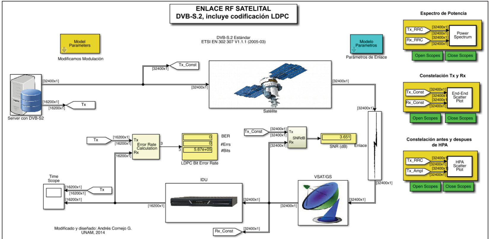
Fig. 4-1. Modelo simplificado de una transmisión satelital hacia una estación remota VSAT basado en el estándar DVB-S2.
