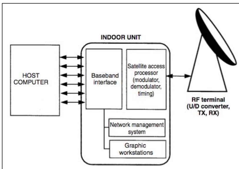
Fig. 2-8. Subsistemas de un HUB. [2]
