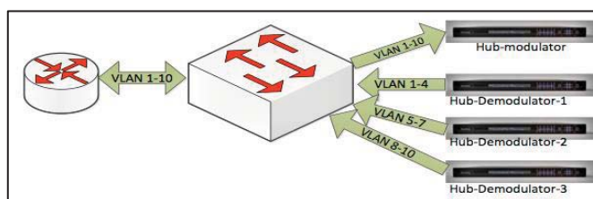
Fig. 3-11. Configuración de agregación Router – Switch, VLAN Networking. [22].
