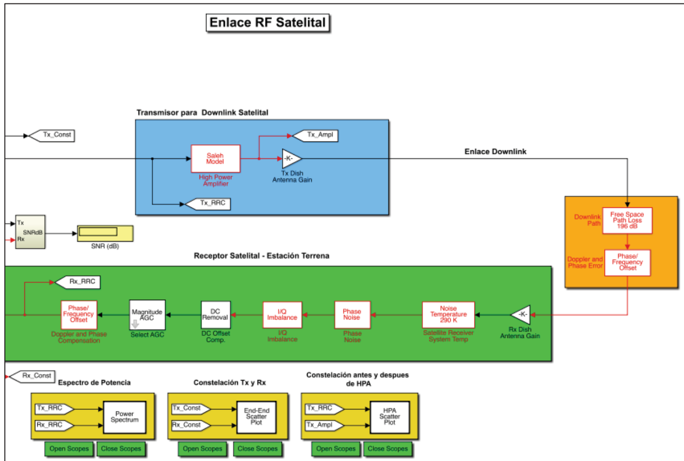
Fig. A2.-2 Modelo Simulink®, Enlace satelital, incluye Transmisor Satelital y el receptor VSAT + Enlace Espacial.
