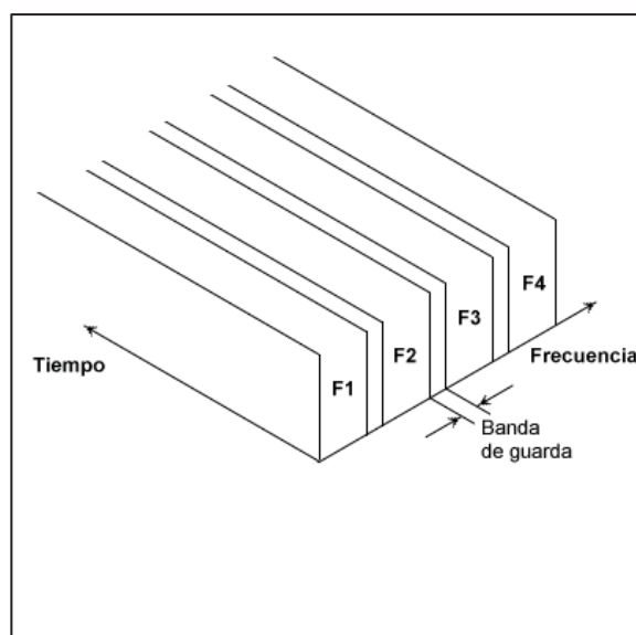
Fig. 1-3. Banda de guarda entre frecuencias en FDMA 4 .
