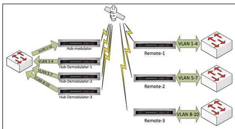
Fig. 3-10. Configuración Punto – Multipunto, con VLAN Networking. [22].
