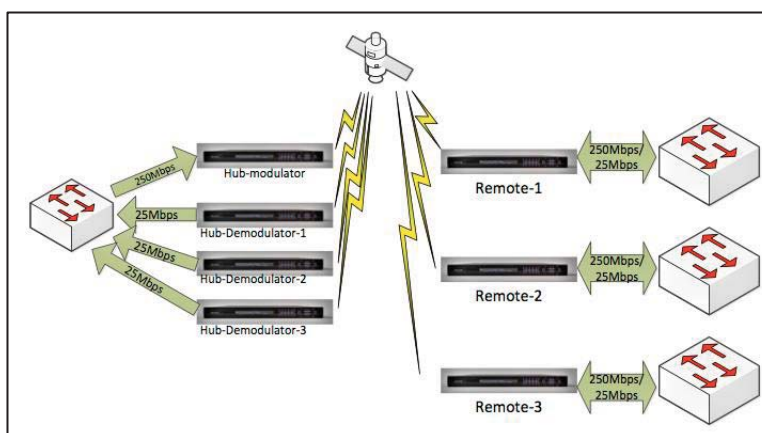
Fig. 3-9. Configuración Punto - Multipunto. [22].
