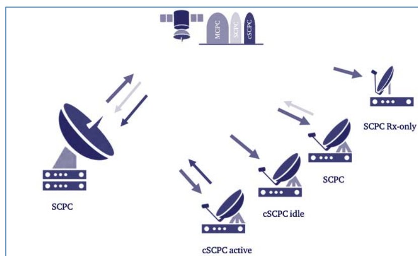
Fig. 1-5. Esquema básico de acceso SCPC y MCPC 16 .
