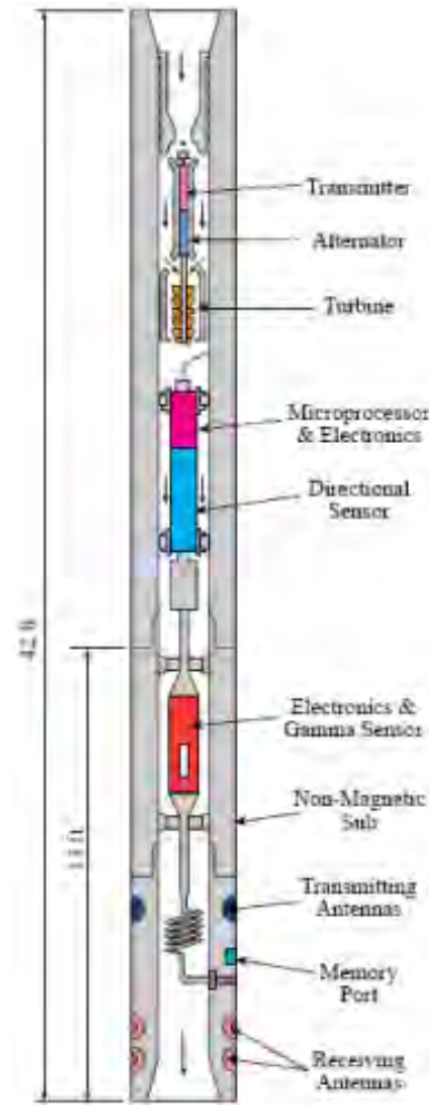
Fig.35 Herramienta MWD 104 .
