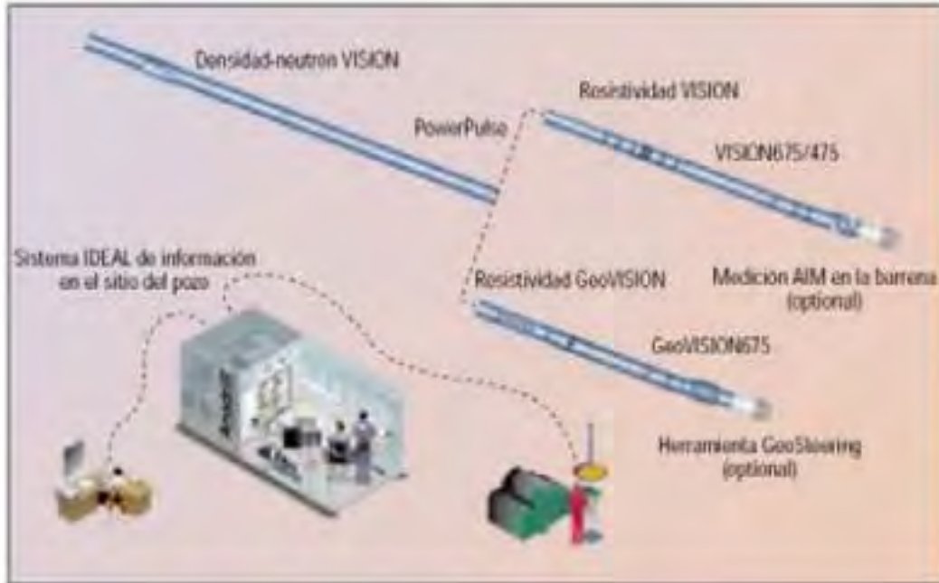
Fig.36 Herramienta LWD 106 .
