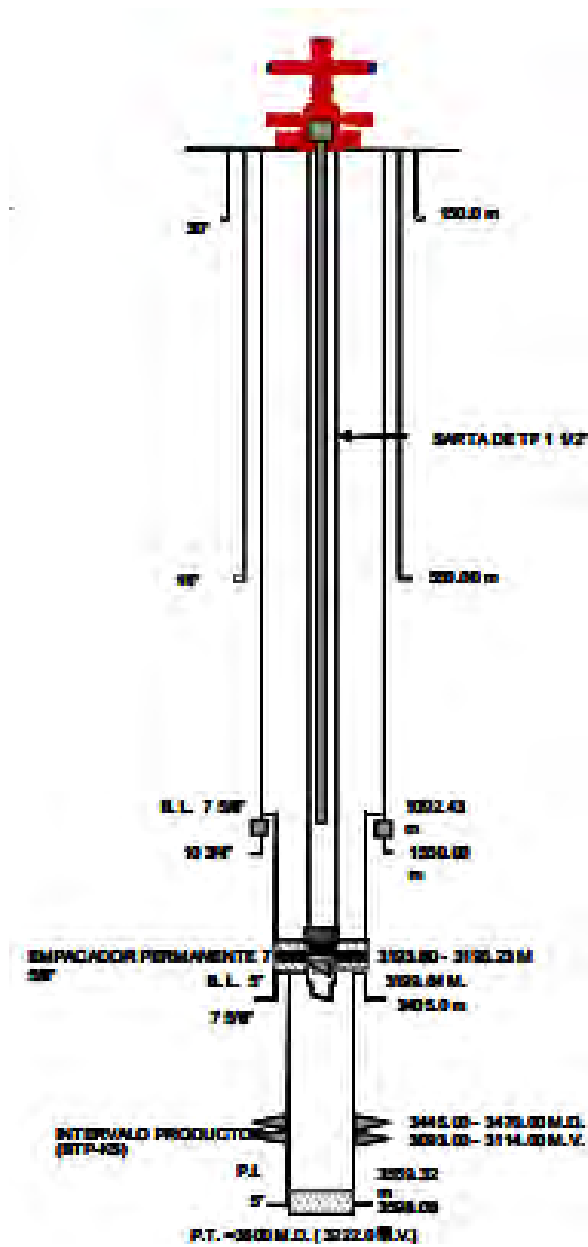
Fig.43 estado mecánico de un pozo 133 .
