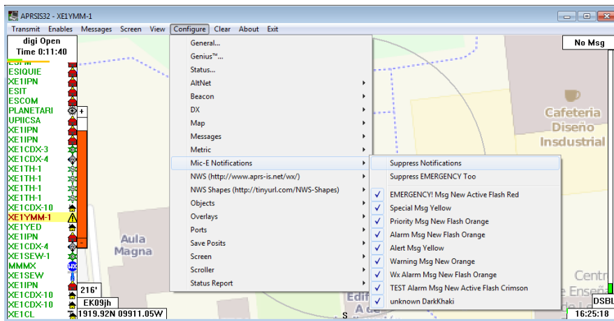
Figura 55. Mensajes Mic-E.
