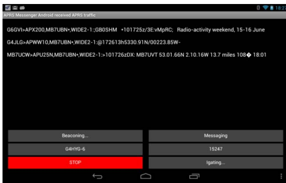
Figura 11. APRS Messenger.
