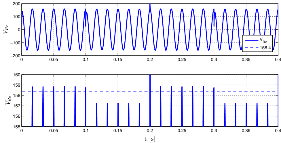
Figura 5.9: Tensión en la resistencia de carga durante el proceso de descarga con R_c variable.
