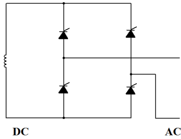
Figura 2.1: SMES basado en Tiristores.
