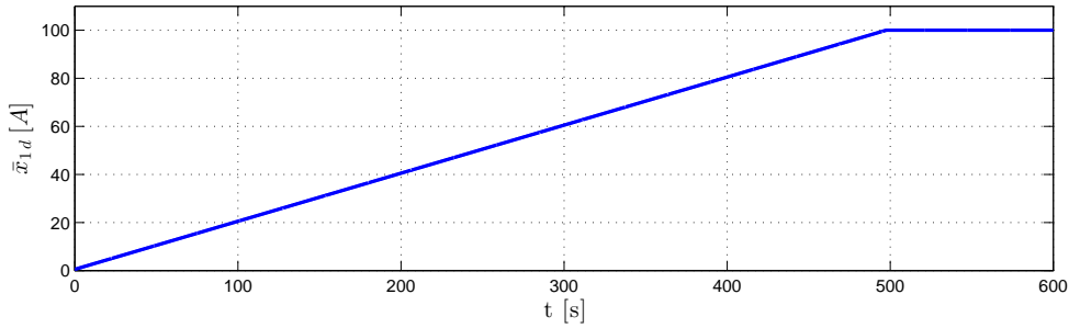
Figura 5.10: Perfil de carga para el inductor L_s .
