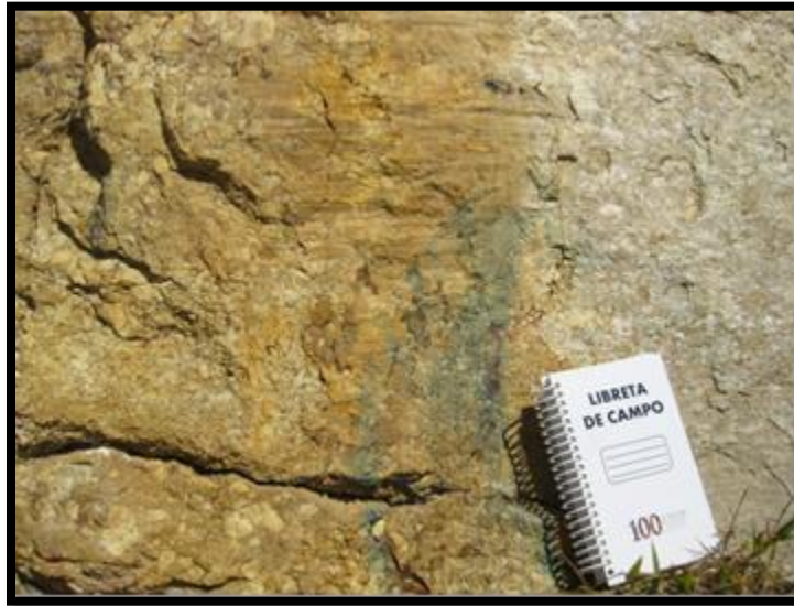
Figura 3.24. Estrías de falla lateral derecha, con dirección NW 24° con 74° de inclinación, ubicada en la parte frontal del anticlinal sobre el Conglomerado Cualac.
