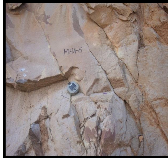
Figura 4.41. Muestra MHA-6. Tamaño de grano de arenas finas, con matriz menor a 15%. Se ubica al norte de Cuescomapa.
