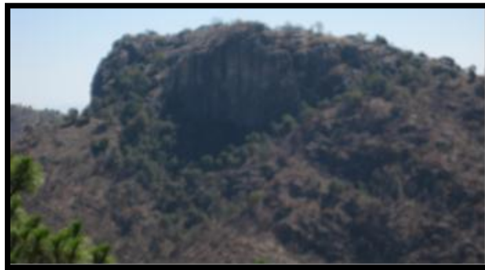
Figura 3.25. Localidad Tres Caminos, afectada por anticlinales y sinclinales de la orogenia Laramide.
