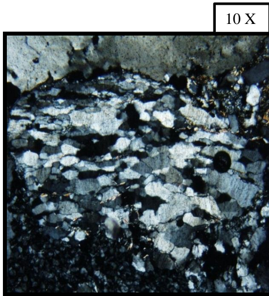
Figura 4.19. Muestra HM-9. Presenta cuarzo con extinción ondulante y un grado de metamorfismo.
