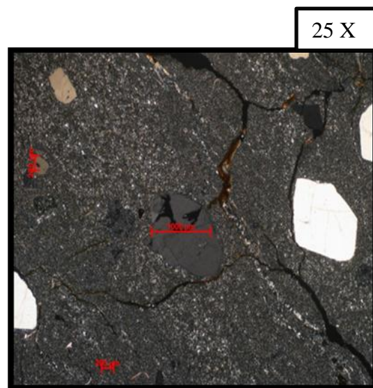
Figura 4.12. Muestra HM-2 La matriz en mayor a 15% los clastos son sub angulosos, presenta cuarzo 70% y feldespatos 30%. Se ubica en la localidad de La Carretera (CCC).
