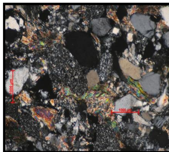
Figura 4.14. Muestra HM-4. Presenta cuarzo 80%, feldespato 15% y micas 15%, la matriz es menor a 15%. Se ubica en la localidad de La Carretera (CCC).
