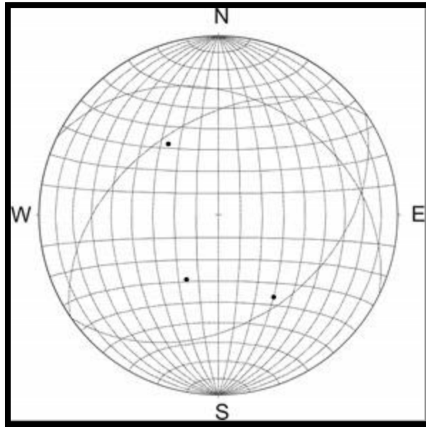
Figura 3.4. Planos de foliación de la secuencia clástica, provocado por metamorfismo.
