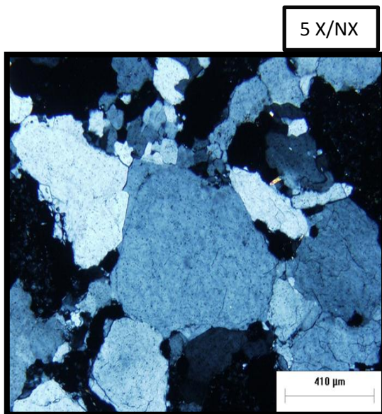
Figura 4.23. Muestra MHA-1. Presenta cuarzo policristalino en 90% y 10% de feldespato, en algunas secciones se presenta el cuarzo fragmentado producto del metamorfismo y en menor cantidad fragmentos de esquisto. Los bordes del cuarzo en algunas partes se presentan en forma onduladas.
