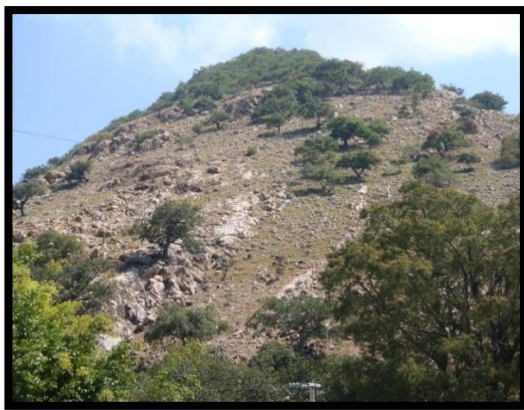
Figura 2.8. Conglomerado de fragmentos de cuarzo, ubicado al sureste de Cualac, Guerrero.
