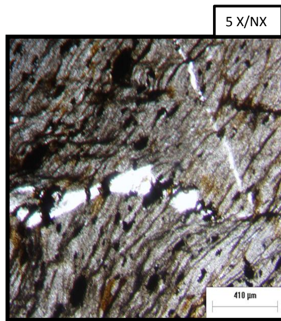
Figura 4.22. Muestra HM-12 (Complejo Acatlán). Esta roca está constituida por cristales con un tamaño de grano tan pequeño que hacen difícil su identificación, presenta una estructura foliada, con bandeamiento de color marrón, de gris a blanco y algunas intercalaciones de óxido de hierro, la mayor parte está compuesta por cuarzo muy fino. Presenta propiedades anisotrópicas con textura lepidoblastica, en algunas zonas se observa cuarzo microcristalino y vetas de cuarzo. Se nombró Filita.
