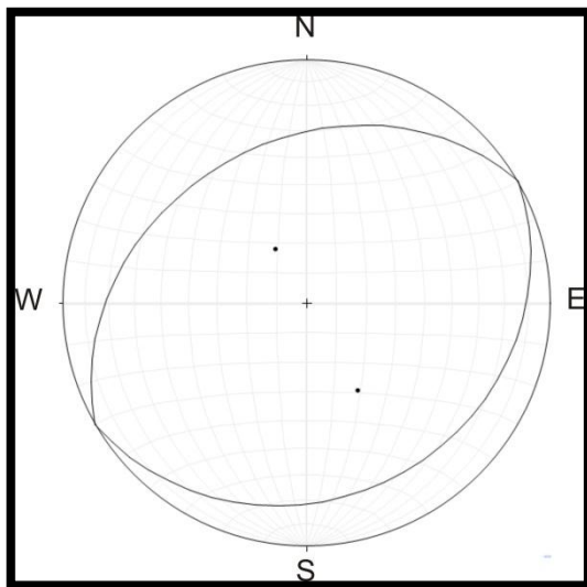
Figura 3.18. Flancos: 240^\circ/34^\circ y 60^\circ/21^\circ de un pliegue en lutitas, ubicado al norte de Tres Caminos.
