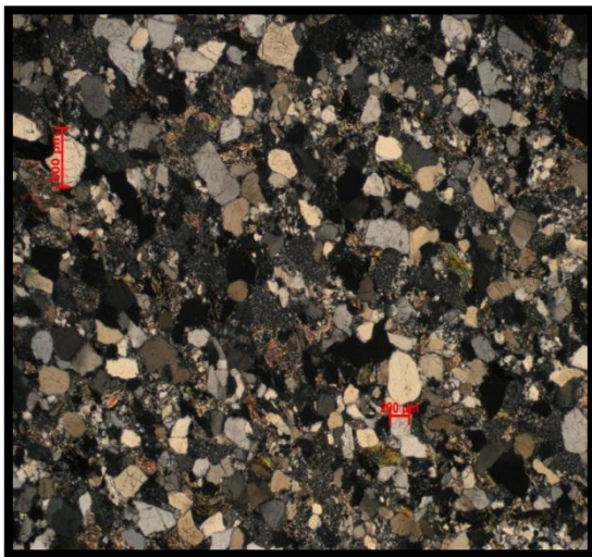
Figura 4.13. Muestra HM-3. Presenta cuarzo 80%, feldespatos 10% y micas 10%, la matriz es menor a 15% algunos cuarzos presentan extinción ondulante. Se ubica en la localidad de La Carretera (CCC).
