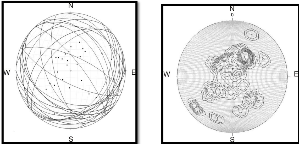
Figura 3.7. Proyección de los planos de estratificación con sus respectivos polos (izquierda) y la densidad de los polos (derecha).
