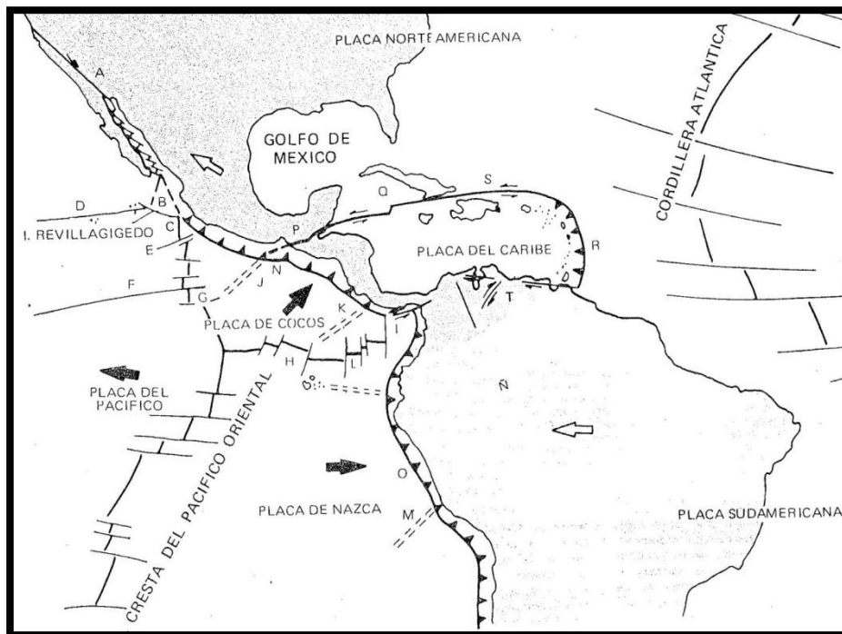
Figura 5.2. Rasgos tectónicos (tomada de Demant, 1978)
