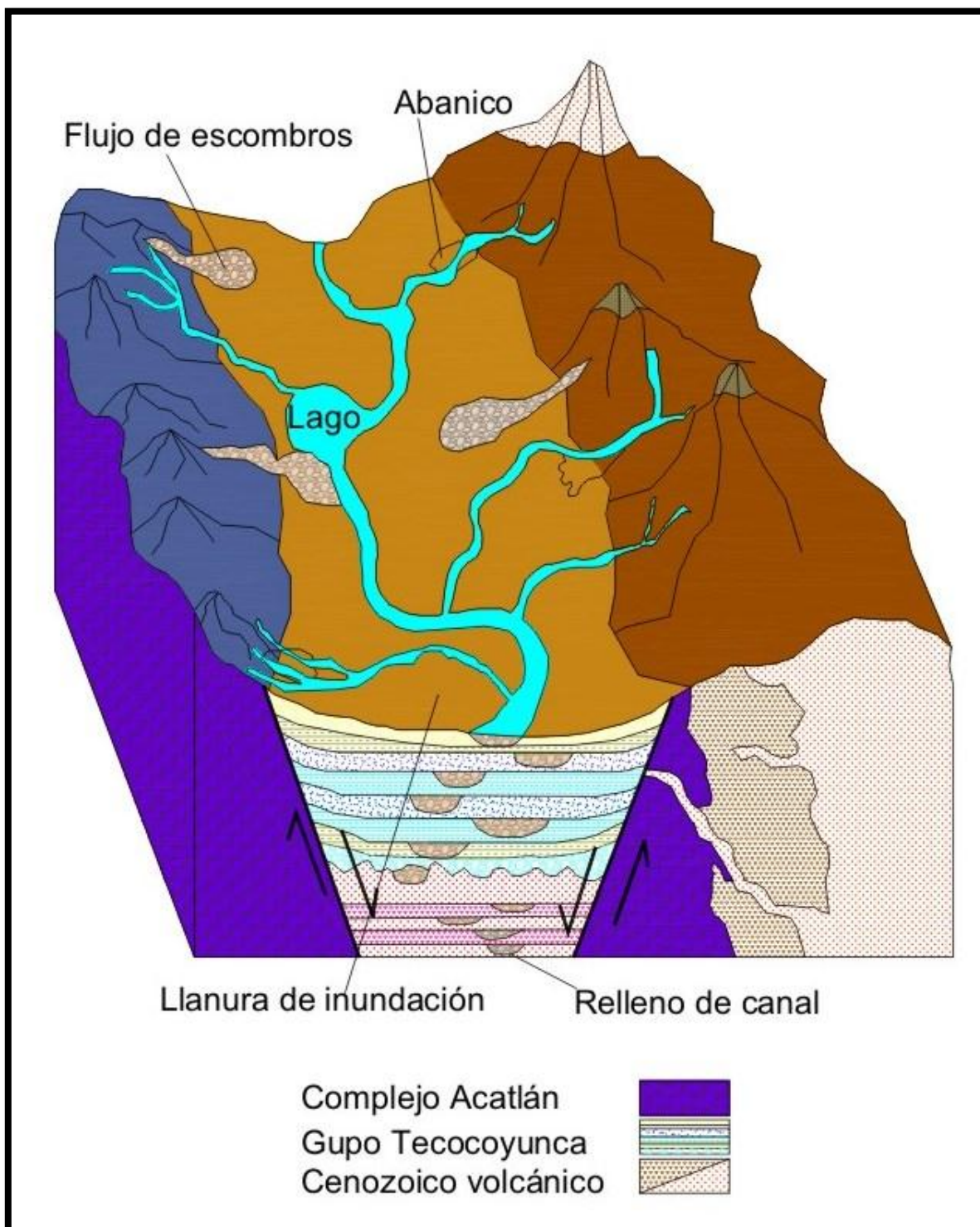
Figura 4.42. Modelo de reconstrucción paleoambiental del Jurásico-Medio-Inferior en los alrededores del poblado Tres Caminos. Al noreste del estado de Guerrero.
