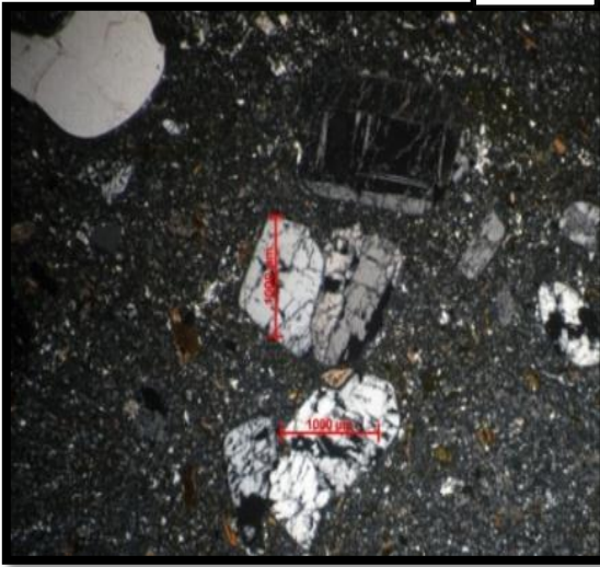
Figura 4.15. Muestra HM-5. Presenta cuarzo 20%, plagioclasas 40%, feldespato 20% y micas 20%. Se ubica en la localidad de La Carretera (CCC).
