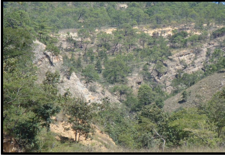
Figura 4.28. Fotografía de la Barranca (localidad CCB) ubicada al oeste del poblado Tres Caminos.
