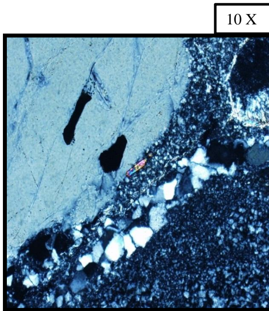
Figura 4.21. Muestra HM-11 Se observa matriz de cuarzo criptocristalino, con vetillas de cuarzo, presenta cuarzo 40%, feldespato en 10% y fragmentos de roca en 50%, en el centro de la fotografía se observa un zircón.
