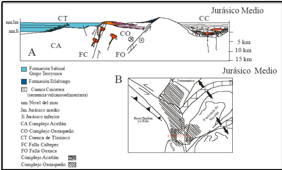
Figura 3.1. Representación del Jurásico en México.
