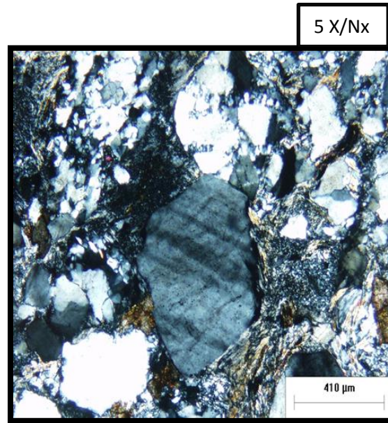
Figura 4.20. Muestra HM-10. Presenta feldespato 20 % y cuarzo 80 % policristalino y microcristalino, en algunas zonas se observan micas alteradas de color marrón y presenta zirrones en muy poca proporción. El feldespato presenta maclas polisintéticas.
