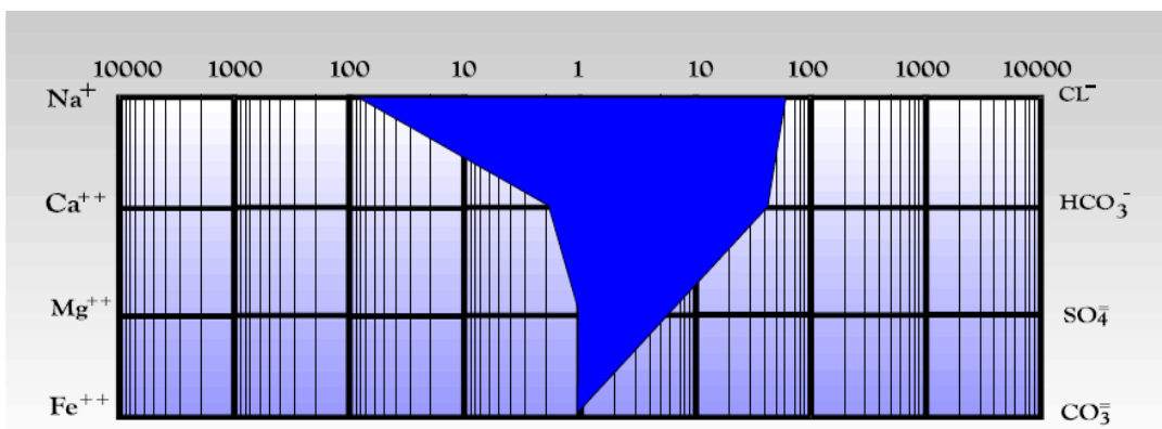
Fig. 3.2 . Grafico de Stiff. Escala logarítmica
