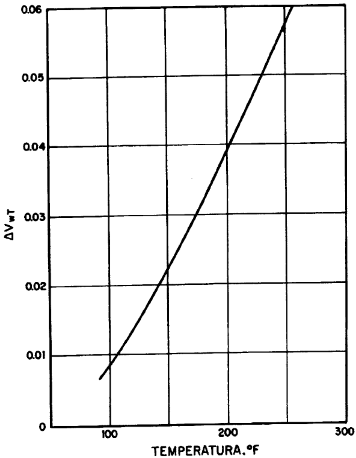
Fig.2.7 \Delta V_{wT} como función de la temperatura del yacimiento
