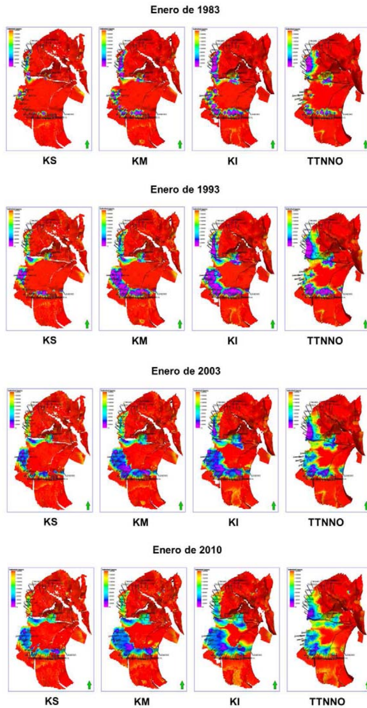
Figura 5.13. Distribución de la salinidad del agua inyectada en el yacimiento a lo largo del espacio y el tiempo.
