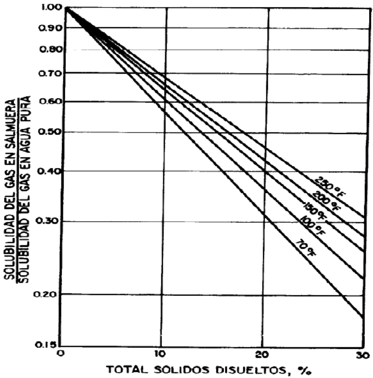
Fig.2.5 Efecto de la salinidad sobre la solubilidad del gas natural en agua
