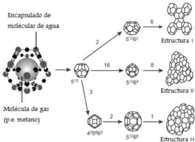
Fig 2.16 Estructura de los hidratos.
