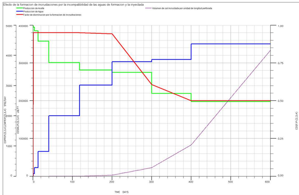
Figura 5.15. Efecto de la formación de incrustaciones en la productividad de un pozo productor.
