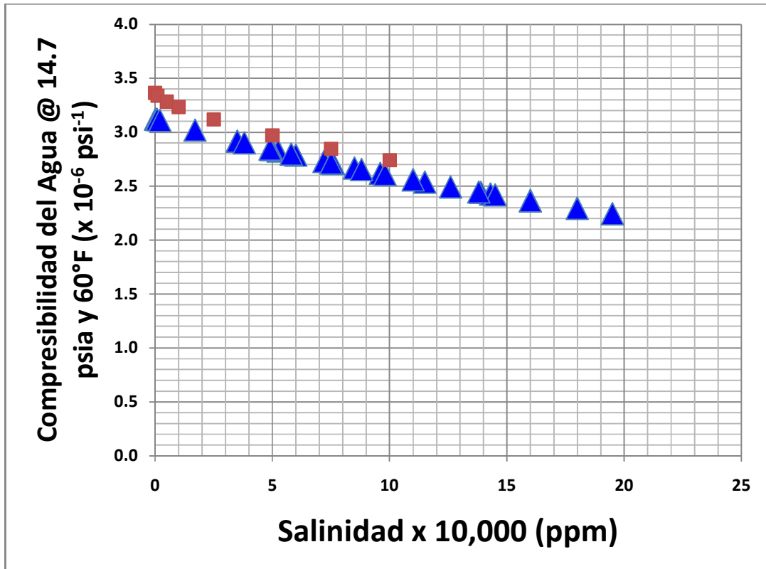
Figura 5.4 – Correlación de la salinidad vs compresibilidad del agua.
