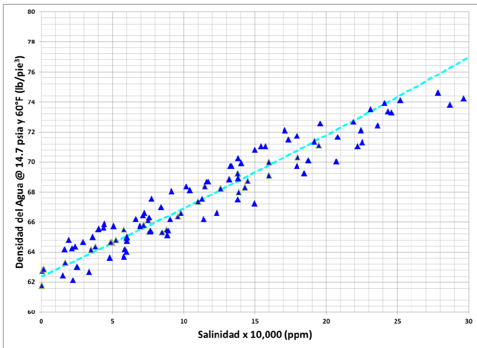
Figura 5.2 – Salinidad vs densidad del agua de diferentes muestras de agua de campos en México que pertenecen a la Región Sur.
