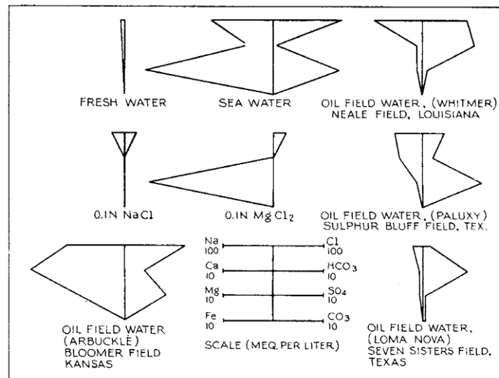
Figura 5.1 – Patrones comunes en la identificación de Aguas
