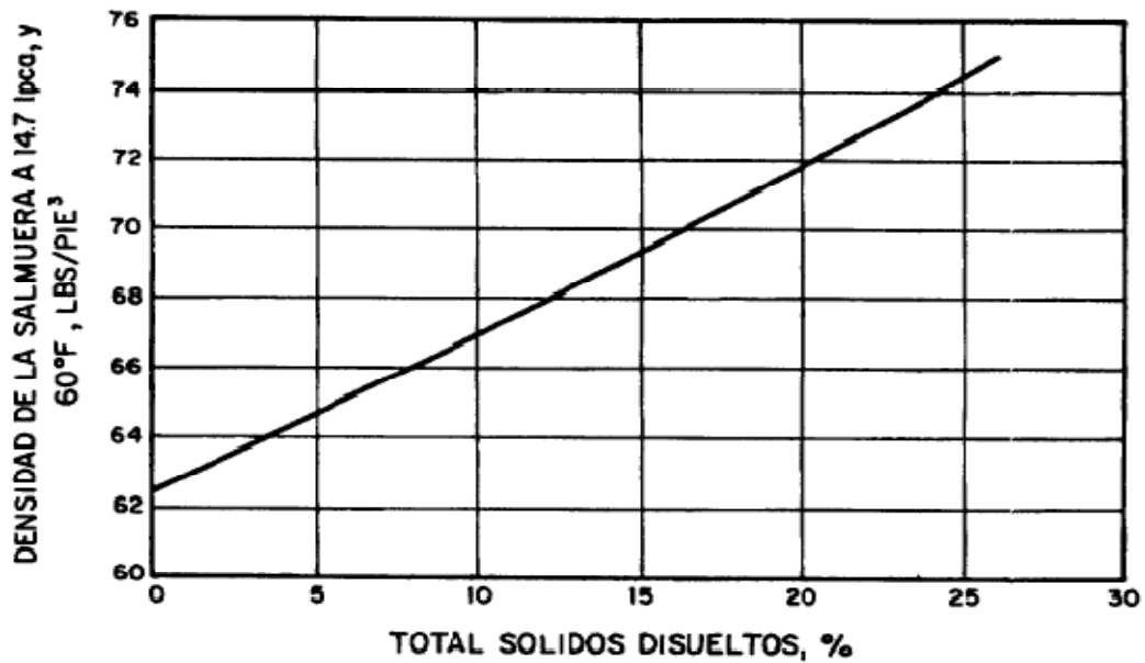
Fig. 2.14 Densidad de la salmuera en función del porcentaje Total de sólidos disueltos
