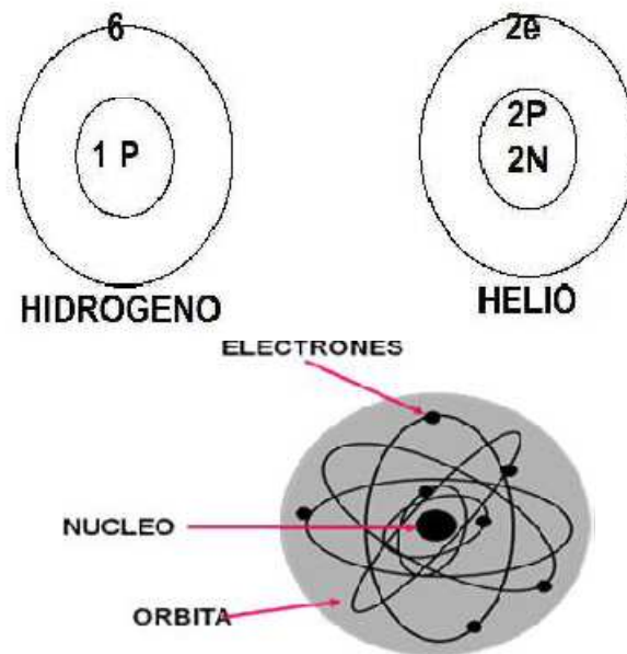
Fig.A.2 Átomo de Hidrogeno, helio y su estructura
