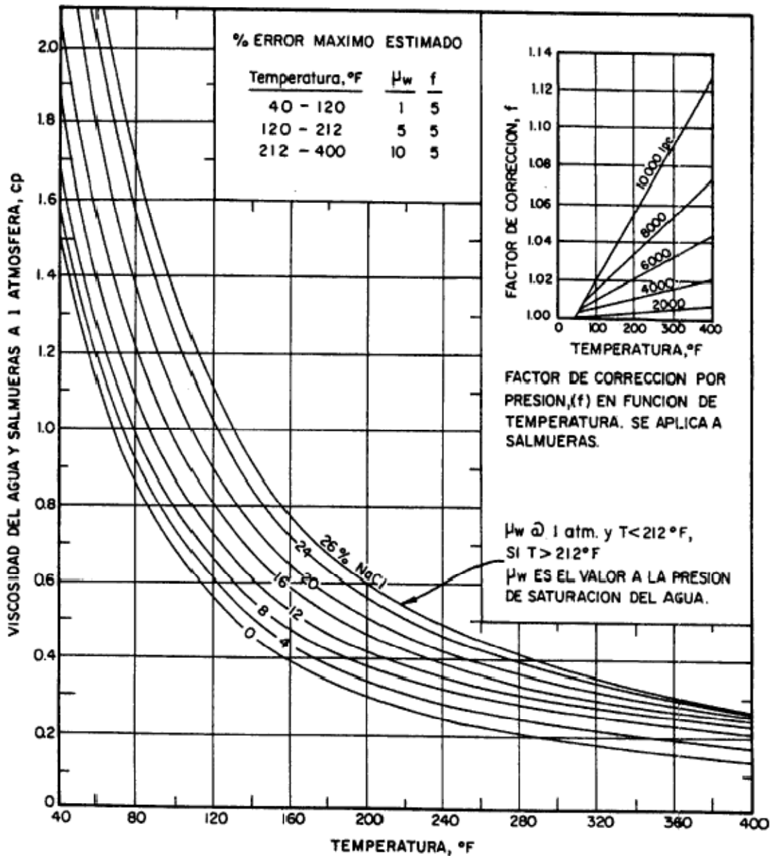
Fig.2.12 Viscosidad del agua a una at. En función de temperatura y salinidad, Para otras presiones seguir la corrección indicada
