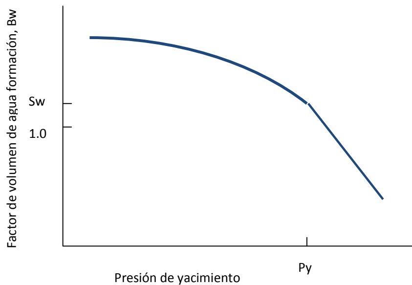
Fig.2.3 Grafica típica del Factor de Volumen de Agua de Formación contra la Presión a Temperatura constante.
