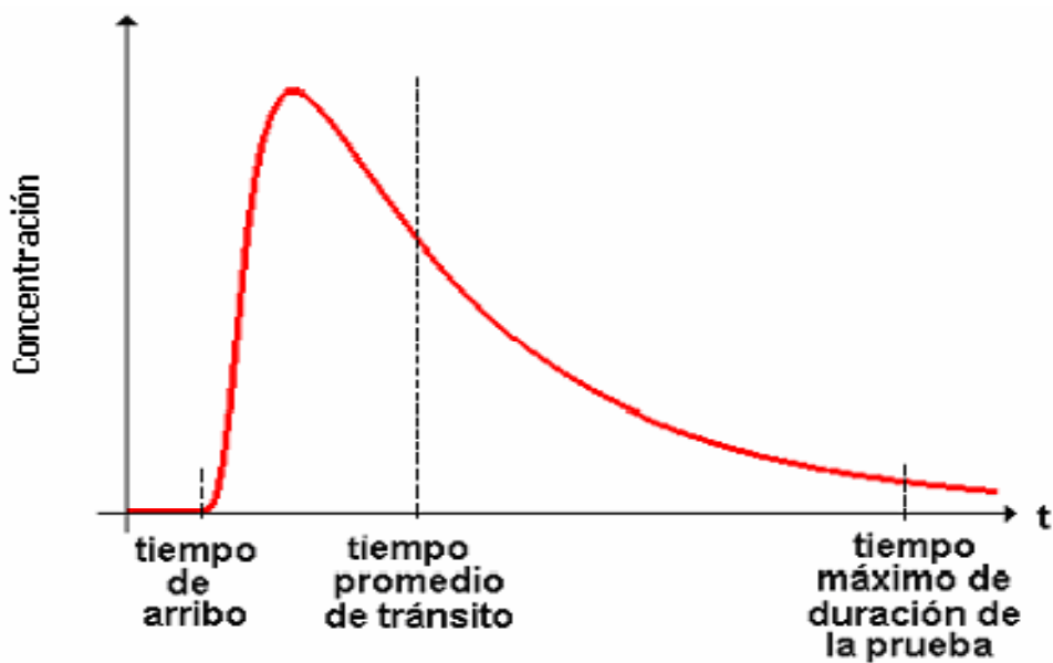
Fig.4.3 Curva hipotética de respuesta de trazador en un pozo monitorizado.
