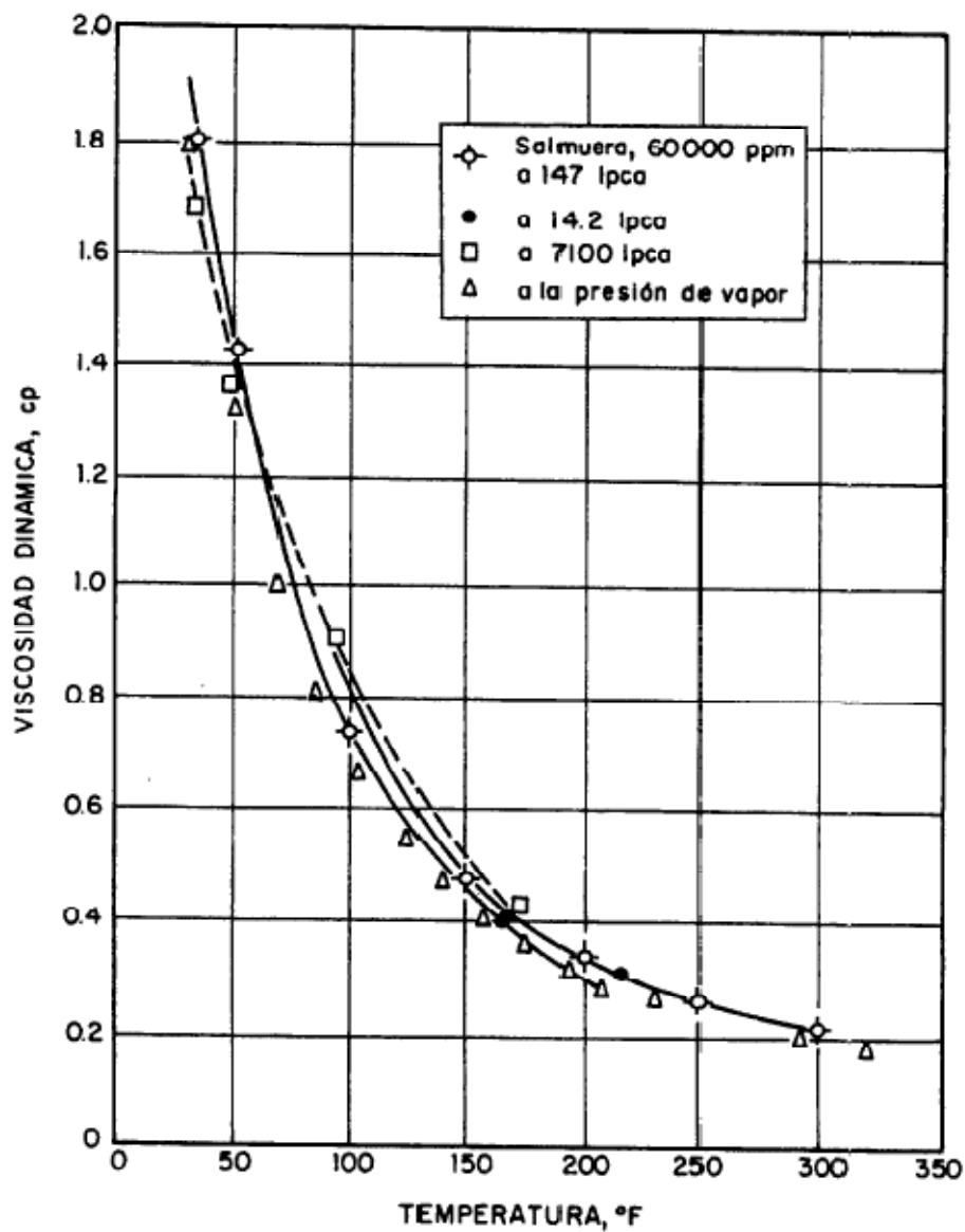
Fig.2.11 Viscosidad del agua en función de temperatura para varias presiones
