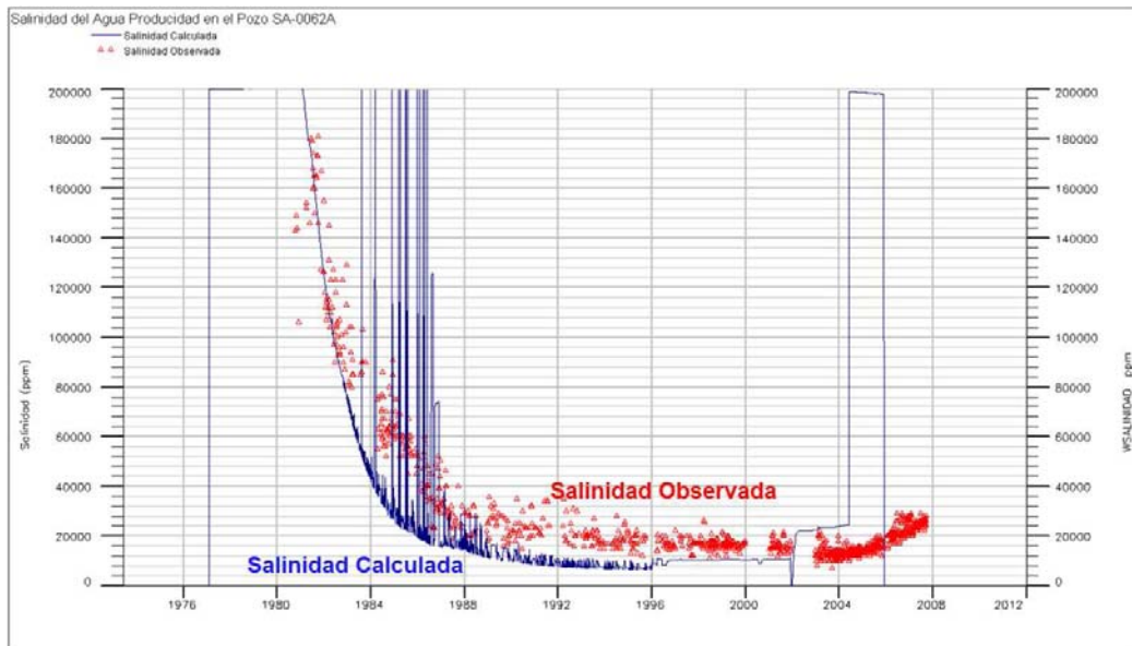
Figura 5.12. Ajuste histórico del salinidad del agua producida en un pozo, del campo en estudio.
