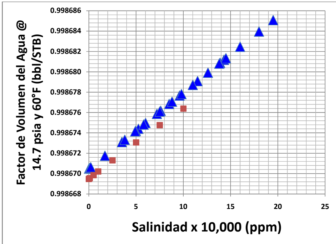
Figura 5.5 – Correlación de salinidad vs factor de volumen del agua
