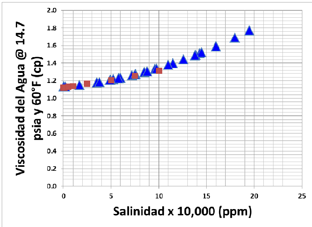
Figura 5.3 – Correlación de la salinidad vs viscosidad del agua.
