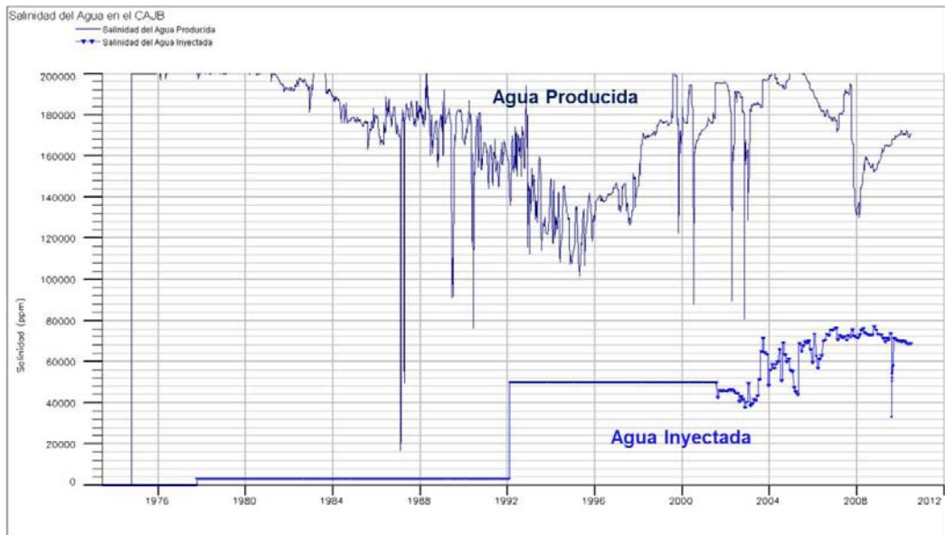
Figura 5.11. Salinidades del agua de formación y el agua de inyección del campo en estudio.
