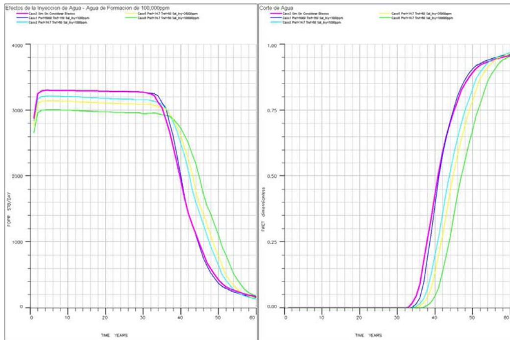
Figura 5.10. Resultados de diversos casos de simulación, variando las propiedades PVT del agua de formación y el agua de inyección.
