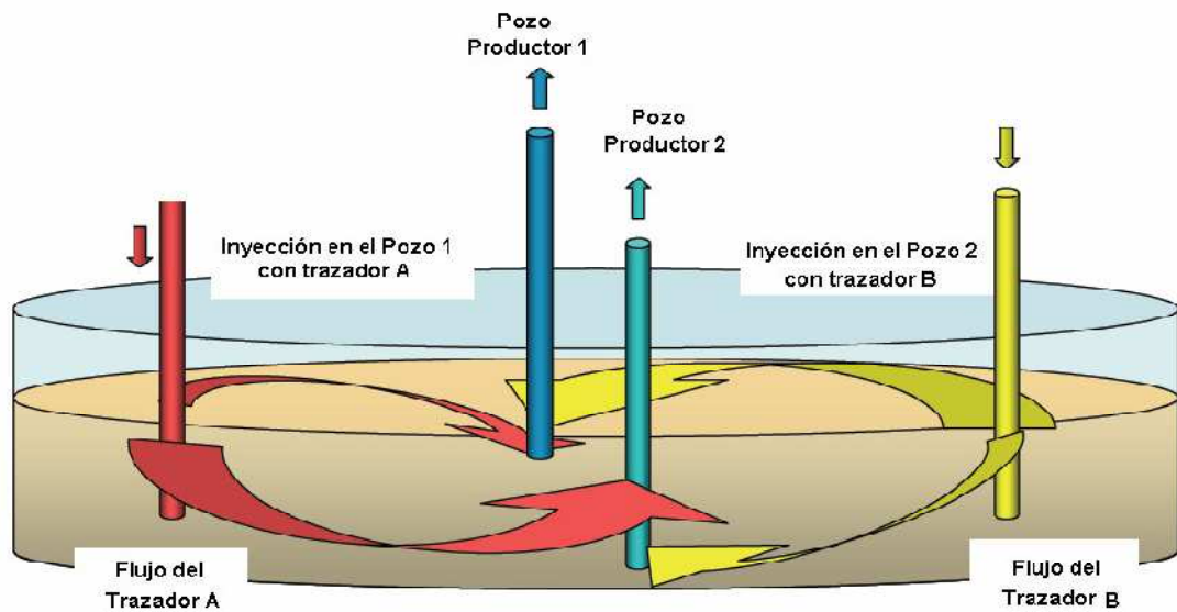
Fig.4.2 Esquema de una prueba de inyección de trazadores.
